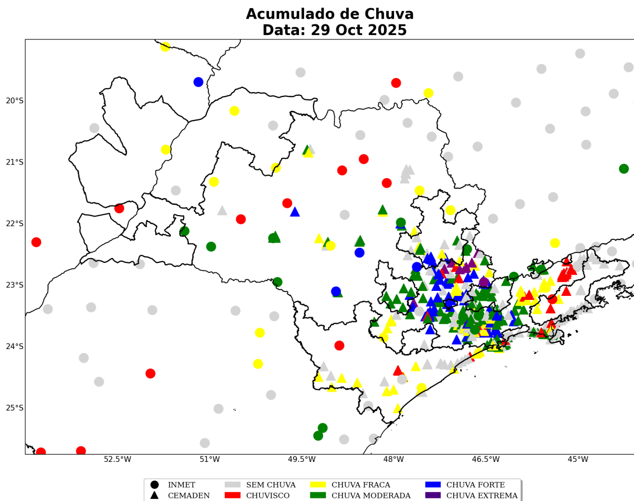
Figura 13: Acumulado diário de precipitação sobre a área de concessão da Neoenergia Elektro para o dia 29 de Outubro, baseado nas estações meteorológicas do INMET e CEMADEN.
