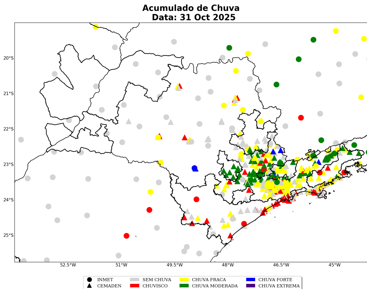
Figura 15: Acumulado diário de precipitação sobre a área de concessão da Neoenergia Elektro para o dia 31 de Outubro, baseado nas estações meteorológicas do INMET e CEMADEN.
