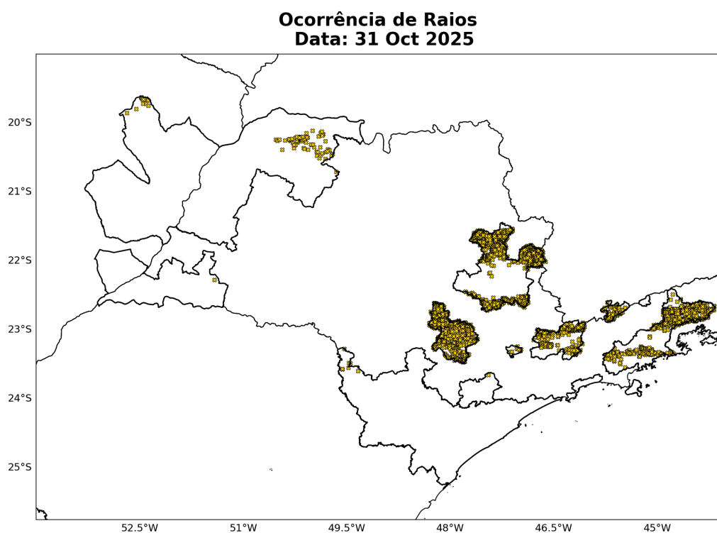
Figura 9: Ocorrências de descargas atmosféricas nuvem-solo detectadas pelo sistema Earth Networks para o dia 31 de Outubro sobre a área de concessão da Neoenergia Elektro.
