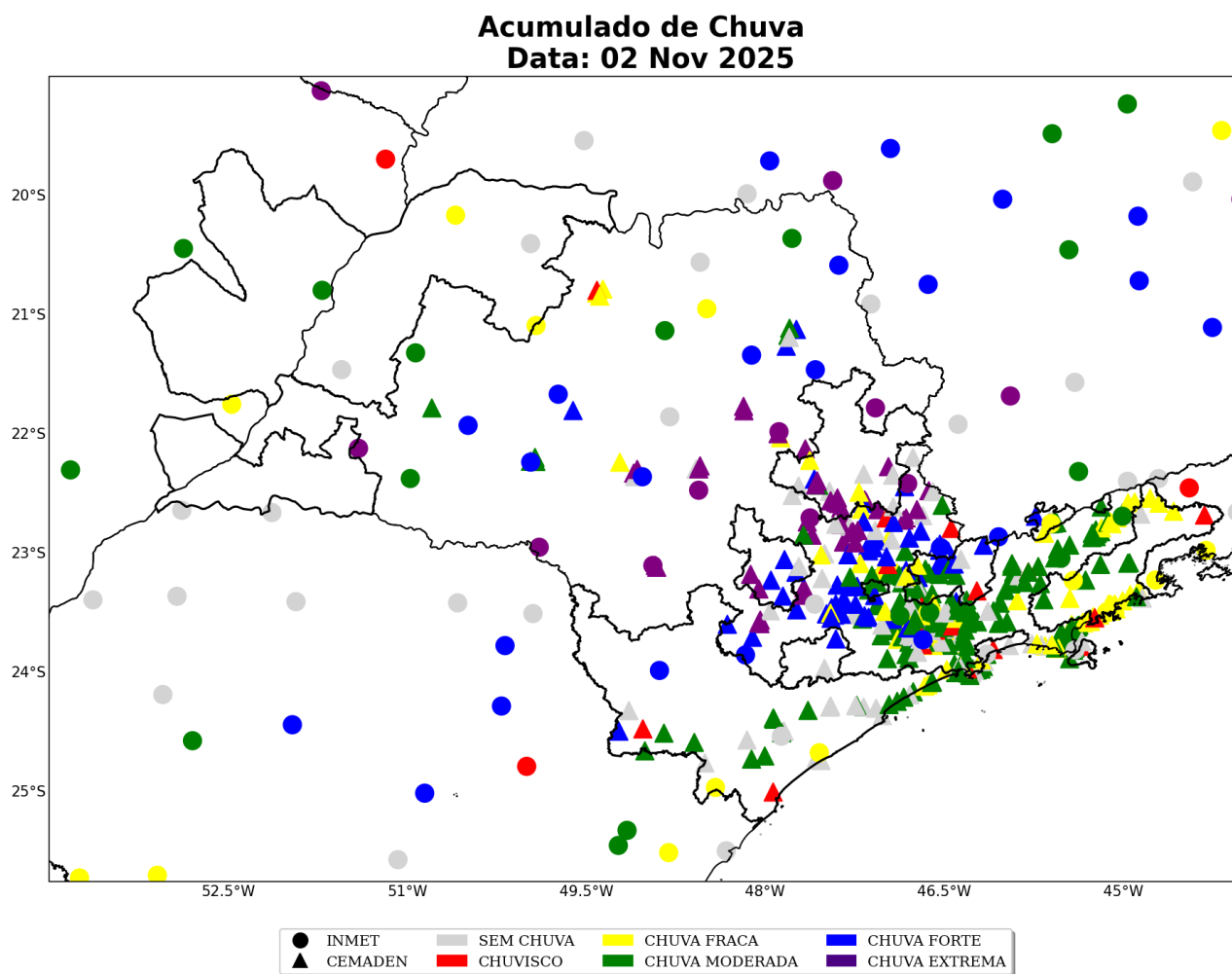
Figura 17: Acumulado diário de precipitação sobre a área de concessão da Neoenergia Elektro para o dia 02 de Novembro, baseado nas estações meteorológicas do INMET e CEMADEN.
