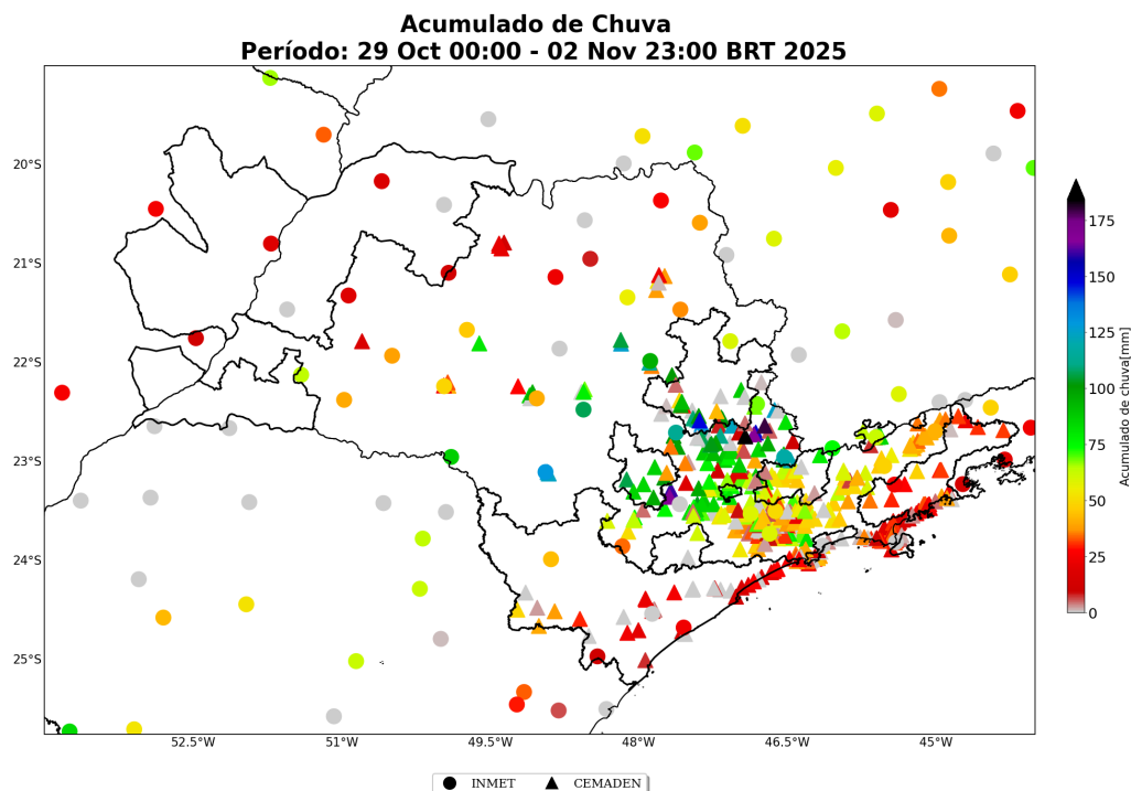
Figura 18: Acumulado de precipitação sobre a área de concessão da Neoenergia Elektro para o período do evento (dias 29 de Outubro a 02 de Novembro de 2025), baseado nas estações meteorológicas do INMET e CEMADEN.
