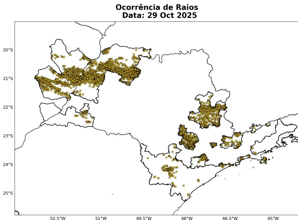
Figura 7: Ocorrências de descargas atmosféricas nuvem-solo detectadas pelo sistema Earth Networks para o dia 29 de Outubro sobre a área de concessão da Neoenergia Elektro.
