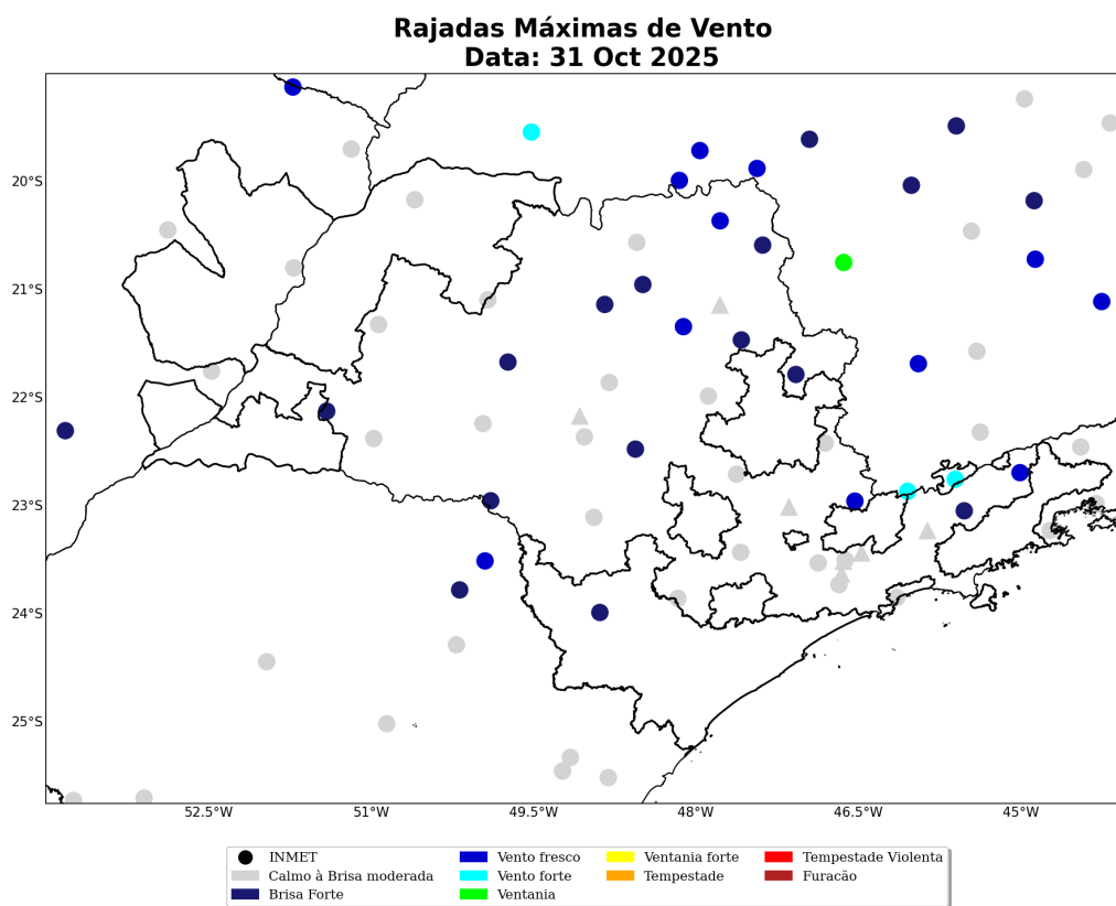
Figura 21: Máxima rajada de vento diária sobre a área de concessão da Neoenergia Elektro para o dia 31 de Outubro, baseado nas estações meteorológicas do INMET.
