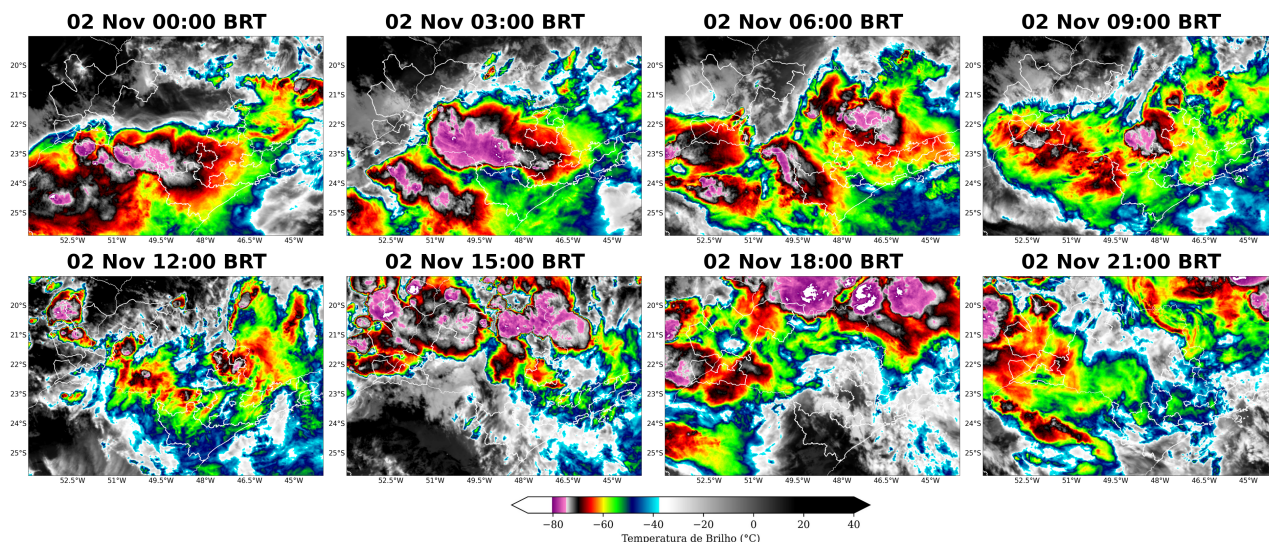
Figura 6: Imagens realçadas do satélite GOES-19 das 00 BRT até 21 BRT (a cada 3 horas) para o dia 02 de Novembro.
