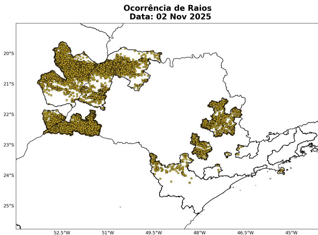
Figura 11: Ocorrências de descargas atmosféricas nuvem-solo detectadas pelo sistema Earth Networks para o dia 02 de Novembro sobre a área de concessão da Neoenergia Elektro.
