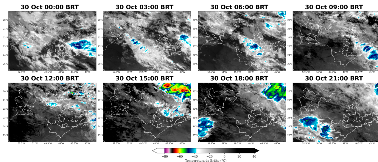
Figura 3: Imagens realçadas do satélite GOES-19 das 00 BRT até 21 BRT (a cada 3 horas) para o dia 30 de Outubro.
