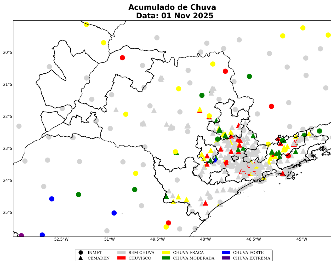
Figura 16: Acumulado diário de precipitação sobre a área de concessão da Neoenergia Elektro para o dia 01 de Novembro, baseado nas estações meteorológicas do INMET e CEMADEN.
