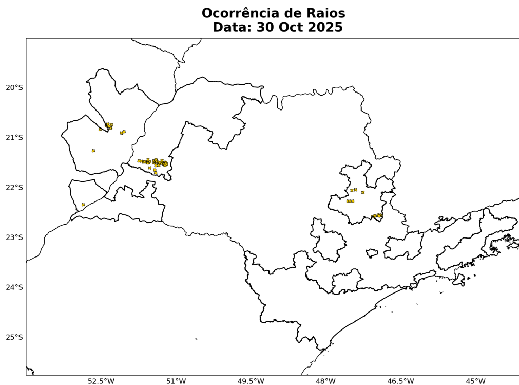
Figura 8: Ocorrências de descargas atmosféricas nuvem-solo detectadas pelo sistema Earth Networks para o dia 30 de Outubro sobre a área de concessão da Neoenergia Elektro.
