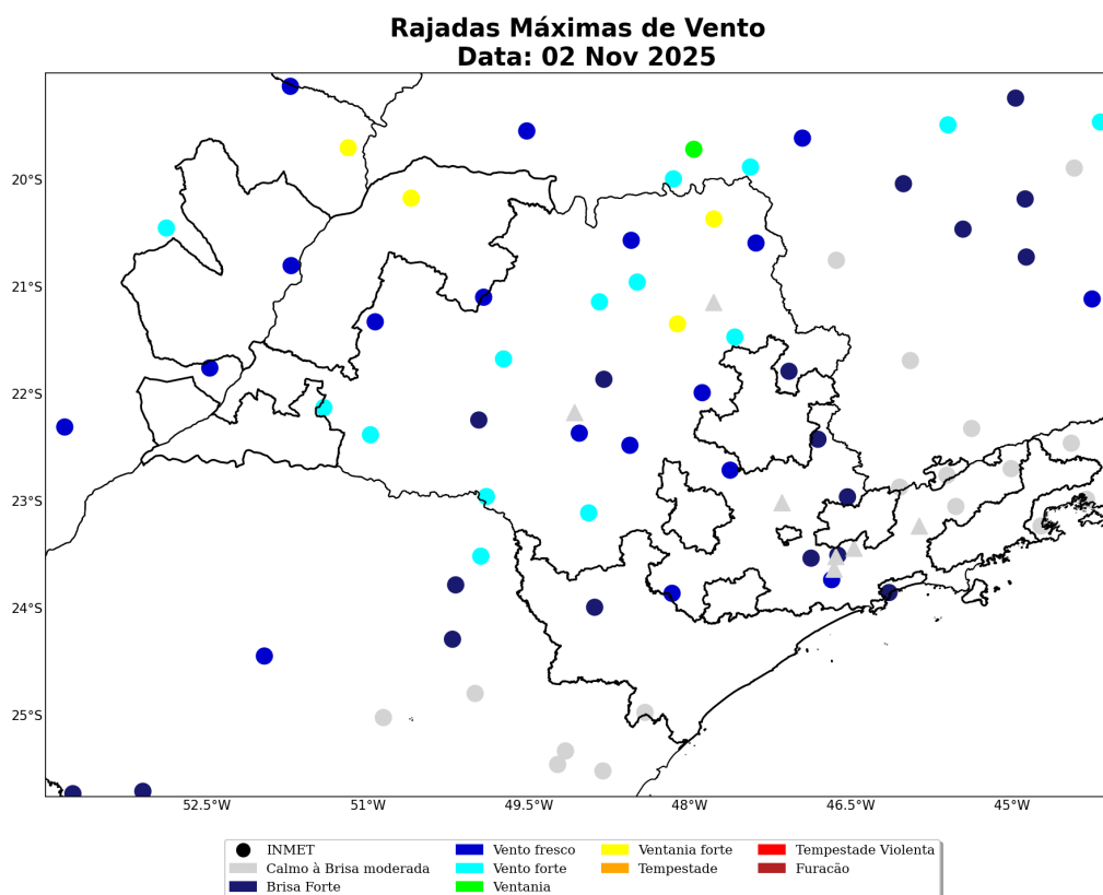
Figura 23: Máxima rajada de vento diária sobre a área de concessão da Neoenergia Elektro para o dia 02 de Novembro, baseado nas estações meteorológicas do INMET.
