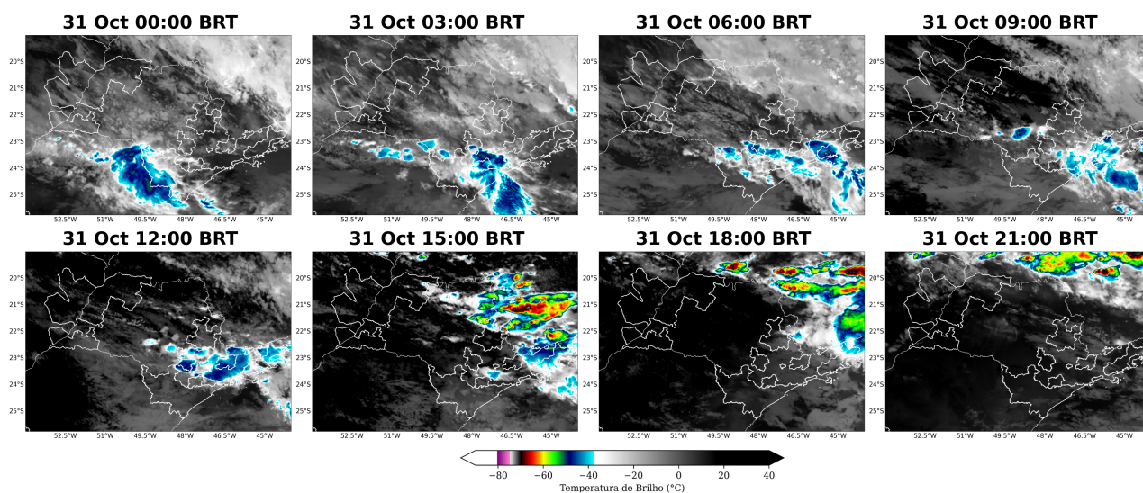
Figura 4: Imagens realçadas do satélite GOES-19 das 00 BRT até 21 BRT (a cada 3 horas) para o dia 31 de Outubro.
