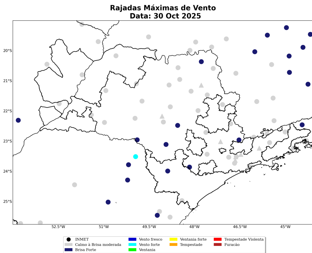
Figura 20: Máxima rajada de vento diária sobre a área de concessão da Neoenergia Elektro para o dia 30 de Outubro, baseado nas estações meteorológicas do INMET.
