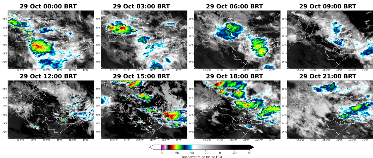
Figura 2: Imagens realçadas do satélite GOES-19 das 00 BRT até 21 BRT (a cada 3 horas) para o dia 29 de Outubro.
