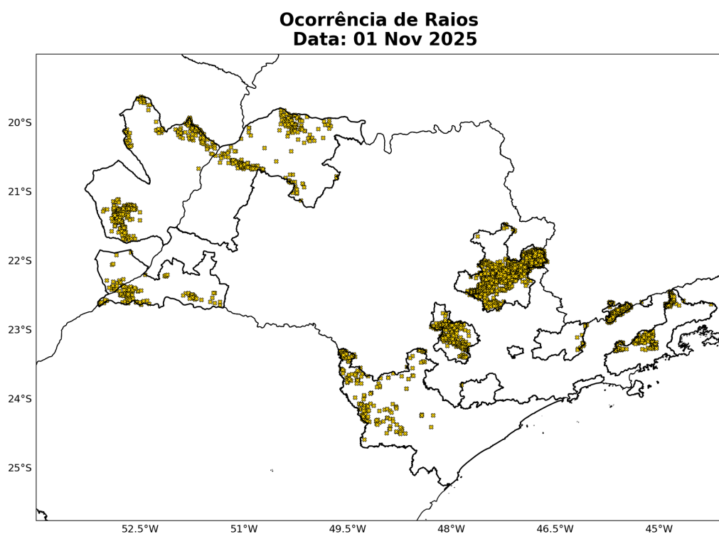
Figura 10: Ocorrências de descargas atmosféricas nuvem-solo detectadas pelo sistema Earth Networks para o dia 01 de Novembro sobre a área de concessão da Neoenergia Elektro.
