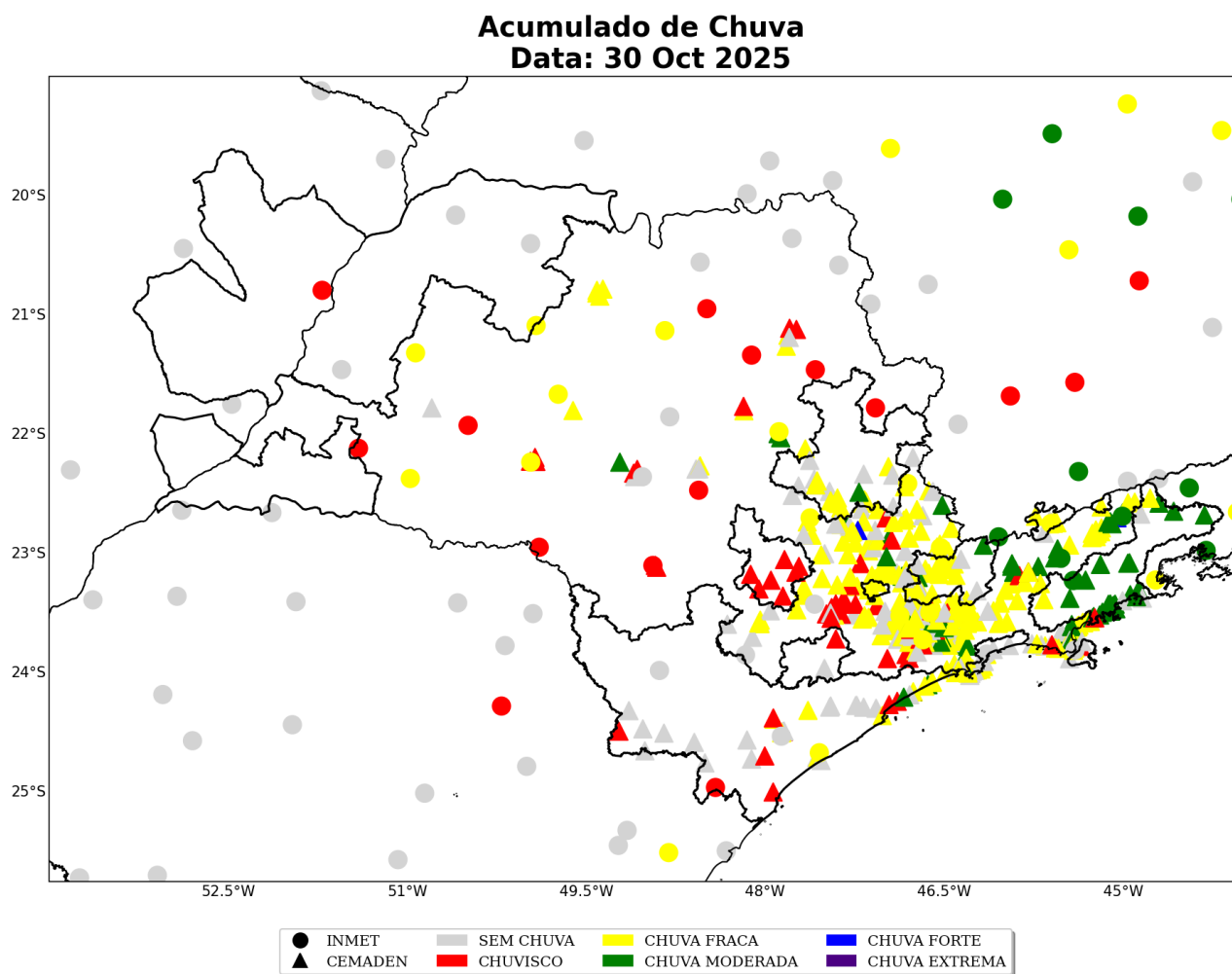
Figura 14: Acumulado diário de precipitação sobre a área de concessão da Neoenergia Elektro para o dia 30 de Outubro, baseado nas estações meteorológicas do INMET e CEMADEN.
