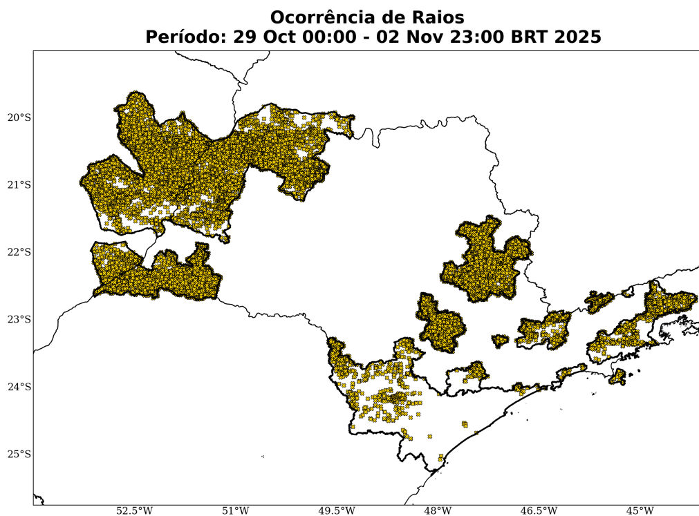
Figura 12: Ocorrências de descargas atmosféricas nuvem-solo detectadas pelo sistema Earth Networks para o período de 29 de Outubro a 02 de Novembro de 2025 sobre a área de concessão da Neoenergia Elektro.
