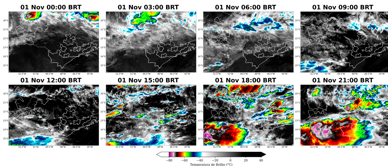
Figura 5: Imagens realçadas do satélite GOES-19 das 00 BRT até 21 BRT (a cada 3 horas) para o dia 01 de Novembro.
