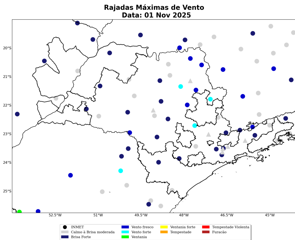
Figura 22: Máxima rajada de vento diária sobre a área de concessão da Neoenergia Elektro para o dia 01 de Novembro, baseado nas estações meteorológicas do INMET.
