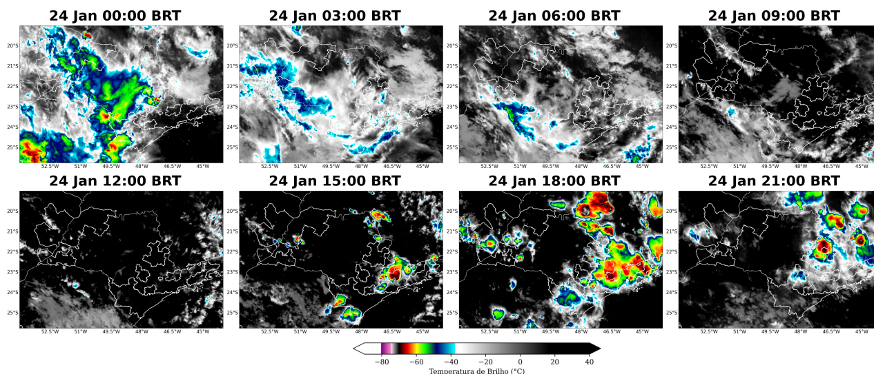
Figura 4: Imagens realçadas do satélite GOES-16 das 00 BRT até 21 BRT (a cada 3 horas) para o dia 24 janeiro.
