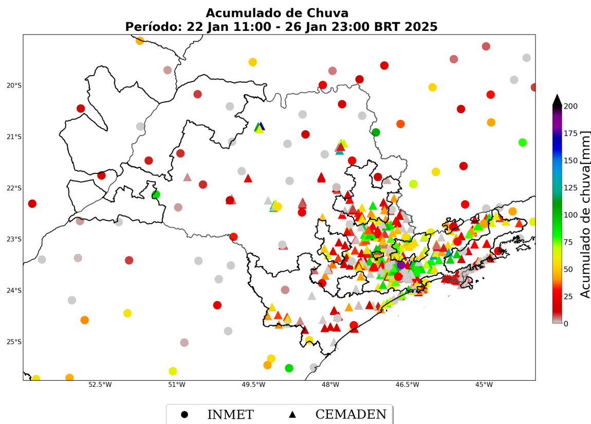
Figura 18: Acumulado de precipitação sobre a área de concessão da Neoenergia-Elektro para o período de 22 a 26 de janeiro de 2025 baseado nas estações meteorológicas do INMET e CEMADEN.
