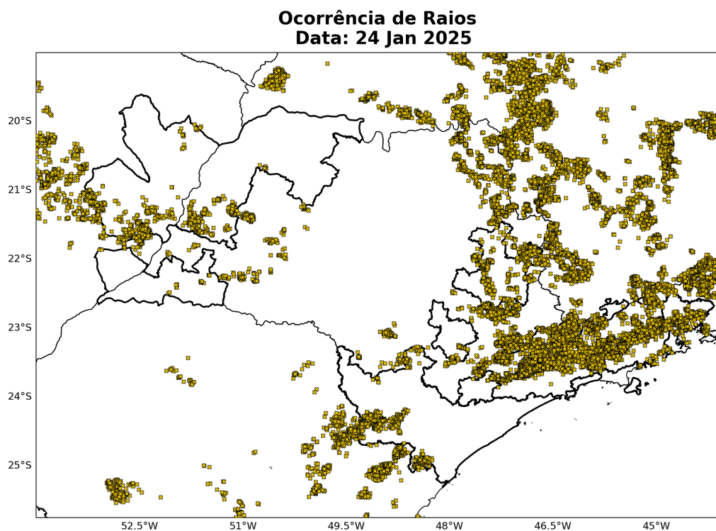
Figura 9: Ocorrências de descargas atmosféricas nuvem-solo detectadas pelo sistema Earth Networks para o dia 24 janeiro sobre a área de concessão da Neoenergia-Elektro.
