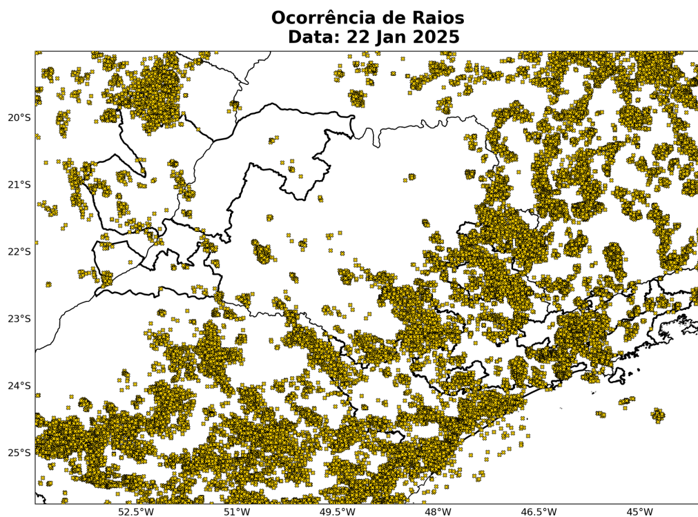
Figura 7: Ocorrências de descargas atmosféricas nuvem-solo detectadas pelo sistema Earth Networks para o dia 22 janeiro sobre a área de concessão da Neoenergia-Elektro.
