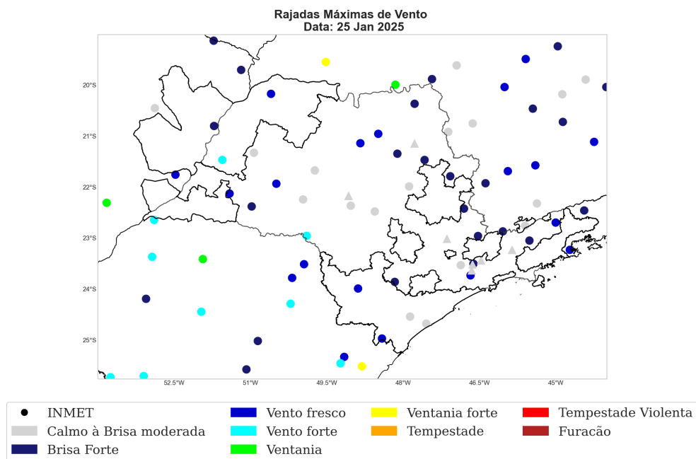
Figura 22: Máxima rajada de vento diária sobre a área de concessão da Neoenergia-Elektro para o dia 25 janeiro, baseado nas estações meteorológicas do INMET.
