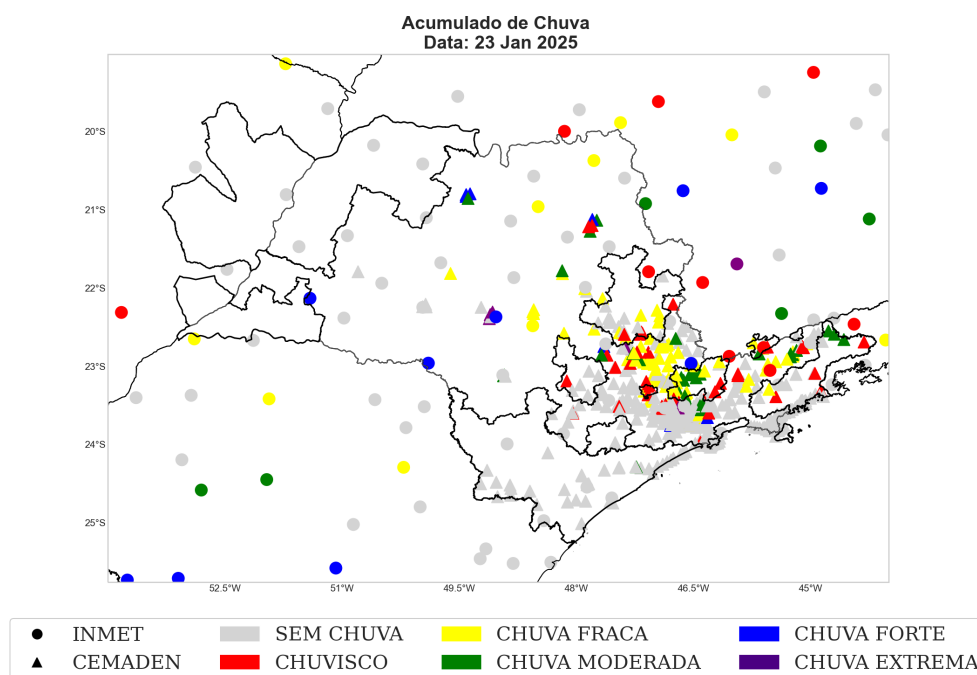
Figura 14: Acumulado de precipitação sobre a área de concessão da Neoenergia-Elektro para o dia 23 janeiro baseado nas estações meteorológicas do INMET e CEMADEN.
