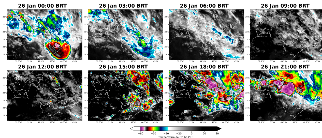
Figura 6: Imagens realçadas do satélite GOES-16 das 00 BRT até 21 BRT (a cada 3 horas) para o dia 26 janeiro.
