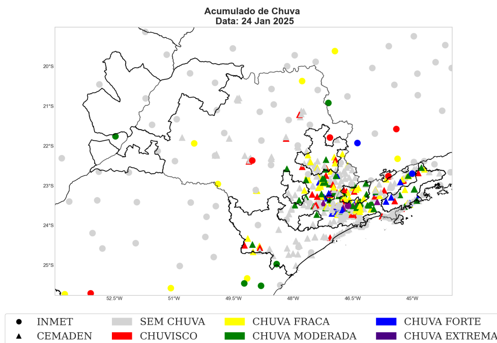
Figura 15: Acumulado de precipitação sobre a área de concessão da Neoenergia-Elektro para o dia 24 janeiro baseado nas estações meteorológicas do INMET e CEMADEN.
