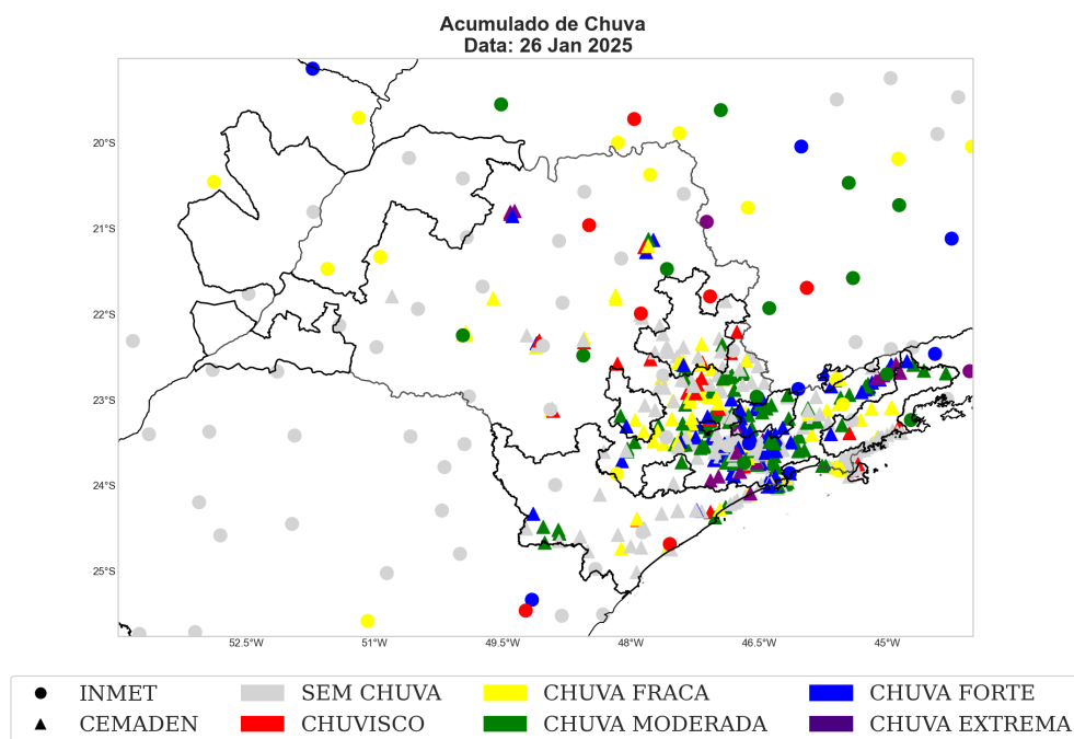
Figura 17: Acumulado diário de precipitação sobre a área de concessão da Neoenergia-Elektro para o dia 26 janeiro, baseado nas estações meteorológicas do INMET e CEMADEN.
