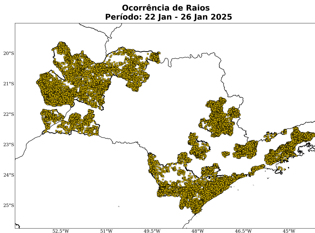
Figura 12: Total de ocorrências de descargas atmosféricas nuvem-solo detectadas pelo sistema Earth Networks para o período 22 a 26 de janeiro de 2025 sobre a área de concessão da Neoenergia-Elektro.
