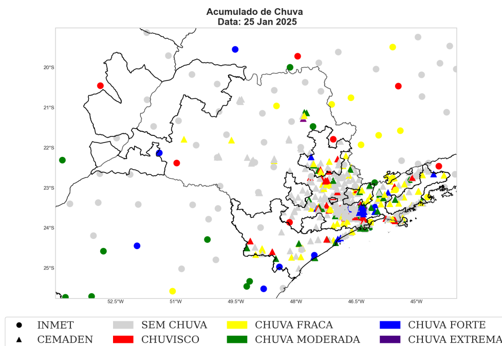
Figura 16: Acumulado diário de precipitação sobre a área de concessão da Neoenergia-Elektro para o dia 25 janeiro, baseado nas estações meteorológicas do INMET e CEMADEN.
