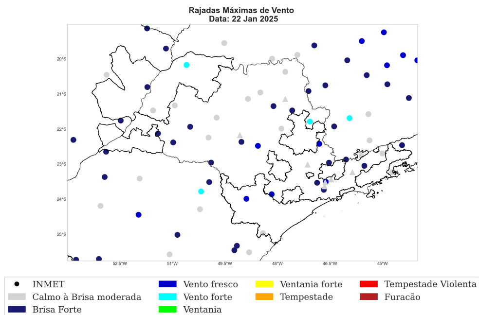
Figura 19: Rajada de vento sobre o estado de São Paulo para o dia 22 janeiro, baseado nas estações meteorológicas do INMET
