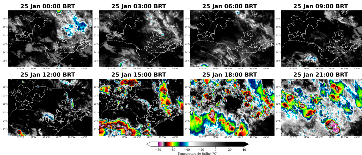
Figura 5: Imagens realçadas do satélite GOES-16 das 00 BRT até 21 BRT (a cada 3 horas) para o dia 25 janeiro.
