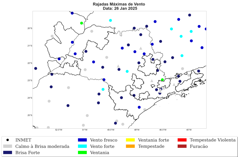
Figura 23: Máxima rajada de vento diária sobre a área de concessão da Neoenergia-Elektro para o dia 26 janeiro, baseado nas estações meteorológicas do INMET.
