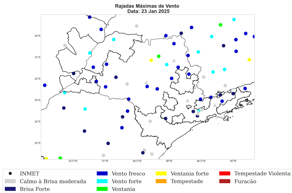
Figura 20: Rajada de vento sobre o estado de São Paulo para o dia 23 janeiro, baseado nas estações meteorológicas do INMET
