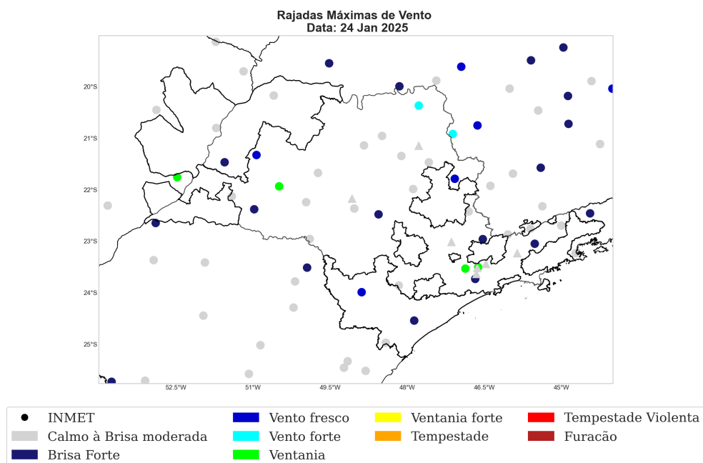
Figura 21: Rajada de vento sobre o estado de São Paulo para o dia 24 janeiro, baseado nas estações meteorológicas do INMET
