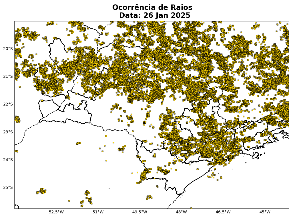
Figura 11: Ocorrências de descargas atmosféricas nuvem-solo detectadas pelo sistema Earth Networks para o dia 26 janeiro sobre a área de concessão da Neoenergia-Elektro.
