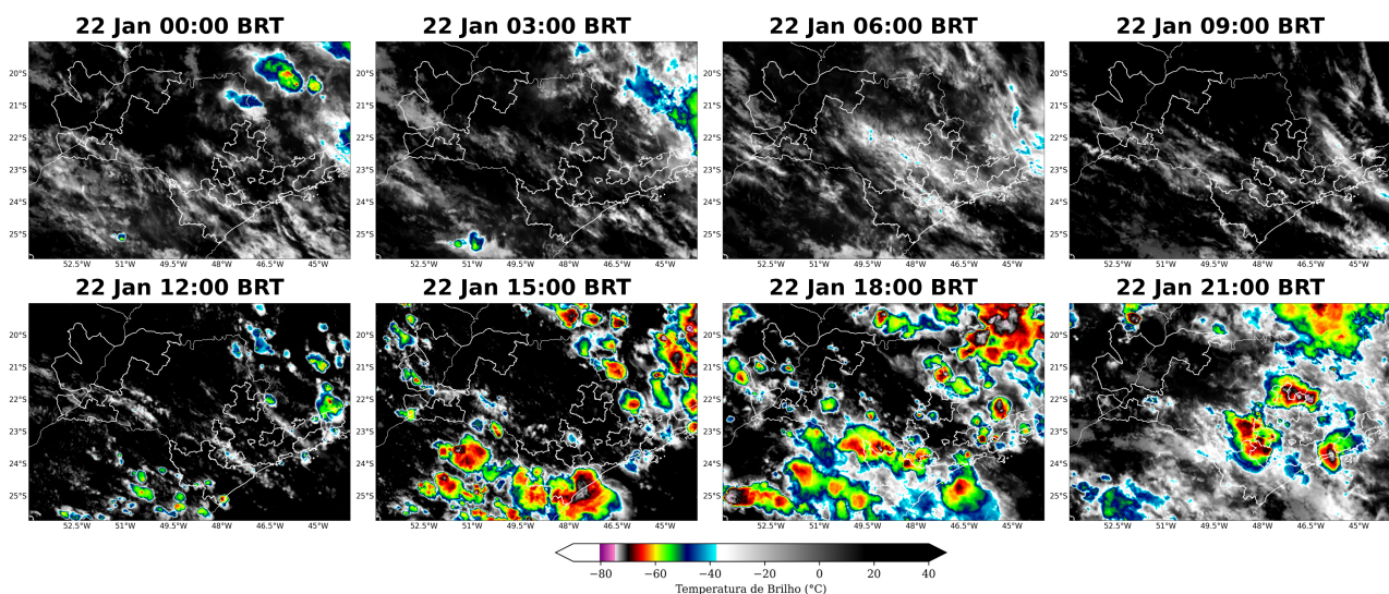
Figura 2: Imagens realçadas do satélite GOES-16 das 00 BRT até 21 BRT (a cada 3 horas) para o dia 22 janeiro.
