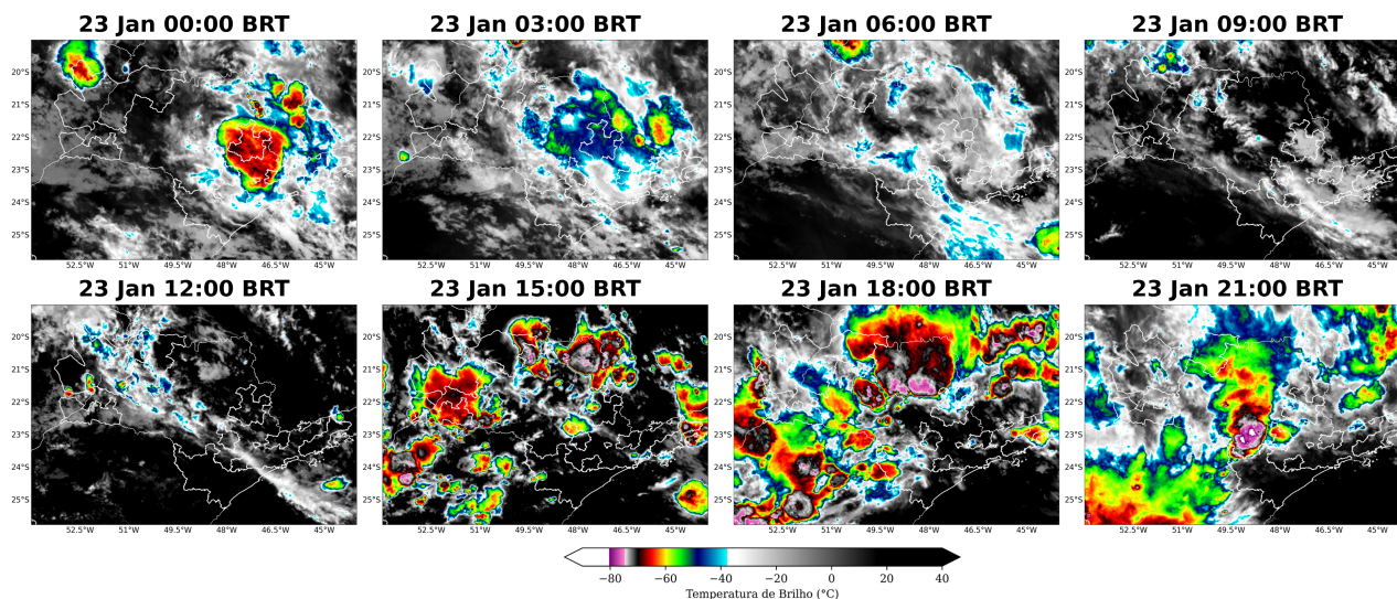
Figura 3: Imagens realçadas do satélite GOES-16 das 00 BRT até 21 BRT (a cada 3 horas) para o dia 23 janeiro.
