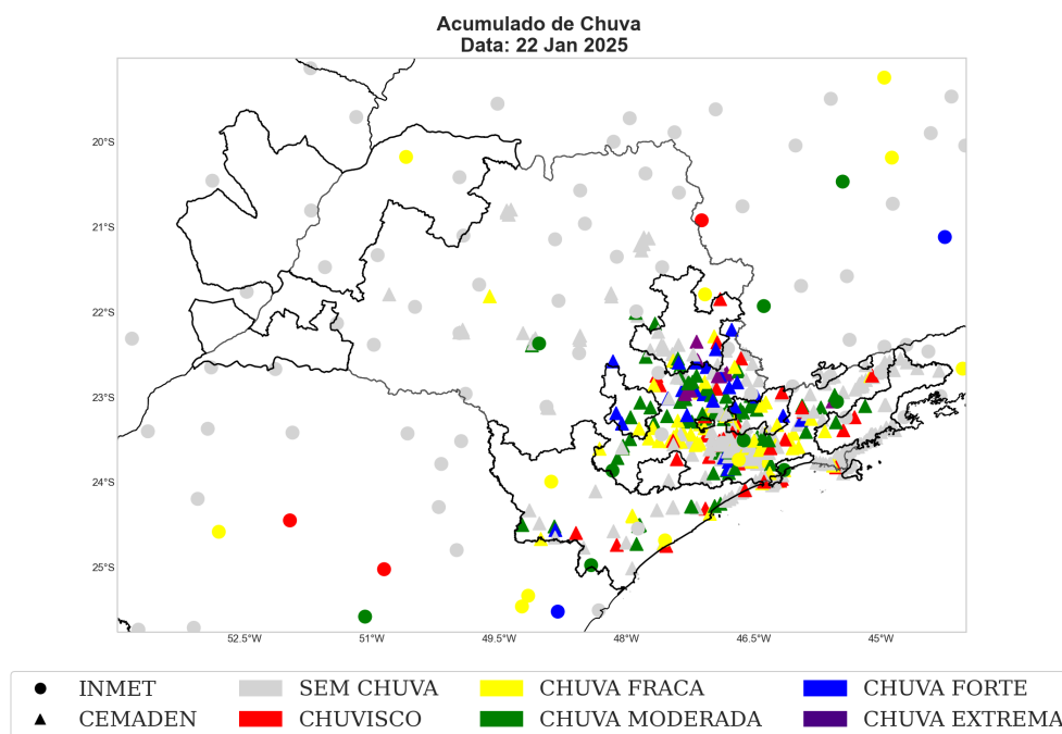
Figura 13: Acumulado de precipitação sobre a área de concessão da Neoenergia-Elektro para o dia 22 janeiro baseado nas estações meteorológicas do INMET e CEMADEN.
