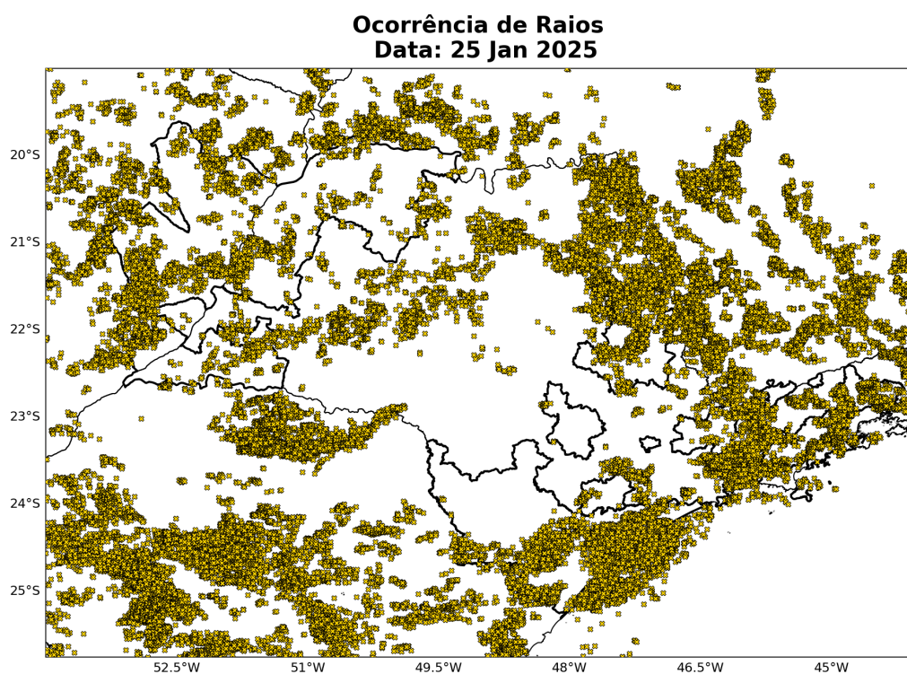
Figura 10: Ocorrências de descargas atmosféricas nuvem-solo detectadas pelo sistema Earth Networks para o dia 25 janeiro sobre a área de concessão da Neoenergia-Elektro.
