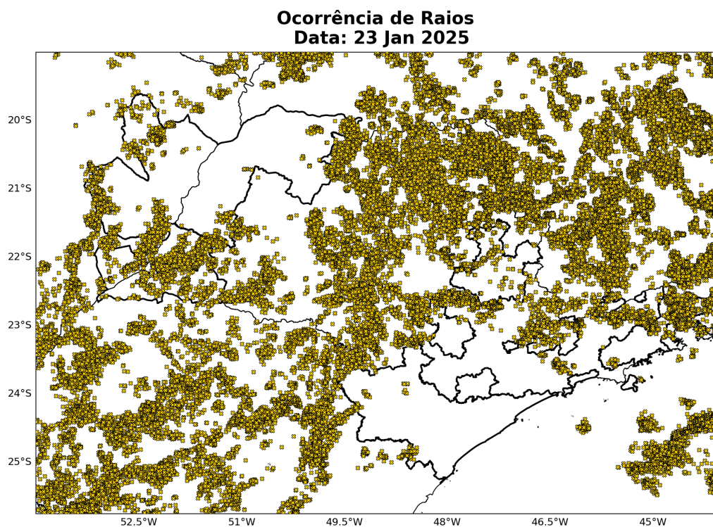
Figura 8: Ocorrências de descargas atmosféricas nuvem-solo detectadas pelo sistema Earth Networks para o dia 23 janeiro sobre a área de concessão da Neoenergia-Elektro.
