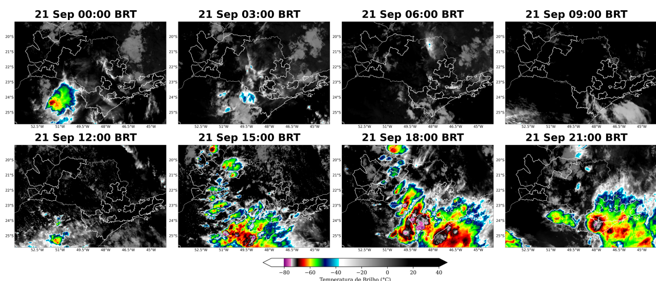
Figura 2: Imagens realçadas do satélite GOES-19 das 00 BRT até 21 BRT (a cada 3 horas) para o dia 21 de Setembro.
