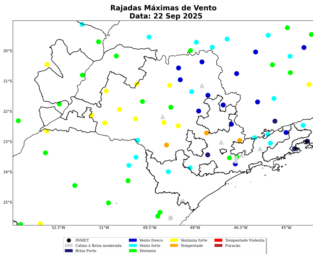
Figura 13: Máxima rajada de vento diária sobre a área de concessão da Neoenergia Elektro para o dia 22 de Setembro, baseado nas estações meteorológicas do INMET.
