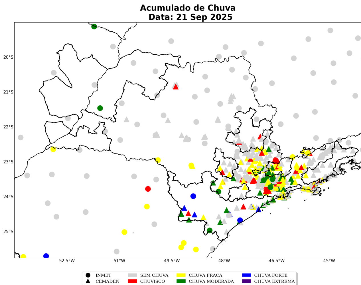
Figura 8: Acumulado diário de precipitação sobre a área de concessão da Neoenergia Elektro para o dia 21 de Setembro, baseado nas estações meteorológicas do INMET e CEMADEN.
