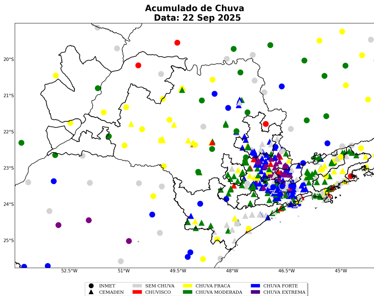
Figura 9: Acumulado diário de precipitação sobre a área de concessão da Neoenergia Elektro para o dia 22 de Setembro, baseado nas estações meteorológicas do INMET e CEMADEN.
