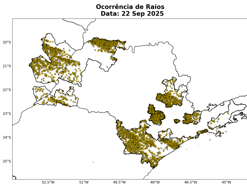
Figura 6: Ocorrências de descargas atmosféricas nuvem-solo detectadas pelo sistema Earth Networks para o dia 22 de Setembro sobre a área de concessão da Neoenergia Elektro.
