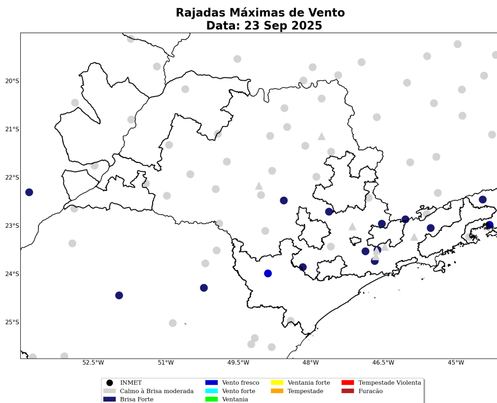
Figura 14: Máxima rajada de vento diária sobre a área de concessão da Neoenergia Elektro para o dia 23 de Setembro, baseado nas estações meteorológicas do INMET.
