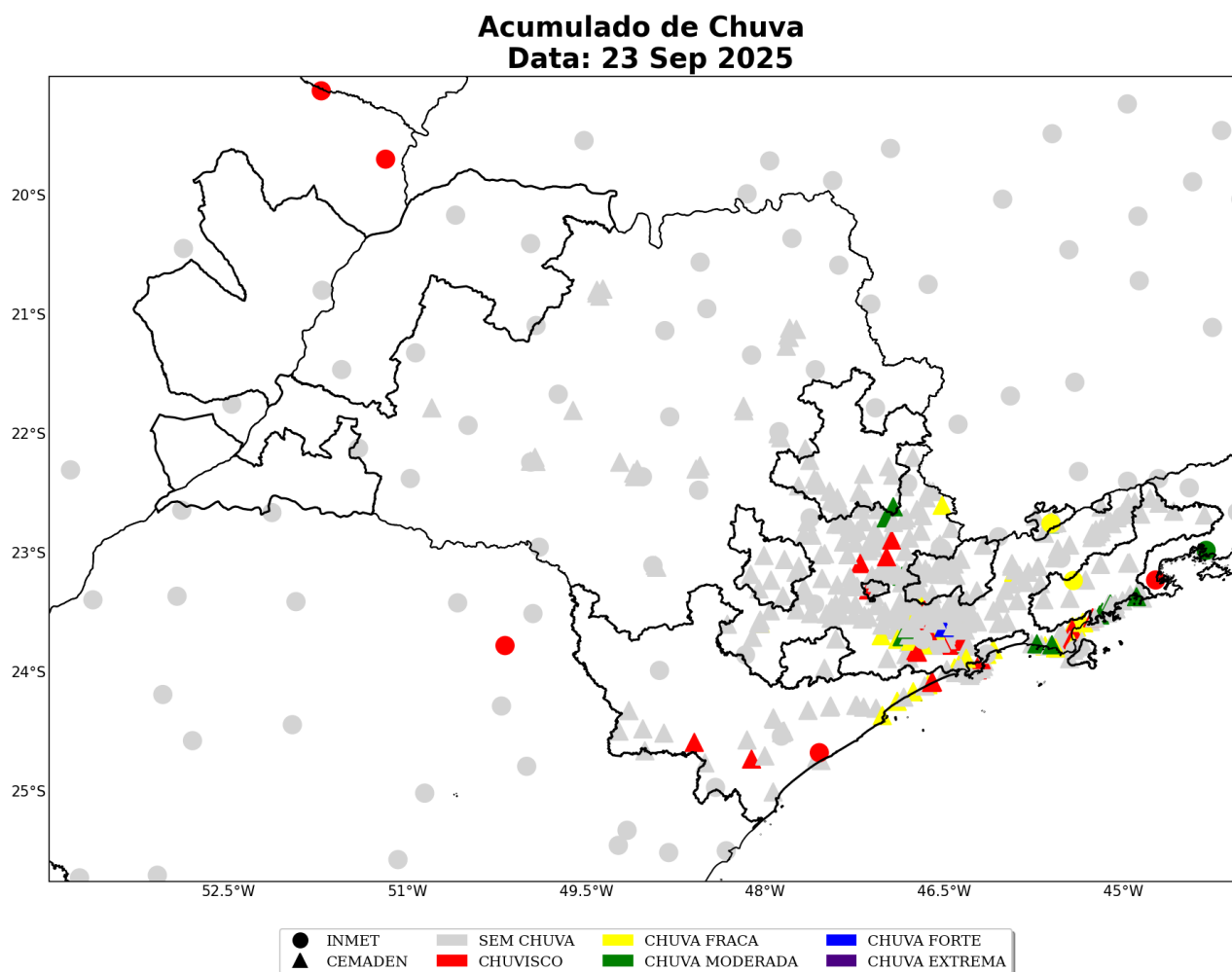
Figura 10: Acumulado diário de precipitação sobre a área de concessão da Neoenergia Elektro para o dia 23 de Setembro, baseado nas estações meteorológicas do INMET e CEMADEN.
