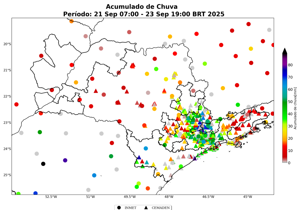
Figura 11: Acumulado de precipitação sobre a área de concessão da Neoenergia Elektro para o período do evento (dias 21 a 23 de Setembro de 2025), baseado nas estações meteorológicas do INMET e CEMADEN.
