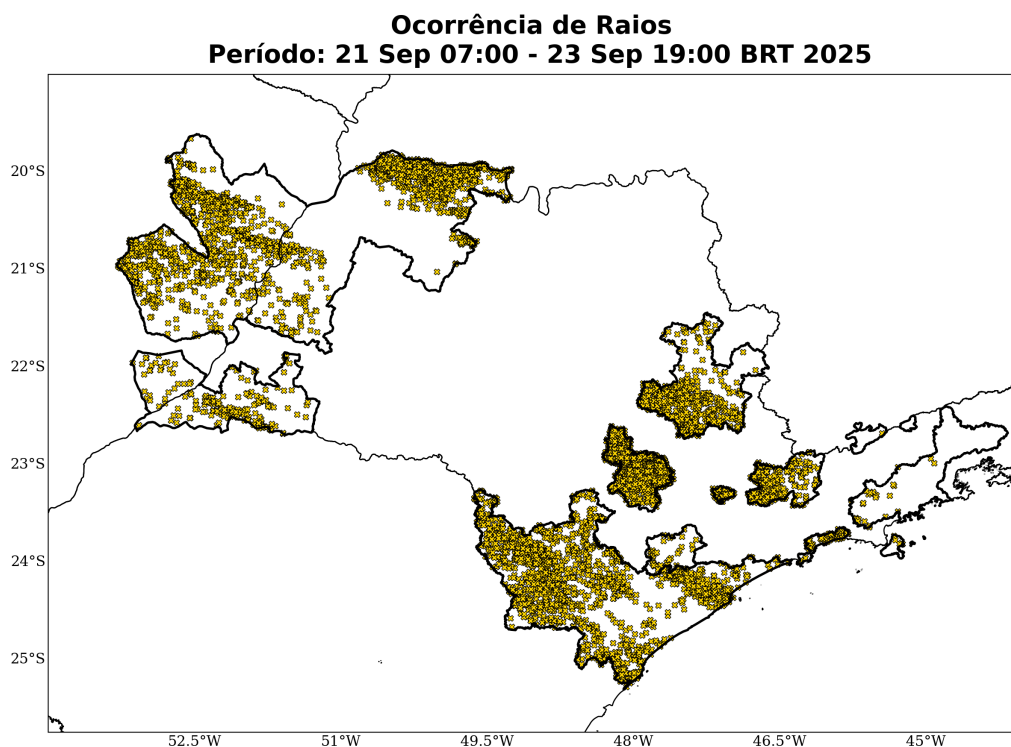
Figura 7: Ocorrências de descargas atmosféricas nuvem-solo detectadas pelo sistema Earth Networks para o período de 21 a 23 de Setembro de 2025 sobre a área de concessão da Neoenergia Elektro.
