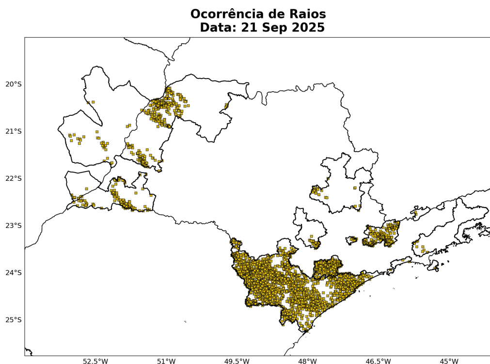
Figura 5: Ocorrências de descargas atmosféricas nuvem-solo detectadas pelo sistema Earth Networks para o dia 21 de Setembro sobre a área de concessão da Neoenergia Elektro.
