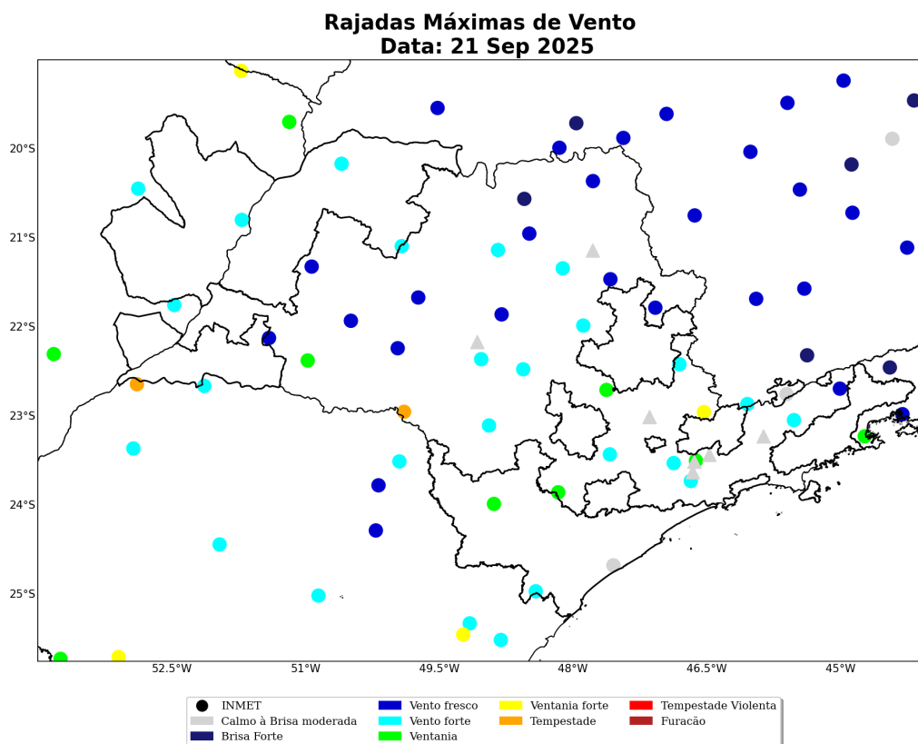
Figura 12: Máxima rajada de vento diária sobre a área de concessão da Neoenergia Elektro para o dia 21 de Setembro, baseado nas estações meteorológicas do INMET.
