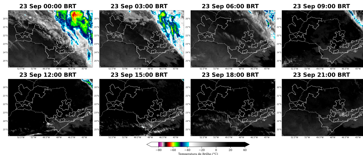
Figura 4: Imagens realçadas do satélite GOES-19 das 00 BRT até 21 BRT (a cada 3 horas) para o dia 23 de Setembro.
