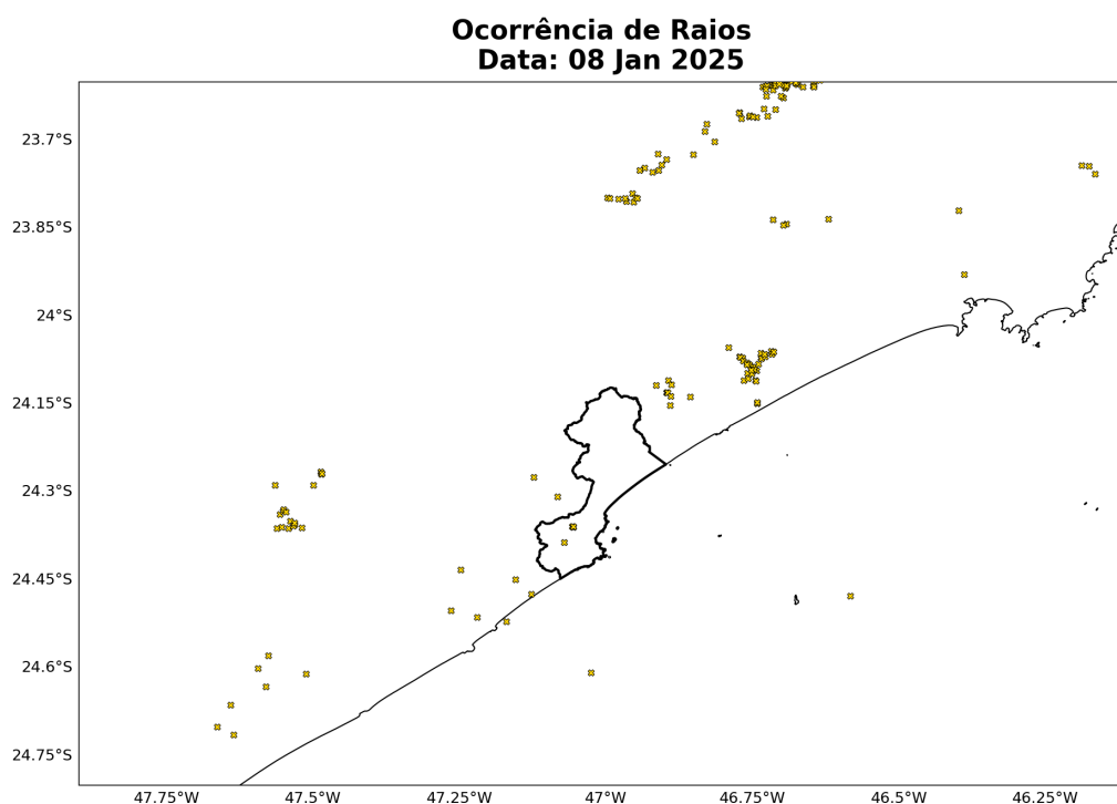
Figura 4: Densidade de descargas atmosféricas nuvem-solo detectadas pelo sistema Earth Networks no dia 08 janeiro de 2025 no município de Peruíbe.
