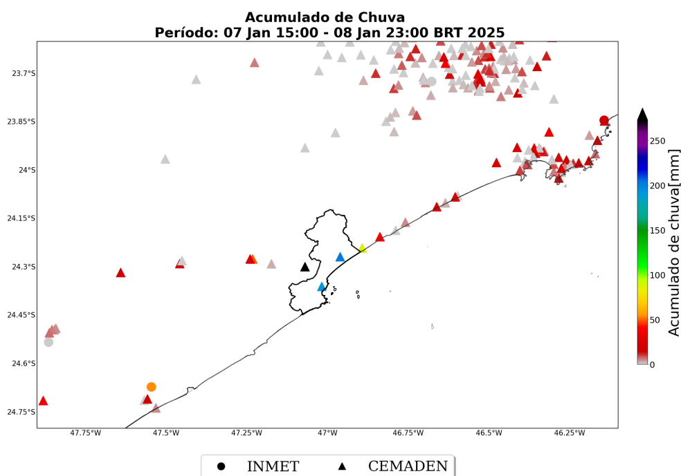
Figura 7: Acumulado de precipitação sobre o município Peruíbe e sobre os municípios circunvizinhos para o período de 07 a 08 de janeiro de 2025 baseado nas estações meteorológicas do INMET e CEMADEN.
