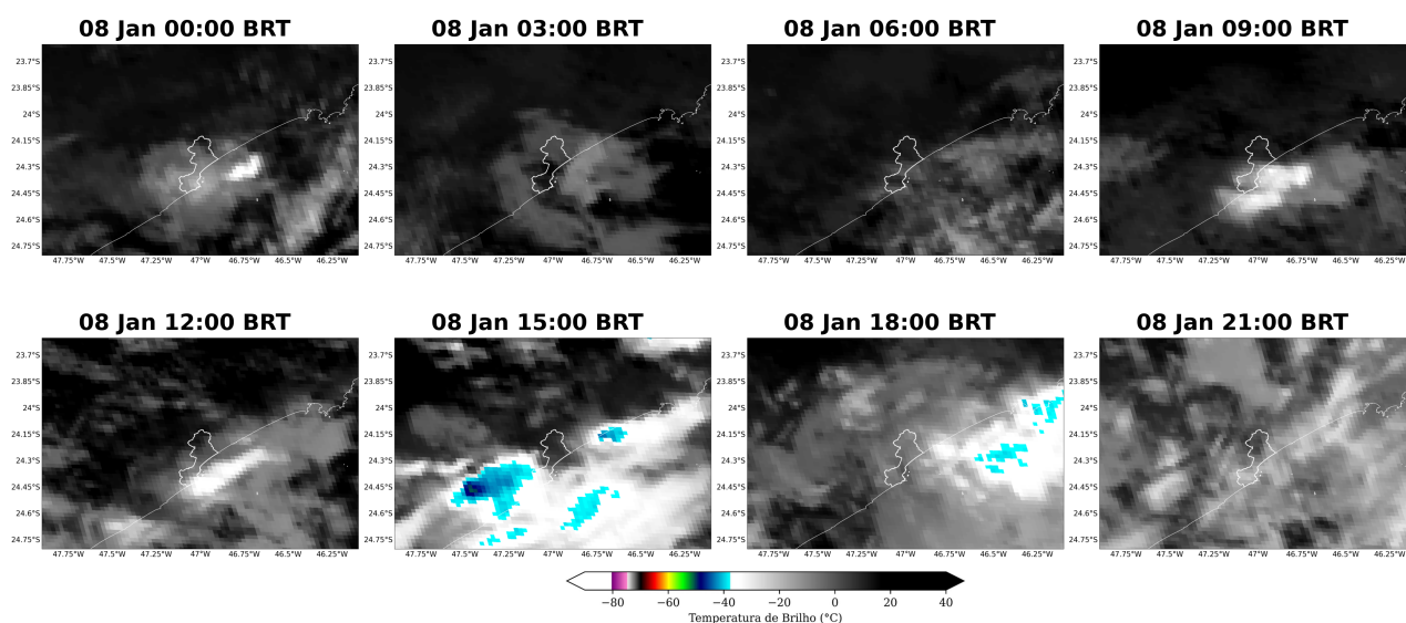
Figura 3: Imagens realçadas do satélite GOES-16 das 00 BRT até 21 BRT (a cada 3 hora) para o dia 08 janeiro de 2025.
