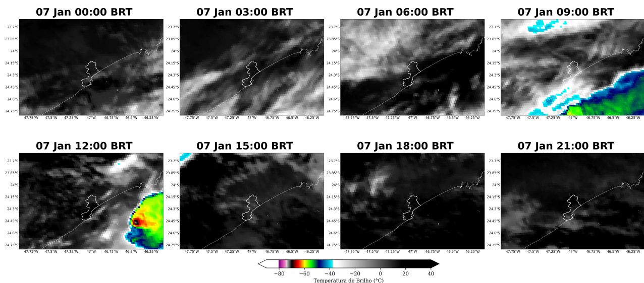
Figura 2: Imagens realçadas do satélite GOES-16 das 00 BRT até 21 BRT (a cada 3 hora) para o dia 07 janeiro de 2025.
