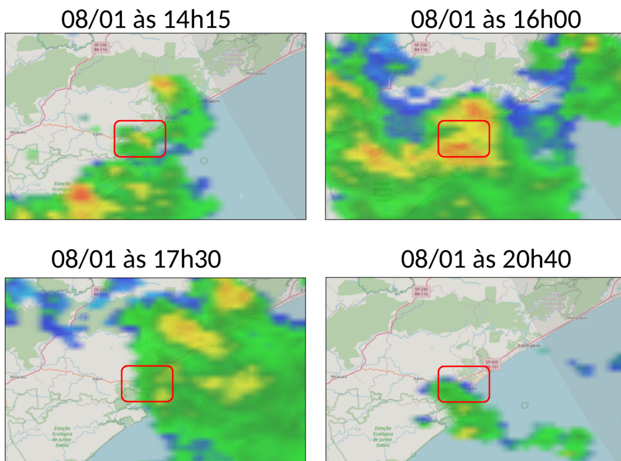
Figura 8: Imagens dos radares meteorológicos de São Paulo, proveniente da REDEMET, o qual apresenta a refletividade (dBZ) e estimativa de precipitação, para o dia 08 janeiro de 2025. O retângulo em vermelho marca a localização do município de Peruíbe. Fonte: REDEMET.
