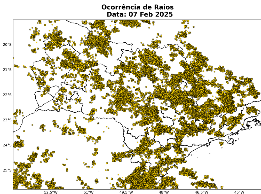
Figura 7: Ocorrências de descargas atmosféricas nuvem-solo detectadas pelo sistema Earth Networks para o dia 07 de Fevereiro sobre a área de concessão da Elektro.
