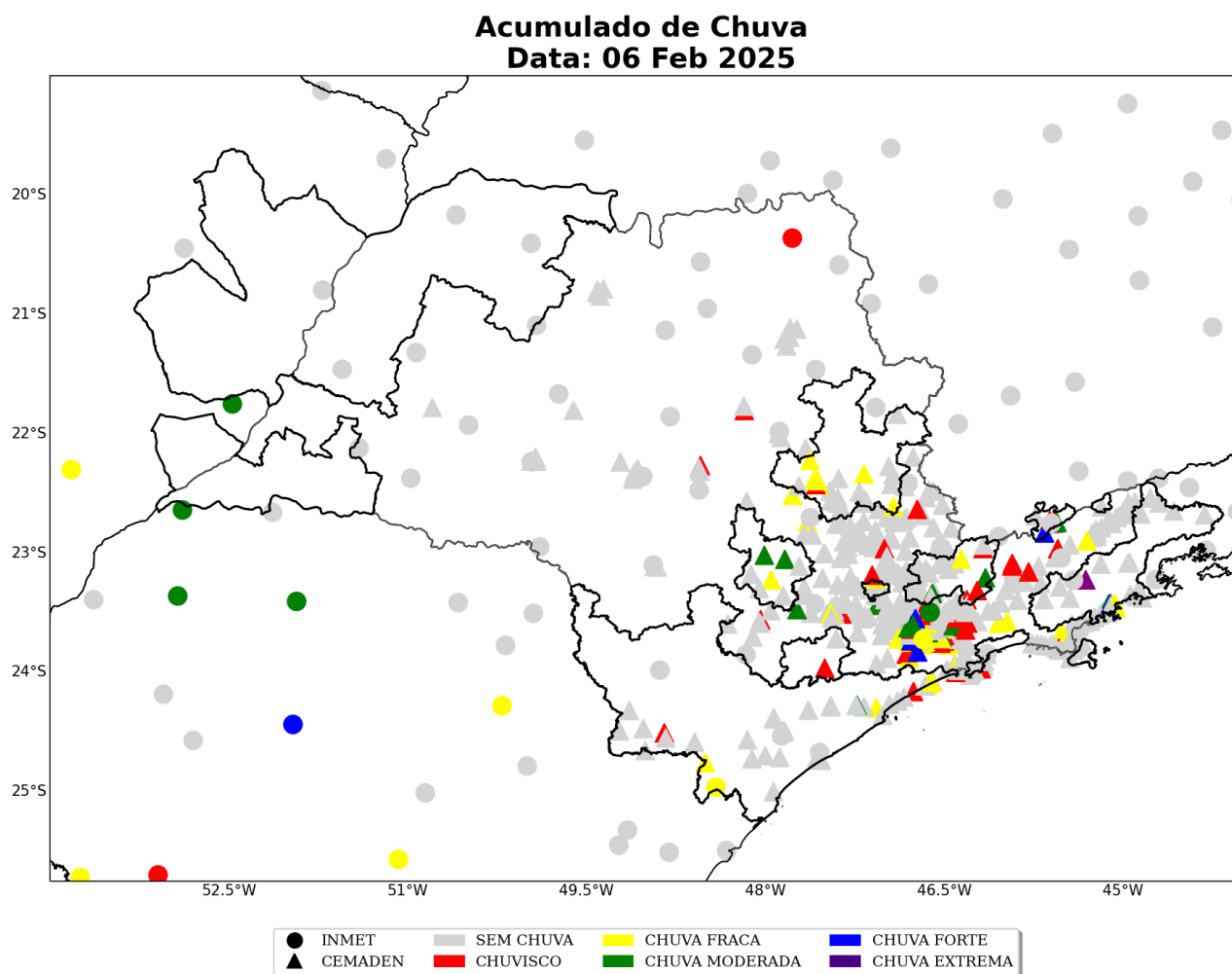
Figura 11: Acumulado diário de precipitação sobre a área de concessão da Elektro para o dia 06 de Fevereiro, baseado nas estações meteorológicas do INMET e CEMADEN.
