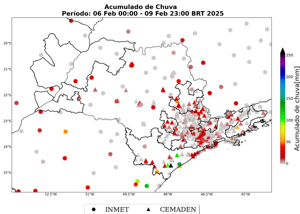
Figura 15: Acumulado de precipitação sobre o estado do São Paulo para o período do evento (dias 06 a 09 de Fevereiro de 2025), baseado nas estações meteorológicas do INMET e CEMADEN.
