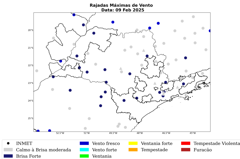
Figura 19: Máxima rajada de vento diária sobre a área de concessão da Elektro para o dia 09 de Fevereiro, baseado nas estações meteorológicas do INMET.
