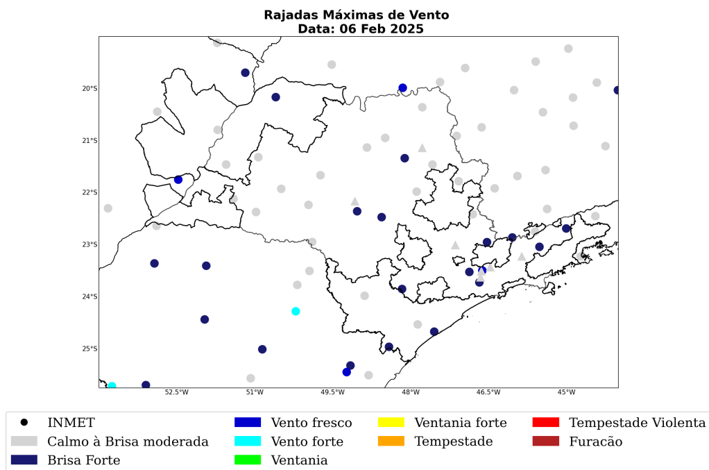
Figura 16: Máxima rajada de vento diária sobre a área de concessão da Elektro para o dia 06 de Fevereiro, baseado nas estações meteorológicas do INMET.
