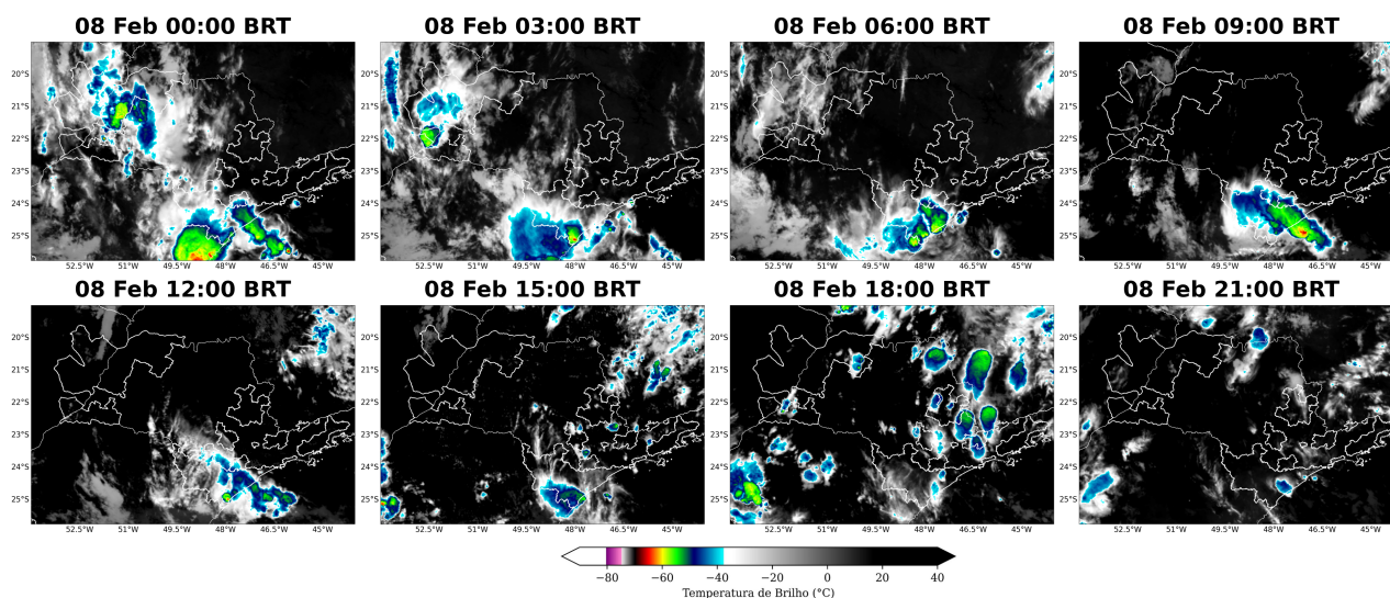
Figura 4: Imagens realçadas do satélite GOES-16 das 00 BRT até 21 BRT (a cada 3 horas) para o dia 08 de Fevereiro.
