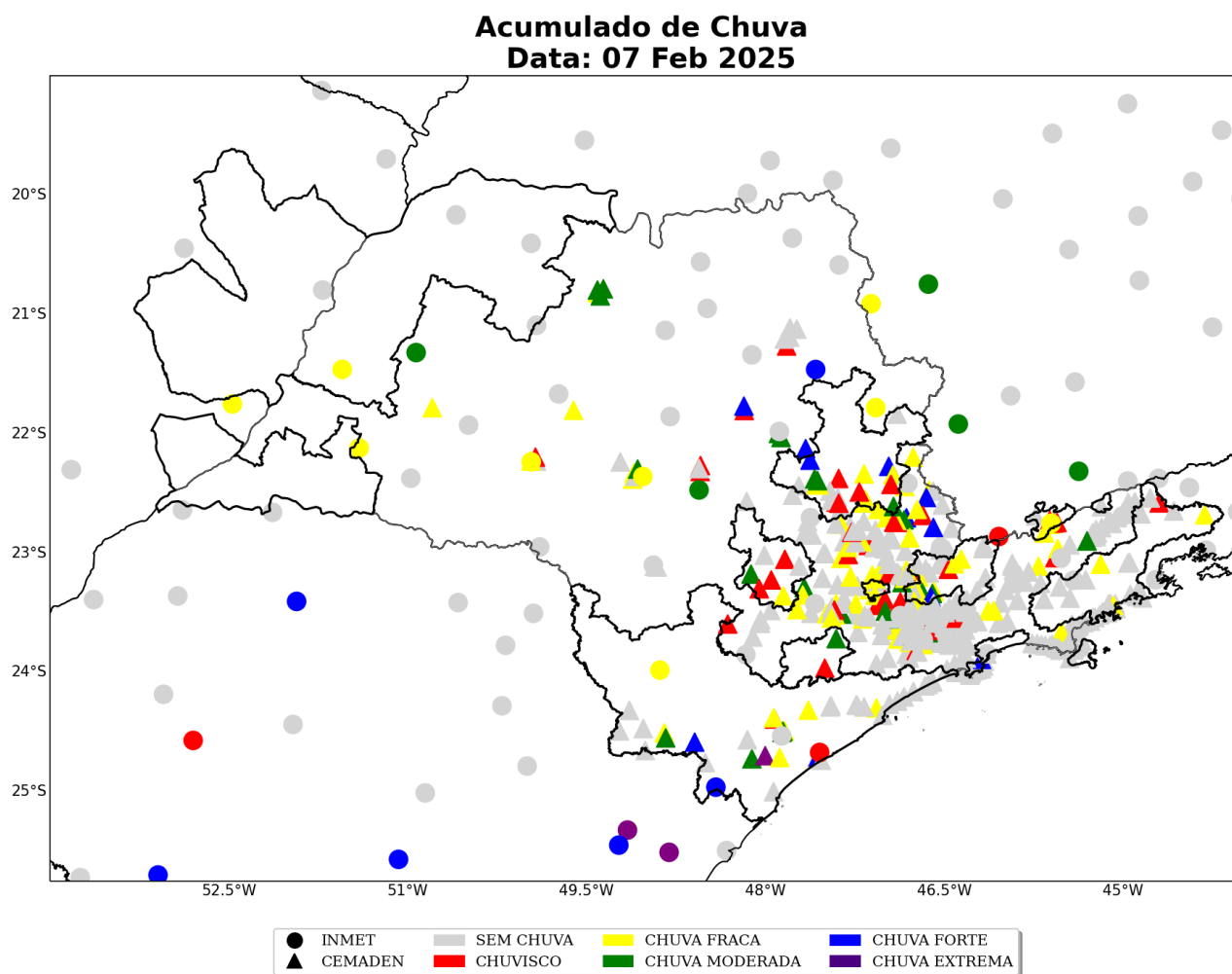
Figura 12: Acumulado diário de precipitação sobre a área de concessão da Elektro para o dia 07 de Fevereiro, baseado nas estações meteorológicas do INMET e CEMADEN.
