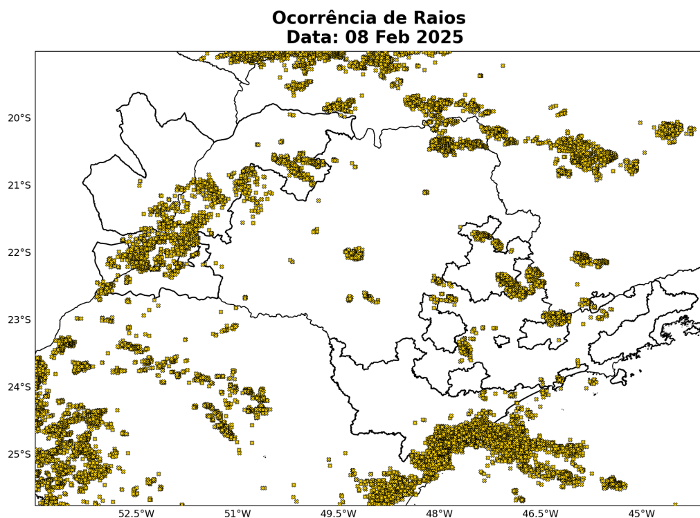
Figura 8: Ocorrências de descargas atmosféricas nuvem-solo detectadas pelo sistema Earth Networks para o dia 08 de Fevereiro sobre a área de concessão da Elektro.
