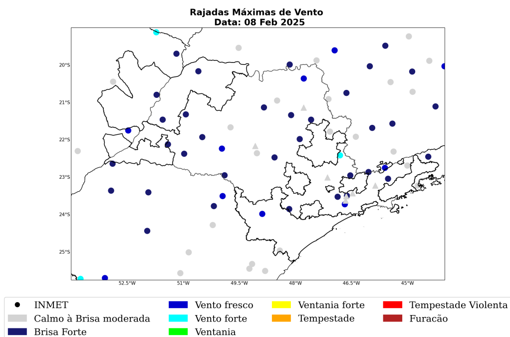
Figura 18: Máxima rajada de vento diária sobre a área de concessão da Elektro para o dia 08 de Fevereiro, baseado nas estações meteorológicas do INMET.
