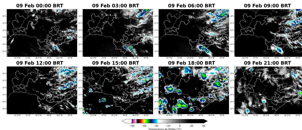
Figura 5: Imagens realçadas do satélite GOES-16 das 00 BRT até 21 BRT (a cada 3 horas) para o dia 09 de Fevereiro.
