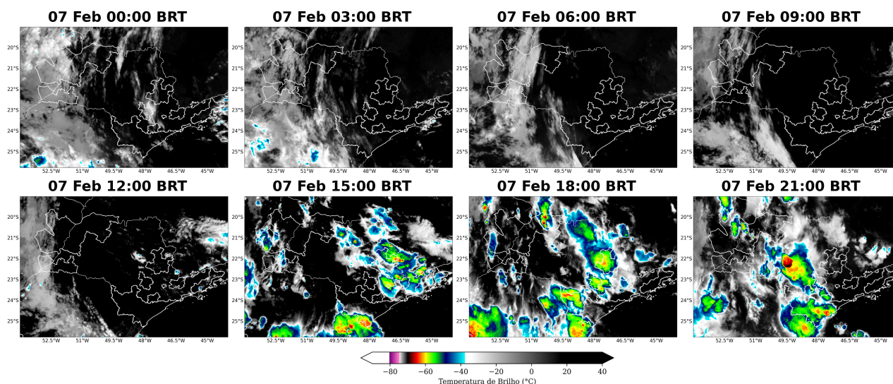
Figura 3: Imagens realçadas do satélite GOES-16 das 00 BRT até 21 BRT (a cada 3 horas) para o dia 07 de Fevereiro.
