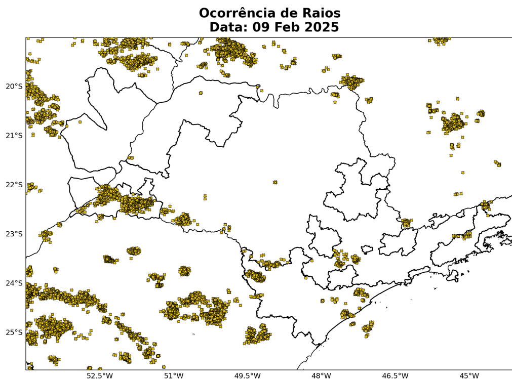
Figura 9: Ocorrências de descargas atmosféricas nuvem-solo detectadas pelo sistema Earth Networks para o dia 09 de Fevereiro sobre a área de concessão da Elektro.
