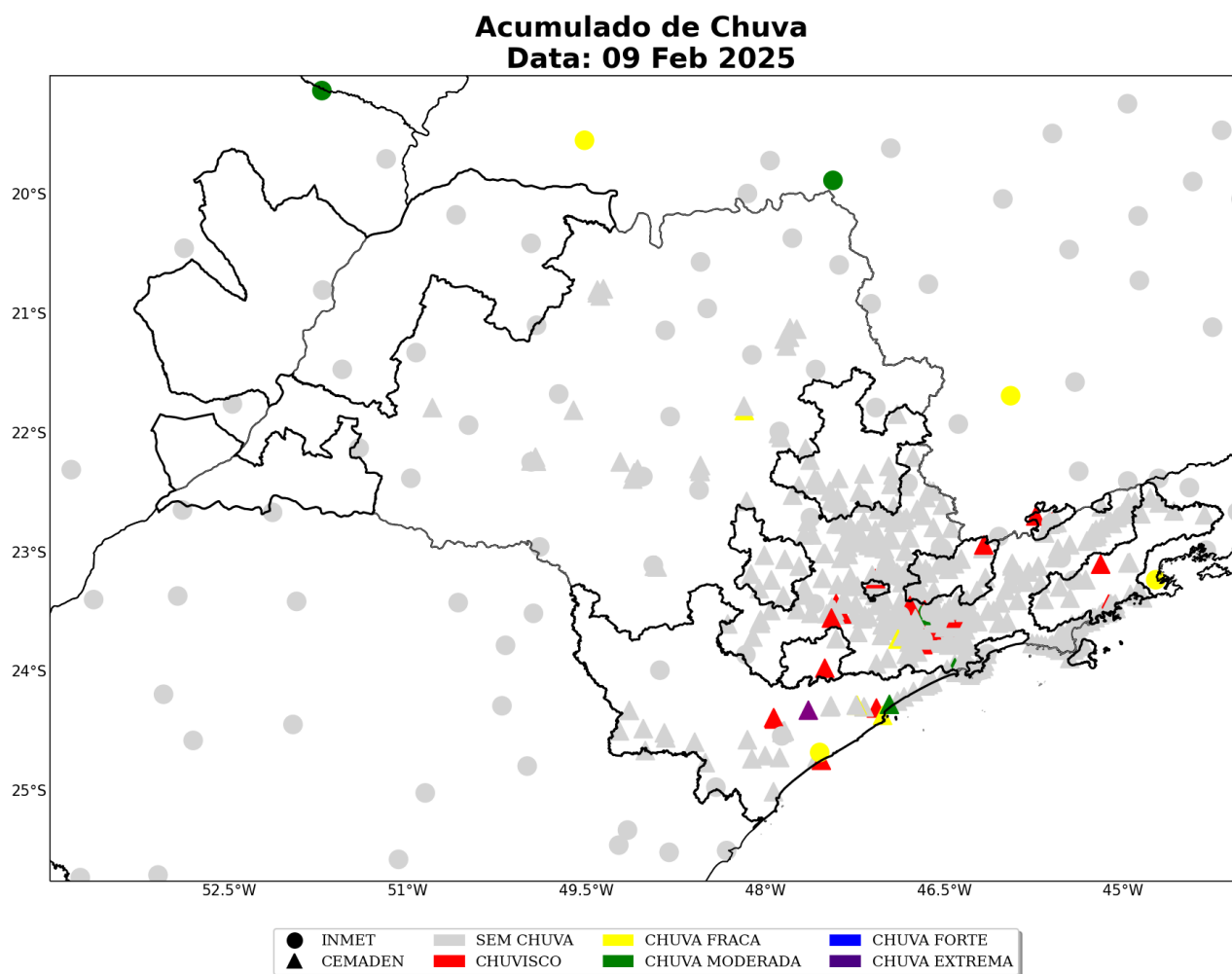
Figura 14: Acumulado diário de precipitação sobre a área de concessão da Elektro para o dia 09 de Fevereiro, baseado nas estações meteorológicas do INMET e CEMADEN.
