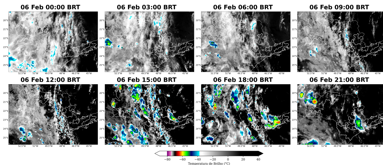
Figura 2: Imagens realçadas do satélite GOES-16 das 00 BRT até 21 BRT (a cada 3 horas) para o dia 06 de Fevereiro.
