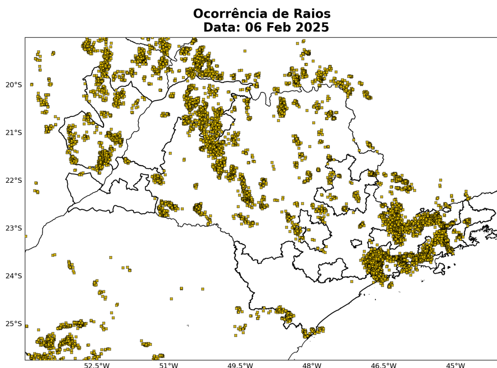
Figura 6: Ocorrências de descargas atmosféricas nuvem-solo detectadas pelo sistema Earth Networks para o dia 06 de Fevereiro sobre a área de concessão da Elektro.
