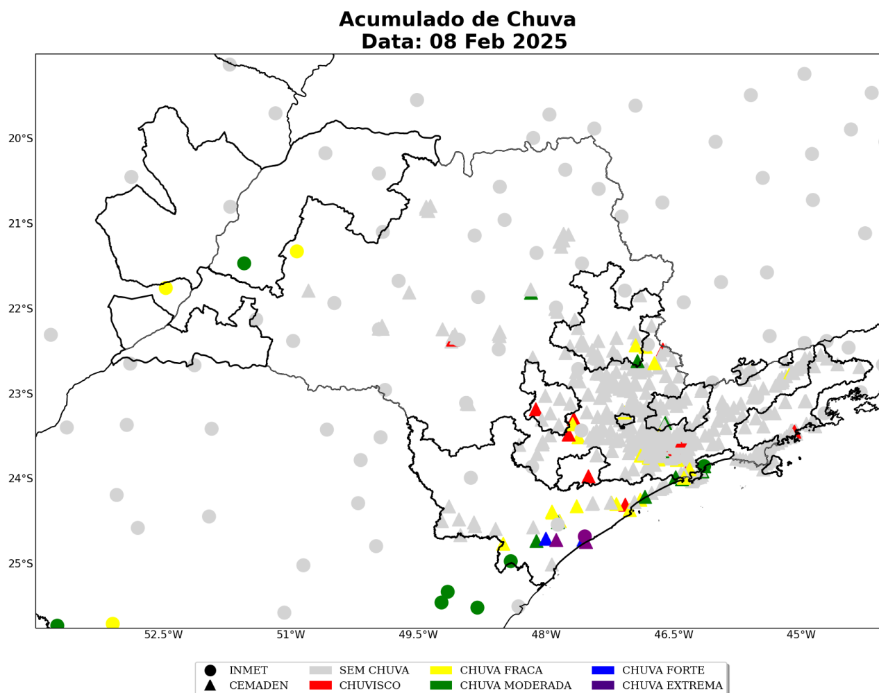
Figura 13: Acumulado diário de precipitação sobre a área de concessão da Elektro para o dia 08 de Fevereiro, baseado nas estações meteorológicas do INMET e CEMADEN.
