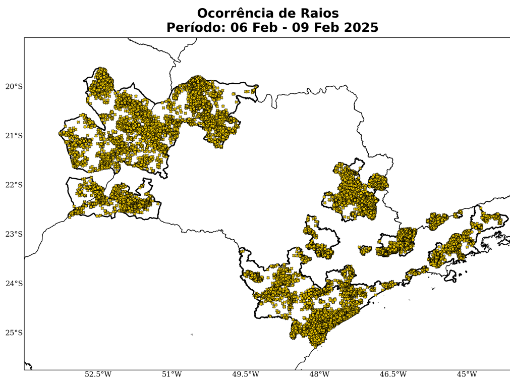
Figura 10: Ocorrências de descargas atmosféricas nuvem-solo detectadas pelo sistema Earth Networks para o período de 06 a 09 de Fevereiro de 2025 sobre a área de concessão da Elektro.
