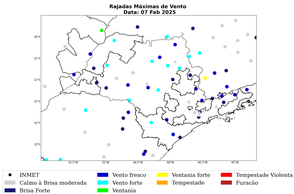
Figura 17: Máxima rajada de vento diária sobre a área de concessão da Elektro para o dia 07 de Fevereiro, baseado nas estações meteorológicas do INMET.
