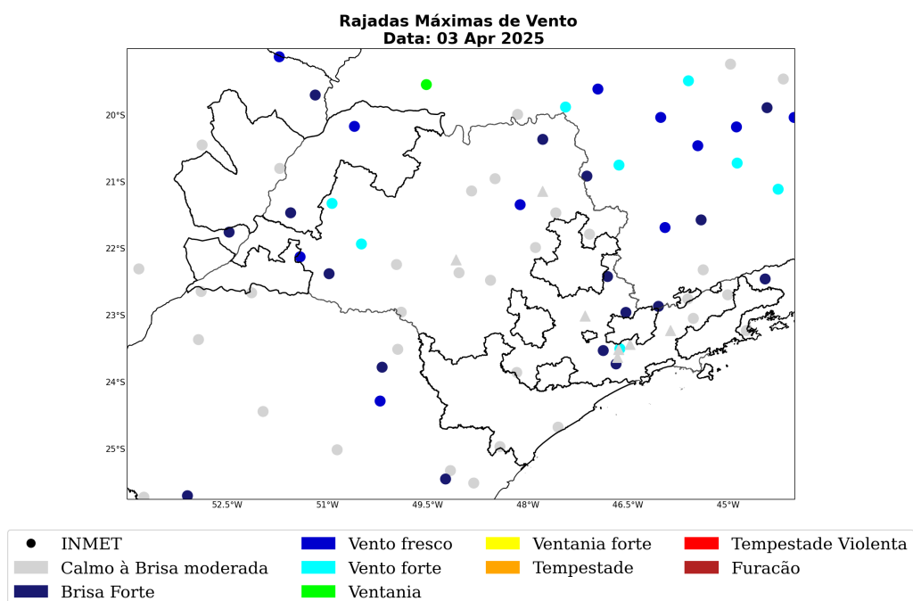
Figura 12: Máxima rajada de vento diária sobre a área de concessão da Neoenergia Elektro para o dia 03 de Abril, baseado nas estações meteorológicas do INMET.
