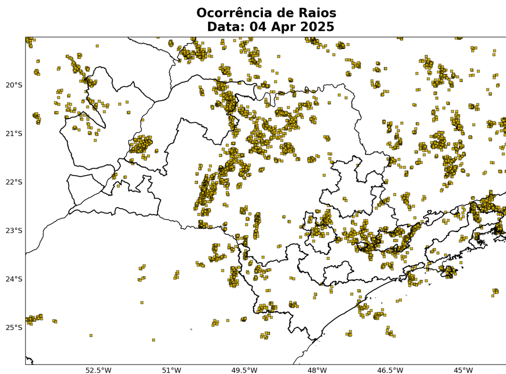
Figura 6: Ocorrências de descargas atmosféricas nuvem-solo detectadas pelo sistema Earth Networks para o dia 04 de Abril sobre a área de concessão da Neoenergia Elektro.
