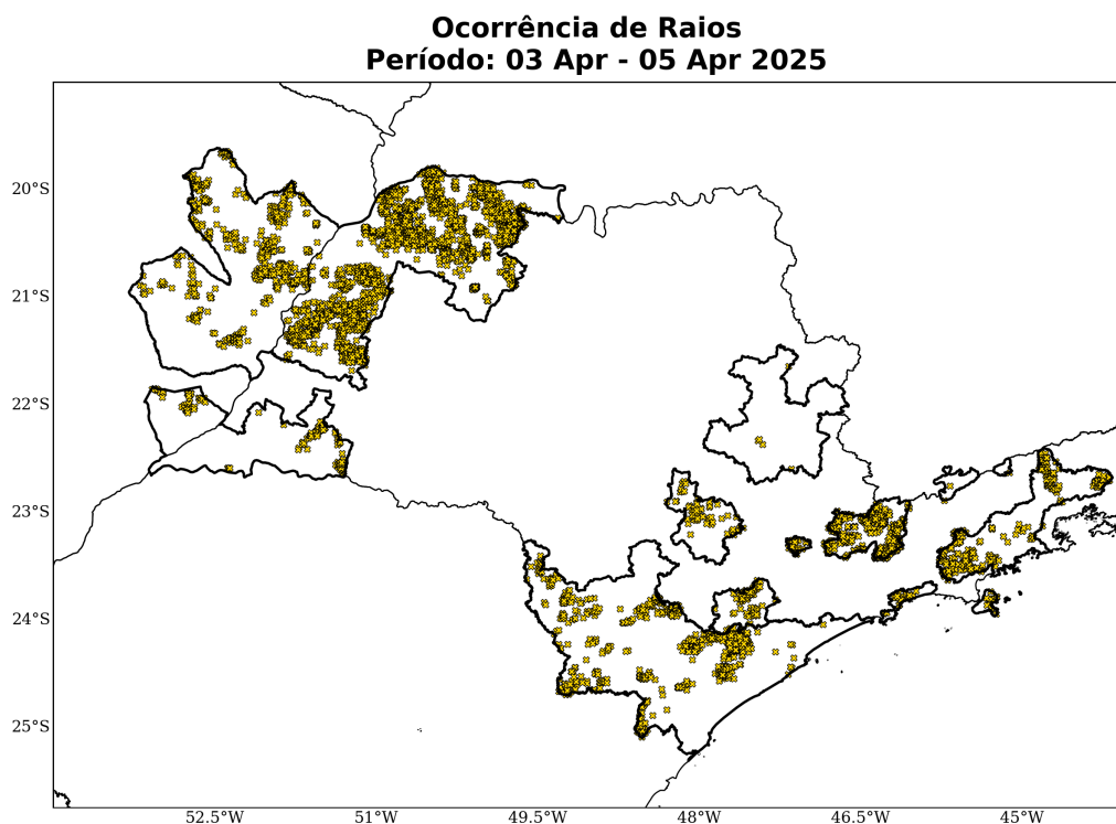
Figura 7: Ocorrências de descargas atmosféricas nuvem-solo detectadas pelo sistema Earth Networks para o período de 03 a 05 de Abril de 2025 sobre a área de concessão da Neoenergia Elektro.
