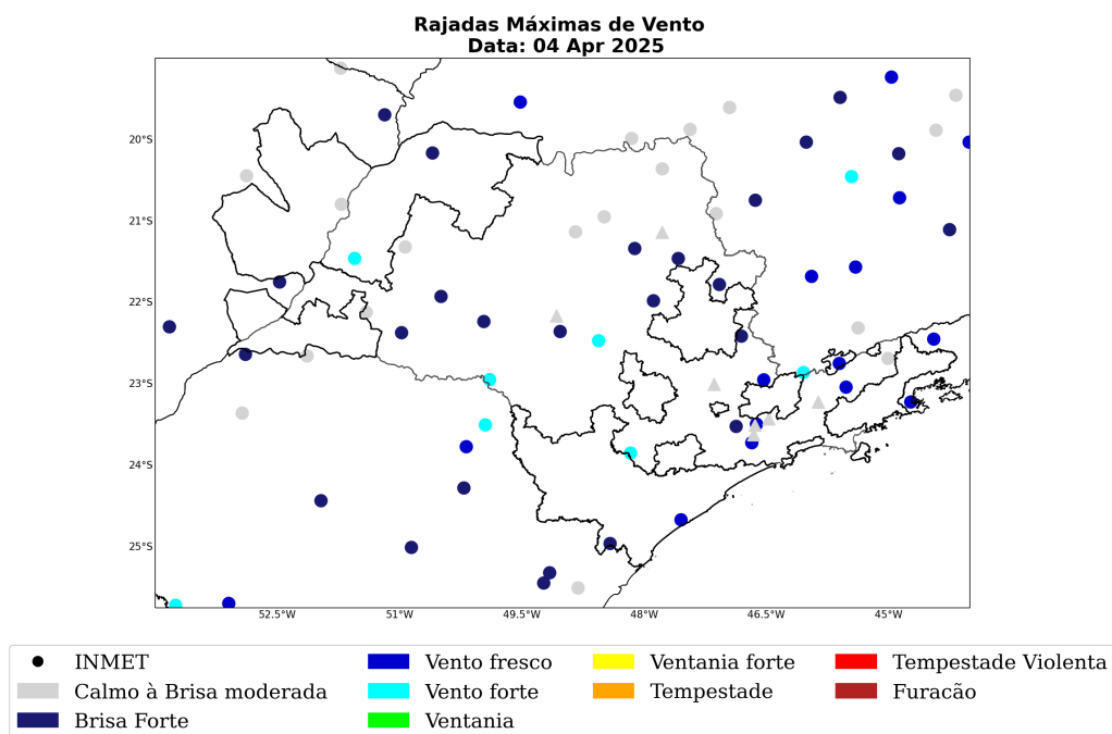
Figura 13: Máxima rajada de vento diária sobre a área de concessão da Neoenergia Elektro para o dia 04 de Abril, baseado nas estações meteorológicas do INMET.
