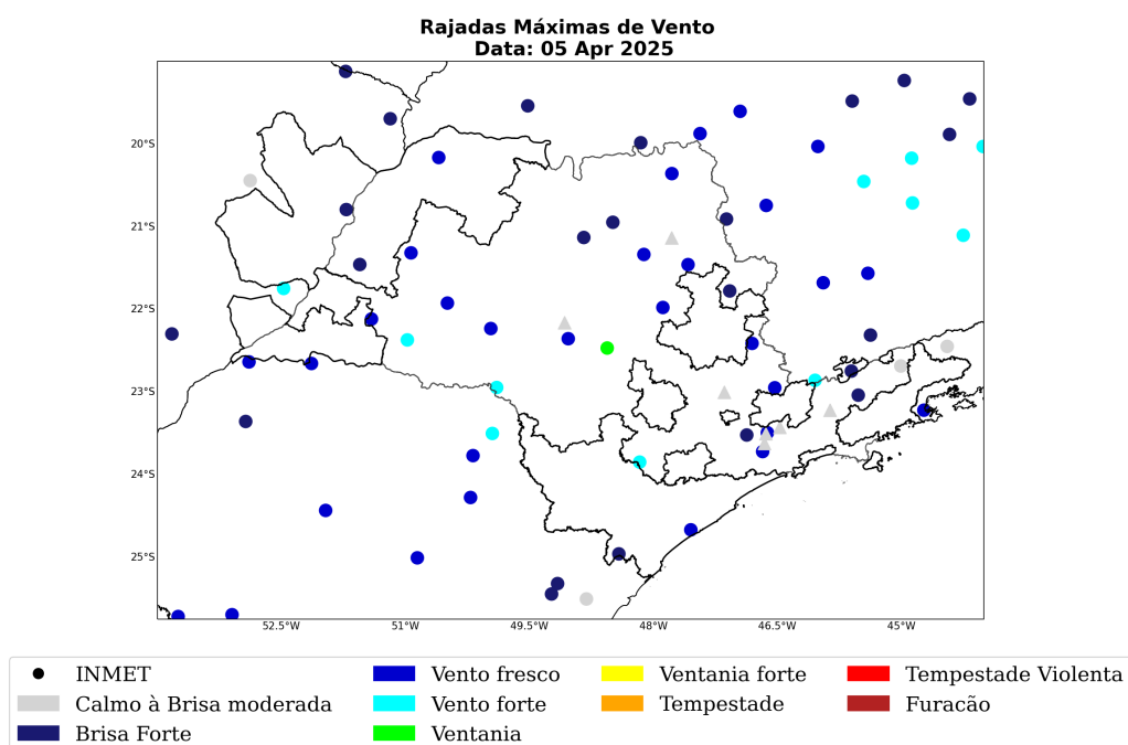
Figura 14: Máxima rajada de vento diária sobre a área de concessão da Neoenergia Elektro para o dia 05 de Abril, baseado nas estações meteorológicas do INMET.
