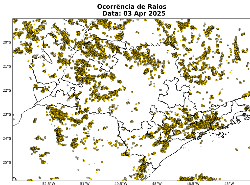
Figura 5: Ocorrências de descargas atmosféricas nuvem-solo detectadas pelo sistema Earth Networks para o dia 03 de Abril sobre a área de concessão da Neoenergia Elektro.
