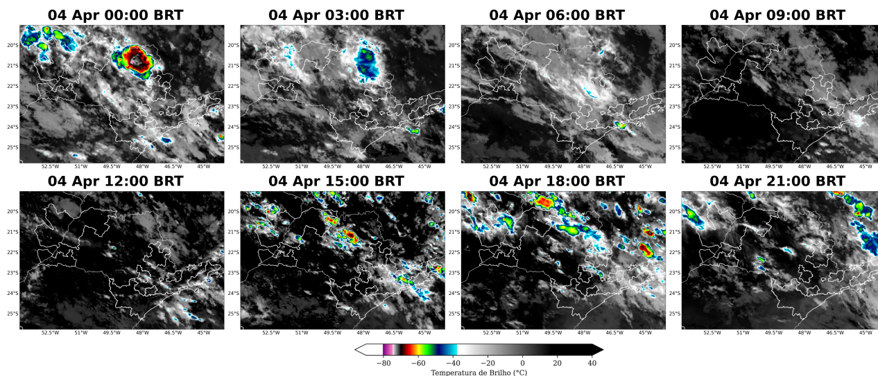
Figura 3: Imagens realçadas do satélite GOES-16 das 00 BRT até 21 BRT (a cada 3 horas) para o dia 04 de Abril.
