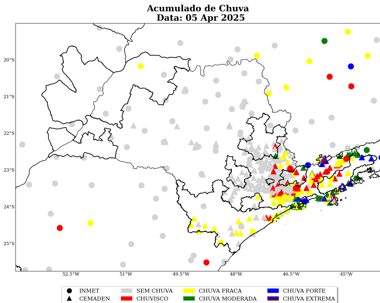
Figura 10: Acumulado diário de precipitação sobre a área de concessão da Neoenergia Elektro para o dia 05 de Abril, baseado nas estações meteorológicas do INMET e CEMADEN.
