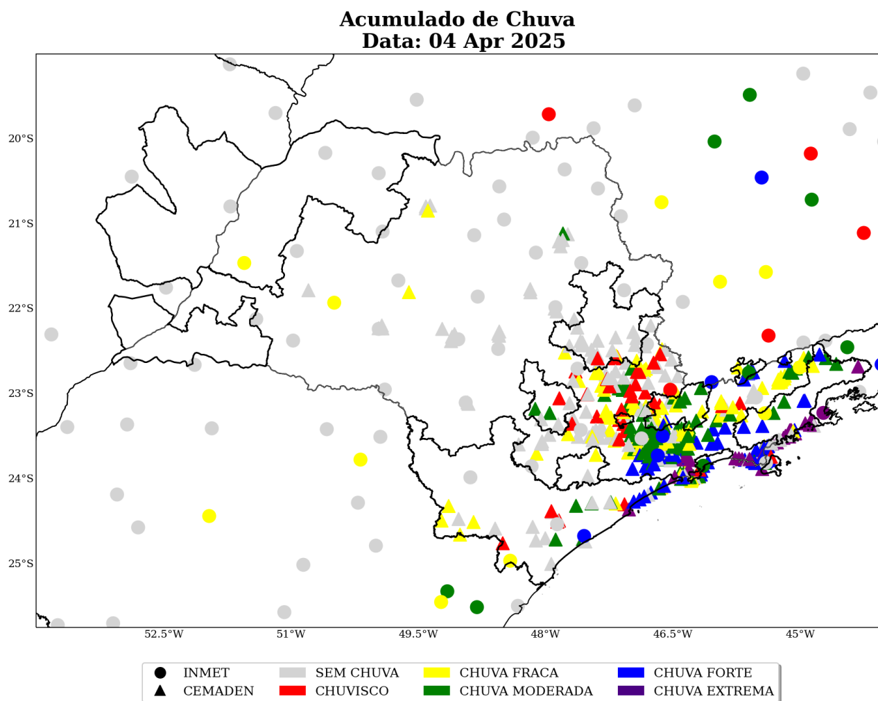
Figura 9: Acumulado diário de precipitação sobre a área de concessão da Neoenergia Elektro para o dia 04 de Abril, baseado nas estações meteorológicas do INMET e CEMADEN.
