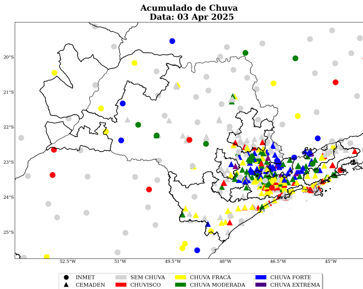
Figura 8: Acumulado diário de precipitação sobre a área de concessão da Neoenergia Elektro para o dia 03 de Abril, baseado nas estações meteorológicas do INMET e CEMADEN.
