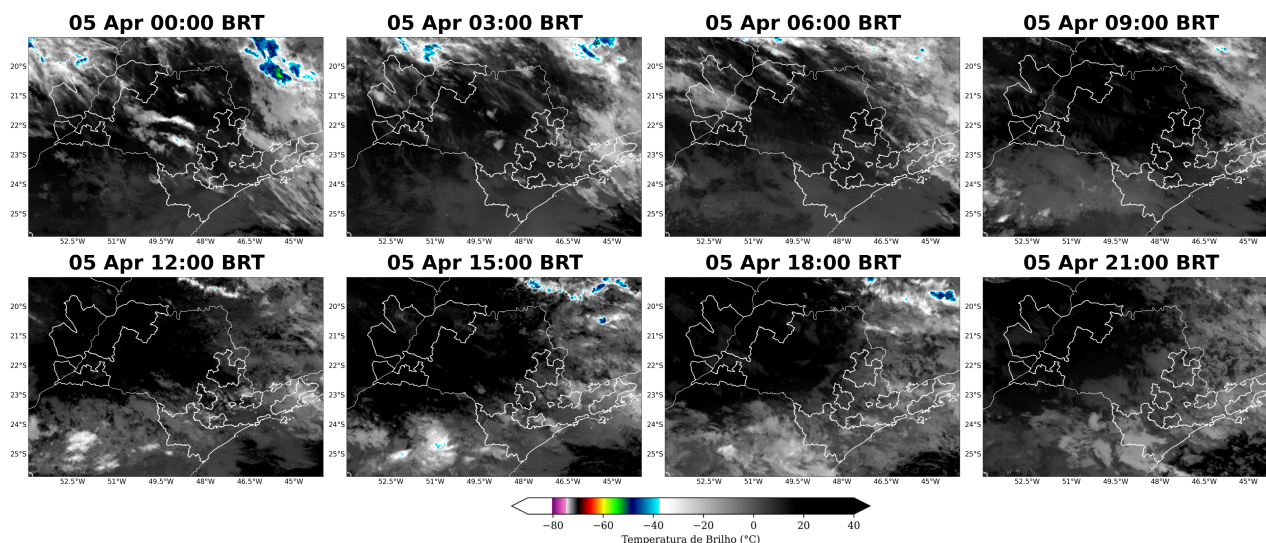
Figura 4: Imagens realçadas do satélite GOES-16 das 00 BRT até 21 BRT (a cada 3 horas) para o dia 05 de Abril.
