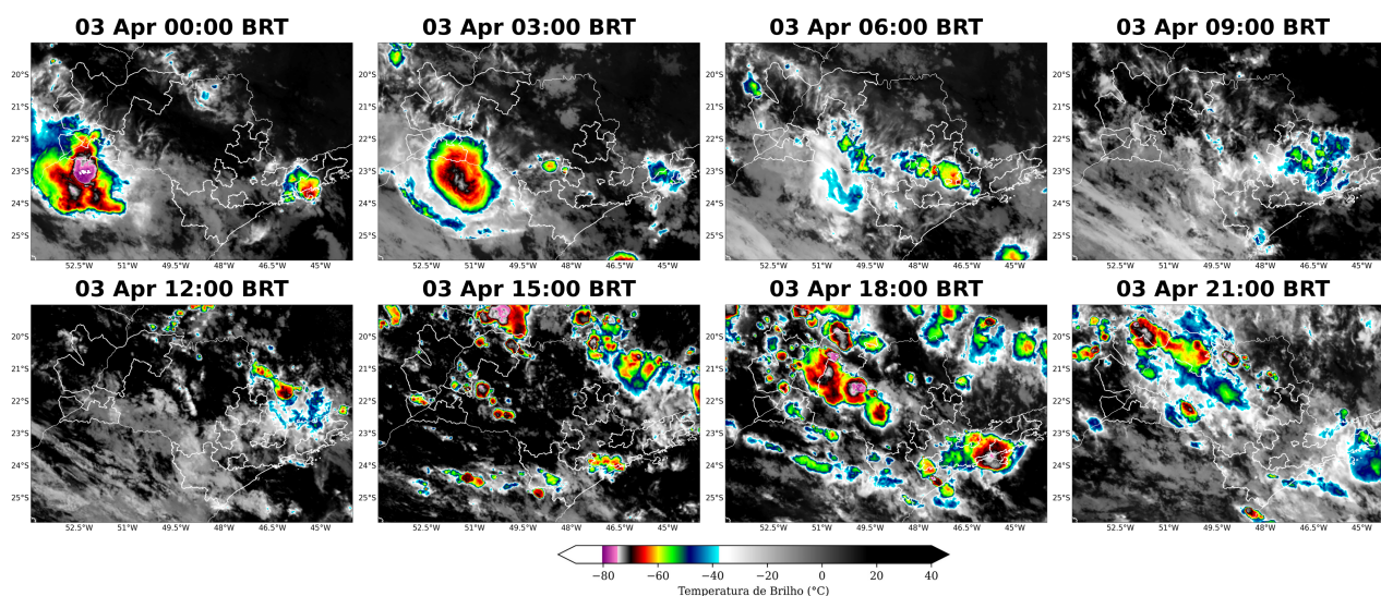
Figura 2: Imagens realçadas do satélite GOES-16 das 00 BRT até 21 BRT (a cada 3 horas) para o dia 03 de Abril.
