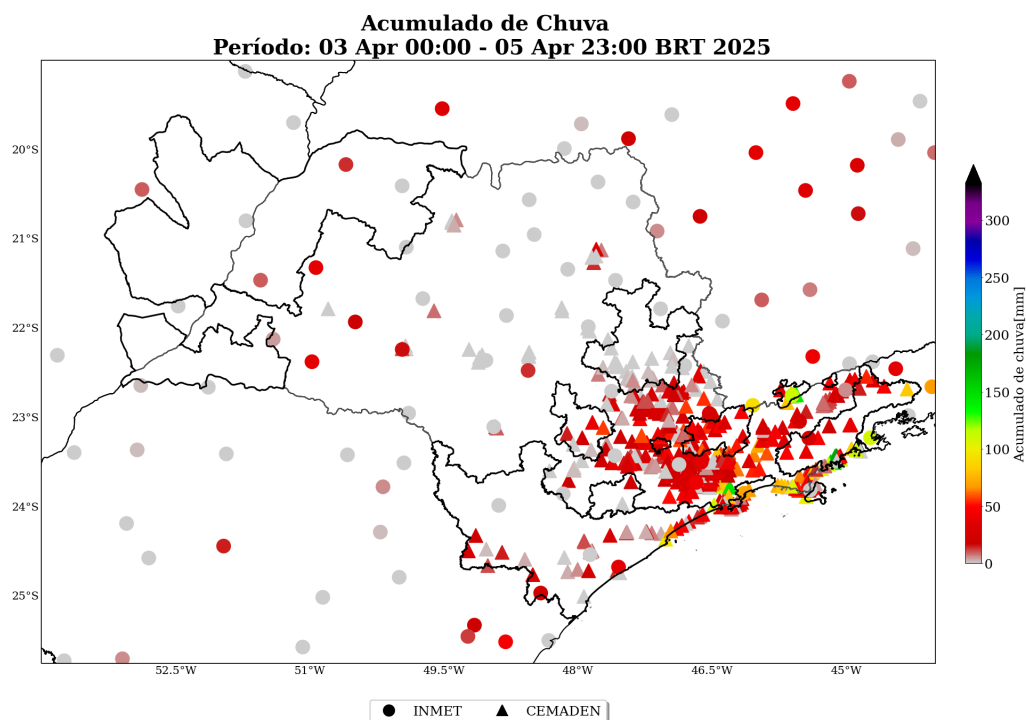
Figura 11: Acumulado de precipitação sobre a área de concessão da Neoenergia Elektro para o período do evento (dias 03 a 05 de Abril de 2025), baseado nas estações meteorológicas do INMET e CEMADEN.
