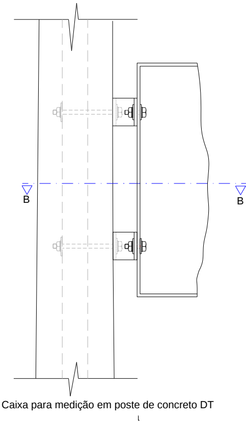
Figura 41 – Sugestões de Fixação da Caixa de Medição em Poste
