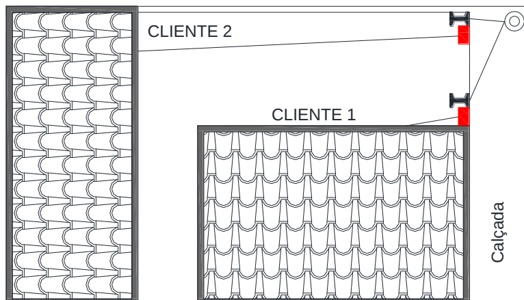
Figura 33 – Disposição da Entrada de Serviço – 4/4
