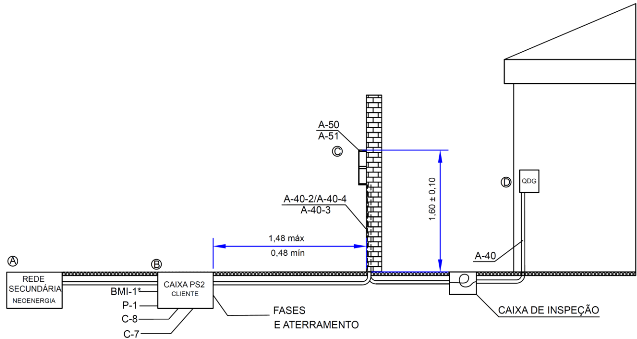
Figura 9 – Entrada de Serviço Subterrânea Derivada de Rede Subterrânea
