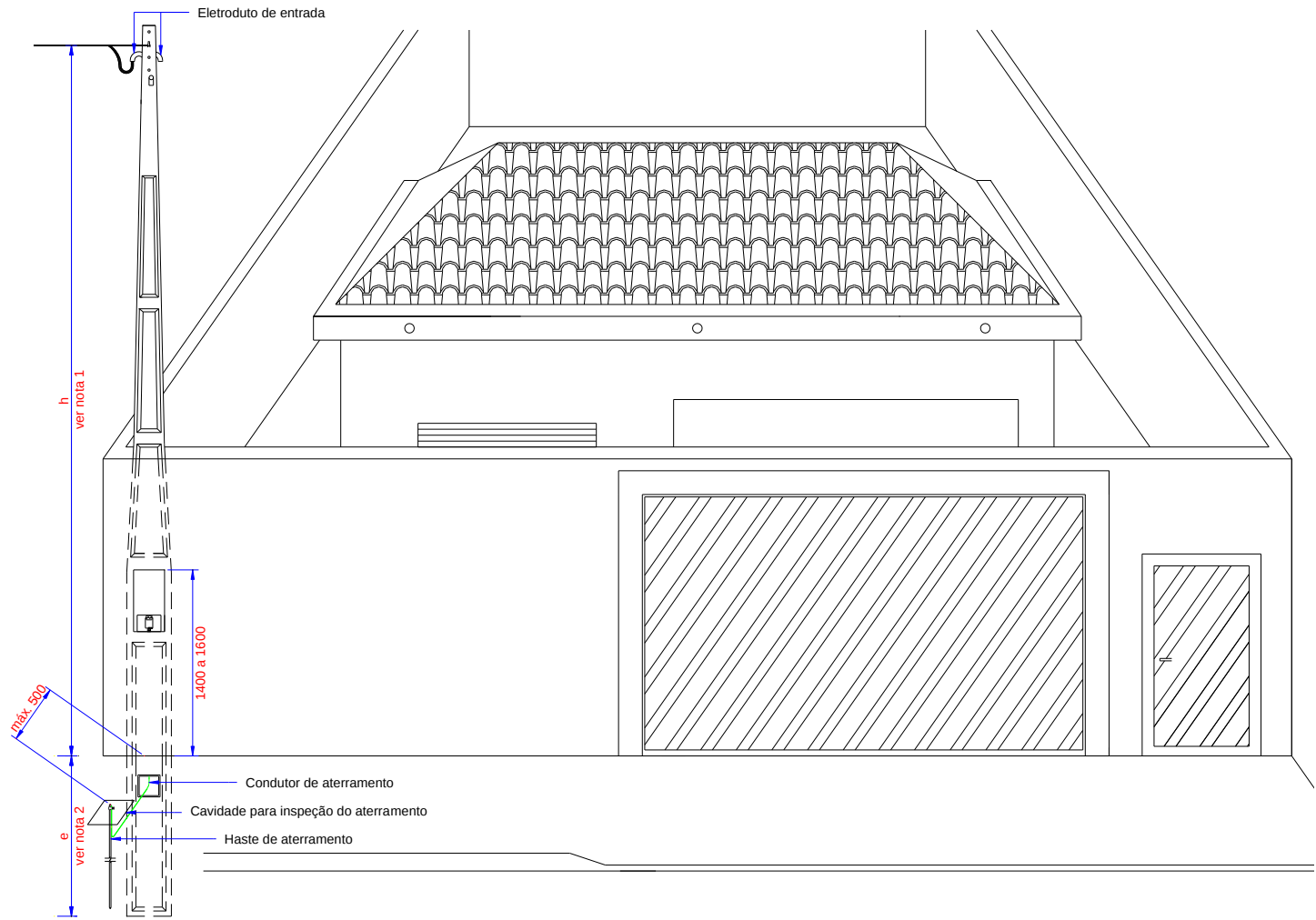
Figura 35 – Dimensões Gerais para Instalação em Muro
