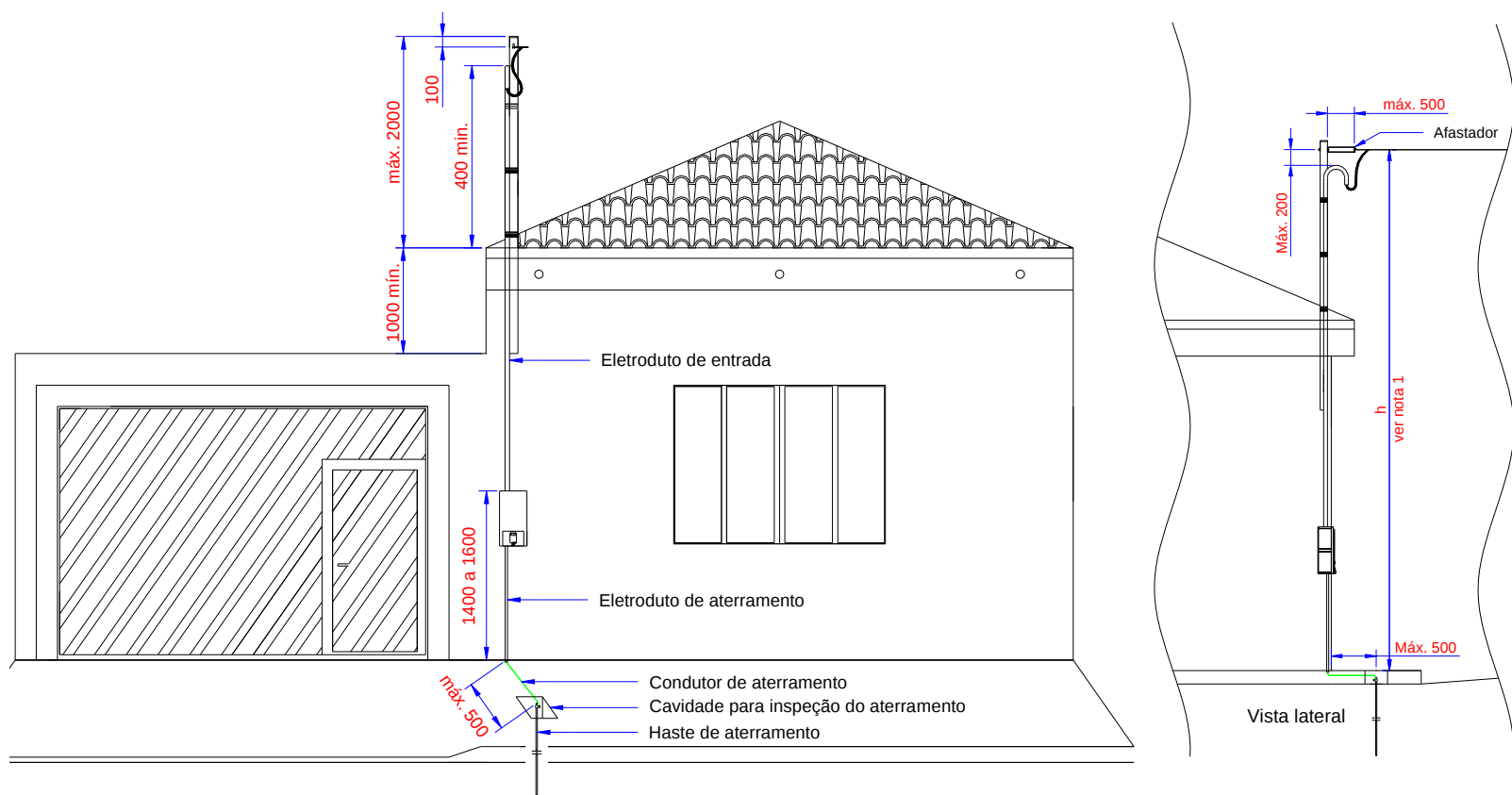
Figura 37 – Dimensões Gerais para instalação em Pontalete – 1/2
