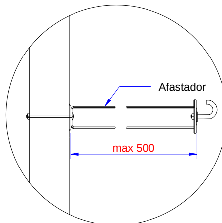
ILUSTRAÇÃO 7 AFASTADOR
