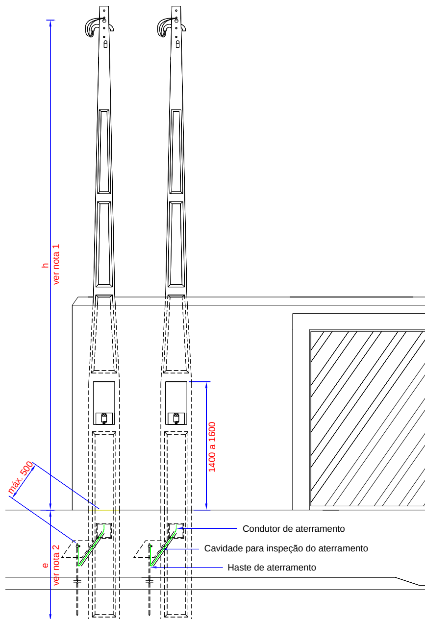
Figura 36 – Dimensões Gerais para Duas Ligações Instaladas em Muro
