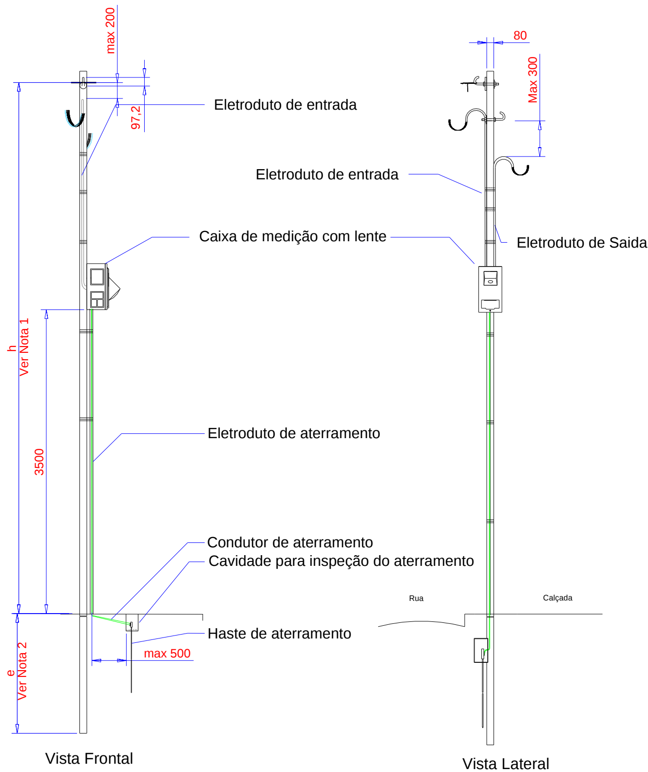
Figura 38 – Dimensões Gerais para Instalação com Caixas com Lente de Aumento – 1/2
