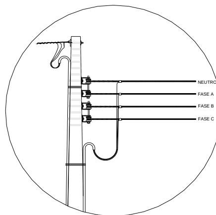
ILUSTRAÇÃO 5 SAÍDA AÉREA
