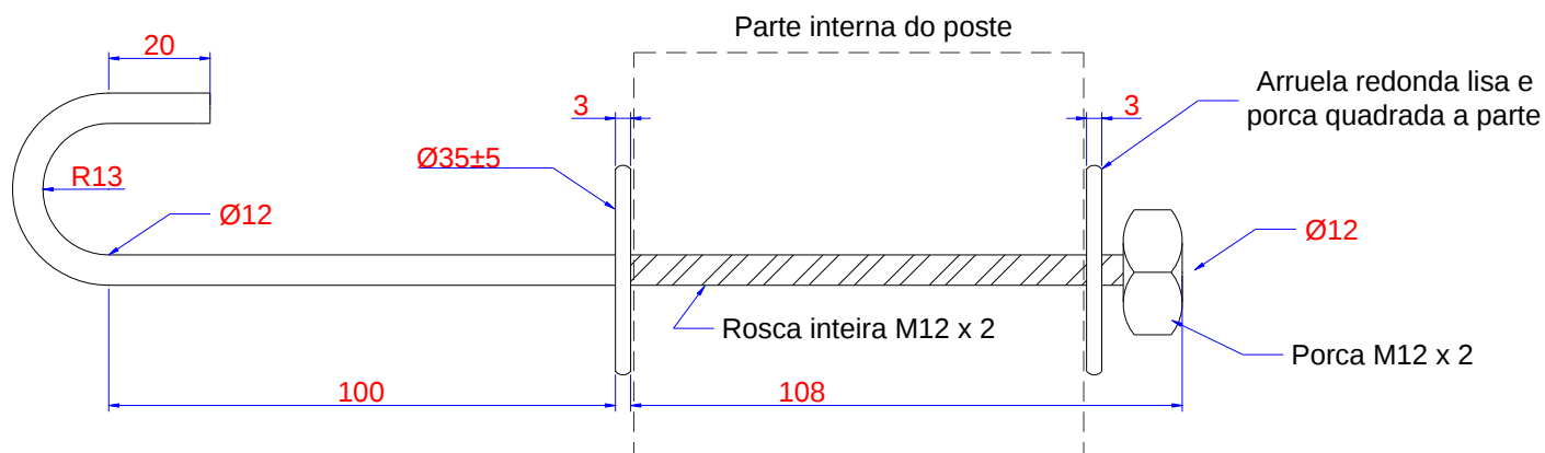
Figura 42a – Gancho Olhal Aberto para Ancoragem de Ramal no Poste
