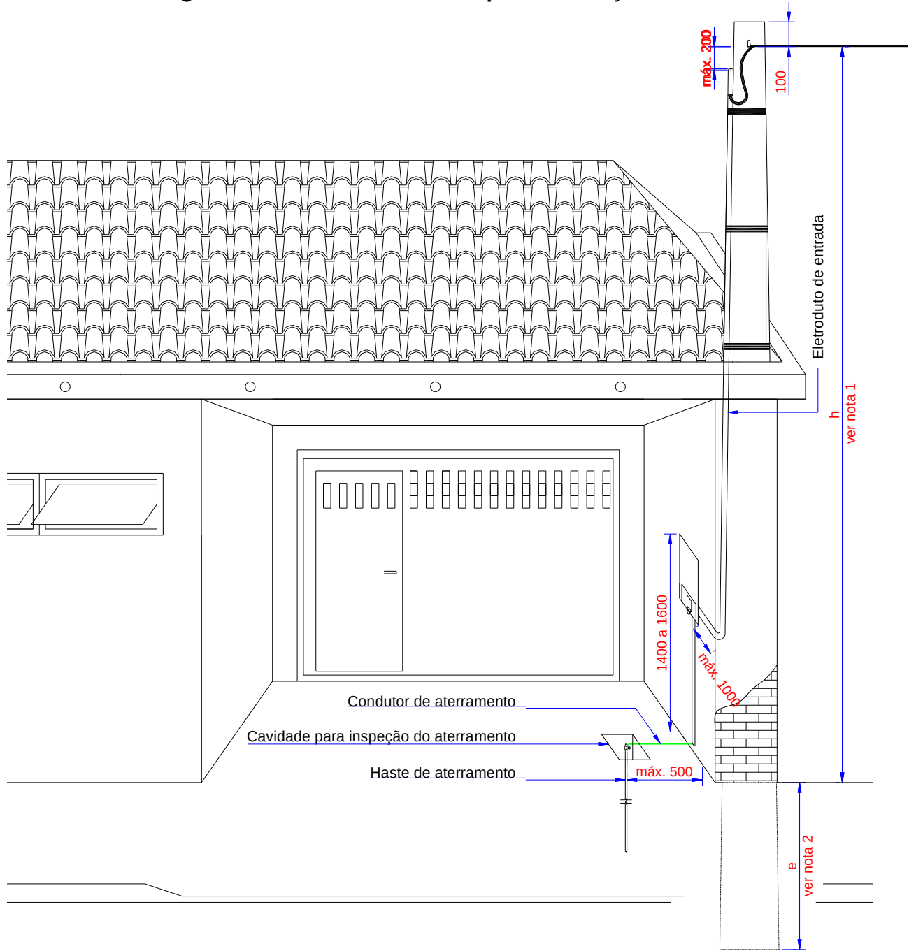
Figura 34 – Dimensões Gerais para Instalação Lateral
