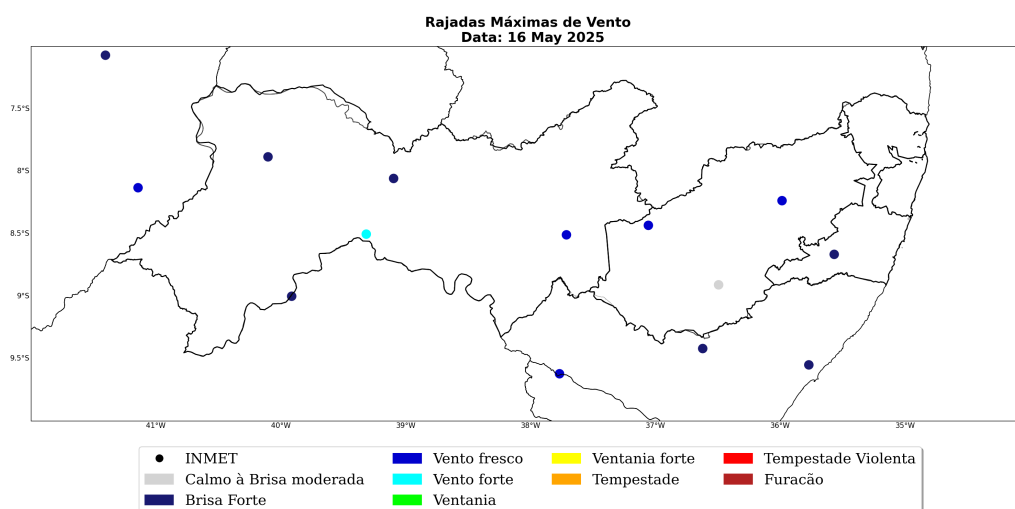
Figura 37: Máxima rajada de vento diária sobre a área de concessão da Neoenergia-PE para o dia 16 de Maio, baseado nas estações meteorológicas do INMET.
