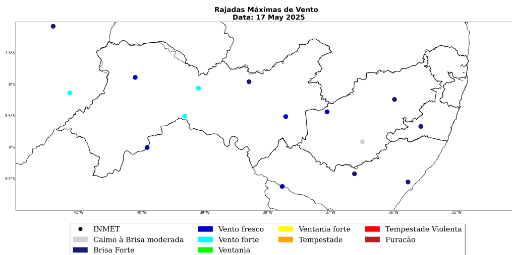
Figura 38: Máxima rajada de vento diária sobre a área de concessão da Neoenergia-PE para o dia 17 de Maio, baseado nas estações meteorológicas do INMET.
