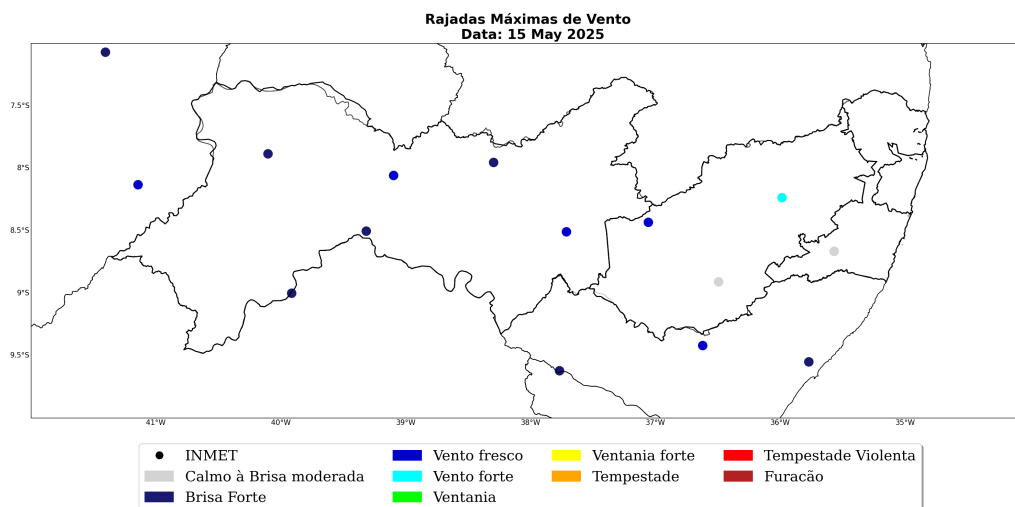
Figura 36: Máxima rajada de vento diária sobre a área de concessão da Neoenergia-PE para o dia 15 de Maio, baseado nas estações meteorológicas do INMET.
