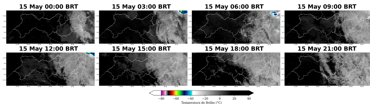
Figura 4: Imagens realçadas do satélite GOES-16 das 00 BRT até 21 BRT (a cada 3 horas) para o dia 15 de Maio.
