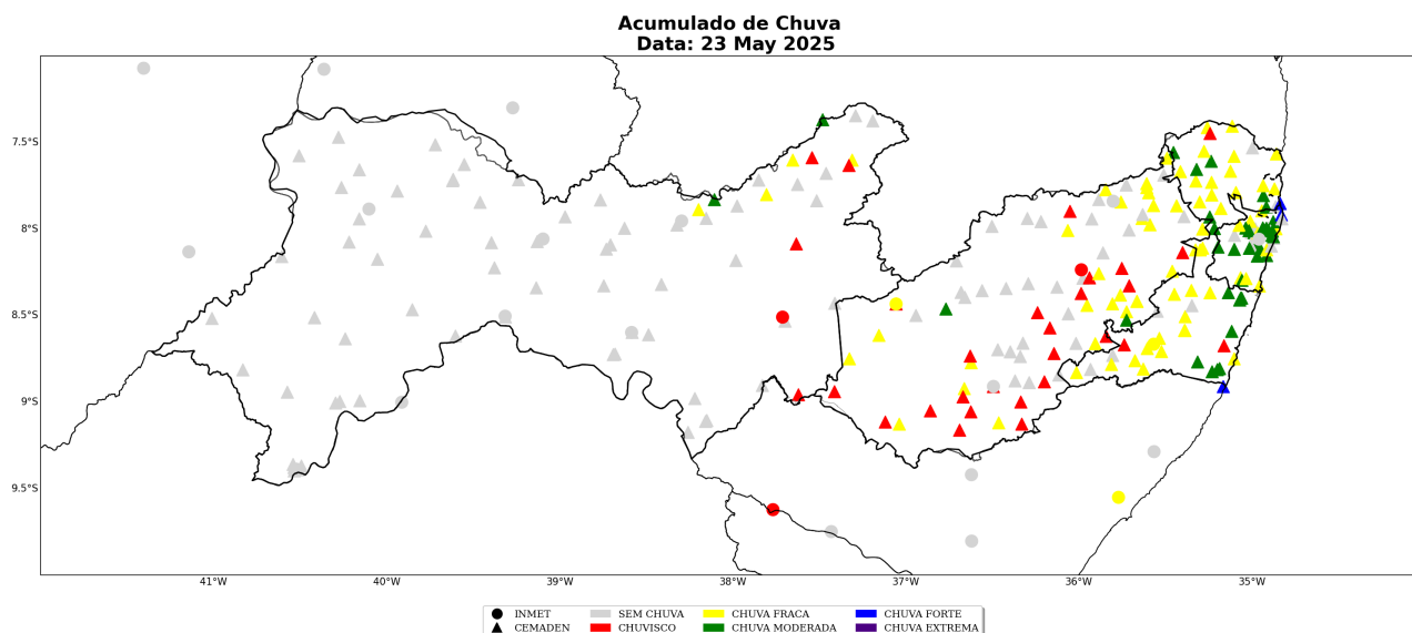
Figura 29: Acumulado diário de precipitação sobre a área de concessão da Neoenergia-PE para o dia 23 de Maio, baseado nas estações meteorológicas do INMET e CEMADEN.
