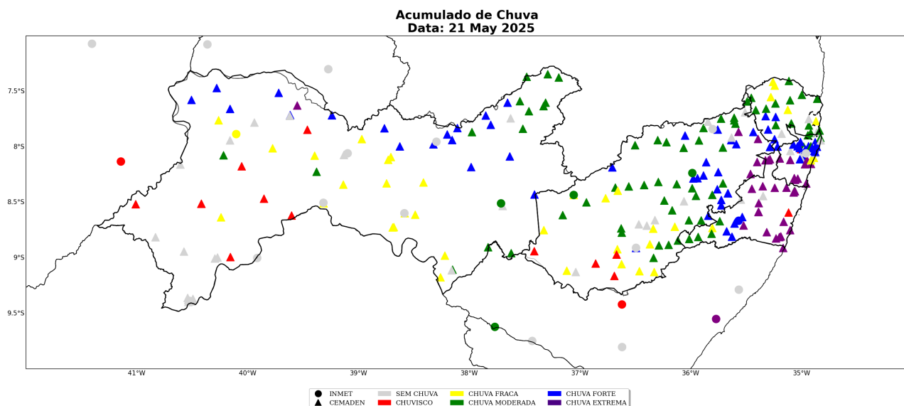
Figura 27: Acumulado diário de precipitação sobre a área de concessão da Neoenergia-PE para o dia 21 de Maio, baseado nas estações meteorológicas do INMET e CEMADEN.
