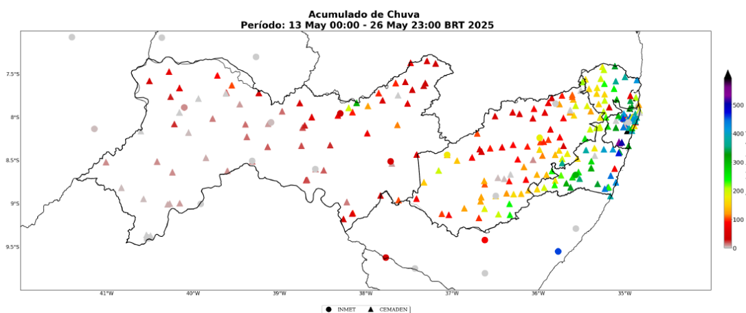
Figura 1 – representação da precipitação do período de 13 a 26 de maio
