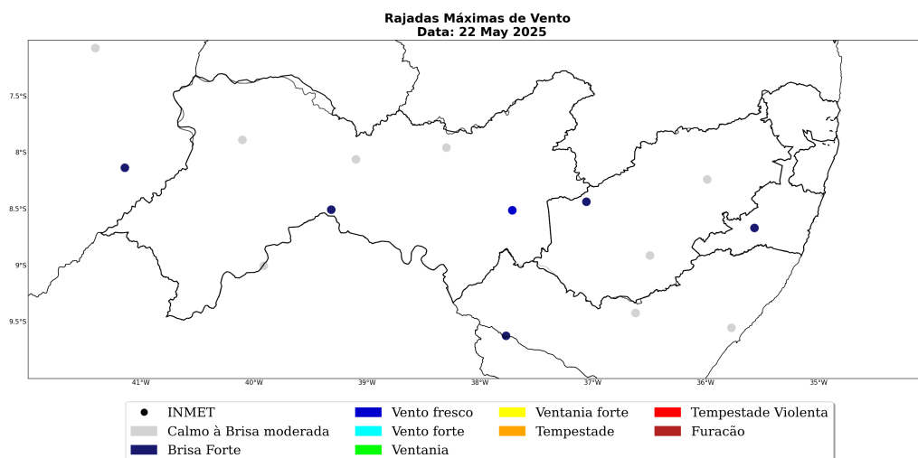
Figura 43: Máxima rajada de vento diária sobre a área de concessão da Neoenergia-PE para o dia 22 de Maio, baseado nas estações meteorológicas do INMET.
