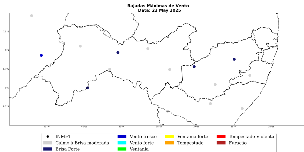
Figura 44: Máxima rajada de vento diária sobre a área de concessão da Neoenergia-PE para o dia 23 de Maio, baseado nas estações meteorológicas do INMET.
