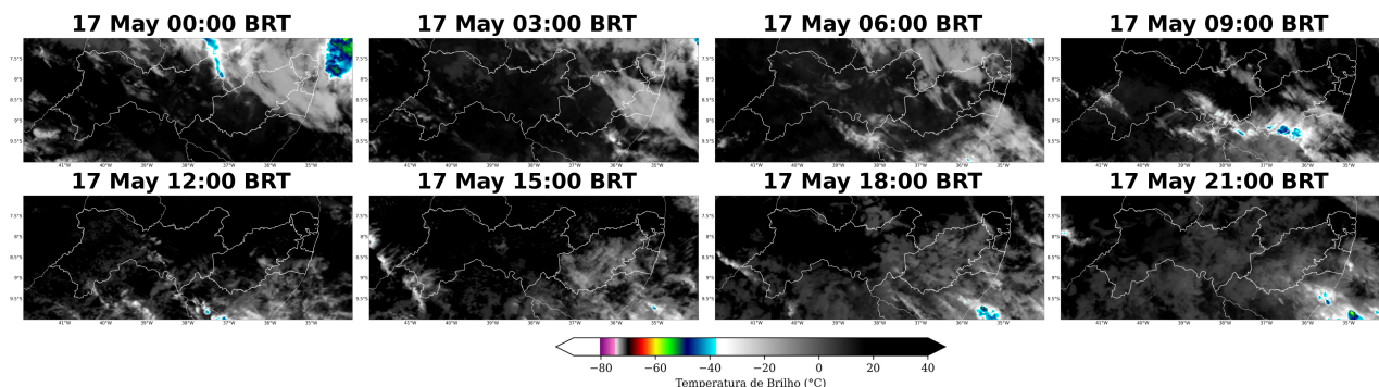
Figura 6: Imagens realçadas do satélite GOES-16 das 00 BRT até 21 BRT (a cada 3 horas) para o dia 17 de Maio.
