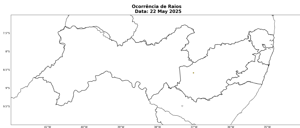
Figura 17: Ocorrências de descargas atmosféricas nuvem-solo detectadas pelo sistema Earth Networks para o dia 22 de Maio sobre a área de concessão da Neoenergia-PE.
