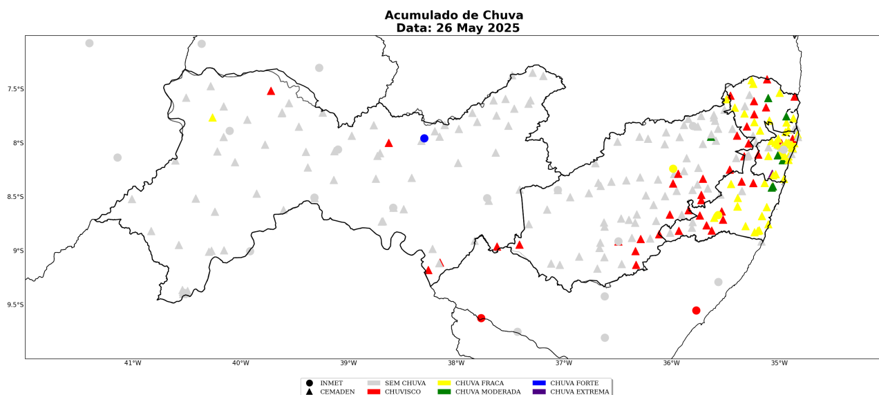
Figura 32: Acumulado diário de precipitação sobre a área de concessão da Neoenergia-PE para o dia 26 de Maio, baseado nas estações meteorológicas do INMET e CEMADEN.
