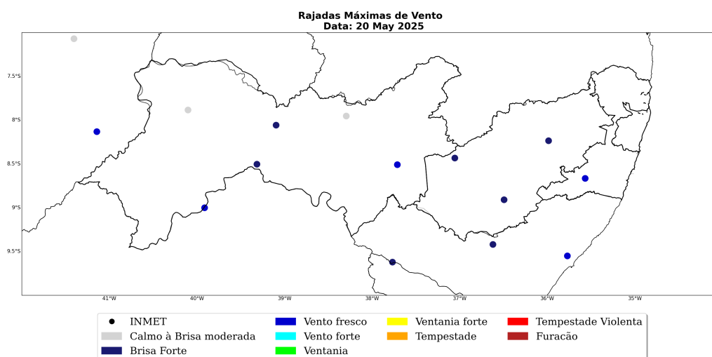
Figura 41: Máxima rajada de vento diária sobre a área de concessão da Neoenergia-PE para o dia 20 de Maio, baseado nas estações meteorológicas do INMET.
