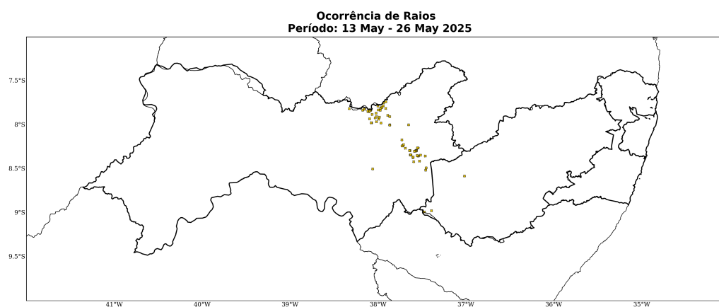
Figura 18: Ocorrências de descargas atmosféricas nuvem-solo detectadas pelo sistema Earth Networks para o período de 13 a 26 de Maio de 2025 sobre a área de concessão da Neoenergia-PE.
