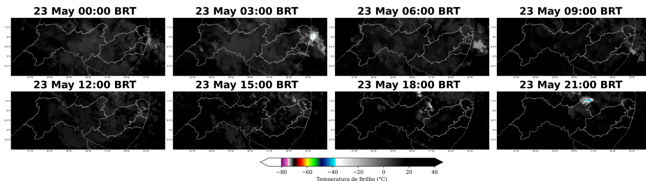
Figura 12: Imagens realçadas do satélite GOES-16 das 00 BRT até 21 BRT (a cada 3 horas) para o dia 23 de Maio.
