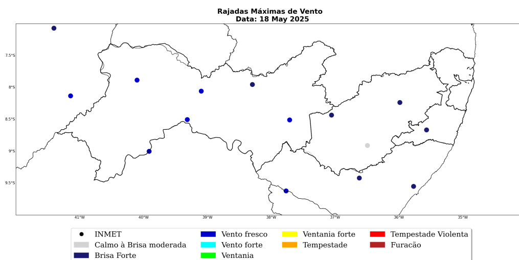
Figura 39: Máxima rajada de vento diária sobre a área de concessão da Neoenergia-PE para o dia 18 de Maio, baseado nas estações meteorológicas do INMET.
