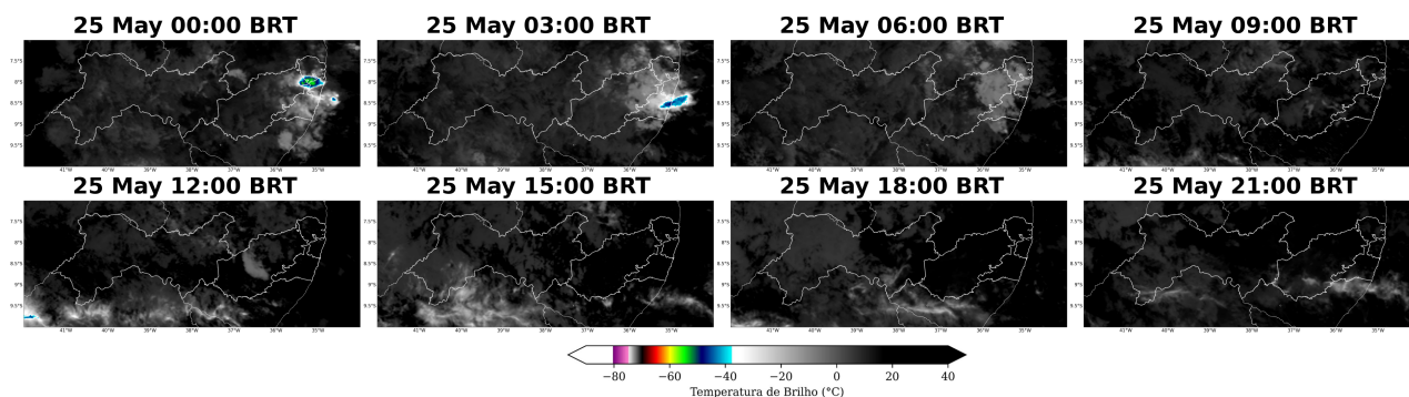
Figura 14: Imagens realçadas do satélite GOES-16 das 00 BRT até 21 BRT (a cada 3 horas) para o dia 25 de Maio.
