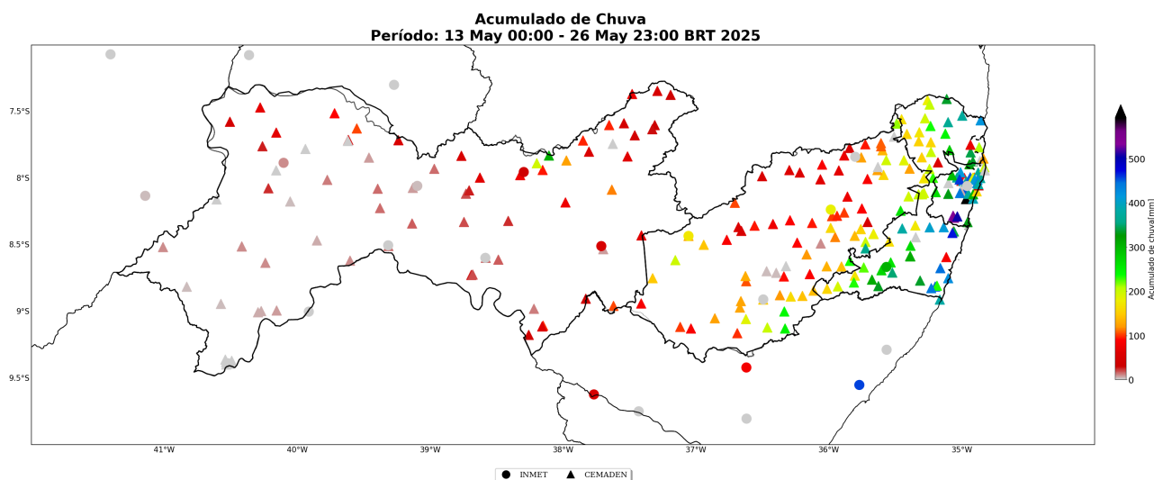
Figura 33: Acumulado de precipitação sobre o estado de Pernambuco para o período do evento (dias 13 a 26 de Maio de 2025), baseado nas estações meteorológicas do INMET e CEMADEN.
