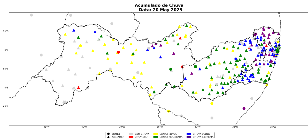
Figura 26: Acumulado diário de precipitação sobre a área de concessão da Neoenergia-PE para o dia 20 de Maio, baseado nas estações meteorológicas do INMET e CEMADEN.
