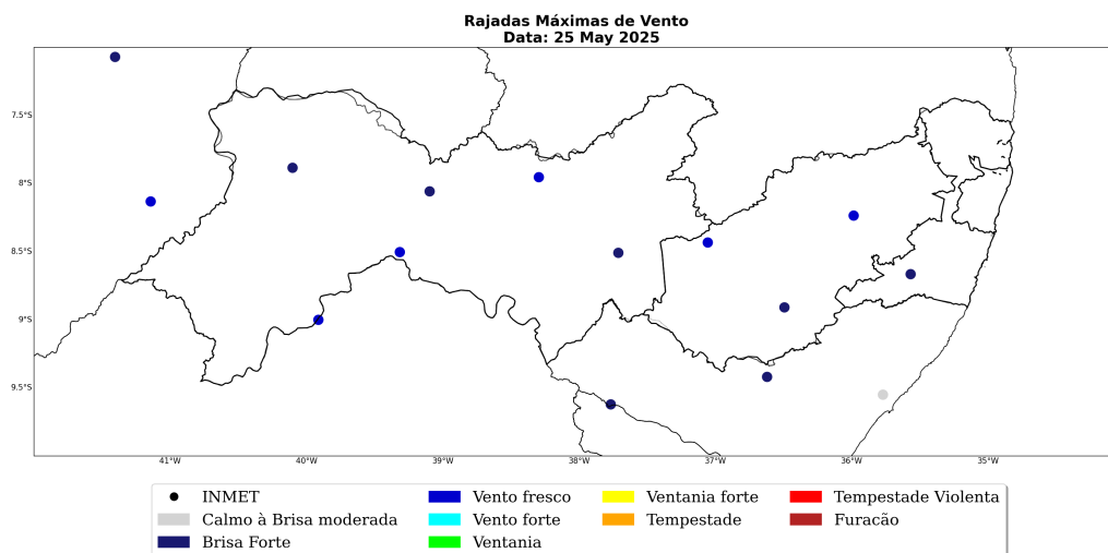
Figura 46: Máxima rajada de vento diária sobre a área de concessão da Neoenergia-PE para o dia 25 de Maio, baseado nas estações meteorológicas do INMET.
