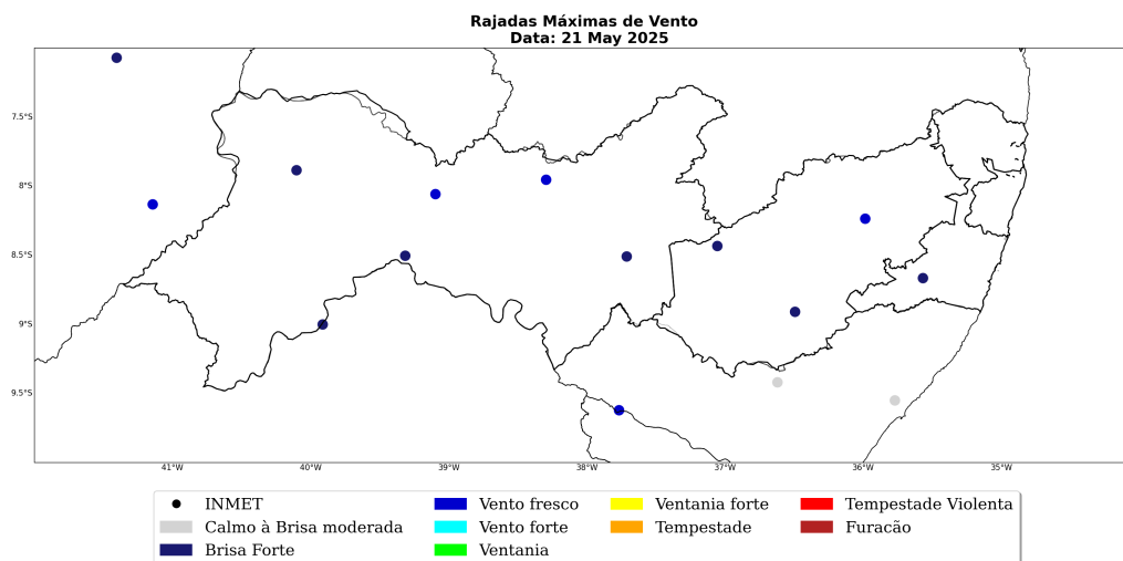
Figura 42: Máxima rajada de vento diária sobre a área de concessão da Neoenergia-PE para o dia 21 de Maio, baseado nas estações meteorológicas do INMET.
