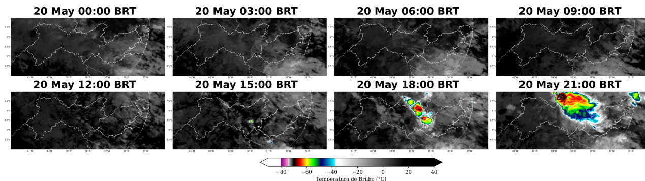
Figura 9: Imagens realçadas do satélite GOES-16 das 00 BRT até 21 BRT (a cada 3 horas) para o dia 20 de Maio.
