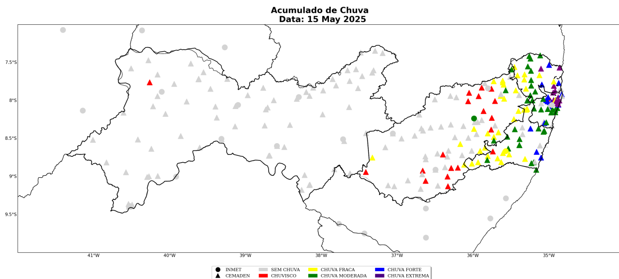
Figura 21: Acumulado diário de precipitação sobre a área de concessão da Neoenergia-PE para o dia 15 de Maio, baseado nas estações meteorológicas do INMET e CEMADEN.
