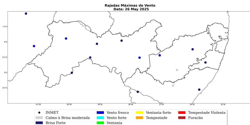
Figura 47: Máxima rajada de vento diária sobre a área de concessão da Neoenergia-PE para o dia 26 de Maio, baseado nas estações meteorológicas do INMET.
