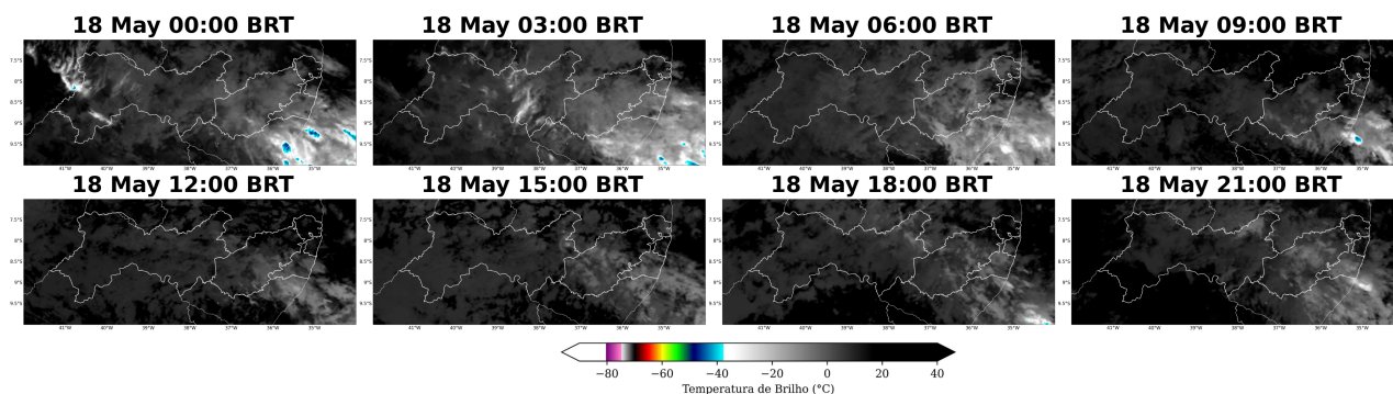
Figura 7: Imagens realçadas do satélite GOES-16 das 00 BRT até 21 BRT (a cada 3 horas) para o dia 18 de Maio.
