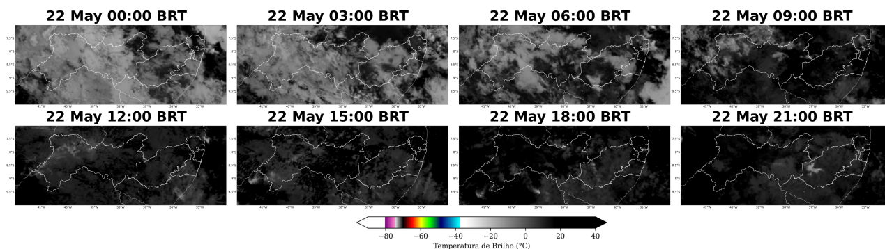
Figura 11: Imagens realçadas do satélite GOES-16 das 00 BRT até 21 BRT (a cada 3 horas) para o dia 22 de Maio.
