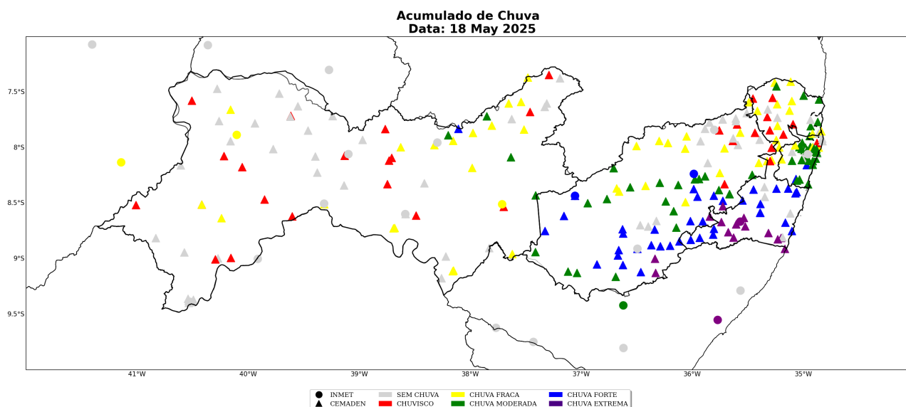
Figura 24: Acumulado diário de precipitação sobre a área de concessão da Neoenergia-PE para o dia 18 de Maio, baseado nas estações meteorológicas do INMET e CEMADEN.
