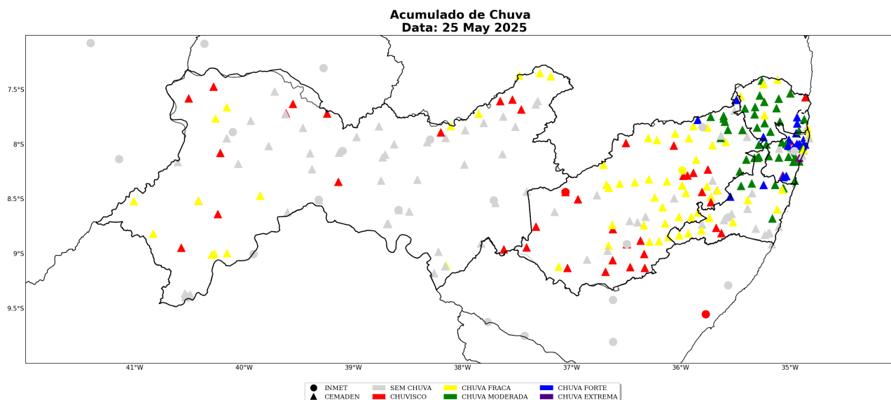
Figura 31: Acumulado diário de precipitação sobre a área de concessão da Neoenergia-PE para o dia 25 de Maio, baseado nas estações meteorológicas do INMET e CEMADEN.
