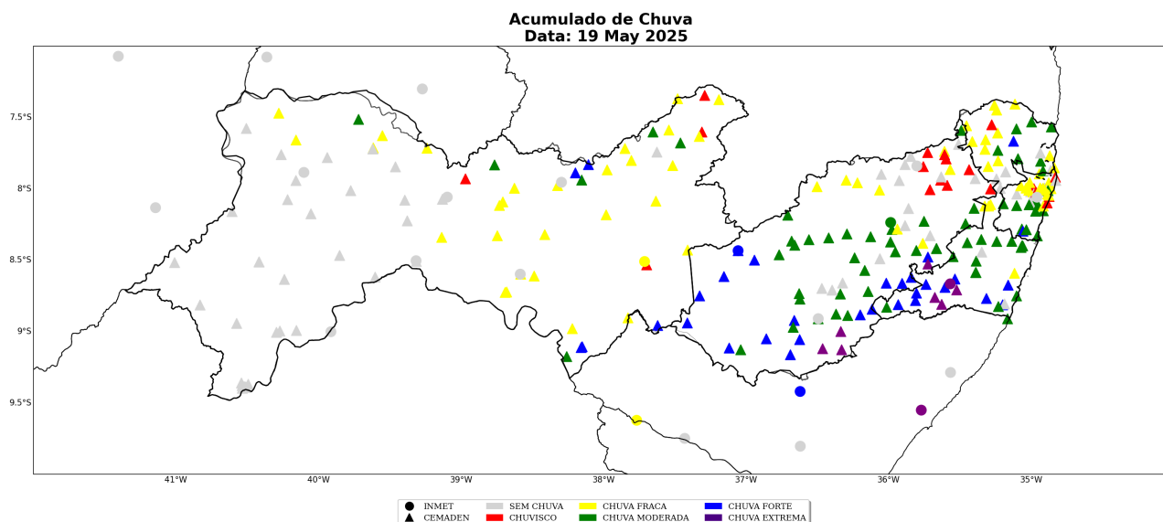
Figura 25: Acumulado diário de precipitação sobre a área de concessão da Neoenergia-PE para o dia 19 de Maio, baseado nas estações meteorológicas do INMET e CEMADEN.
