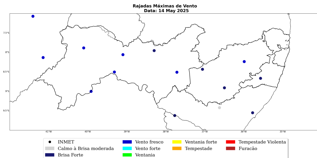
Figura 35: Máxima rajada de vento diária sobre a área de concessão da Neoenergia-PE para o dia 14 de Maio, baseado nas estações meteorológicas do INMET.
