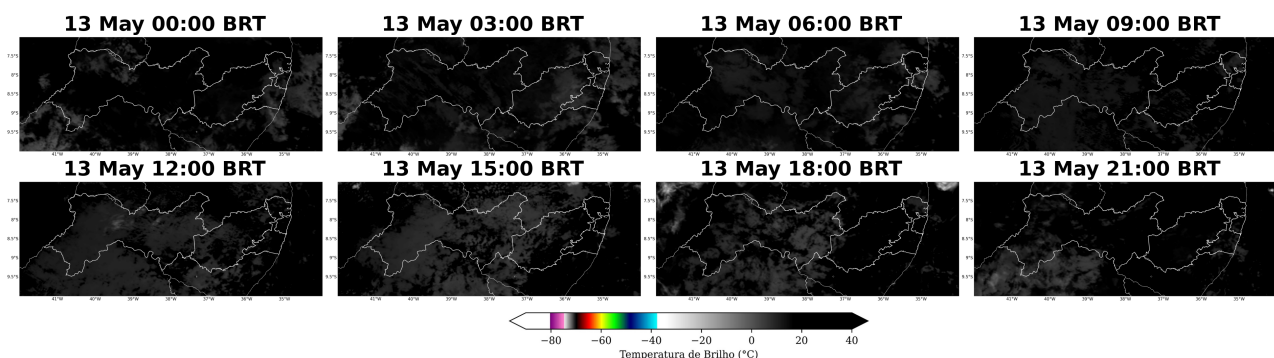
Figura 2: Imagens realçadas do satélite GOES-16 das 00 BRT até 21 BRT (a cada 3 horas) para o dia 13 de Maio.
