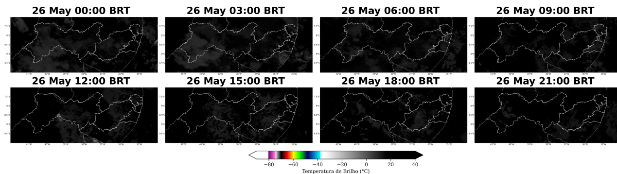
Figura 15: Imagens realçadas do satélite GOES-16 das 00 BRT até 21 BRT (a cada 3 horas) para o dia 26 de Maio.
