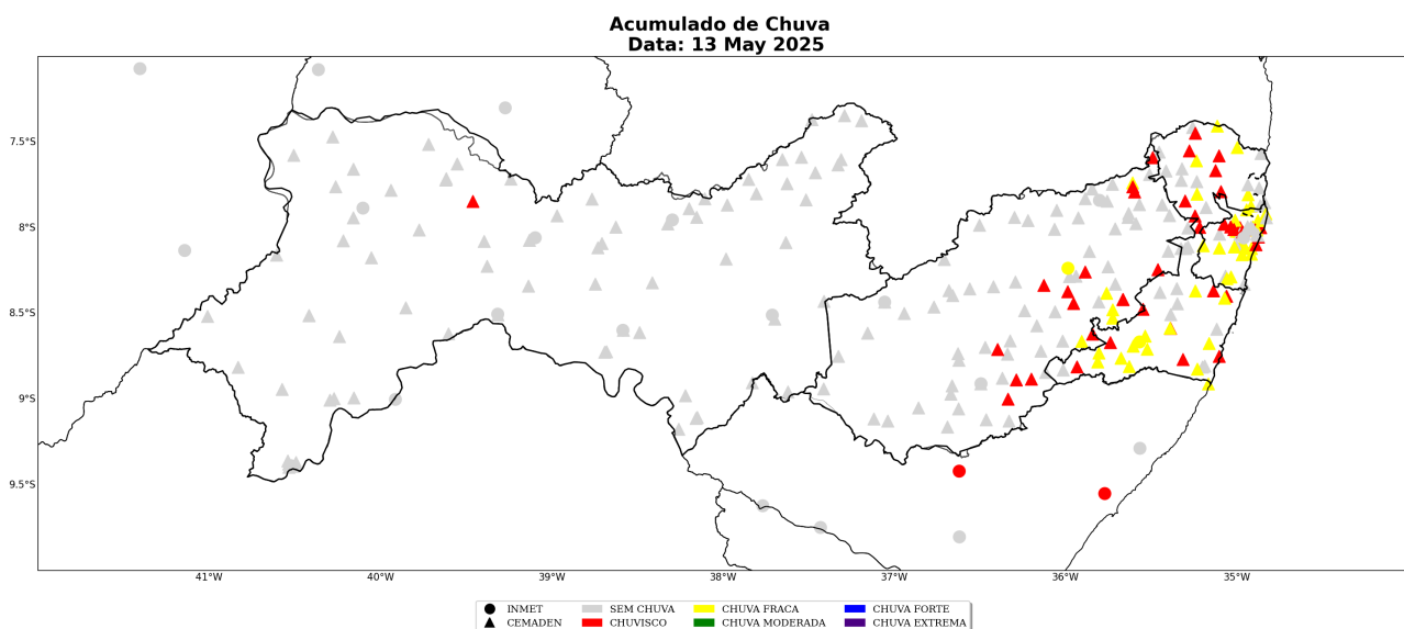
Figura 19: Acumulado diário de precipitação sobre a área de concessão da Neoenergia-PE para o dia 13 de Maio, baseado nas estações meteorológicas do INMET e CEMADEN.
