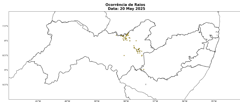
Figura 16: Ocorrências de descargas atmosféricas nuvem-solo detectadas pelo sistema Earth Networks para o dia 20 de Maio sobre a área de concessão da Neoenergia-PE.
