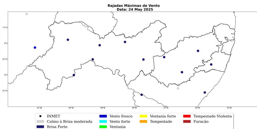
Figura 45: Máxima rajada de vento diária sobre a área de concessão da Neoenergia-PE para o dia 24 de Maio, baseado nas estações meteorológicas do INMET.
