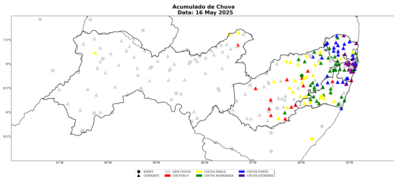
Figura 22: Acumulado diário de precipitação sobre a área de concessão da Neoenergia-PE para o dia 16 de Maio, baseado nas estações meteorológicas do INMET e CEMADEN.
