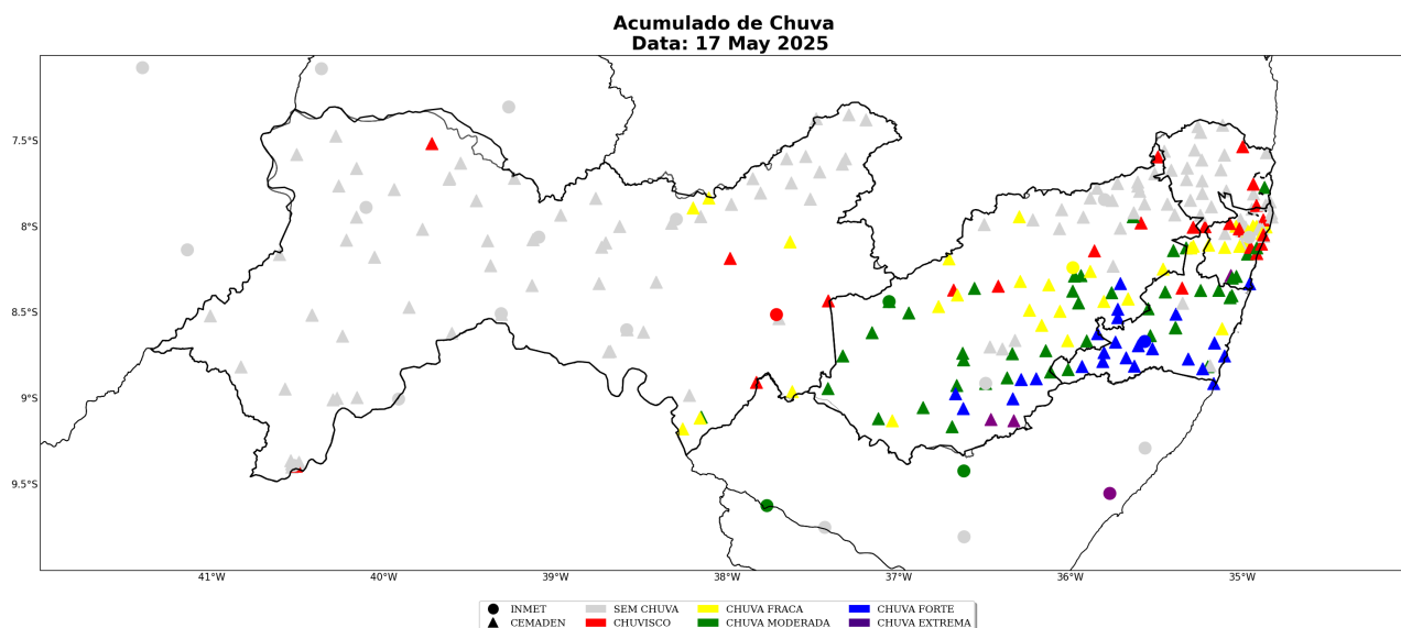
Figura 23: Acumulado diário de precipitação sobre a área de concessão da Neoenergia-PE para o dia 17 de Maio, baseado nas estações meteorológicas do INMET e CEMADEN.
