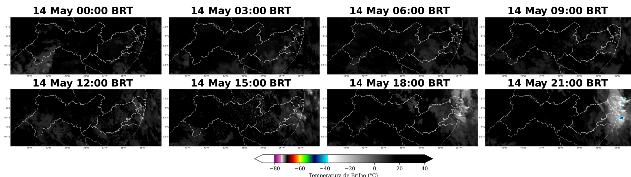
Figura 3: Imagens realçadas do satélite GOES-16 das 00 BRT até 21 BRT (a cada 3 horas) para o dia 14 de Maio.
