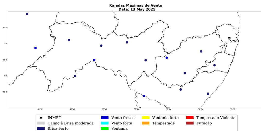
Figura 34: Máxima rajada de vento diária sobre a área de concessão da Neoenergia-PE para o dia 13 de Maio, baseado nas estações meteorológicas do INMET.
