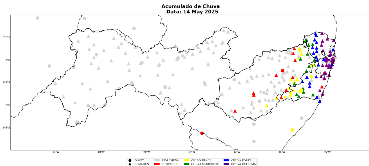
Figura 20: Acumulado diário de precipitação sobre a área de concessão da Neoenergia-PE para o dia 14 de Maio, baseado nas estações meteorológicas do INMET e CEMADEN.
