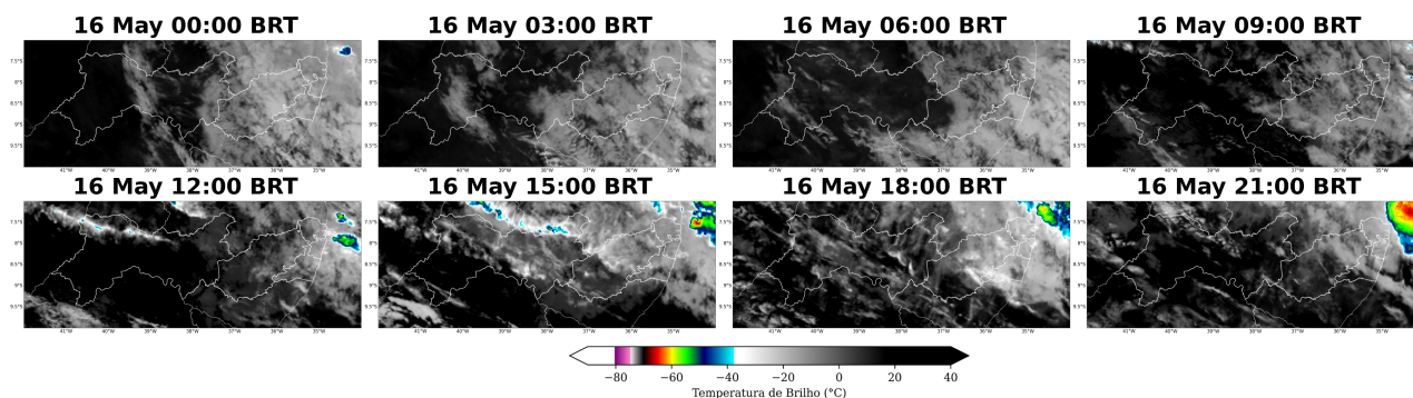
Figura 5: Imagens realçadas do satélite GOES-16 das 00 BRT até 21 BRT (a cada 3 horas) para o dia 16 de Maio.
