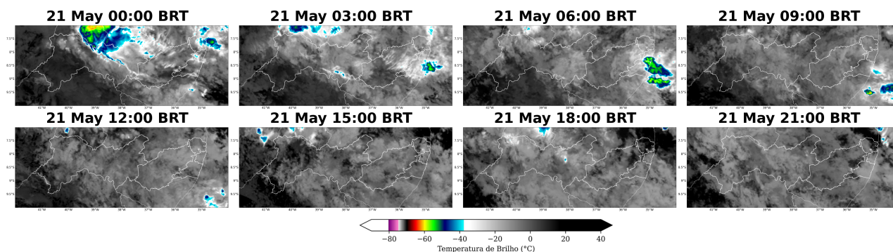
Figura 10: Imagens realçadas do satélite GOES-16 das 00 BRT até 21 BRT (a cada 3 horas) para o dia 21 de Maio.
