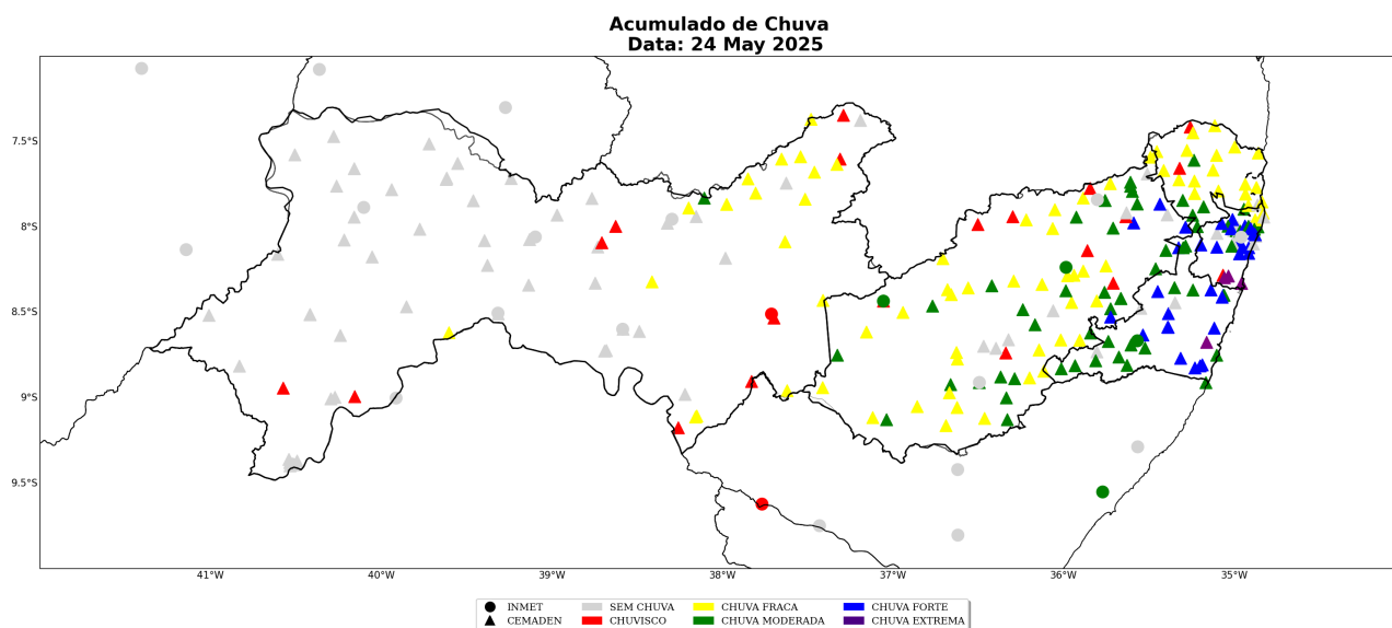
Figura 30: Acumulado diário de precipitação sobre a área de concessão da Neoenergia-PE para o dia 24 de Maio, baseado nas estações meteorológicas do INMET e CEMADEN.
