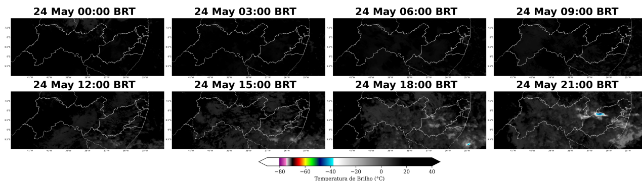
Figura 13: Imagens realçadas do satélite GOES-16 das 00 BRT até 21 BRT (a cada 3 horas) para o dia 24 de Maio.
