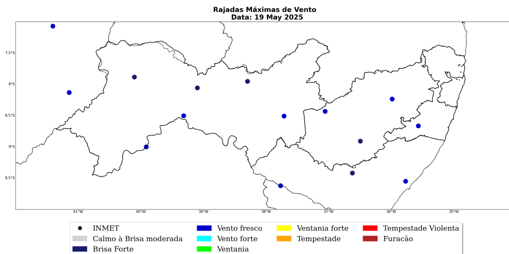
Figura 40: Máxima rajada de vento diária sobre a área de concessão da Neoenergia-PE para o dia 19 de Maio, baseado nas estações meteorológicas do INMET.
