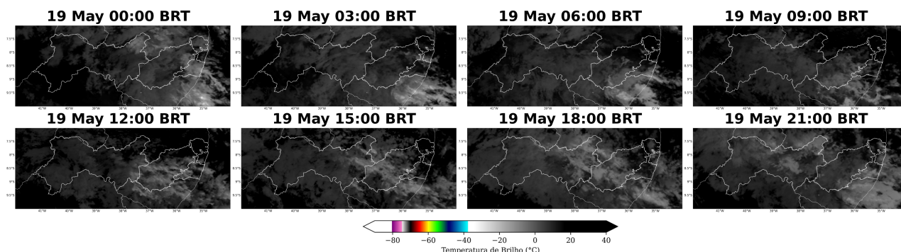
Figura 8: Imagens realçadas do satélite GOES-16 das 00 BRT até 21 BRT (a cada 3 horas) para o dia 19 de Maio.
