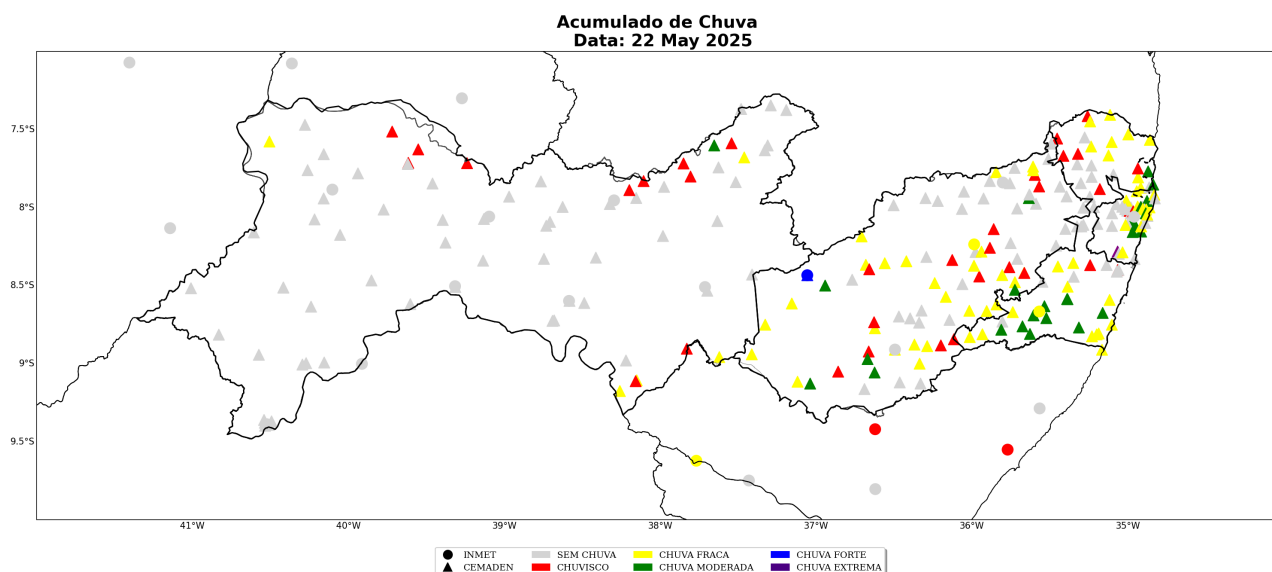
Figura 28: Acumulado diário de precipitação sobre a área de concessão da Neoenergia-PE para o dia 22 de Maio, baseado nas estações meteorológicas do INMET e CEMADEN.
