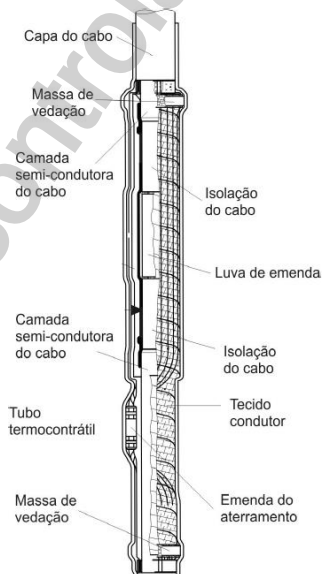
Figura 12 - Emenda Termocontrátil
