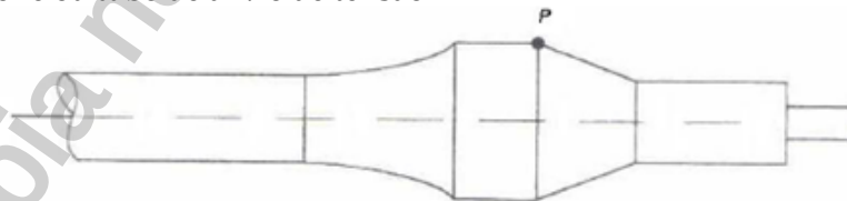
Figura 09 – Cone ou tubo de alívio de tensão
