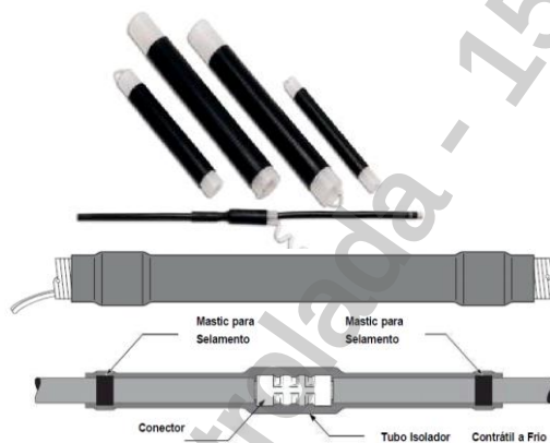
Figura 13 – Emenda Retrátil a Frio
