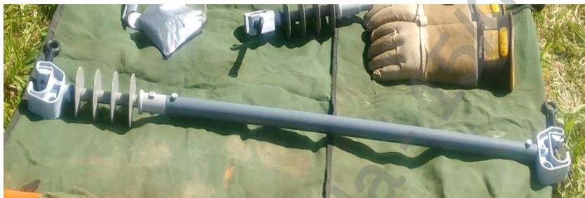
Figura 02 – Instalação da garra sem isolador com pino travante
