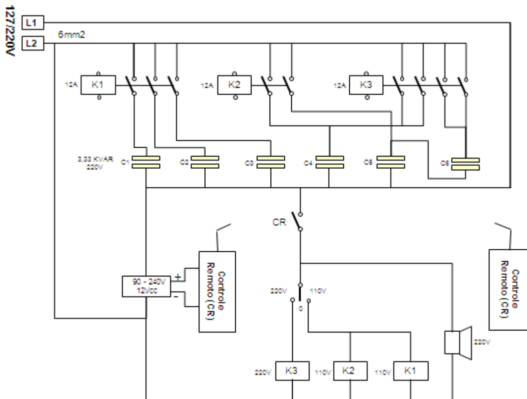
Circuito elétrico
