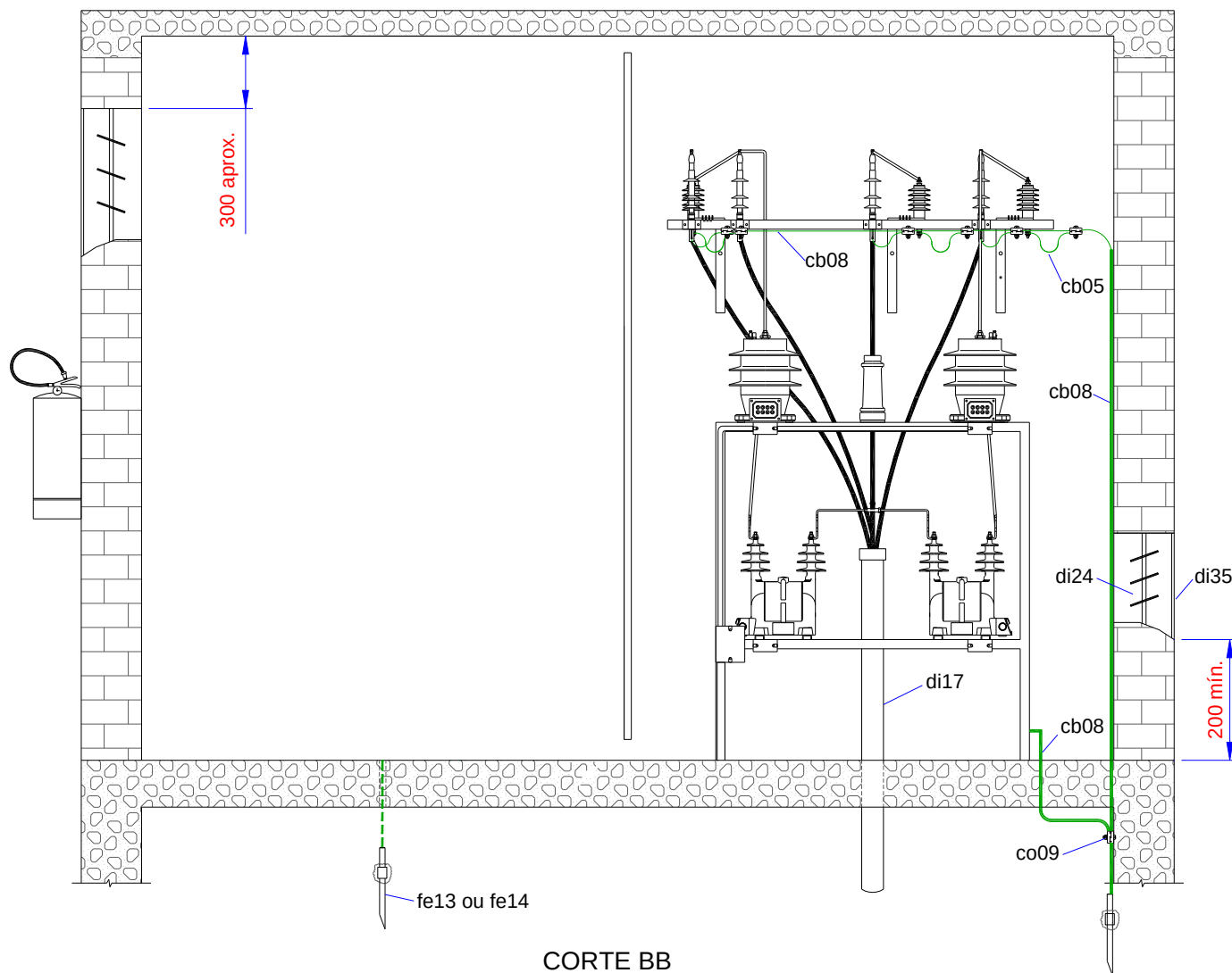
Figura 20 - Subestação Abrigada de Medição e Proteção Entrada Subterrânea – Medição AT (3/3)
