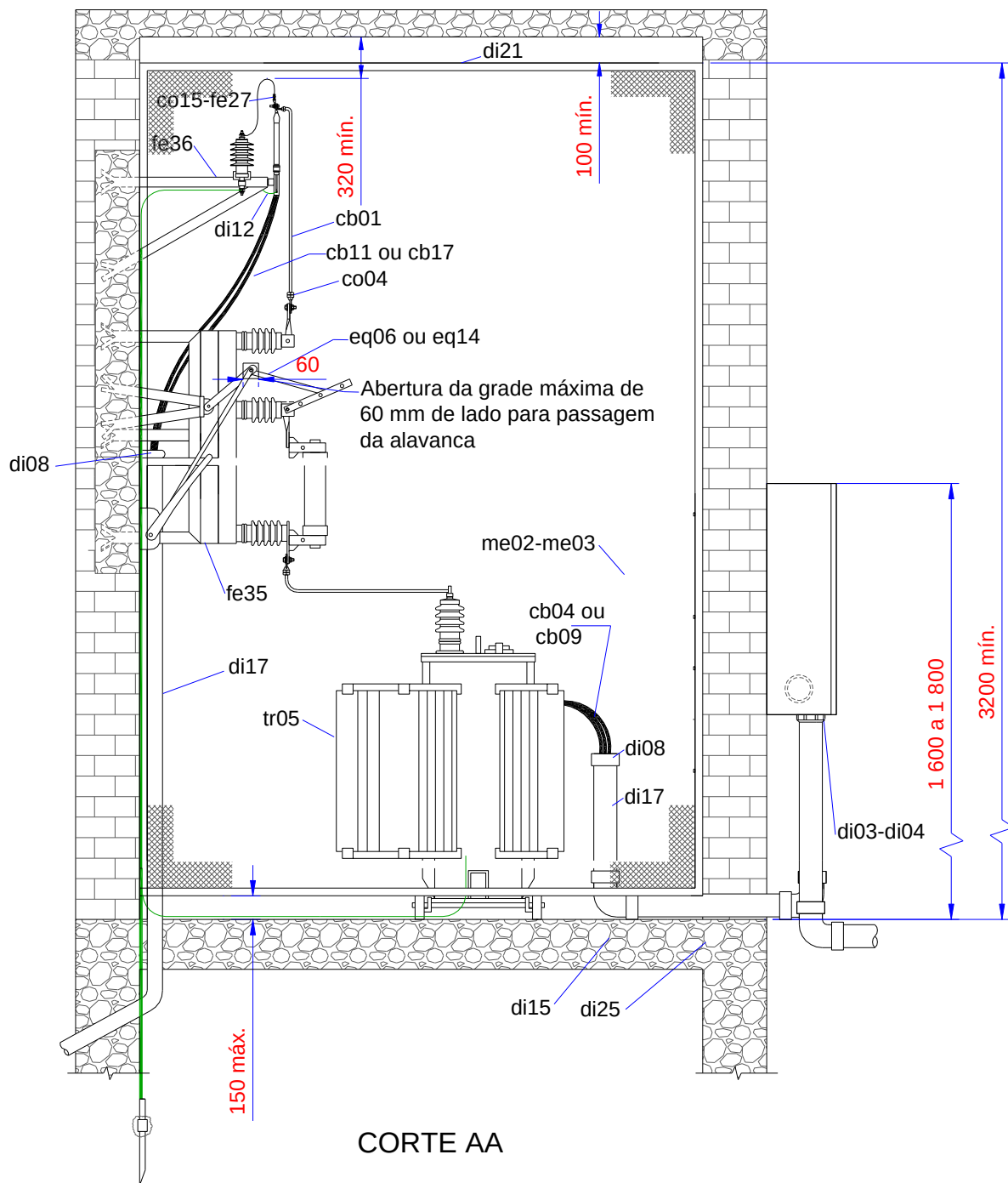
Figura 19 - Subestação Abrigada de Transformação Entrada Subterrânea – Medição BT (2/3)
