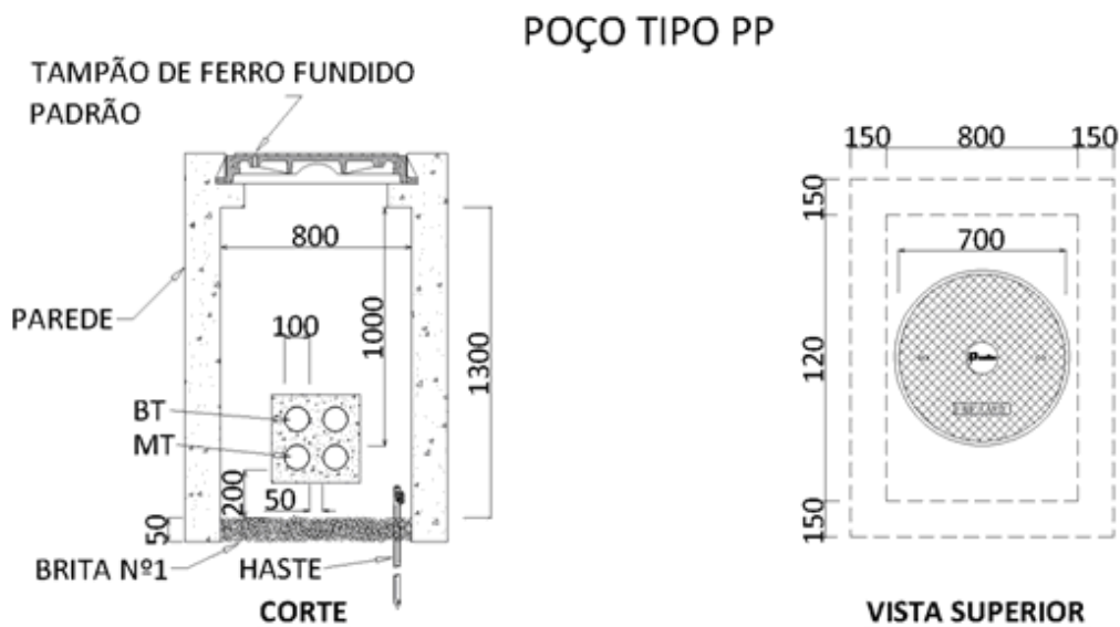
Figura 8 - Poço de Passagem para Ramal de Conexão Subterrâneo
