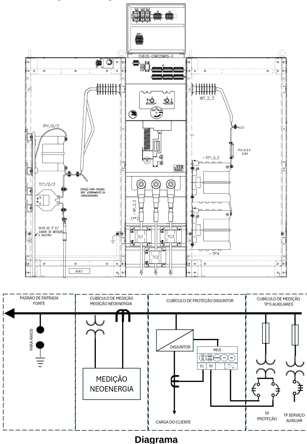
Figura 36 – Medição e Proteção até 300 kVA com Transformadores Auxiliares
