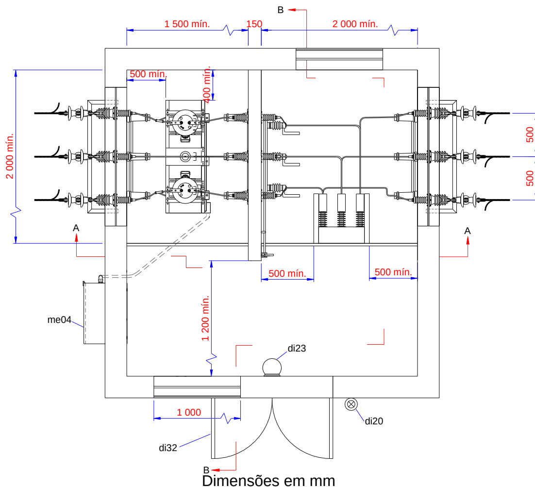
Figura 22 - Subestação Abrigada de Medição e Proteção Entrada Aérea – Medição AT (1/3)
