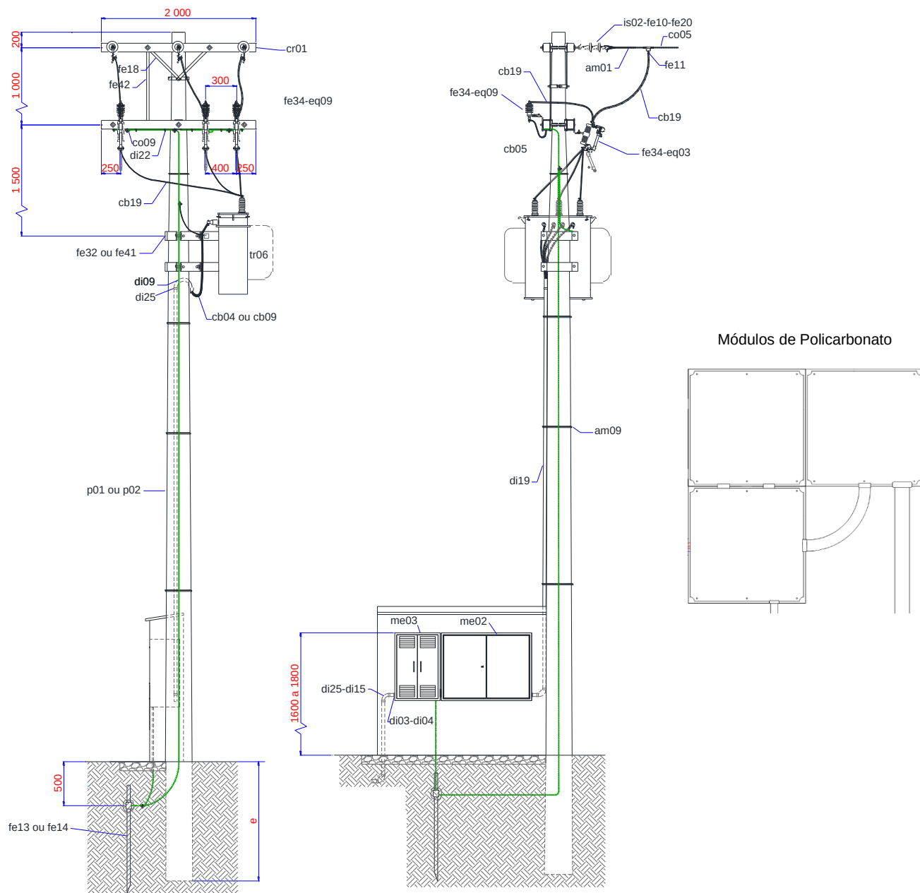
Figura 16 - Posto de Transformação em Poste 13,8 kV (Medição Indireta) (2/2) – Exclusivo Neoenergia Elektro
