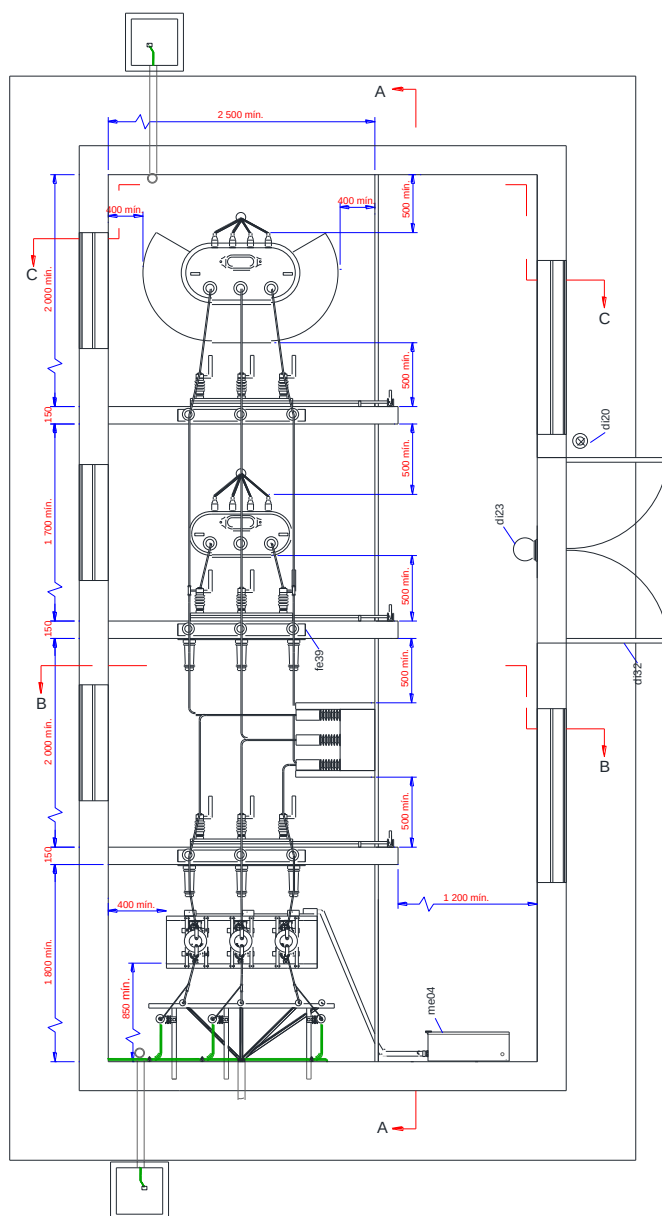
Figura 25 - Subestação Abrigada de Medição, Proteção e Transformação - Entrada Subterrânea – Medição em AT (1/4)
