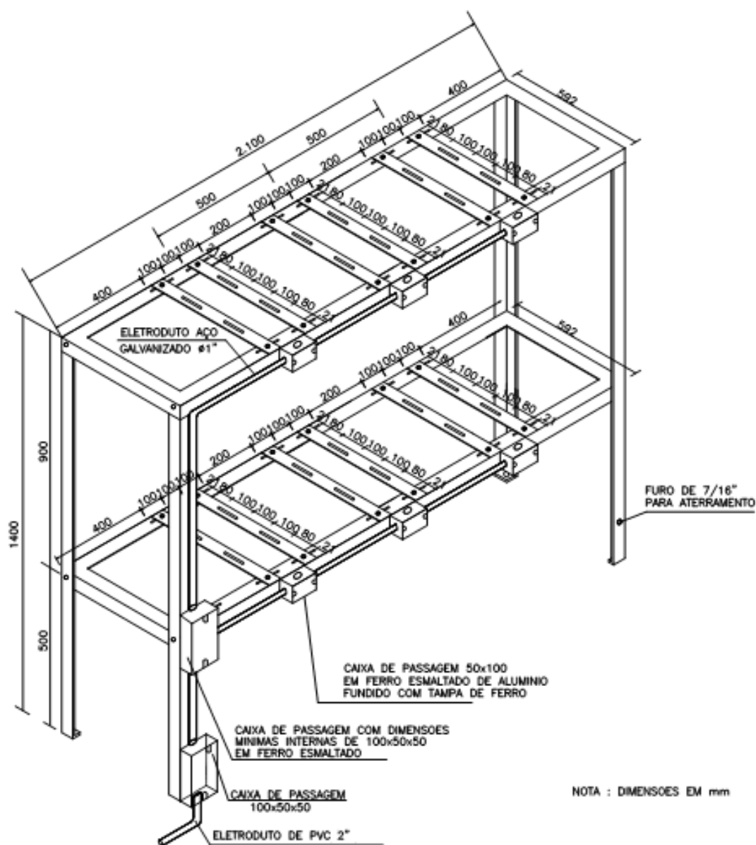
Figura 32 - Medição em Média Tensão – Suporte para TC e TP- Caveleto para Montagem de TC e TP em 36,2 kV (2/3)
