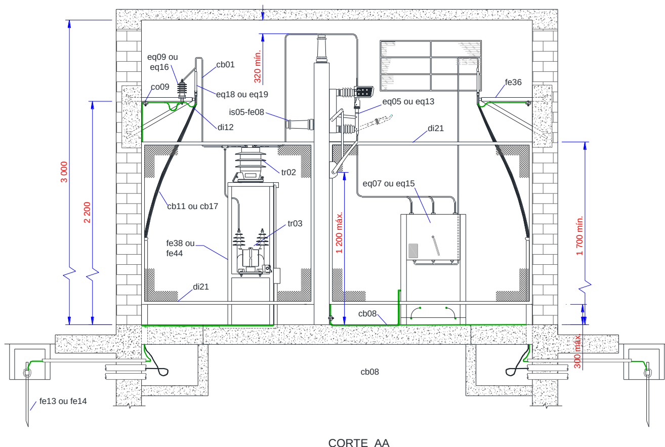
Figura 20 - Subestação Abrigada de Medição e Proteção Entrada Subterrânea – Medição AT (2/3)
