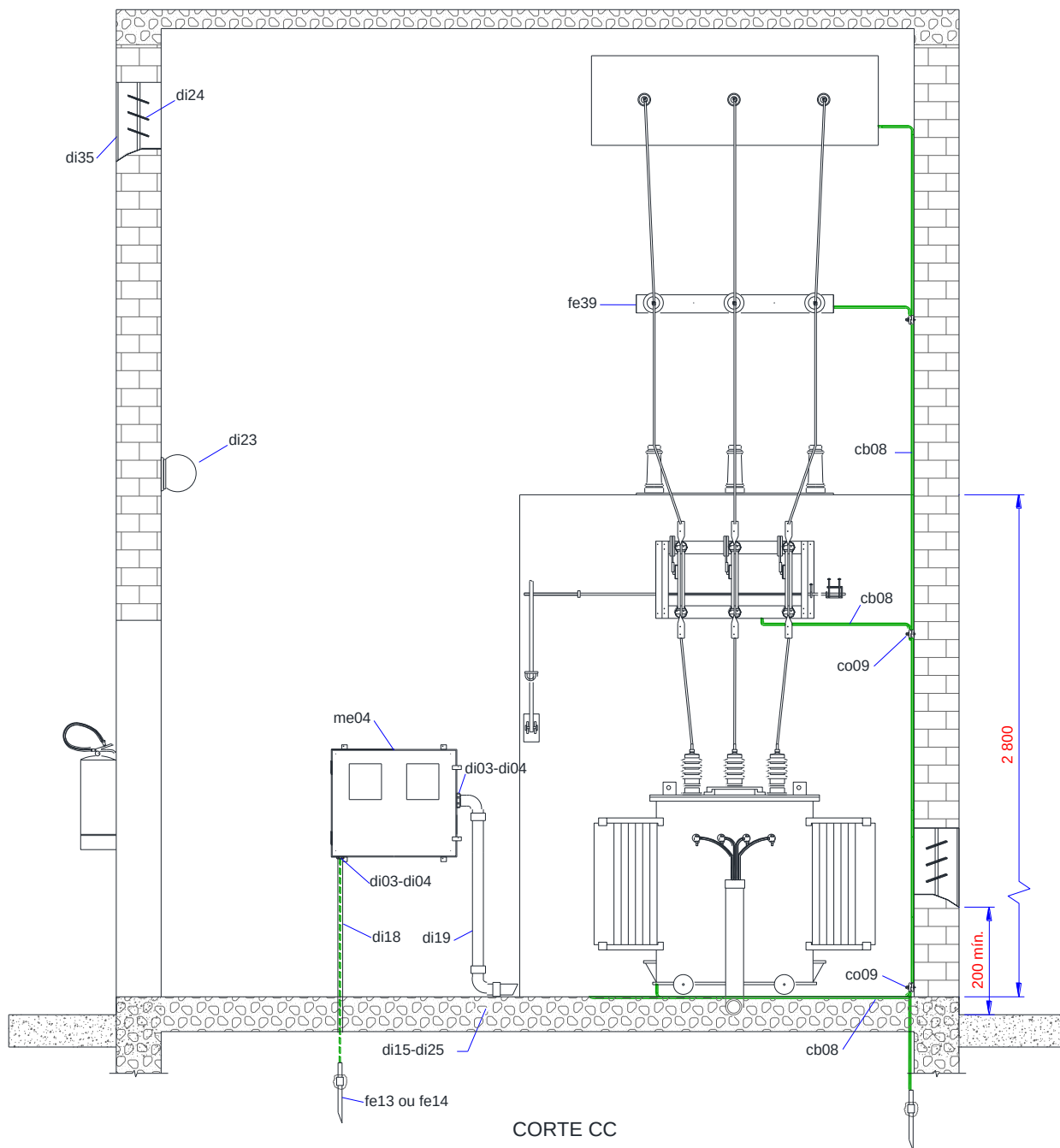
Figura 23 - Subestação Abrigada de Medição, Proteção e Transformação – Entrada Aérea – Medição em AT (4/4)
