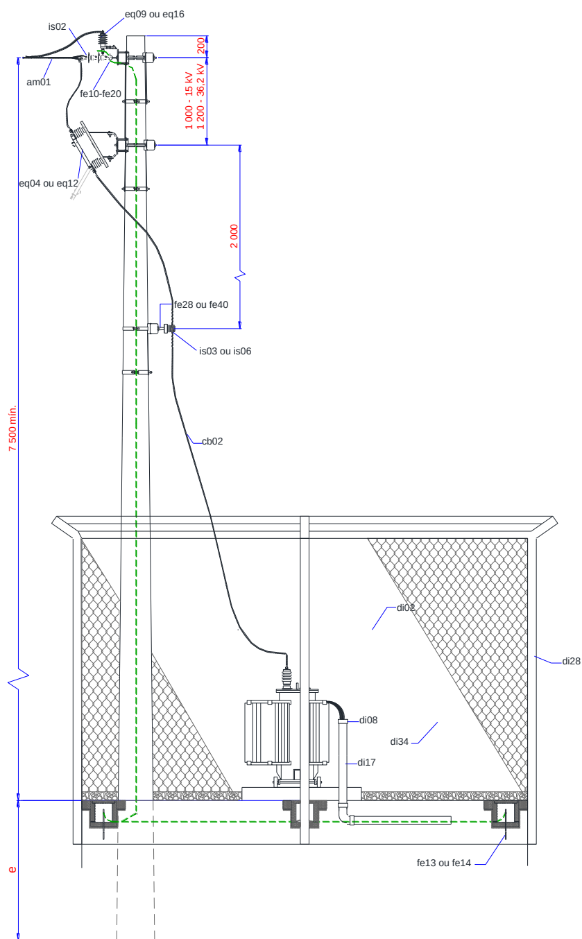
Figura 27 - Subestação ao Tempo Acima de 300 kVA - Entrada Aérea (3/3)
