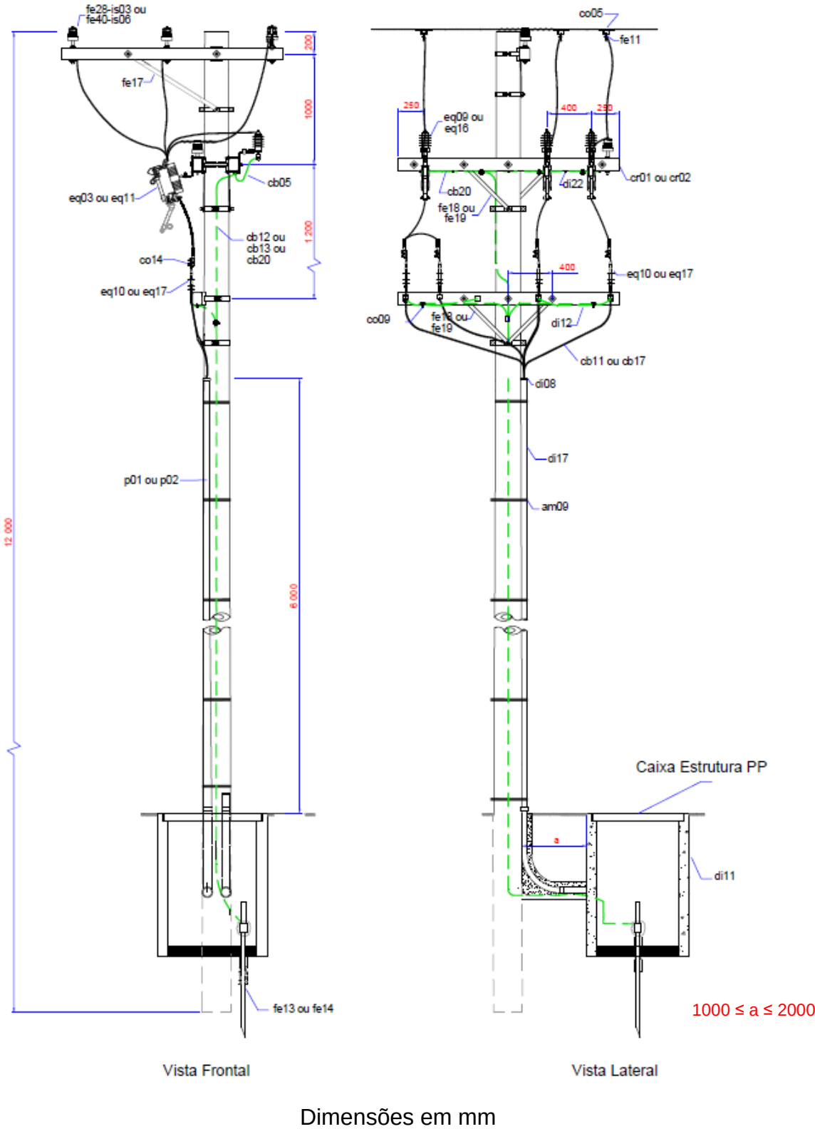
Figura 3 - Ramal de Entrada Subterrâneo – Derivação Rede Convencional
