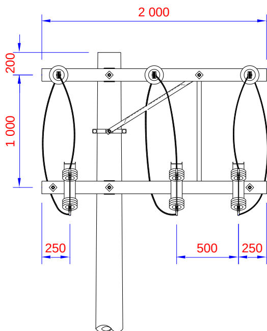
Figura 2 - Instalação de Seccionador Unipolar – Posição Horizontal (Poste Particular) (2/2) 13,8 kV
