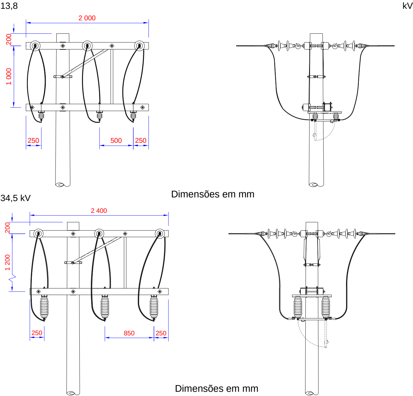
Figura 2 - Instalação de Seccionador Unipolar – Posição Horizontal (Poste Particular) (1/2)
