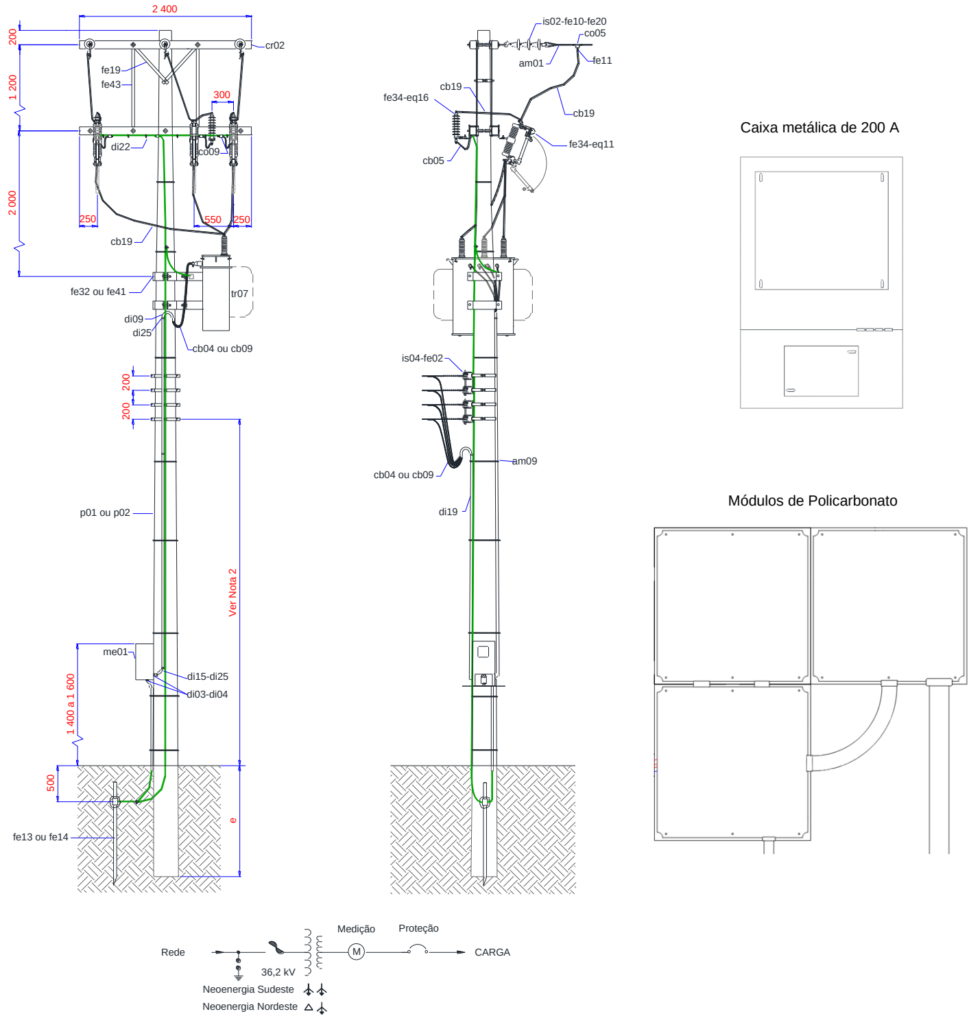
Figura 15 - Posto de Transformação em Poste - 36,2 kV (Medição Direta)
