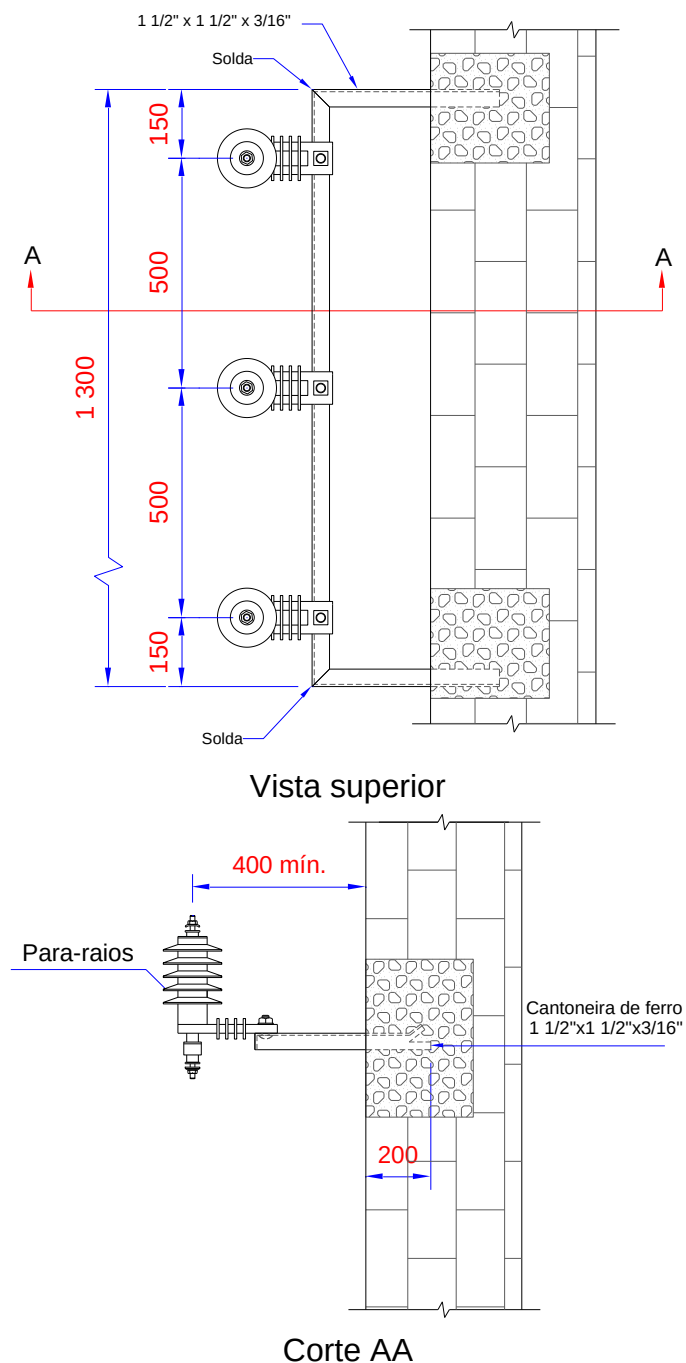
Figura 28 - Detalhes Construtivos em Subestações - Instalação de Para-raios (3/4)
