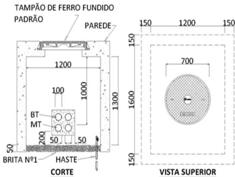
Figura 9 - Poço de Emenda para Ramal de Conexão Subterrâneo Poço Tipo – PE
