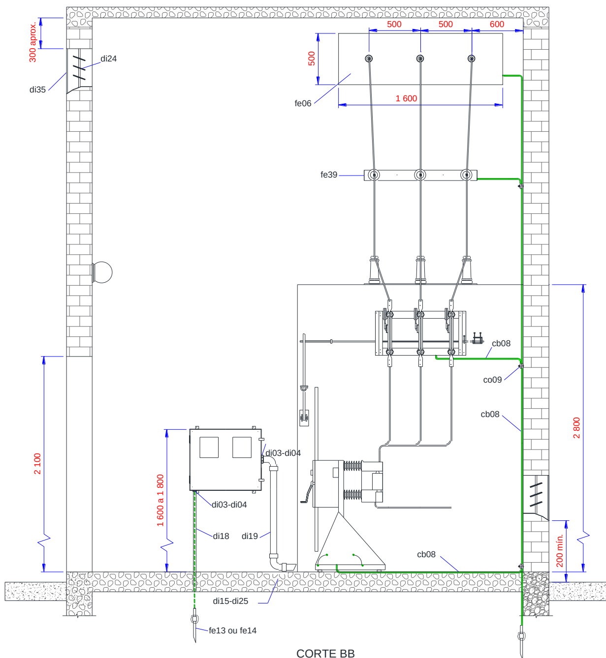
CORTE BB Dimensões em mm
