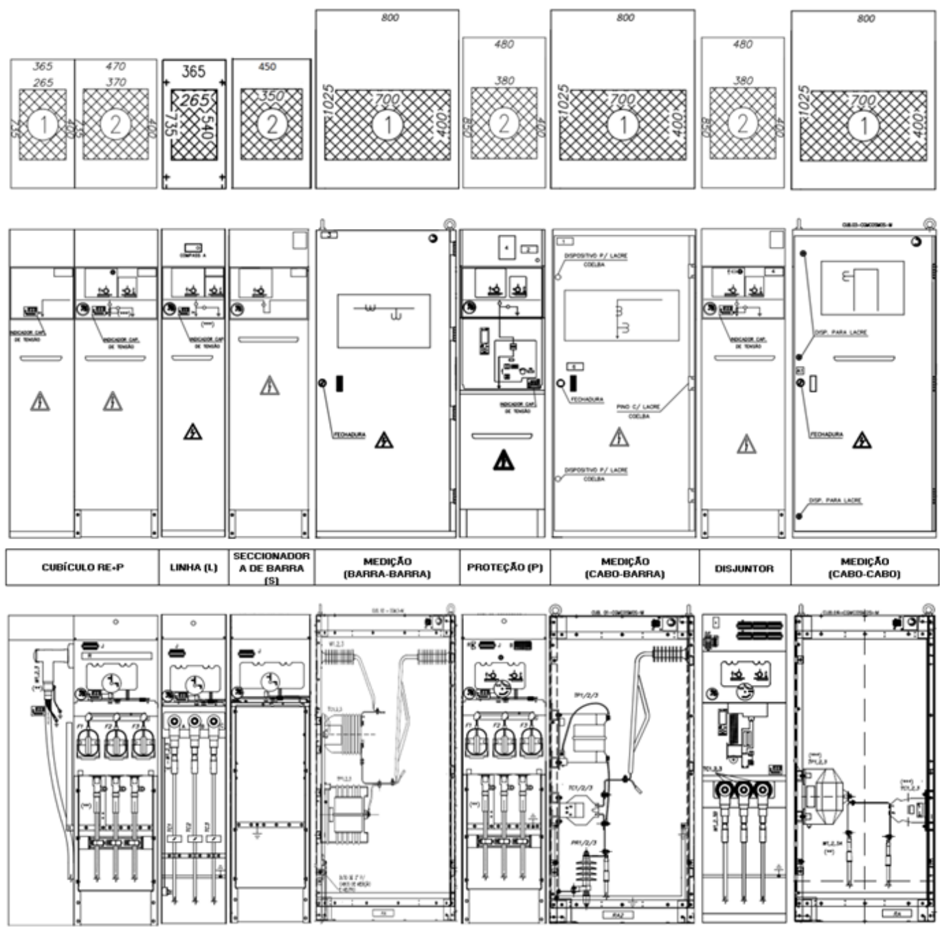
Figura 35 - Cubículos (Desenho Referência)
