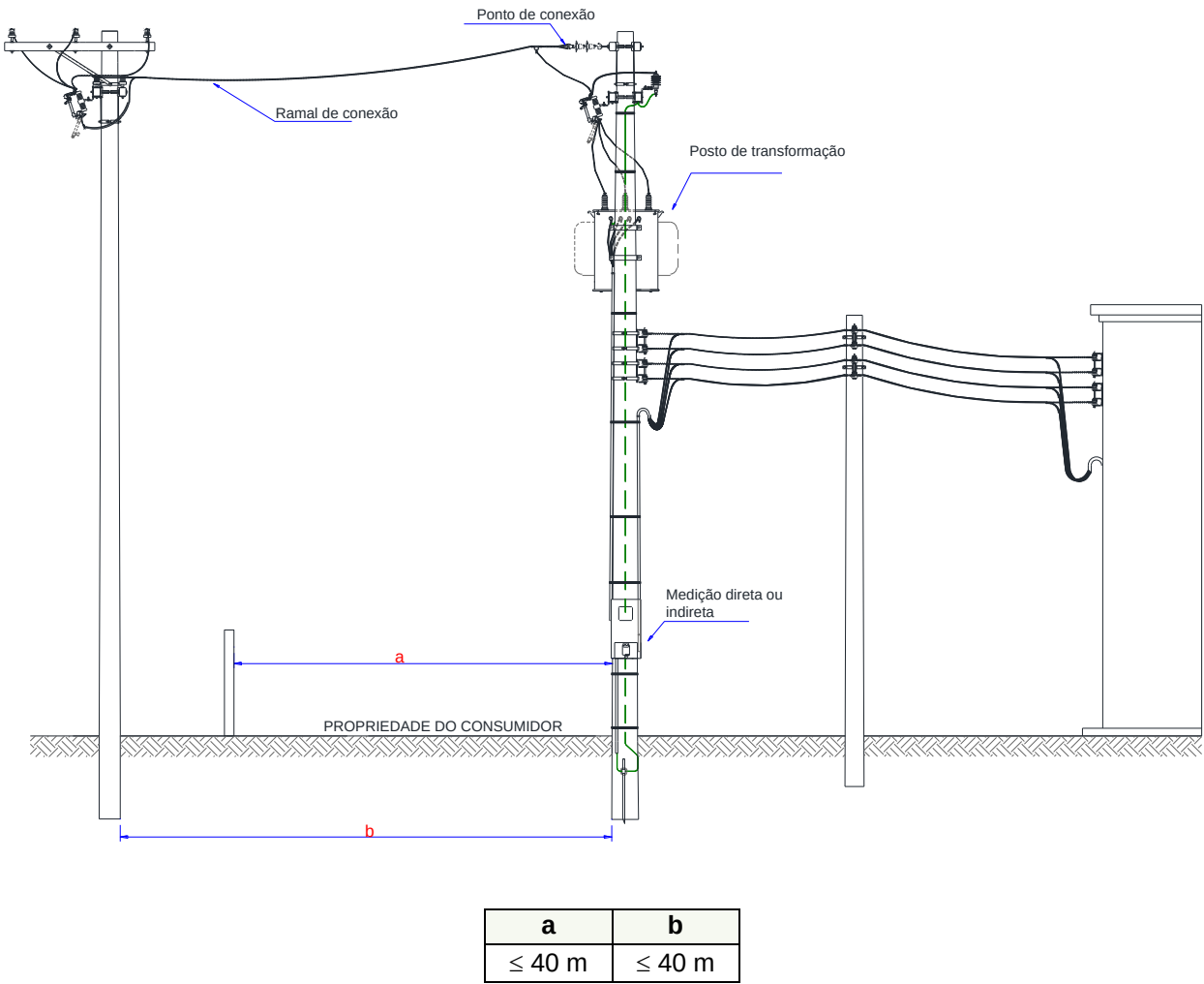
Figura 1 - Elementos da Entrada de Serviço (4/5)
