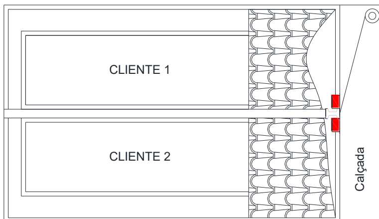
Figura 34 – Disposição da Entrada de Serviço – 2/4
