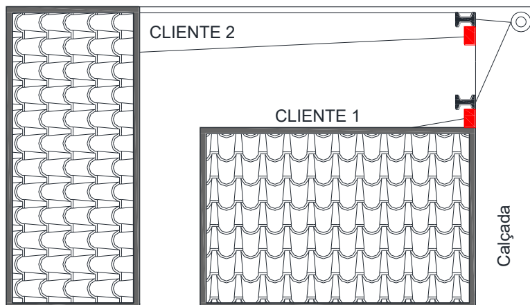
Figura 34 – Disposição da Entrada de Serviço – 4/4
