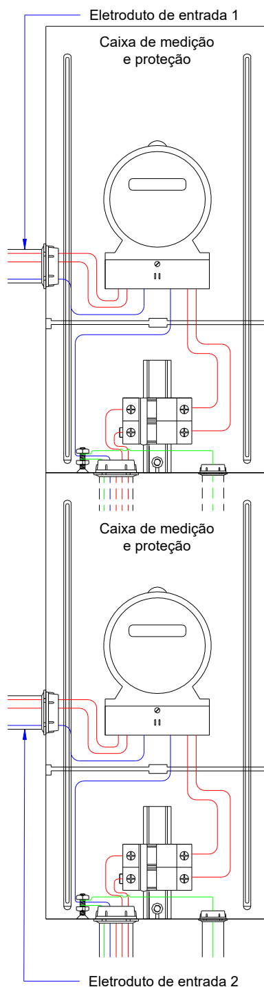
Figura 24 – Padrão de Entrada de Energia com Duas Medições Dispostas Verticalmente e Entradas Independentes
