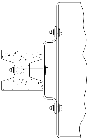
Corte B-B
