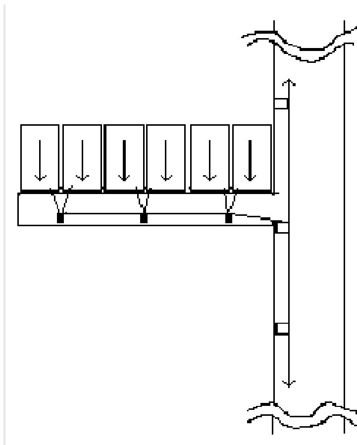
Figura 28 – Conexão de Unidades Consumidoras Situadas em Vielas
