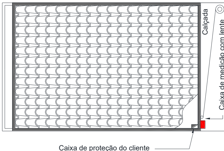
Figura 34 – Disposição da Entrada de Serviço – 3/4
