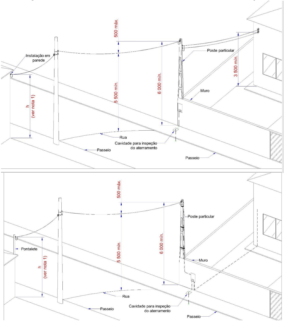
Figura 30 – Alturas Mínimas dos Condutores da Entrada de Serviço
