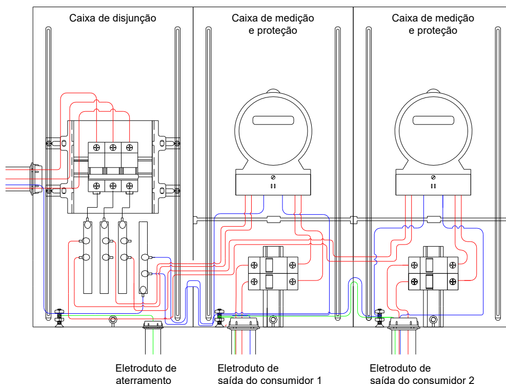
Figura 25 – Padrão de Entrada de Energia com Duas Medições e um Único Eletroduto de Entrada
