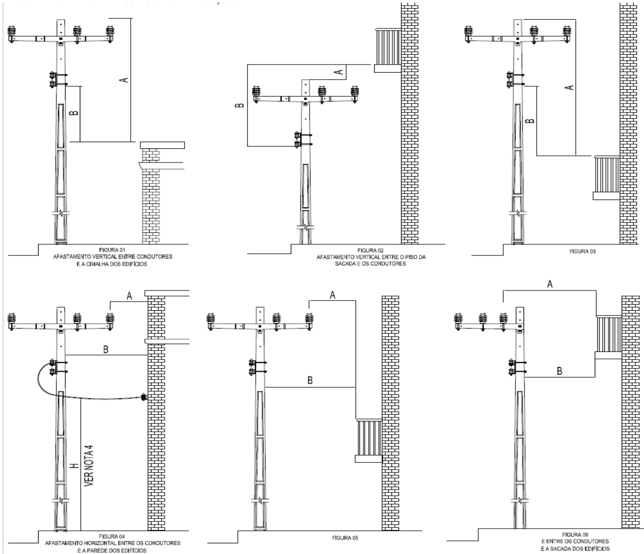
Figura 29 – Afastamentos Mínimos entre Condutores e Edificações
