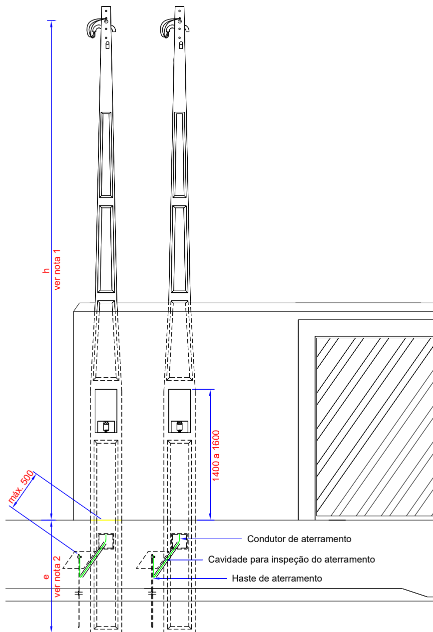
Figura 37 – Dimensões Gerais para Duas Ligações Instaladas em Muro
