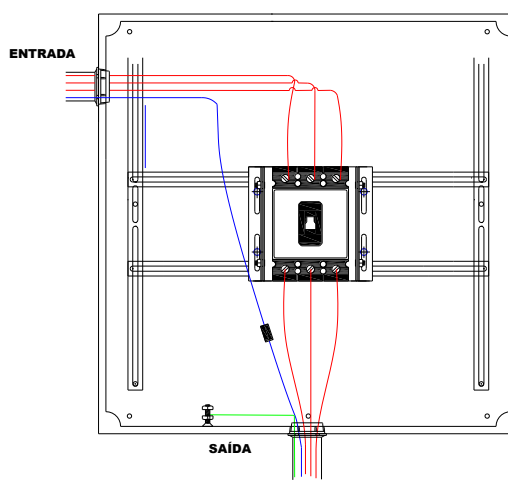
ILUSTRAÇÃO 8 PROTEÇÃO INDIRETA DESLOCADA
