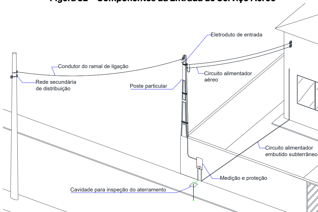
Figura 32 – Componentes da Entrada de Serviço Aéreo
