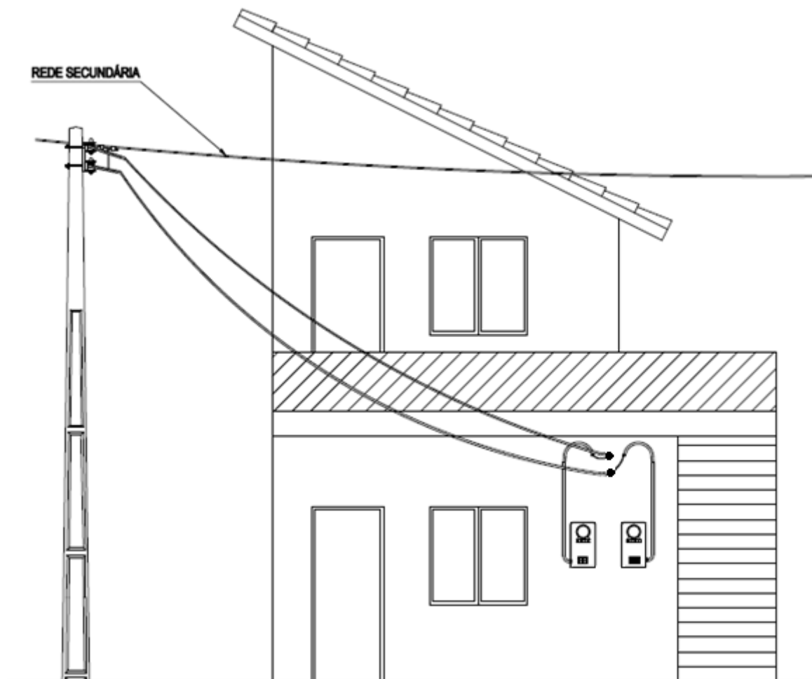
Figura 27 – Modelo de Ligação em Tensão Secundária de Duas Unidades Consumidoras Situadas em um Mesmo Terreno Sem Área de Uso Comum
