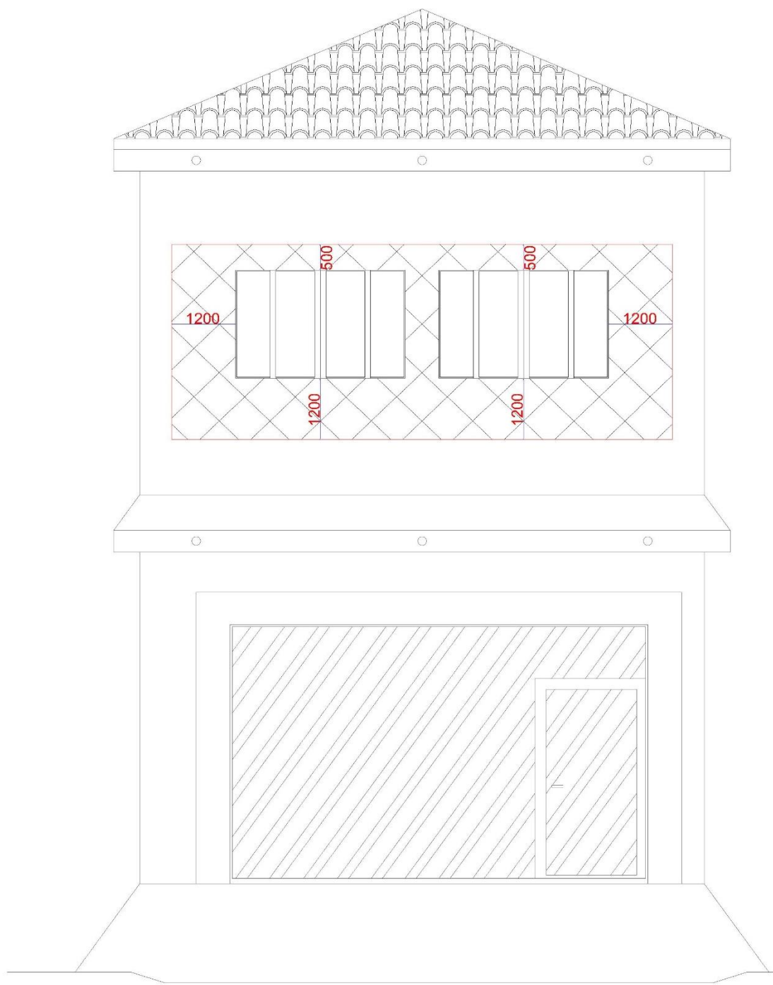
Figura 31 – Afastamentos Mínimos para Entrada de Serviço em Fachada
