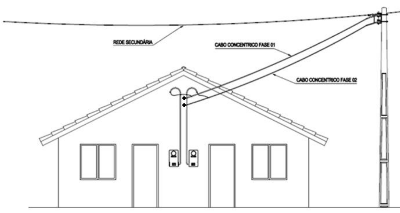
Figura 26 – Modelo de Ligação em Tensão Secundária de Casas Geminadas
