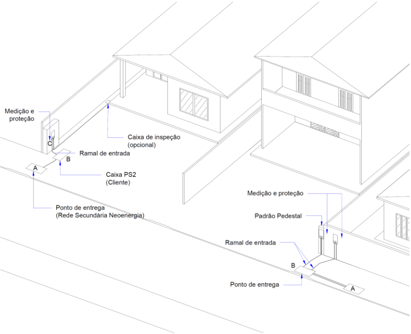
Padrão Subterrâneo derivado de Rede Subterrânea
