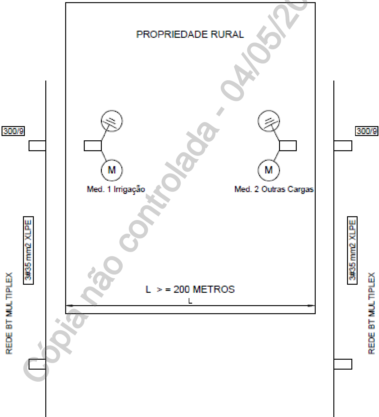
Figura 20 - Situação do Ponto de Conexão –Distinto para o Consumidor Irrigante em Baixa Tensão
