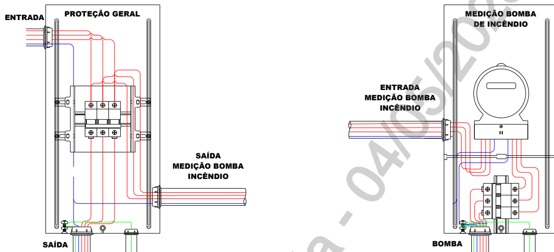
ILUSTRAÇÃO 9 PROTEÇÃO GERAL DESLOCADA COM BOMBA DE INCÊNDIO
