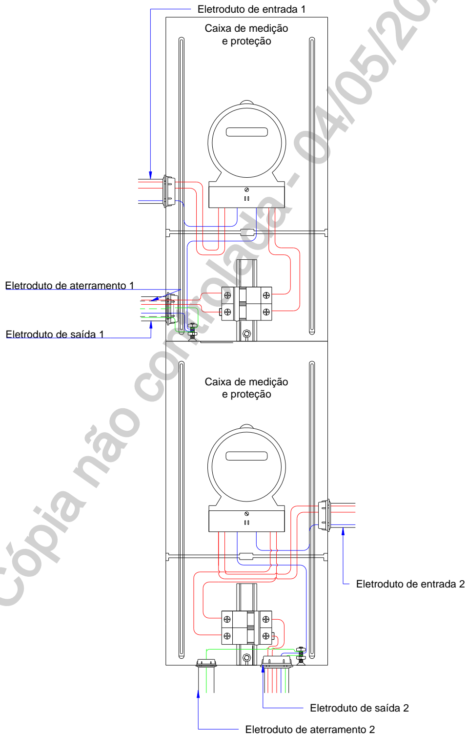
Figura 22 - Padrão de Entrada de Energia com Duas Medições Dispostas Verticalmente e Entradas Independentes
