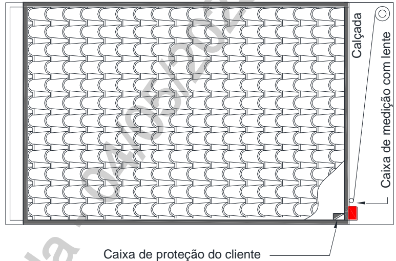
Figura 29 – Disposição da Entrada de Serviço
