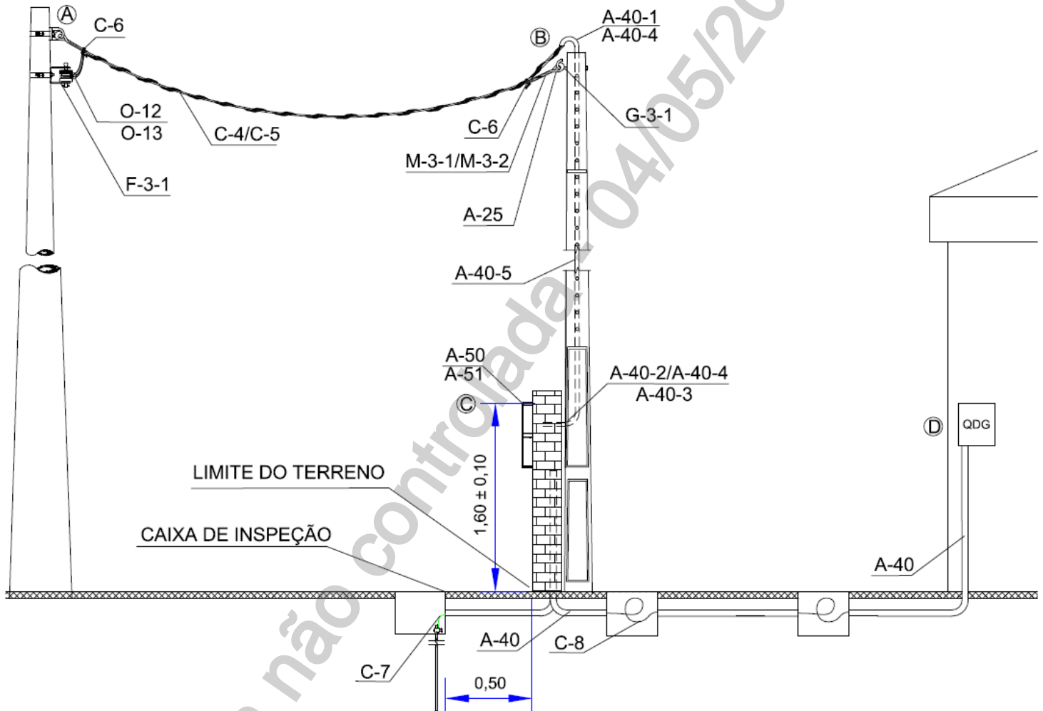
Figura 2 - Entrada de Serviço Aérea com Travessia de Rua - Medição no Muro - Ramal de Distribuição Subterrâneo (Desenho Ilustrativo)
