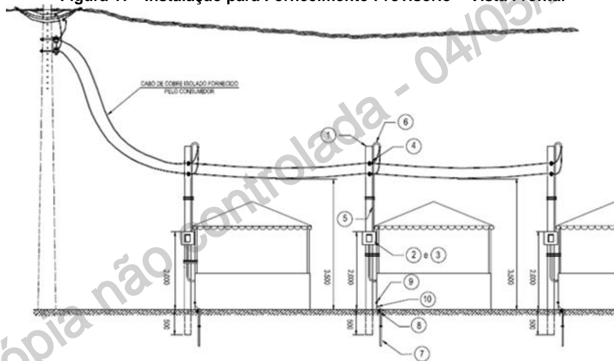
Figura 17 - Instalação para Fornecimento Provisório – Vista Frontal
