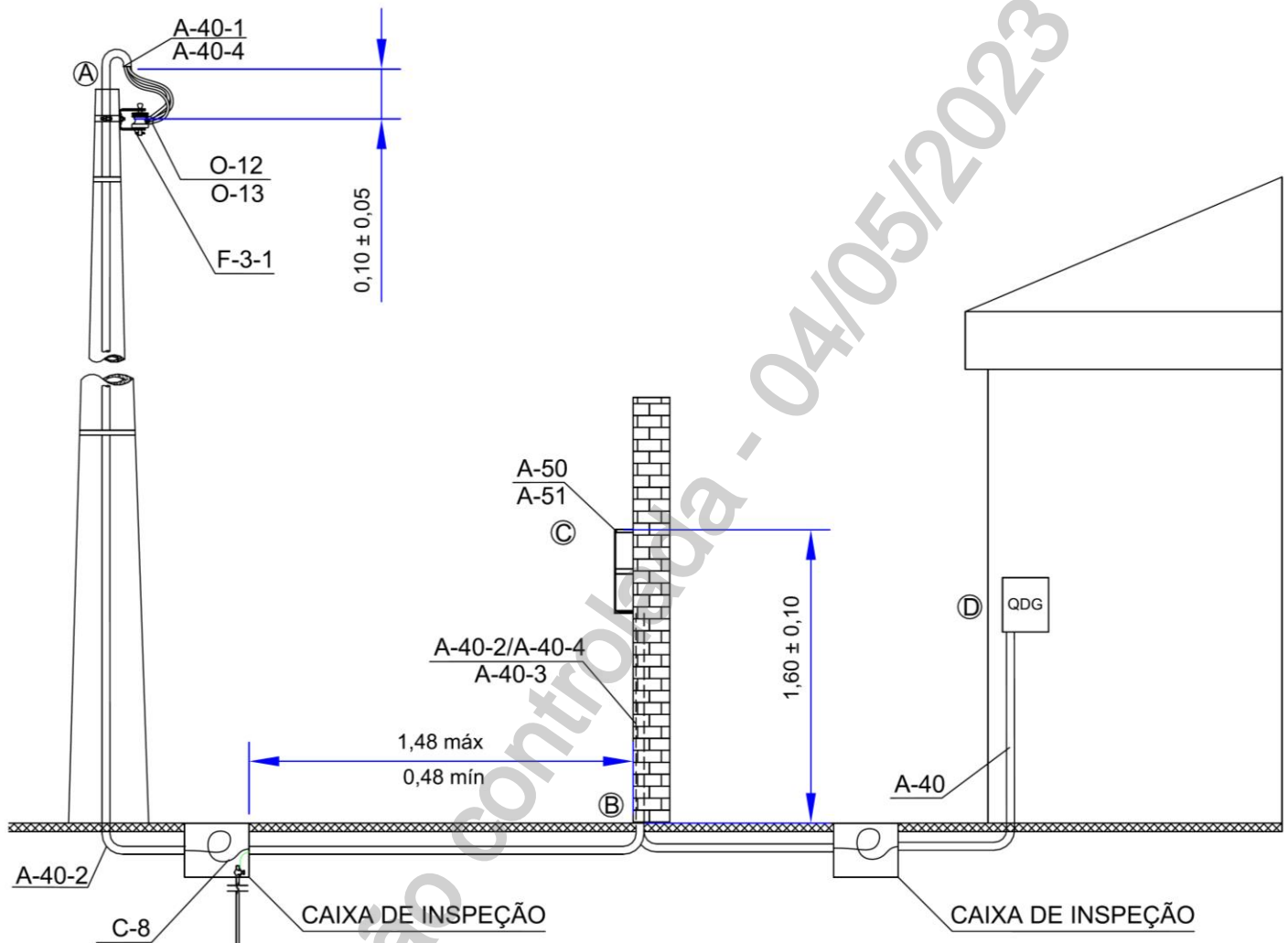
Figura 8 - Entrada de Serviço Subterrânea Derivada de Rede Aérea
