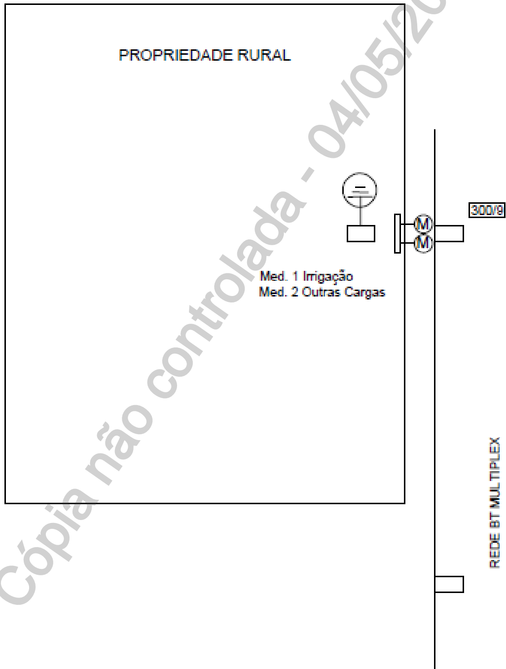
Figura 19 - Situação do Ponto de Conexão - Único para o Consumidor Irrigante em Baixa Tensão
