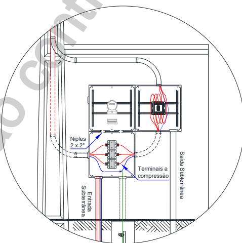
ILUSTRAÇÃO 53 INDIRETA EM MURETA
