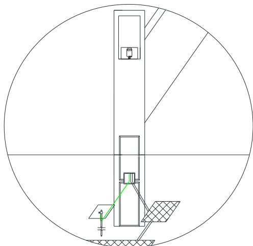
ILUSTRAÇÃO 31 FRONTAL PEDESTAL SUBTERRÂNEA
