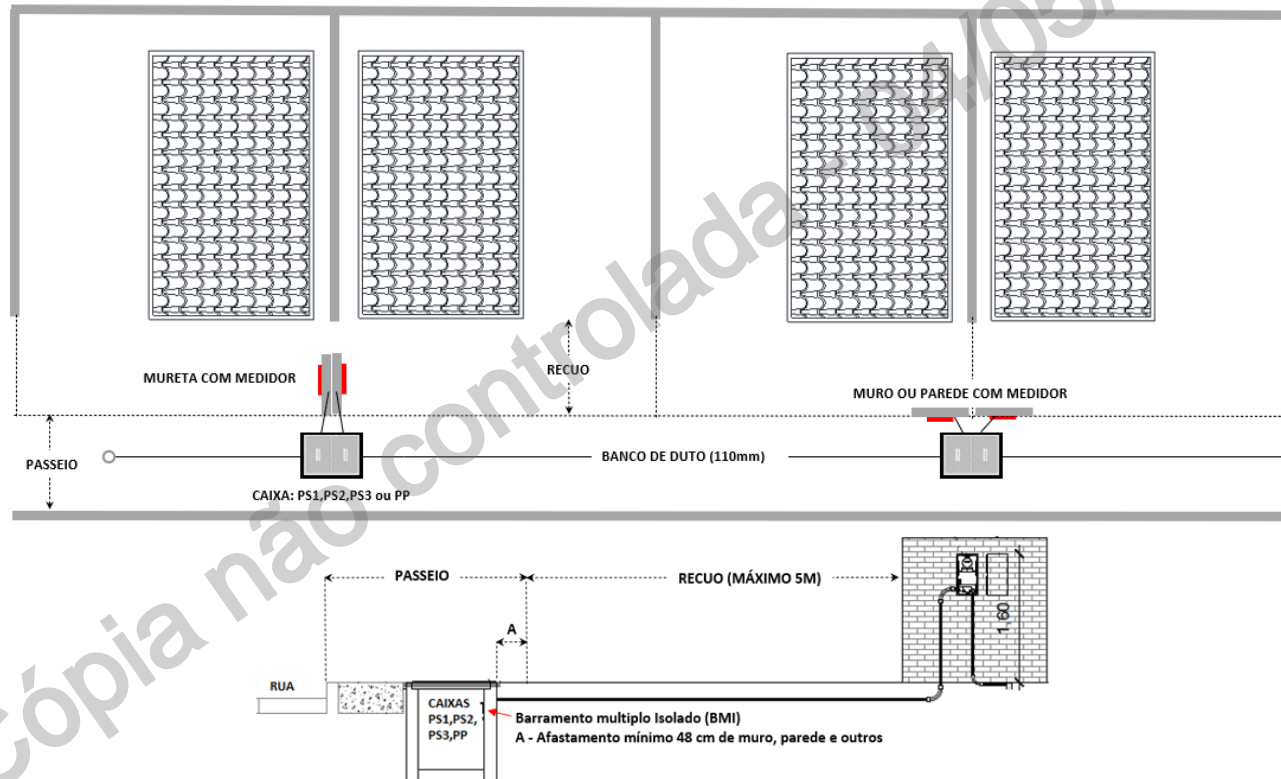
Figura 33 – Disposição da Entrada de Serviço em Área Urbana - Padrão Subterrâneo
