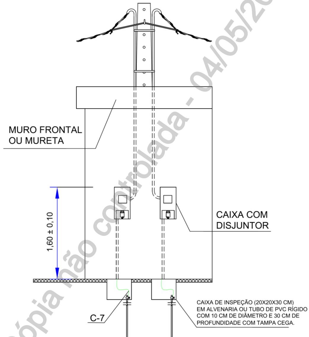
Figura 21 - Padrão de Entrada de Energia com Duas Medições Dispostas Horizontalmente e Eletrodutos de Entrada Independentes
