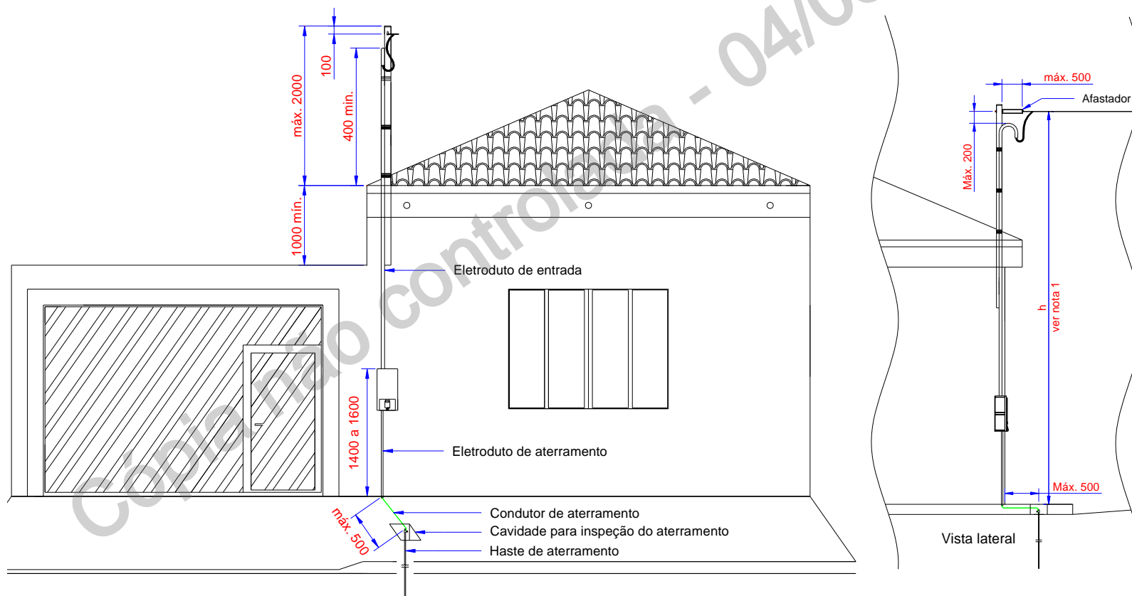
Figura 37 – Dimensões Gerais para instalação em Pontaete
