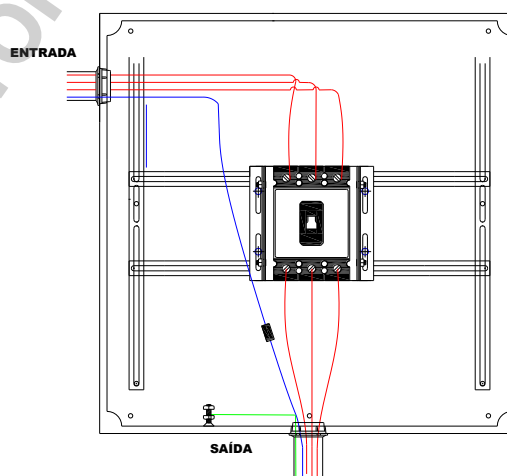
ILUSTRAÇÃO 8 PROTEÇÃO INDIRETA DESLOCADA
