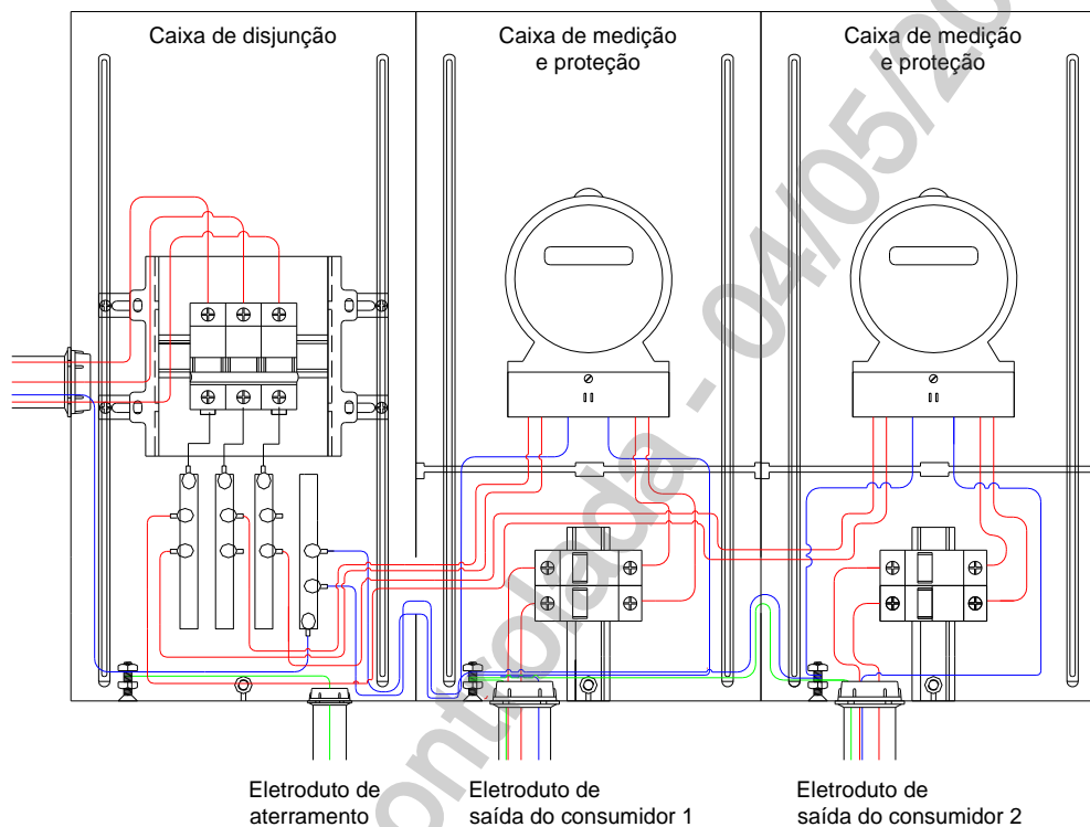
Figura 23 - Padrão de Entrada de Energia com Duas Medições e um Único Eletroduto de Entrada
