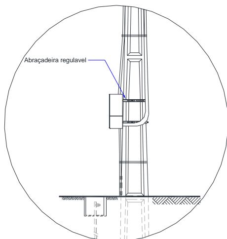
ILUSTRAÇÃO 14 INSTALAÇÃO AO TEMPO
