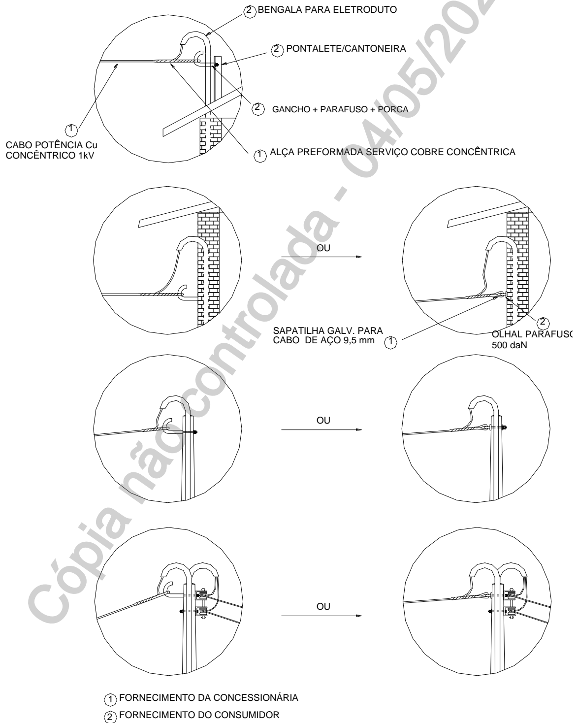
Figura 12 - Detalhes de Pontos de Conexão Monofásico
