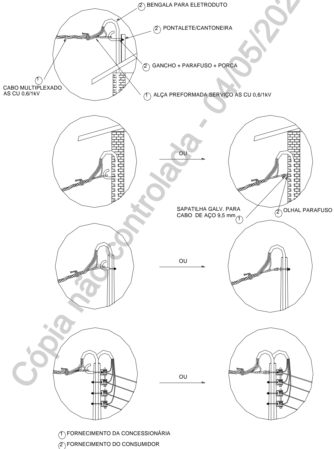
Figura 13 - Detalhes de Pontos de Conexão Bifásico e Trifásico
