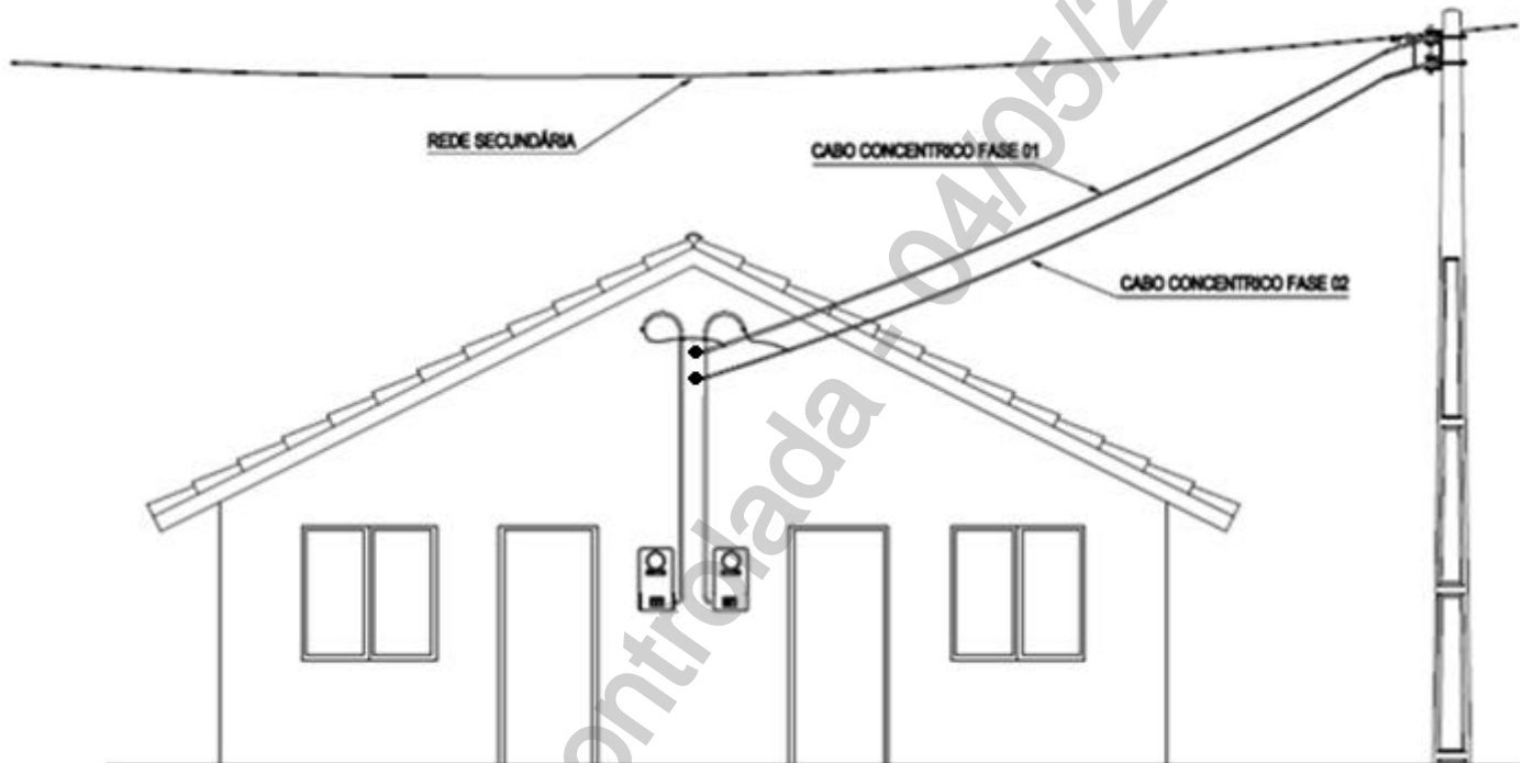
Figura 24 - Modelo de Ligação em Tensão Secundária de Casas Geminadas
