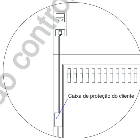
ILUSTRAÇÃO 20 FRONTAL CAIXA COM LENTE
