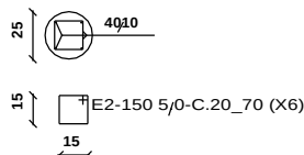
ARMADURA DAS BROCAS
