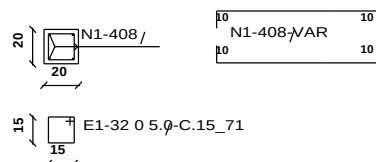
ARMADURA DAS BROCAS
