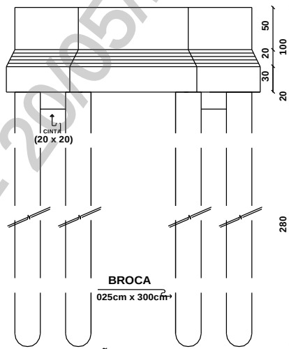
ELEVÇÃO FRONTAL
