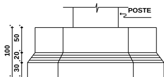
ELEVÇÃO FRONTAL
