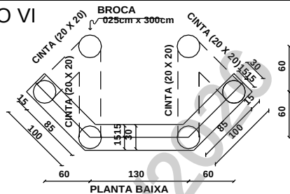
PLANTA BAIXA
