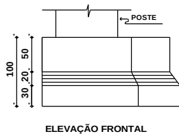
ELEVAÇÃO FRONTAL
