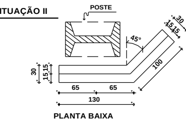
PLANTA BAIXA
