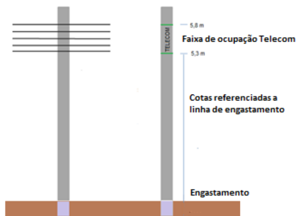
Figura 3 – Identificação das Faixas Destinadas às Operadoras de Telecomunicação
