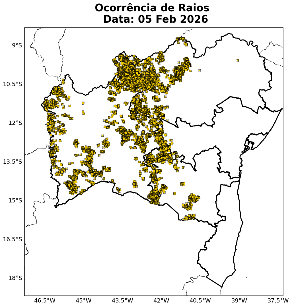
Figura 15: Ocorrências de descargas atmosféricas nuvem-solo detectadas pelo sistema Earth Networks para o dia 05 de Fevereiro sobre a área de concessão da COELBA.
