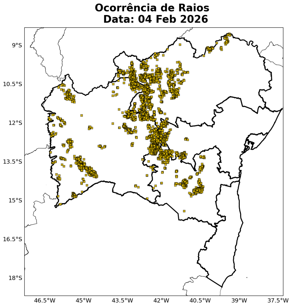
Figura 14: Ocorrências de descargas atmosféricas nuvem-solo detectadas pelo sistema Earth Networks para o dia 04 de Fevereiro sobre a área de concessão da COELBA.
