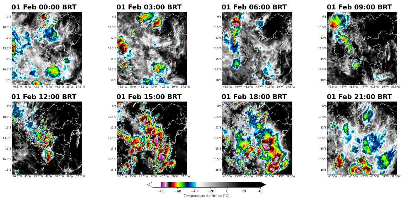
Figura 2: Imagens realçadas do satélite GOES-19 das 00 BRT até 21 BRT (a cada 3 horas) para o dia 01 de Fevereiro.
