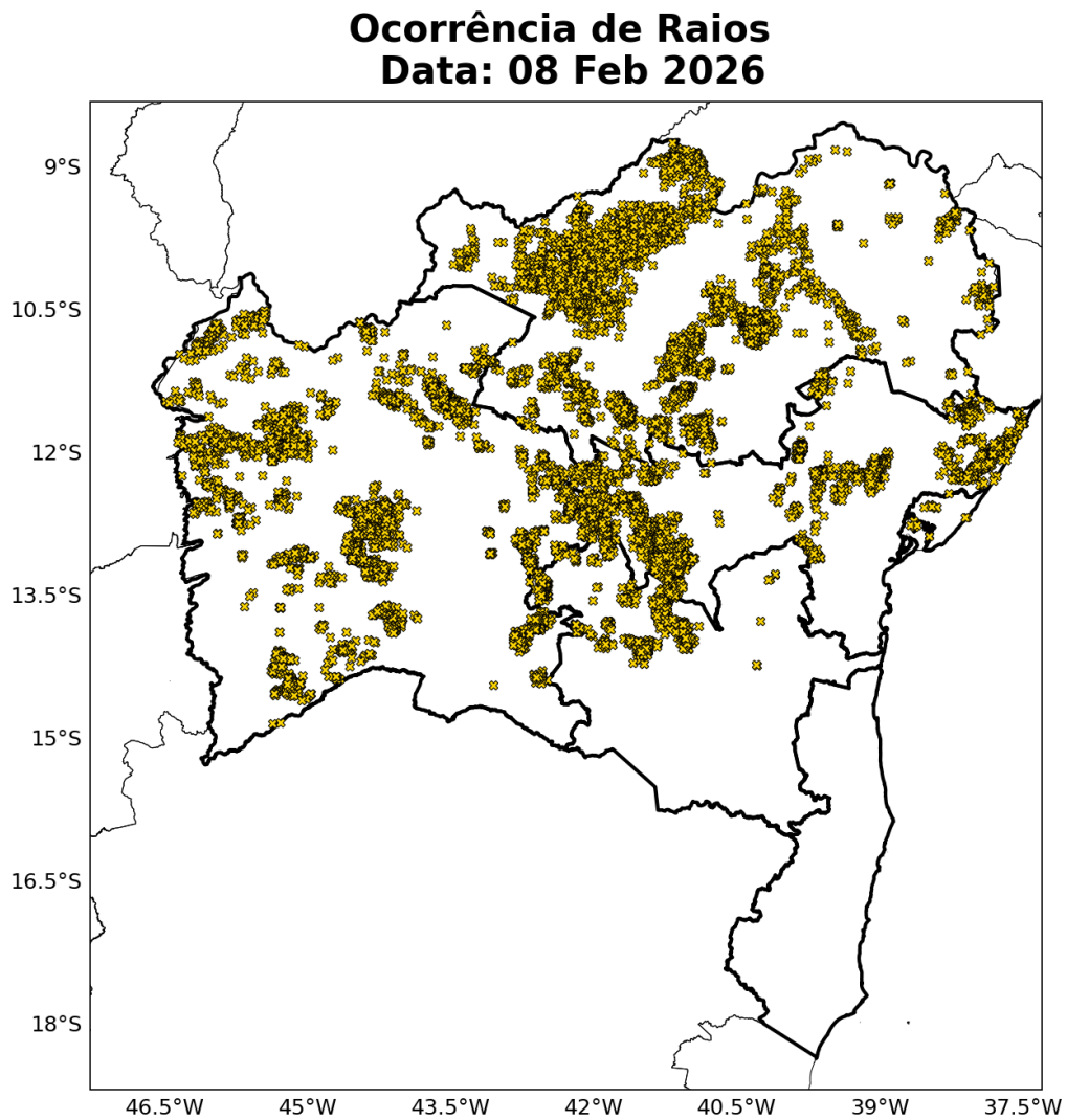
Figura 18: Ocorrências de descargas atmosféricas nuvem-solo detectadas pelo sistema Earth Networks para o dia 08 de Fevereiro sobre a área de concessão da COELBA.
