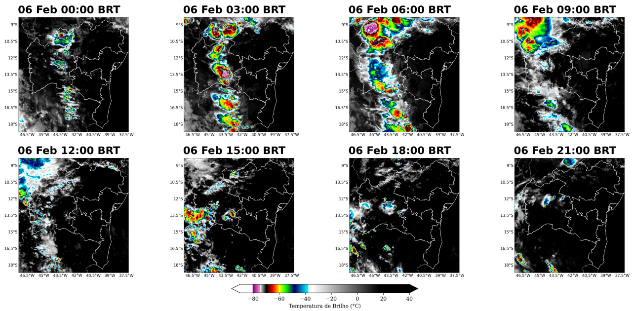
Figura 7: Imagens realçadas do satélite GOES-19 das 00 BRT até 21 BRT (a cada 3 horas) para o dia 06 de Fevereiro.
