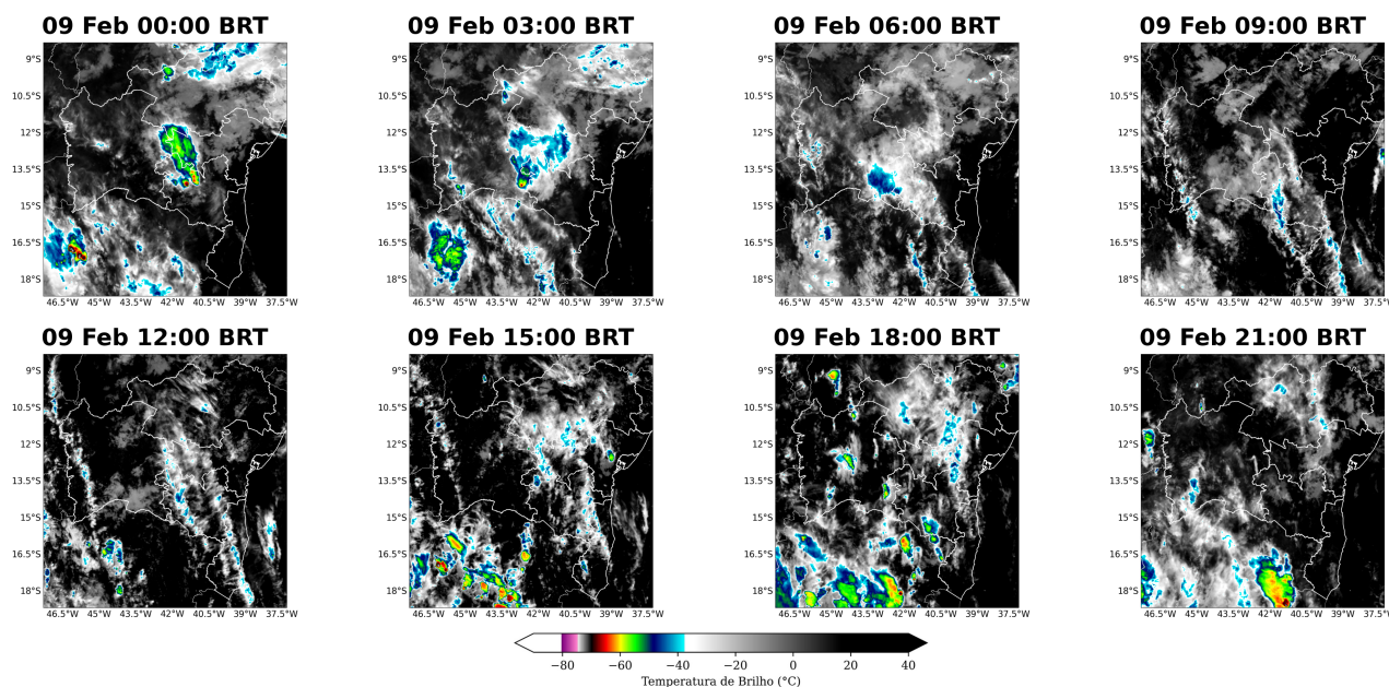
Figura 10: Imagens realçadas do satélite GOES-19 das 00 BRT até 21 BRT (a cada 3 horas) para o dia 09 de Fevereiro.
