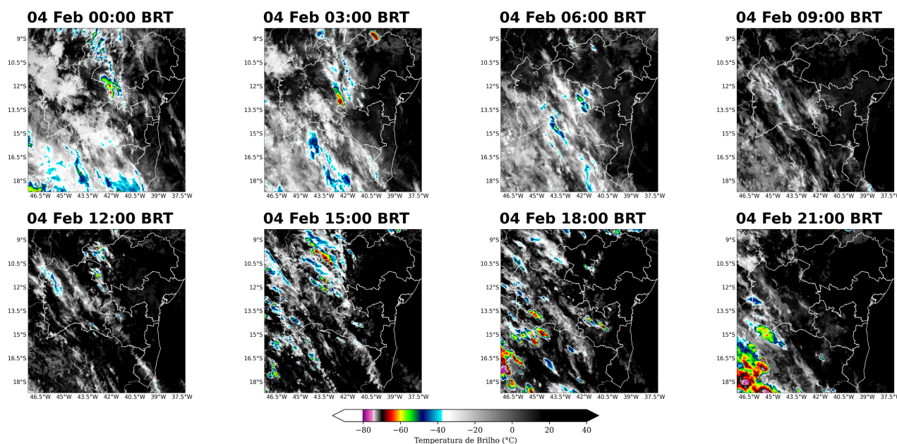
Figura 5: Imagens realçadas do satélite GOES-19 das 00 BRT até 21 BRT (a cada 3 horas) para o dia 04 de Fevereiro.
