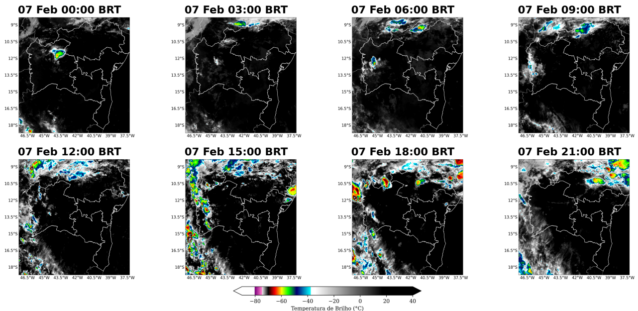
Figura 8: Imagens realçadas do satélite GOES-19 das 00 BRT até 21 BRT (a cada 3 horas) para o dia 07 de Fevereiro.
