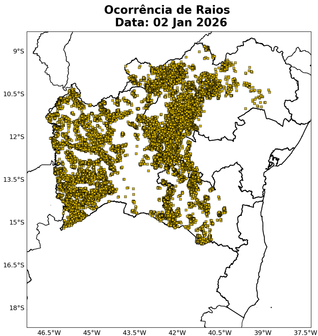
Figura 12: Ocorrências de descargas atmosféricas nuvem-solo detectadas pelo sistema Earth Networks para o dia 02 de Janeiro sobre a área de concessão da COELBA.
