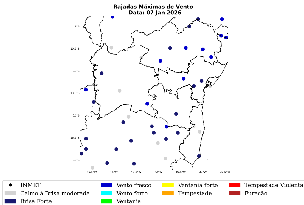
Figura 37: Máxima rajada de vento diária sobre a área de concessão da COELBA para o dia 07 de Janeiro, baseado nas estações meteorológicas do INMET.
