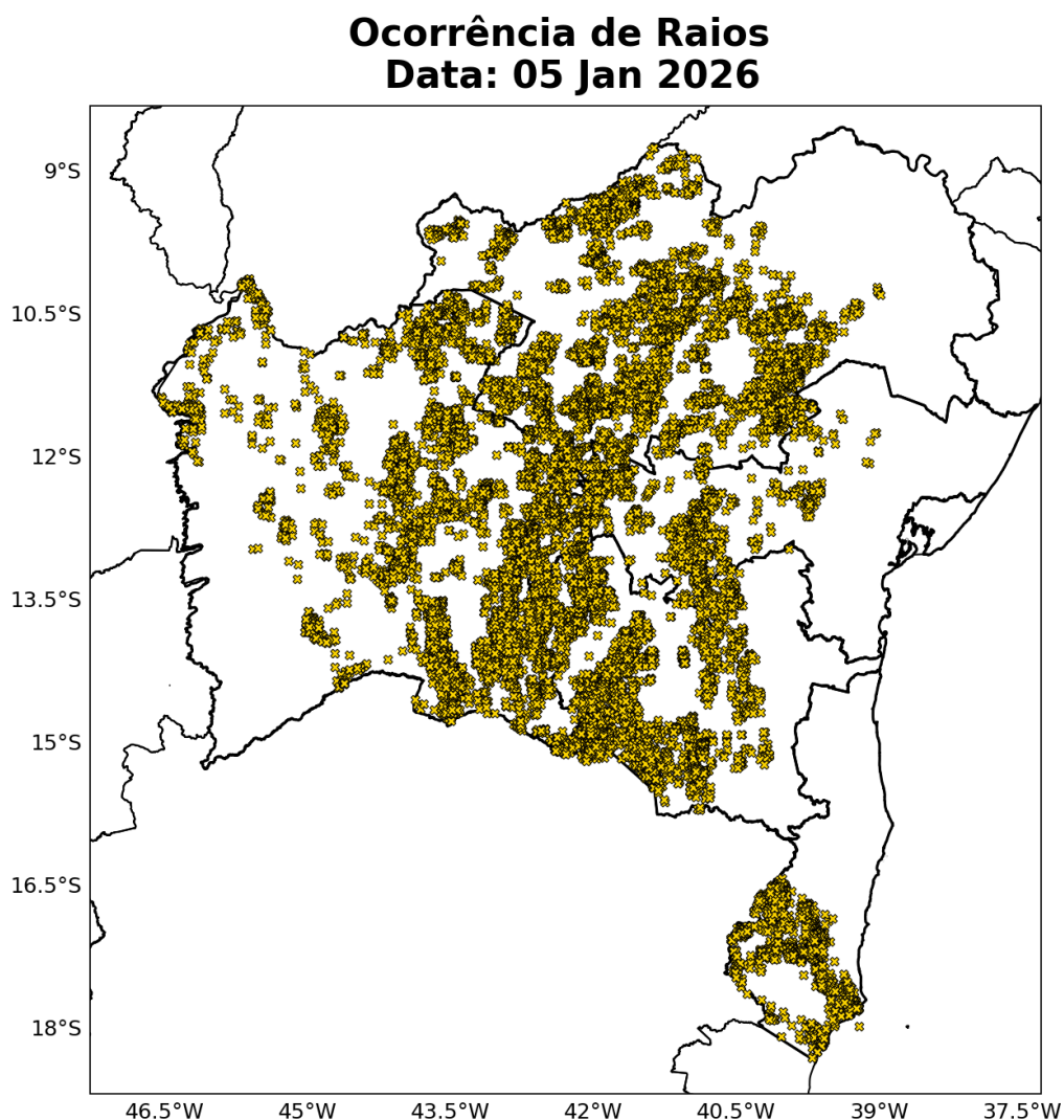
Figura 15: Ocorrências de descargas atmosféricas nuvem-solo detectadas pelo sistema Earth Networks para o dia 05 de Janeiro sobre a área de concessão da COELBA.
