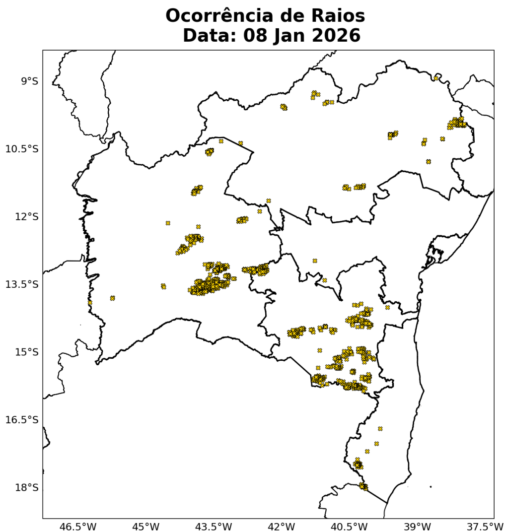
Figura 18: Ocorrências de descargas atmosféricas nuvem-solo detectadas pelo sistema Earth Networks para o dia 08 de Janeiro sobre a área de concessão da COELBA.
