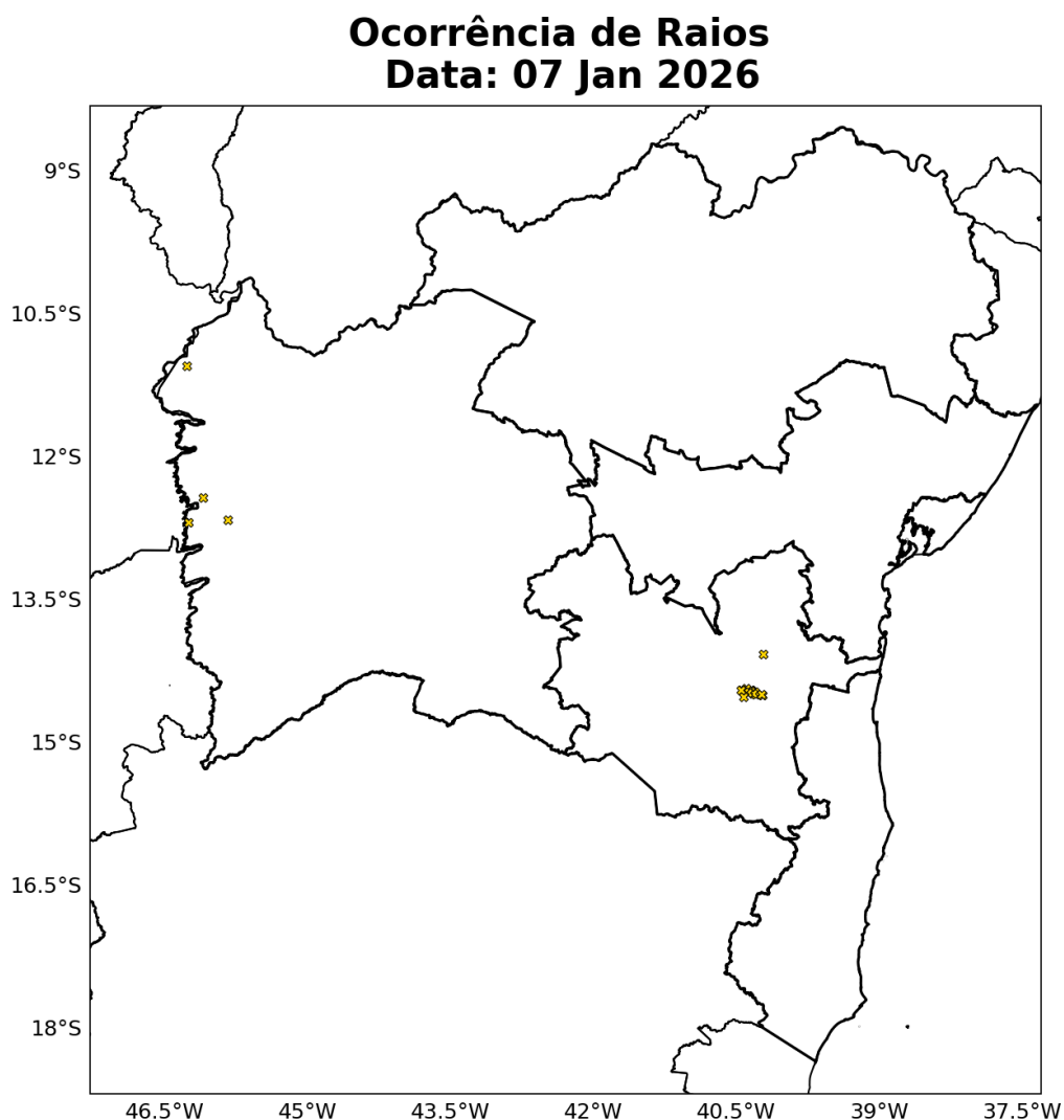
Figura 17: Ocorrências de descargas atmosféricas nuvem-solo detectadas pelo sistema Earth Networks para o dia 07 de Janeiro sobre a área de concessão da COELBA.
