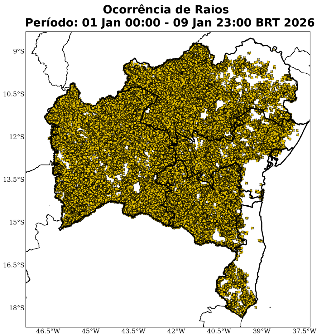
Figura 20: Ocorrências de descargas atmosféricas nuvem-solo detectadas pelo sistema Earth Networks para o período de 01 a 09 de Janeiro de 2026 sobre a área de concessão da COELBA.
