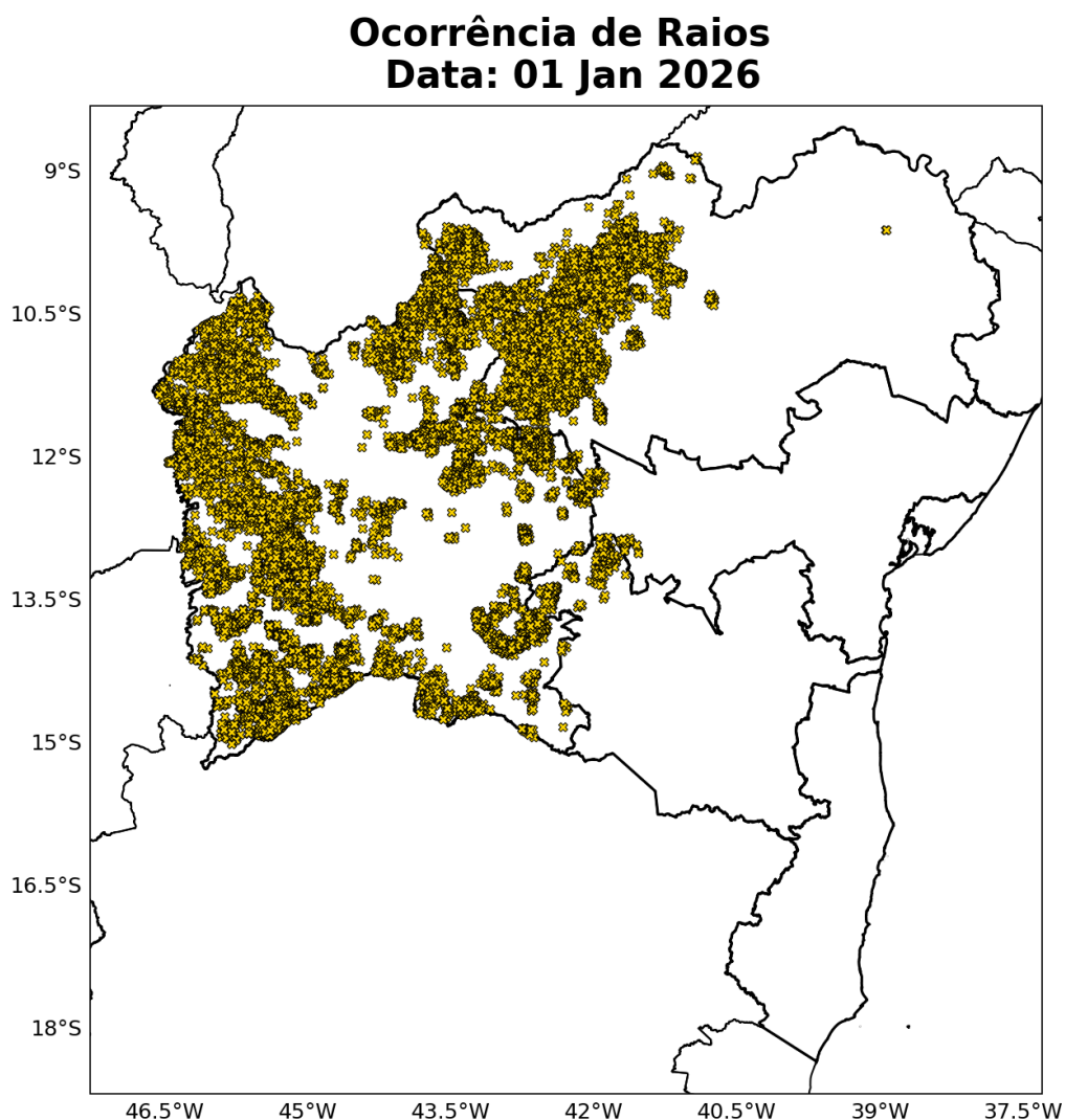
Figura 11: Ocorrências de descargas atmosféricas nuvem-solo detectadas pelo sistema Earth Networks para o dia 01 de Janeiro sobre a área de concessão da COELBA.
