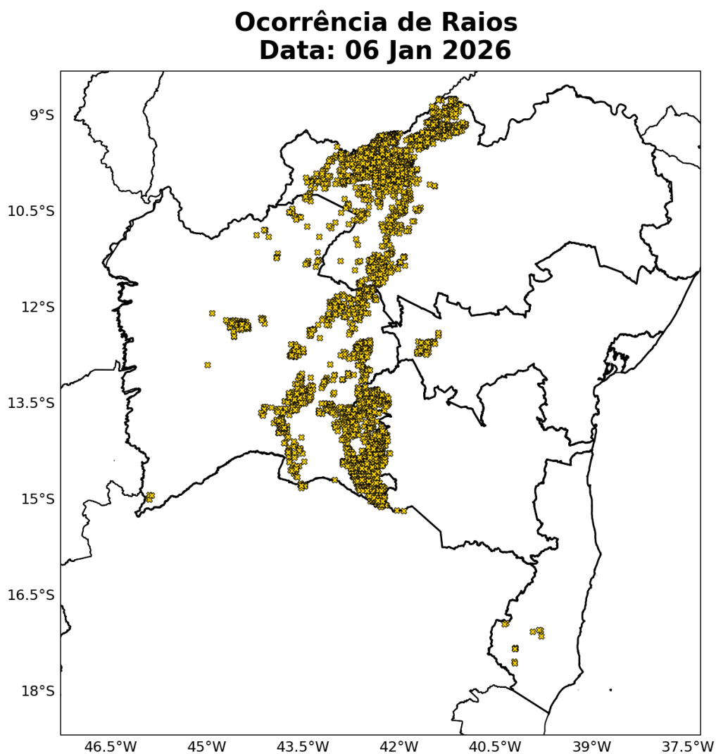
Figura 16: Ocorrências de descargas atmosféricas nuvem-solo detectadas pelo sistema Earth Networks para o dia 06 de Janeiro sobre a área de concessão da COELBA.
