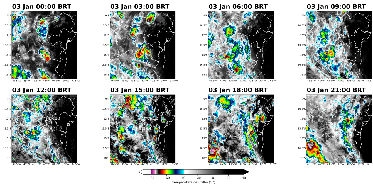
Figura 4: Imagens realçadas do satélite GOES-19 das 00 BRT até 21 BRT (a cada 3 horas) para o dia 03 de Janeiro.
