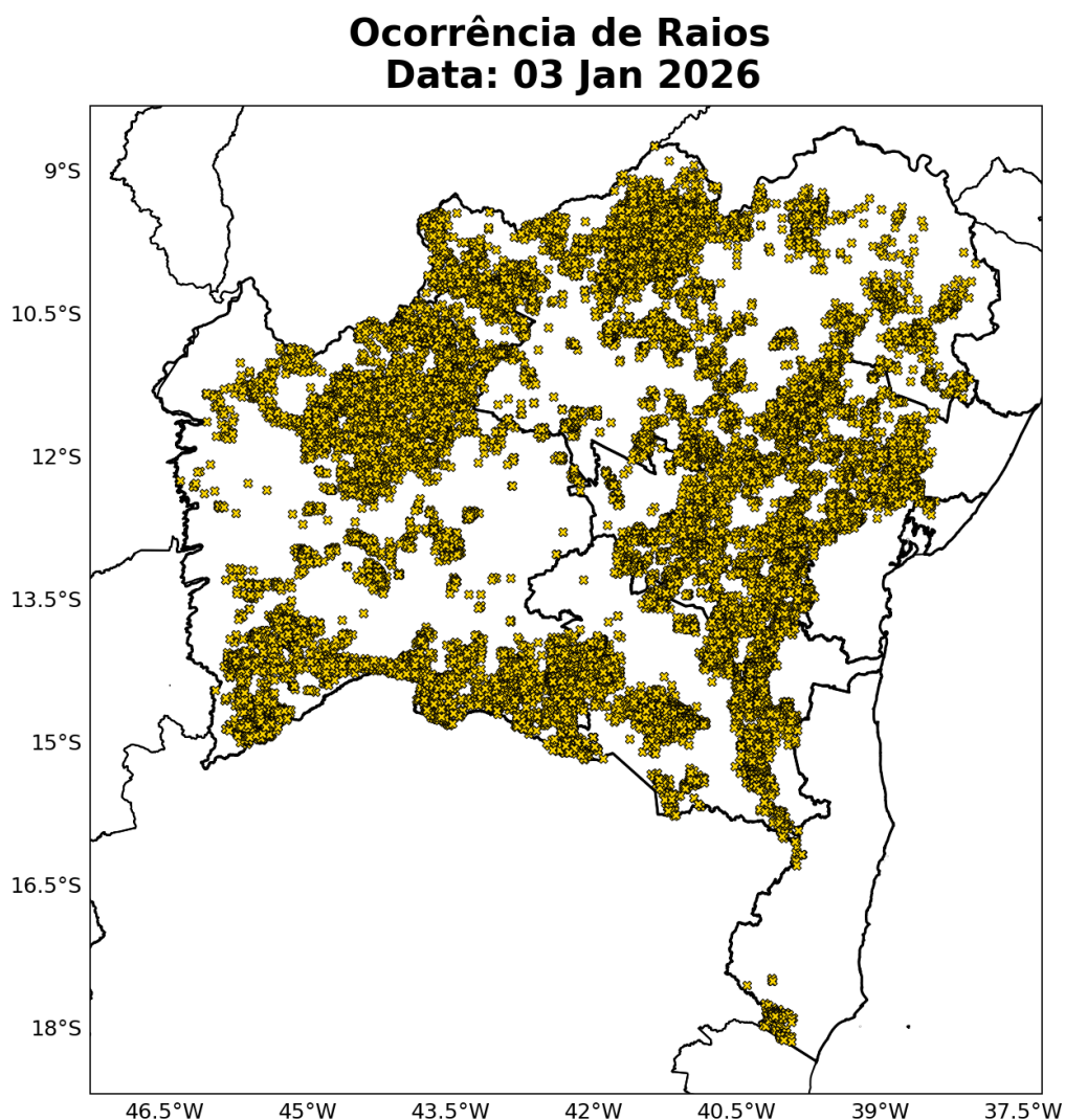
Figura 13: Ocorrências de descargas atmosféricas nuvem-solo detectadas pelo sistema Earth Networks para o dia 03 de Janeiro sobre a área de concessão da COELBA.
