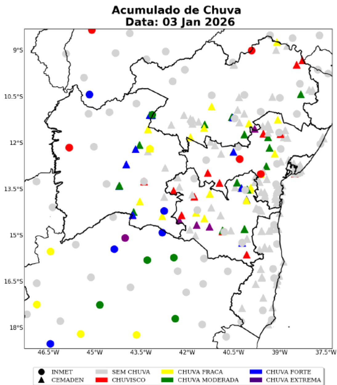
Figura 1 – Mapa do acumulado de chuva sobre o estado da Bahia em 03 de janeiro.
