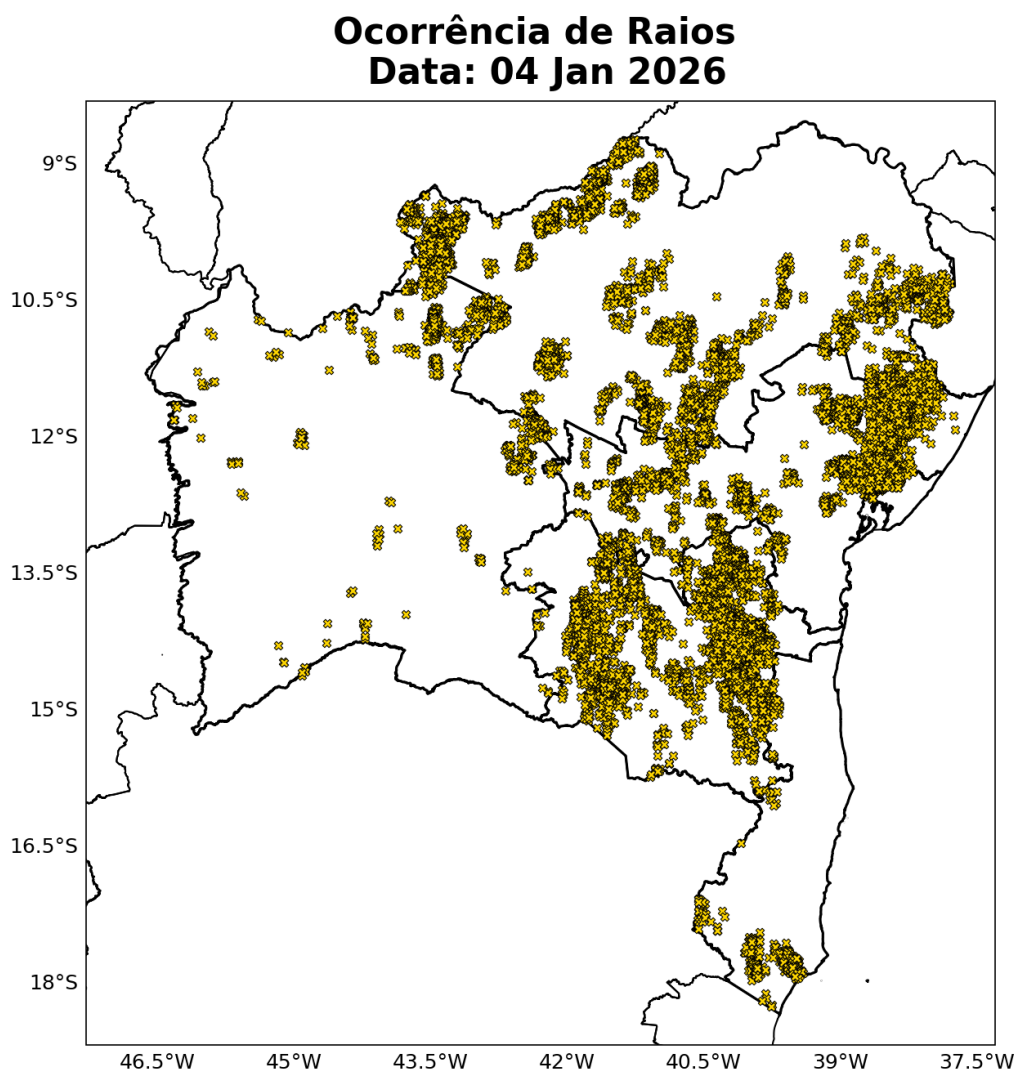
Figura 14: Ocorrências de descargas atmosféricas nuvem-solo detectadas pelo sistema Earth Networks para o dia 04 de Janeiro sobre a área de concessão da COELBA.
