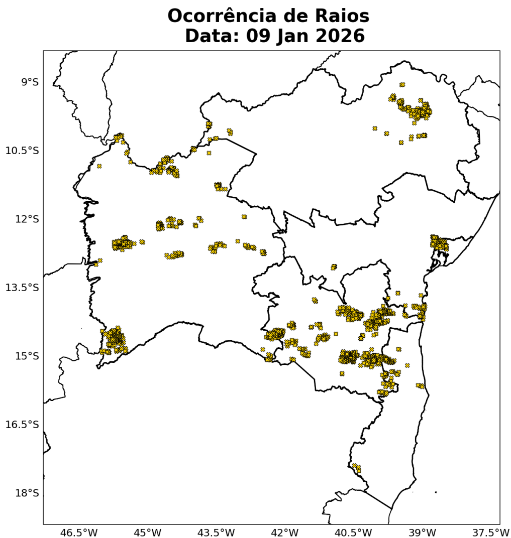
Figura 19: Ocorrências de descargas atmosféricas nuvem-solo detectadas pelo sistema Earth Networks para o dia 09 de Janeiro sobre a área de concessão da COELBA.
