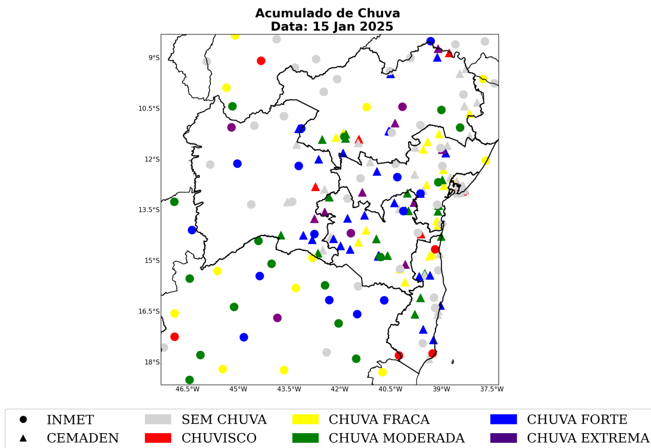
Figura 53: Acumulado diário de precipitação sobre o estado de Bahia para o dia 15 de janeiro, baseado nas estações meteorológicas do INMET e CEMADEN.
