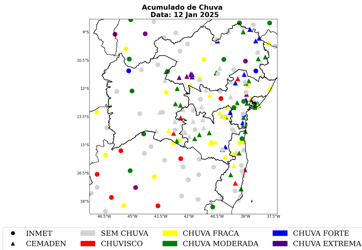
Figura 50: Acumulado diário de precipitação sobre o estado de Bahia para o dia 12 de janeiro, baseado nas estações meteorológicas do INMET e CEMADEN.
