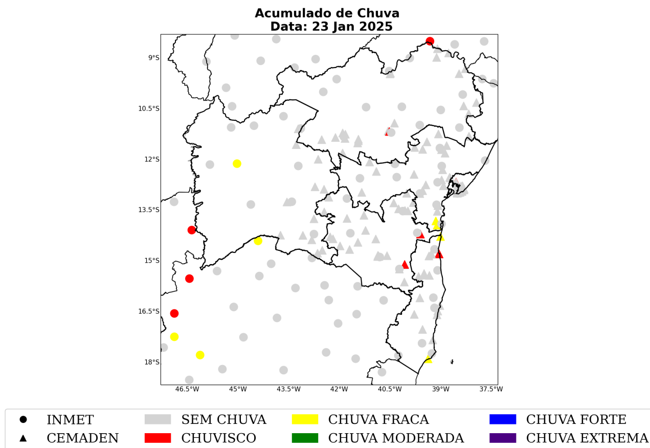
Figura 61: Acumulado diário de precipitação sobre a área de concessão da Neoenergia-COELBA para o dia 23 de janeiro, baseado nas estações meteorológicas do INMET e CEMADEN.
