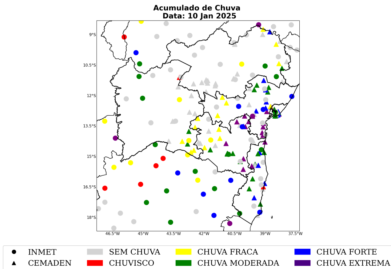
Figura 48: Acumulado diário de precipitação sobre o estado de Bahia para o dia 10 de janeiro, baseado nas estações meteorológicas do INMET e CEMADEN.
