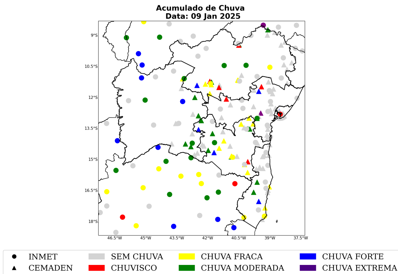
Figura 47: Acumulado diário de precipitação sobre o estado de Bahia para o dia 09 de janeiro, baseado nas estações meteorológicas do INMET e CEMADEN.
