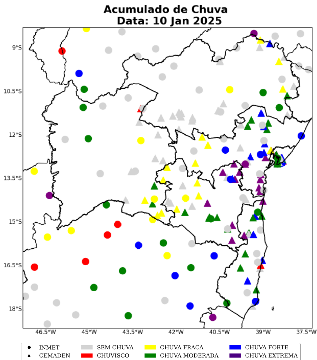
Figura 1 – Mapa do acumulado de chuva sobre o estado da Bahia entre 10 de janeiro.
