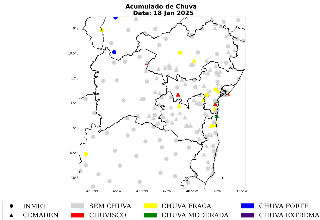
Figura 56: Acumulado diário de precipitação sobre a área de concessão da Neoenergia-COELBA para o dia 18 de janeiro, baseado nas estações meteorológicas do INMET e CEMADEN.
