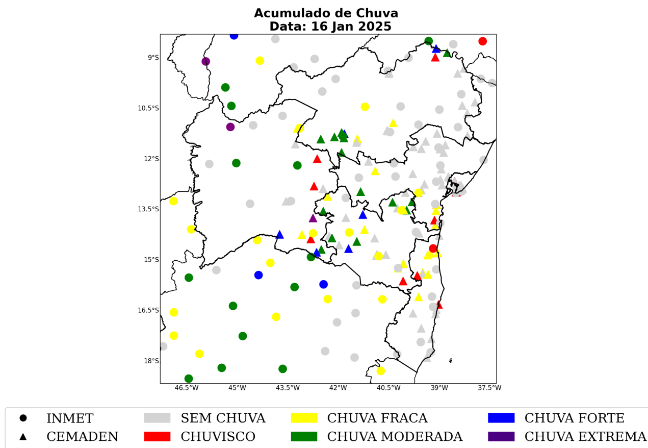
Figura 54: Acumulado diário de precipitação sobre a área de concessão da Neoenergia-COELBA para o dia 16 de janeiro, baseado nas estações meteorológicas do INMET e CEMADEN.
