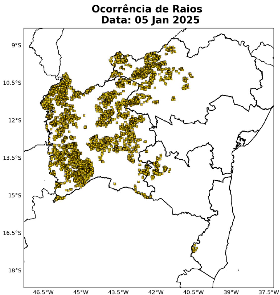
Figura 3 – Mapa de descargas atmosféricas sobre o estado da Bahia no dia 05 de janeiro.
