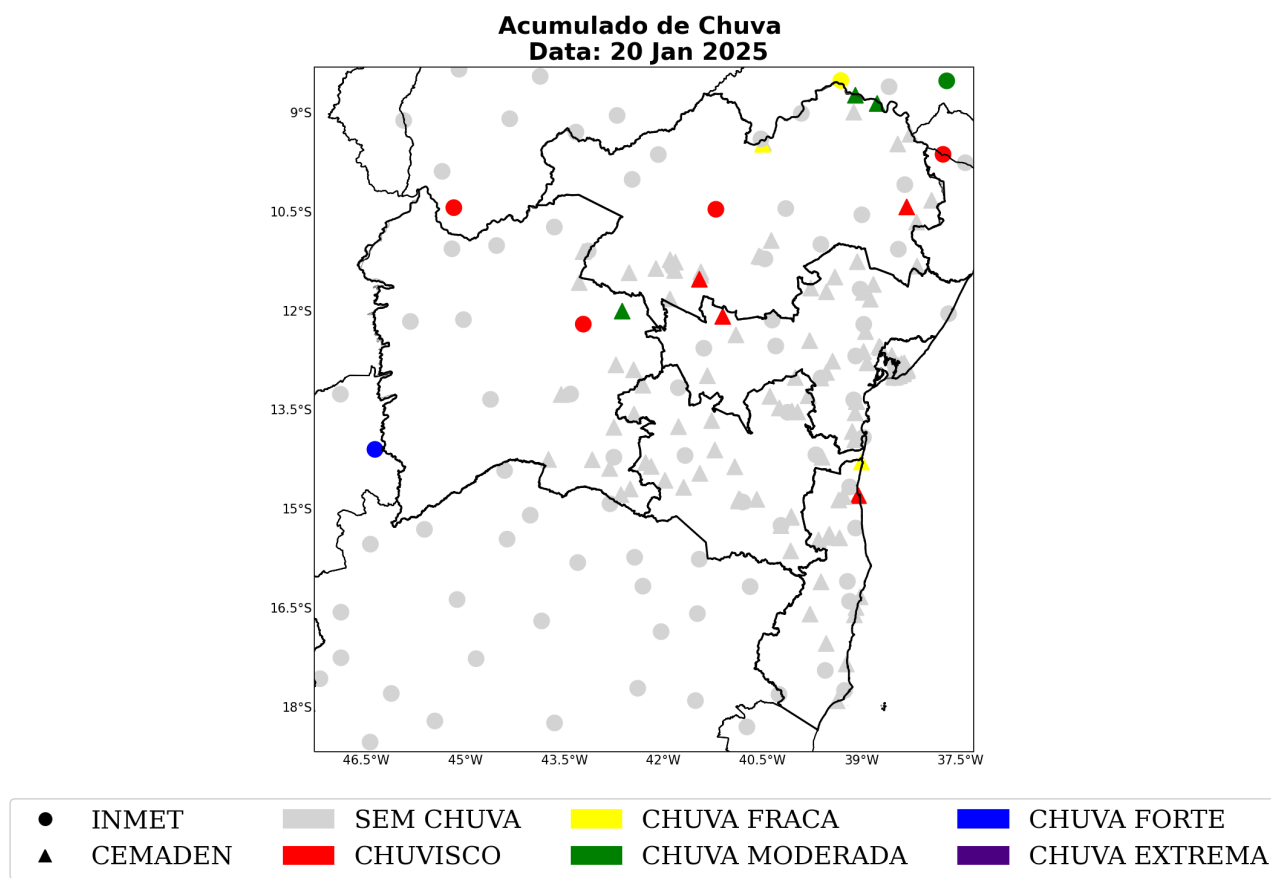
Figura 58: Acumulado diário de precipitação sobre a área de concessão da Neoenergia-COELBA para o dia 20 de janeiro, baseado nas estações meteorológicas do INMET e CEMADEN.
