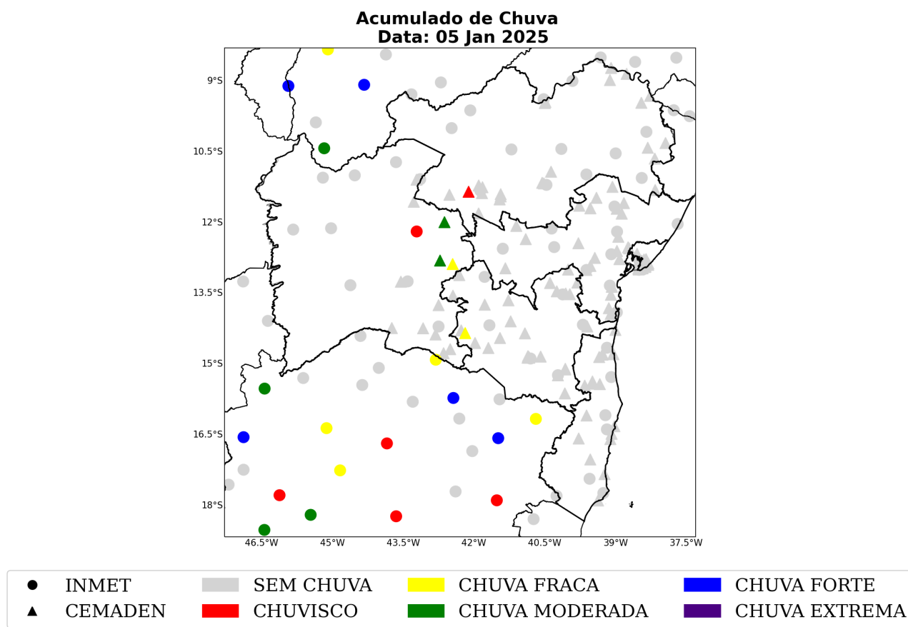
Figura 43: Acumulado diário de precipitação sobre o estado de Bahia para o dia 05 de janeiro, baseado nas estações meteorológicas do INMET e CEMADEN.
