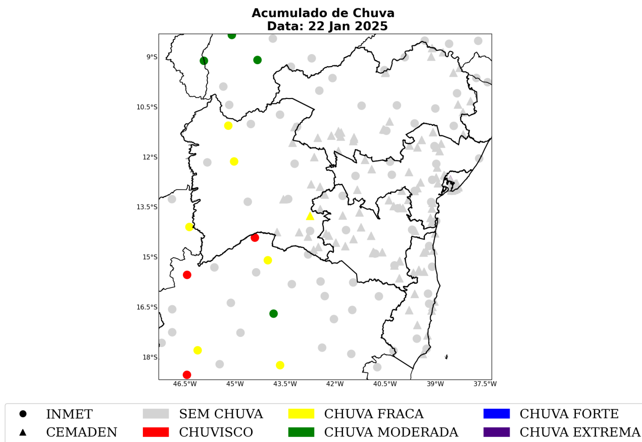
Figura 60: Acumulado diário de precipitação sobre a área de concessão da Neoenergia-COELBA para o dia 22 de janeiro, baseado nas estações meteorológicas do INMET e CEMADEN.
