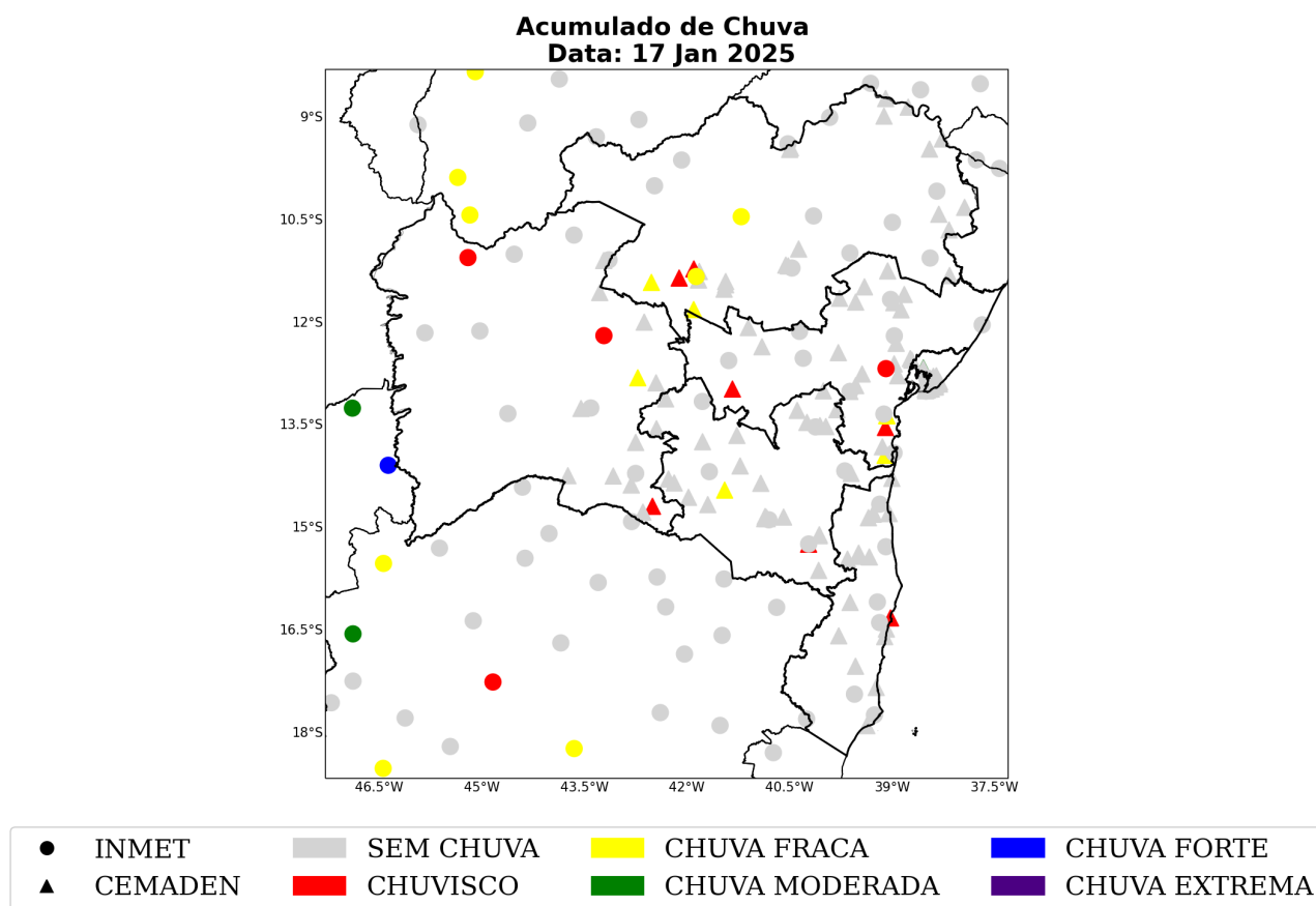
Figura 55: Acumulado diário de precipitação sobre a área de concessão da Neoenergia-COELBA para o dia 17 de janeiro, baseado nas estações meteorológicas do INMET e CEMADEN.
