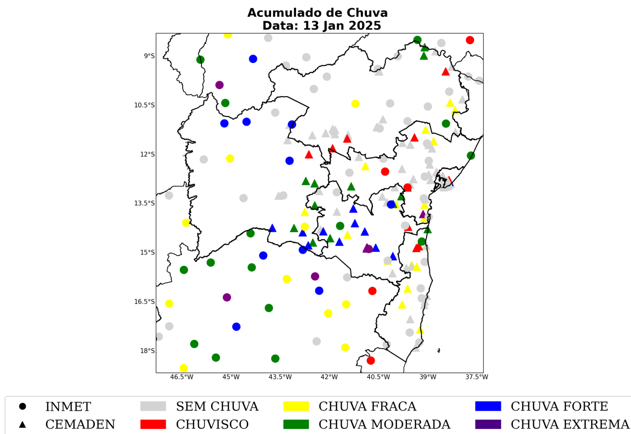
Figura 51: Acumulado diário de precipitação sobre o estado de Bahia para o dia 13 de janeiro, baseado nas estações meteorológicas do INMET e CEMADEN.
