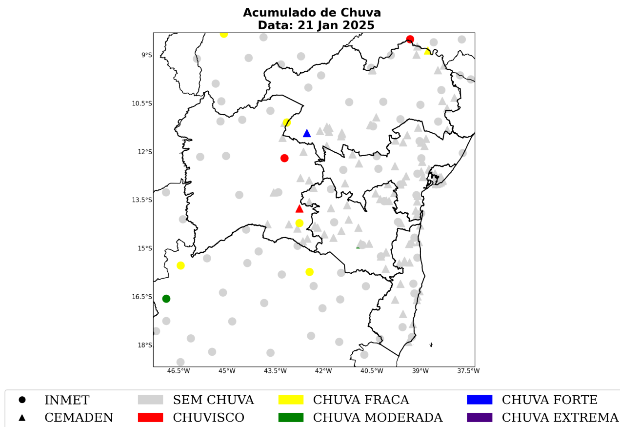
Figura 59: Acumulado diário de precipitação sobre a área de concessão da Neoenergia-COELBA para o dia 21 de janeiro, baseado nas estações meteorológicas do INMET e CEMADEN.
