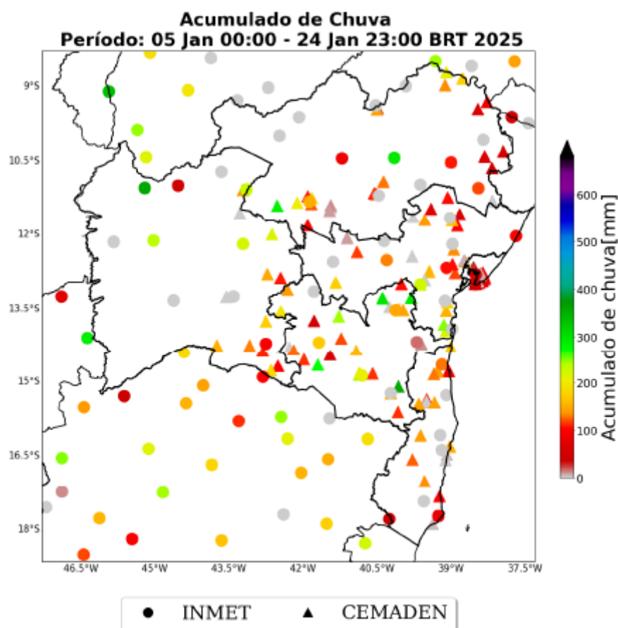
Figura 8 – Mapa Acumulado de Chuva de 05 a 24 de janeiro.
