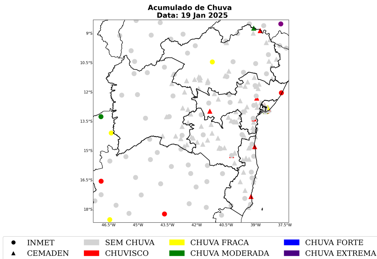
Figura 57: Acumulado diário de precipitação sobre a área de concessão da Neoenergia-COELBA para o dia 19 de janeiro, baseado nas estações meteorológicas do INMET e CEMADEN.
