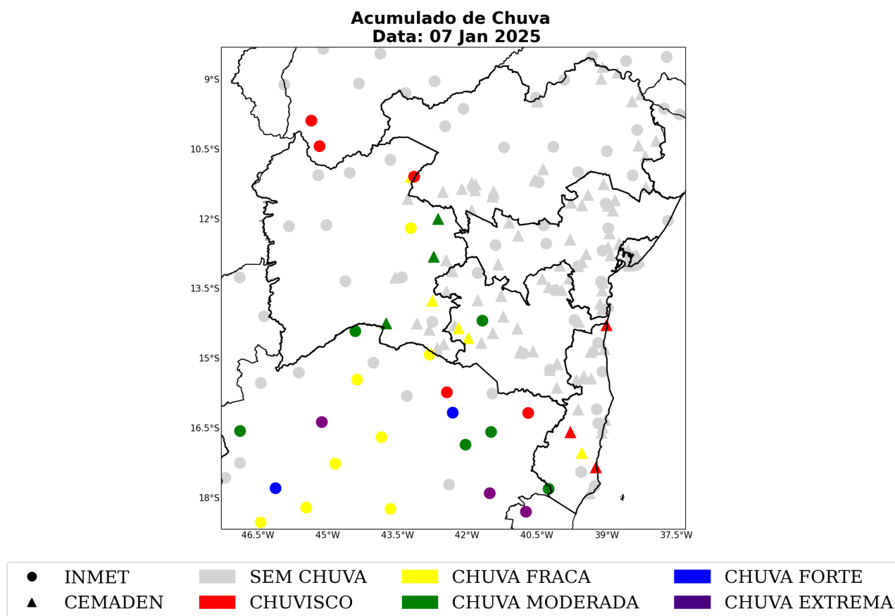
Figura 29: Acumulado diário de precipitação sobre o estado de Bahia para o dia 07 de janeiro, baseado nas estações meteorológicas do INMET e CEMADEN.
