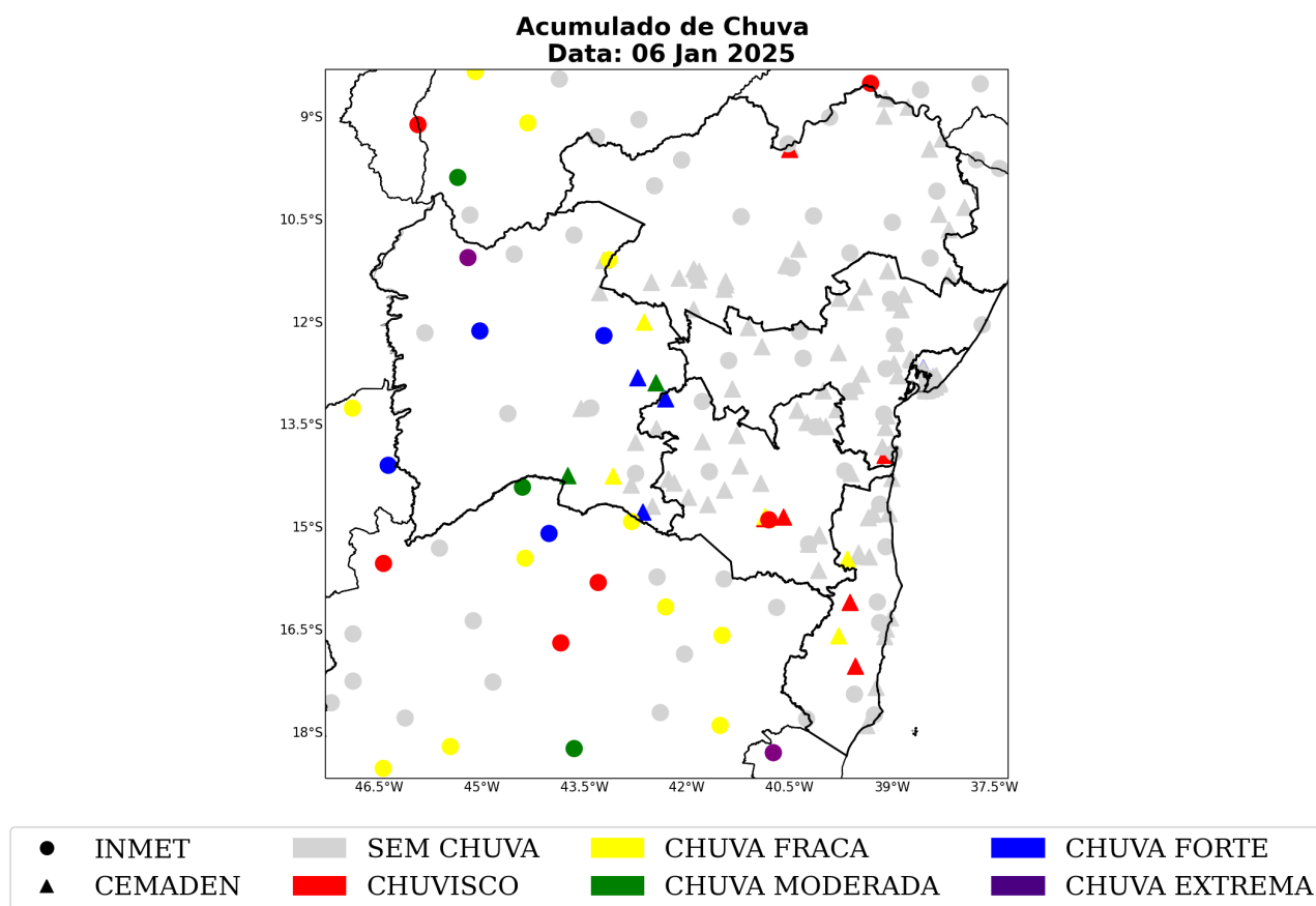
Figura 28: Acumulado diário de precipitação sobre o estado de Bahia para o dia 06 de janeiro, baseado nas estações meteorológicas do INMET e CEMADEN.
