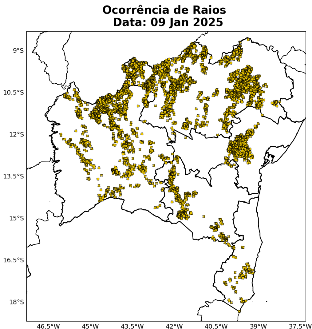
Figura 18: Ocorrência de descargas atmosféricas nuvem-solo detectadas pelo sistema Earth Networks para o dia 09 de janeiro sobre a área de concessão da Neoenergia-COELBA.
