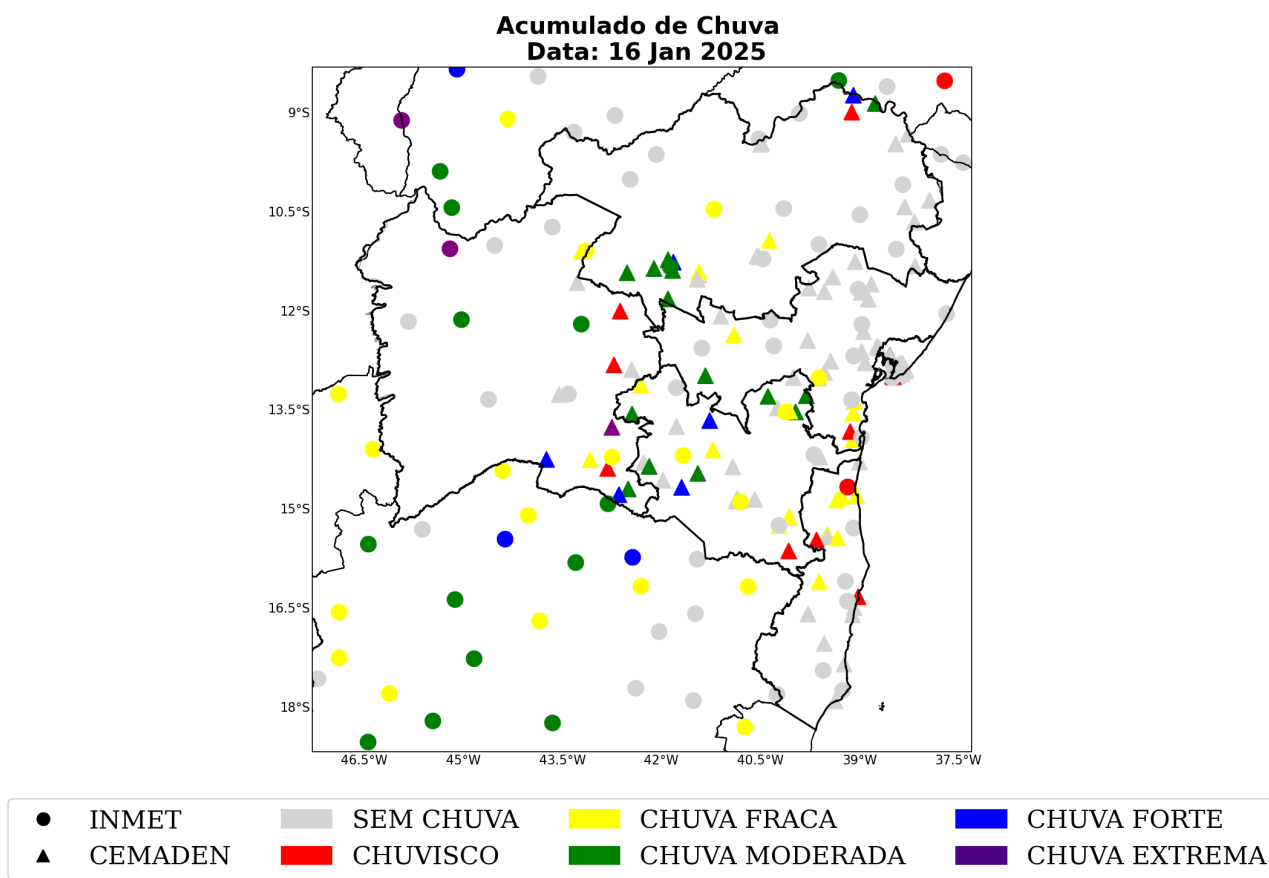
Figura 38: Acumulado diário de precipitação sobre a área de concessão da Neoenergia-COELBA para o dia 16 de janeiro, baseado nas estações meteorológicas do INMET e CEMADEN.
