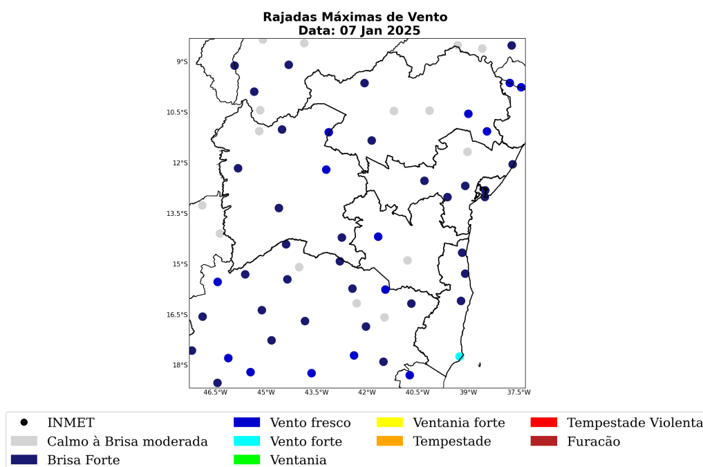
Figura 42: Rajada de vento sobre o estado de Bahia para o dia 07 de janeiro, baseado nas estações meteorológicas do INMET.
