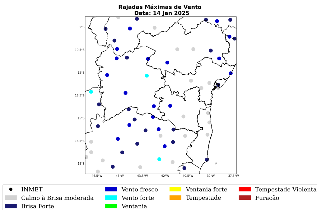
Figura 49: Rajada de vento sobre o estado de Bahia para o dia 14 de janeiro, baseado nas estações meteorológicas do INMET.
