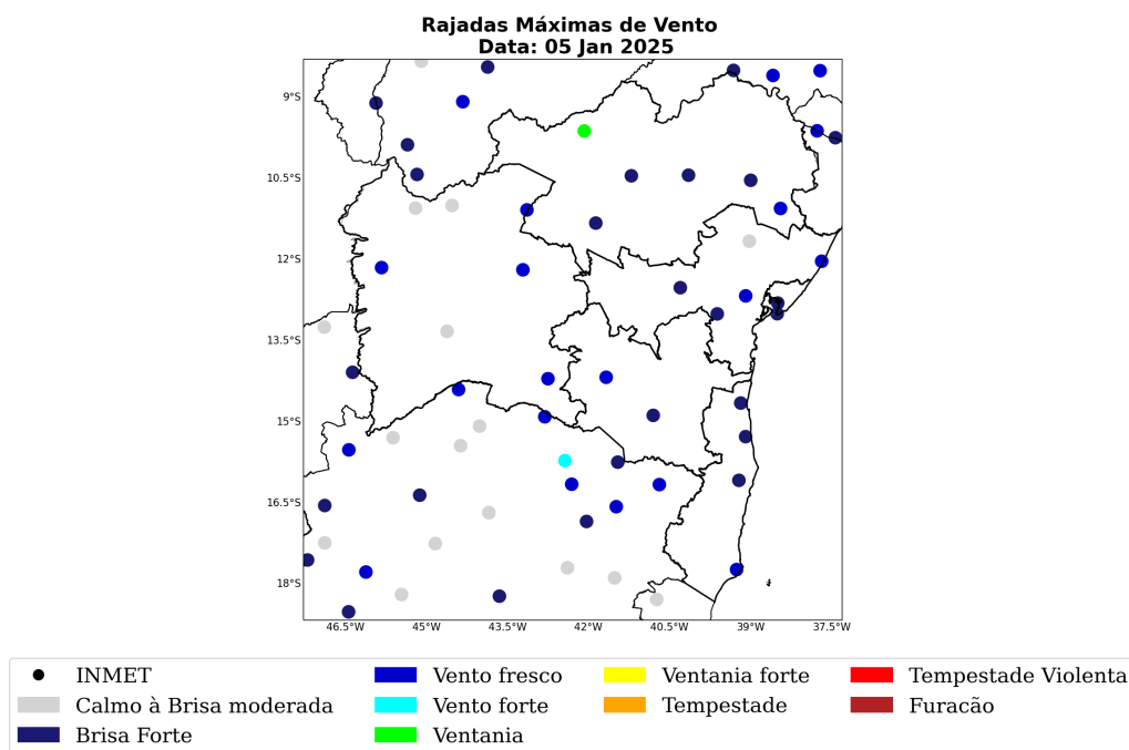
Figura 40: Rajada de vento sobre o estado de Bahia para o dia 05 de janeiro, baseado nas estações meteorológicas do INMET.
