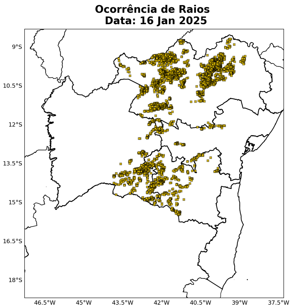
Figura 25: Densidade de descargas atmosféricas nuvem-solo detectadas pelo sistema Earth Networks para o dia 16 de janeiro sobre a área de concessão da Neoenergia-COELBA.
