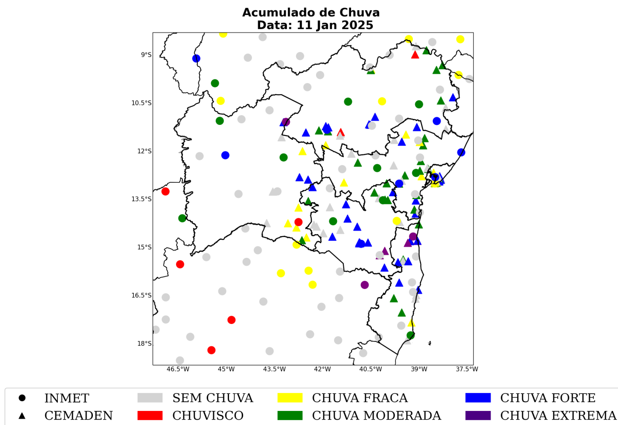
Figura 33: Acumulado diário de precipitação sobre o estado de Bahia para o dia 11 de janeiro, baseado nas estações meteorológicas do INMET e CEMADEN.
