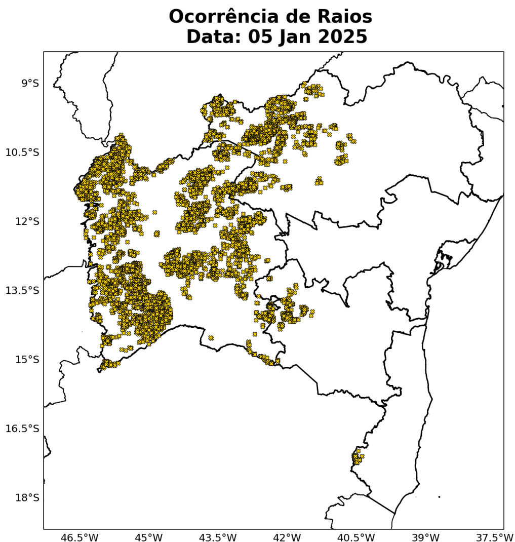
Figura 14: Ocorrência de descargas atmosféricas nuvem-solo detectadas pelo sistema Earth Networks para o dia 05 de janeiro sobre a área de concessão da Neoenergia-COELBA.
