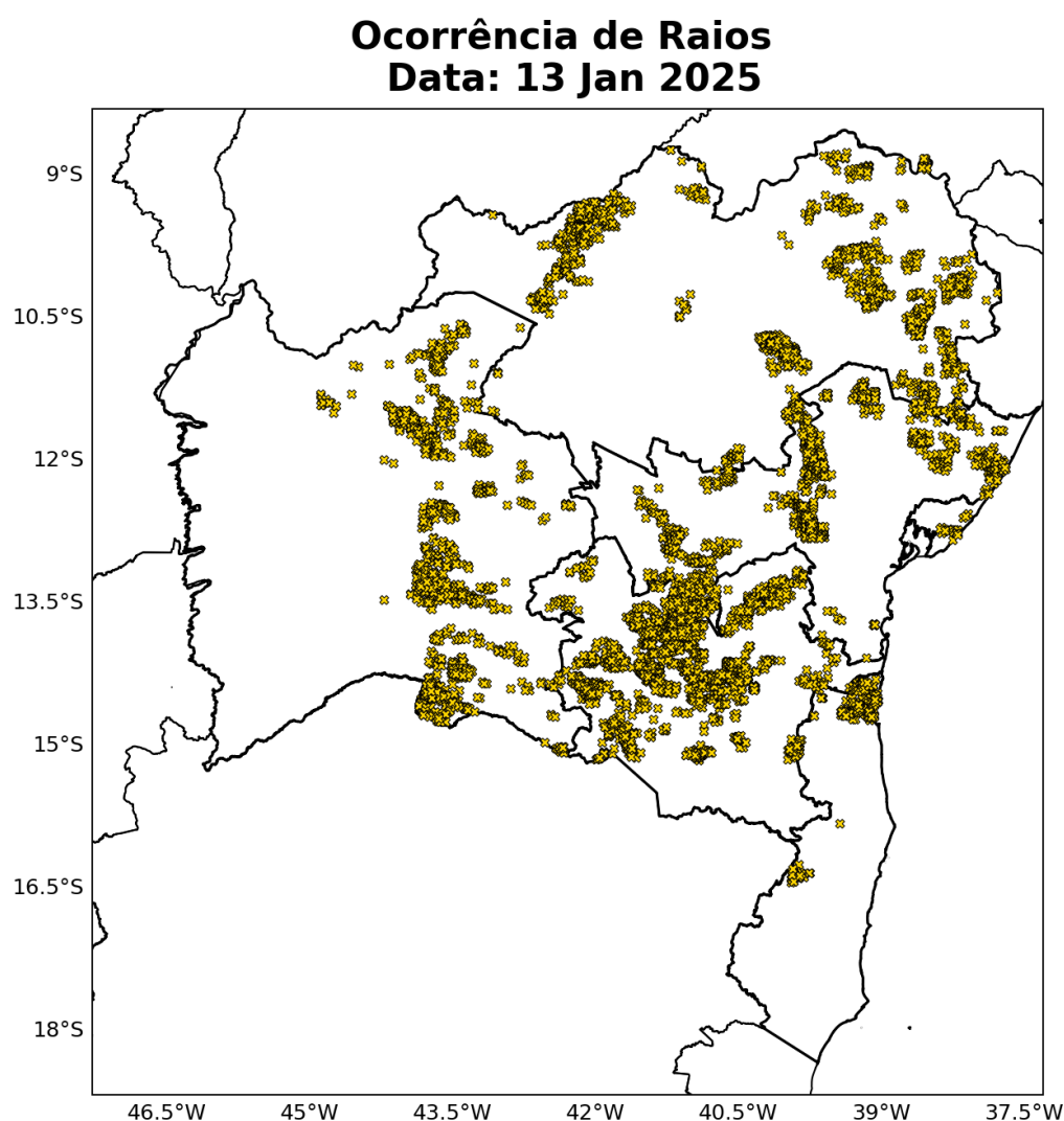
Figura 22: Ocorrência de descargas atmosféricas nuvem-solo detectadas pelo sistema Earth Networks para o dia 13 de janeiro sobre a área de concessão da Neoenergia-COELBA.
