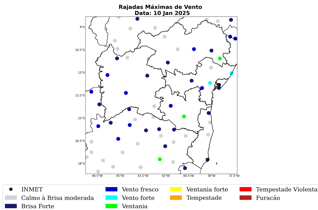
Figura 45: Rajada de vento sobre o estado de Bahia para o dia 10 de janeiro, baseado nas estações meteorológicas do INMET.
