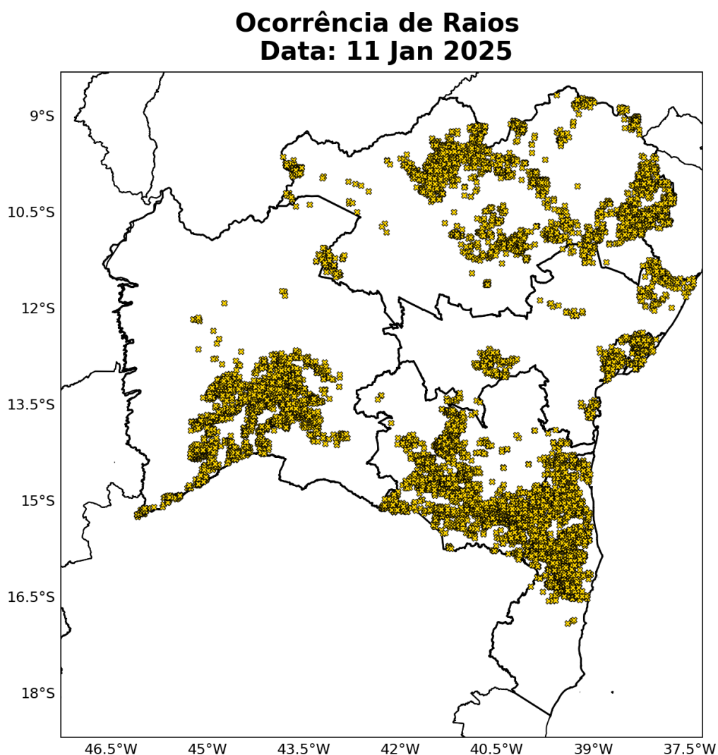
Figura 20: Ocorrência de descargas atmosféricas nuvem-solo detectadas pelo sistema Earth Networks para o dia 11 de janeiro sobre a área de concessão da Neoenergia-COELBA.
