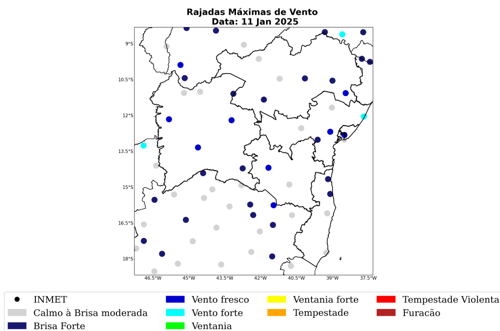
Figura 46: Rajada de vento sobre o estado de Bahia para o dia 11 de janeiro, baseado nas estações meteorológicas do INMET.
