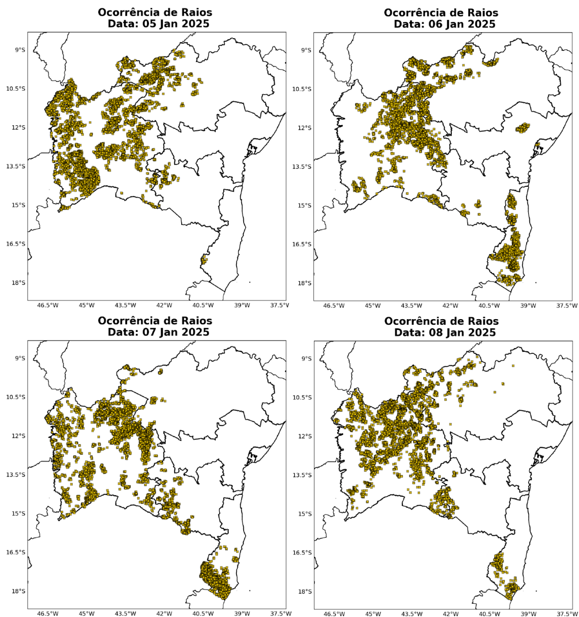
Figura 20 – Mapas de ocorrência de raios nos dias 05, 06, 07 e 08 de janeiro.
