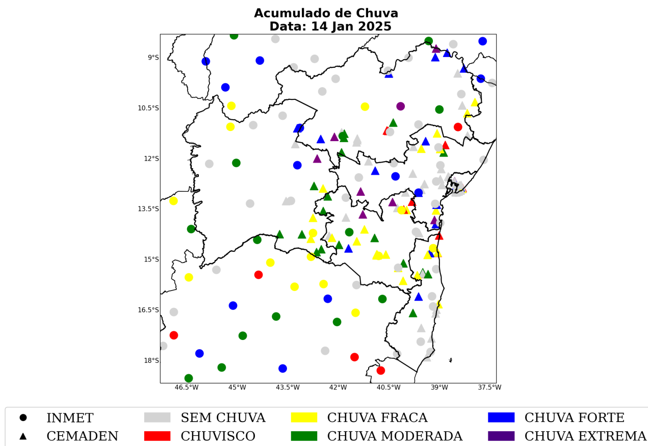
Figura 36: Acumulado diário de precipitação sobre o estado de Bahia para o dia 14 de janeiro, baseado nas estações meteorológicas do INMET e CEMADEN.
