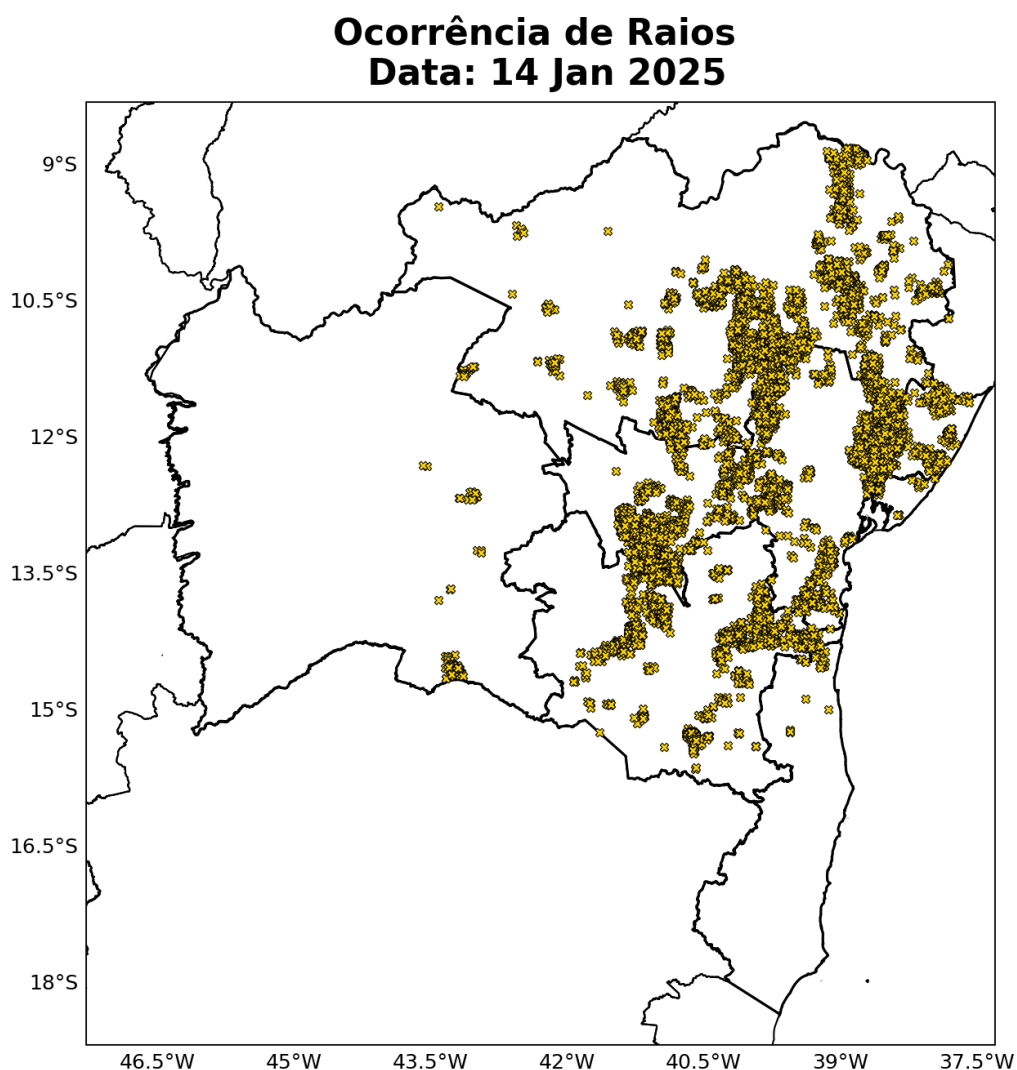
Figura 23: Ocorrência de descargas atmosféricas nuvem-solo detectadas pelo sistema Earth Networks para o dia 14 de janeiro sobre a área de concessão da Neoenergia-COELBA.
