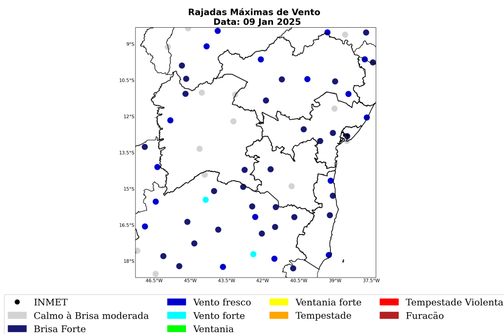
Figura 44: Rajada de vento sobre o estado de Bahia para o dia 09 de janeiro, baseado nas estações meteorológicas do INMET.
