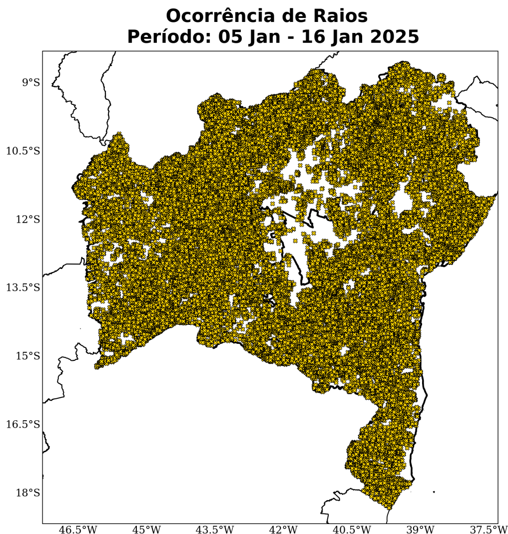
Figura 26: Ocorrência de descargas atmosféricas nuvem-solo detectadas pelo sistema Earth Networks para o período de 05 a 16 de janeiro de 2025 sobre a área de concessão da Neoenergia-COELBA.
