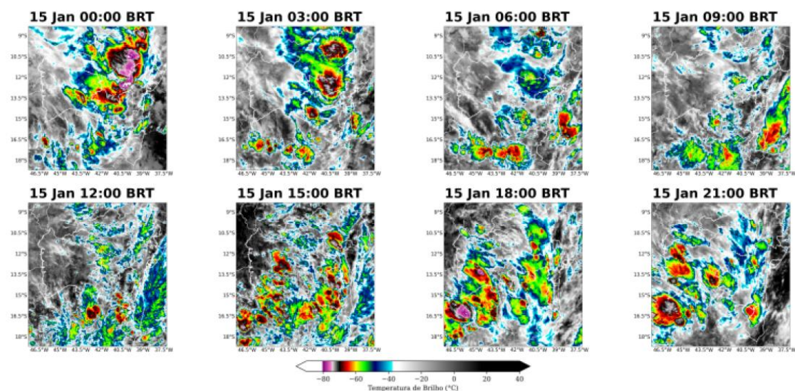
Figura 19 – Imagens realçadas do satélite GOES-16 das 00h00, 03h00, 06h00, 09h00, 12h00, 15h00, 18h00, e 21h00 do dia 15 de janeiro de 2025. Fonte: Climatempo
