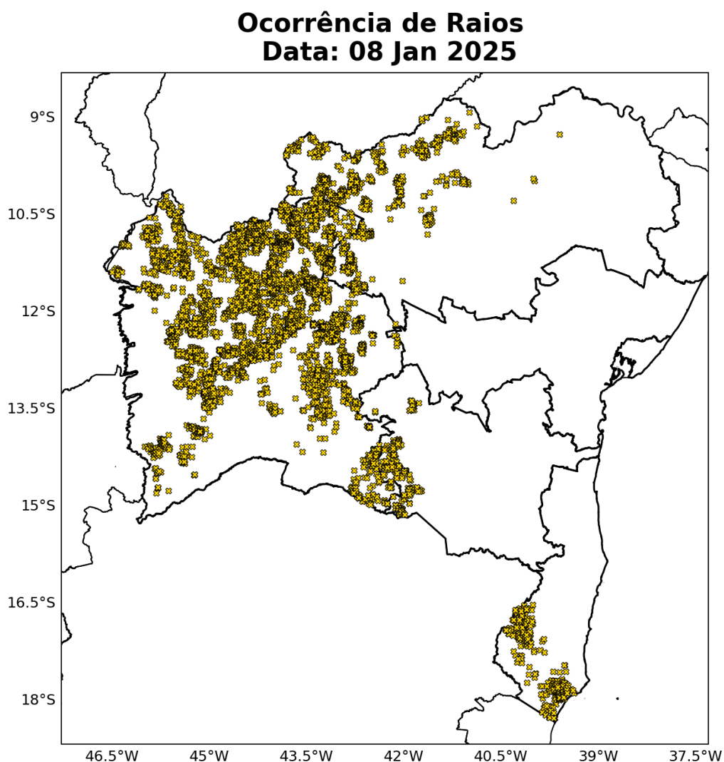
Figura 17: Ocorrência de descargas atmosféricas nuvem-solo detectadas pelo sistema Earth Networks para o dia 08 de janeiro sobre a área de concessão da Neoenergia-COELBA.
