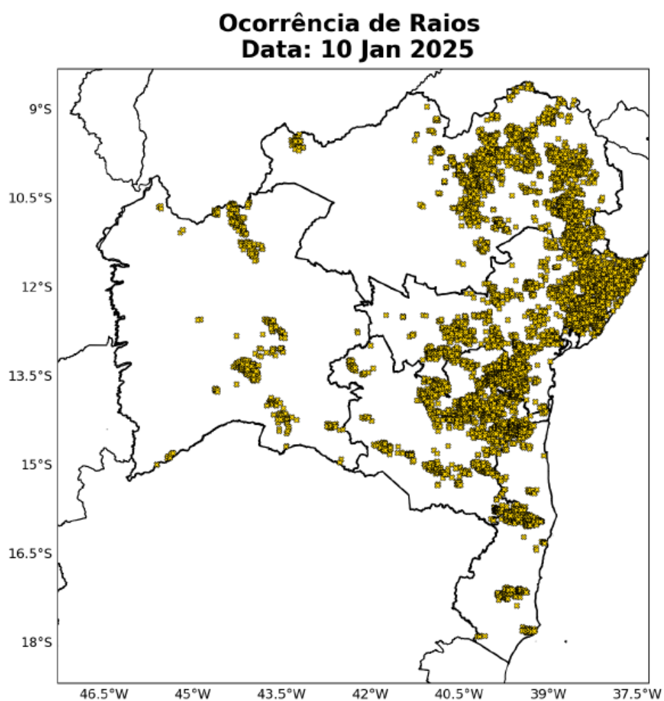
Figura 3 – Mapa de descargas atmosféricas sobre o estado da Bahia no dia 10 de janeiro.
