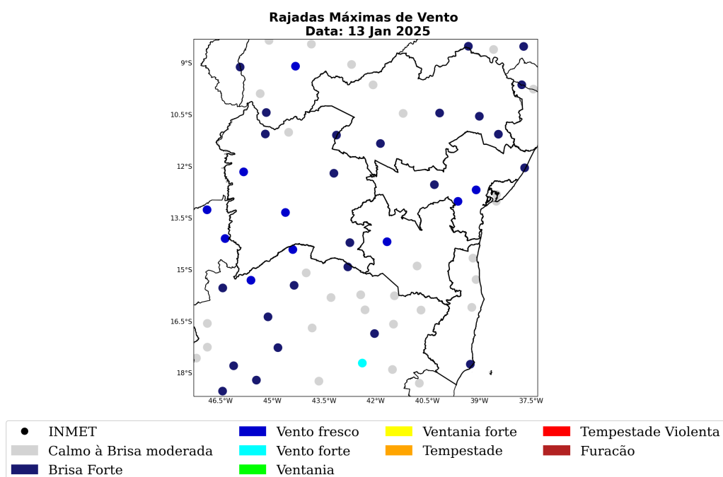
Figura 48: Rajada de vento sobre o estado de Bahia para o dia 13 de janeiro, baseado nas estações meteorológicas do INMET.
