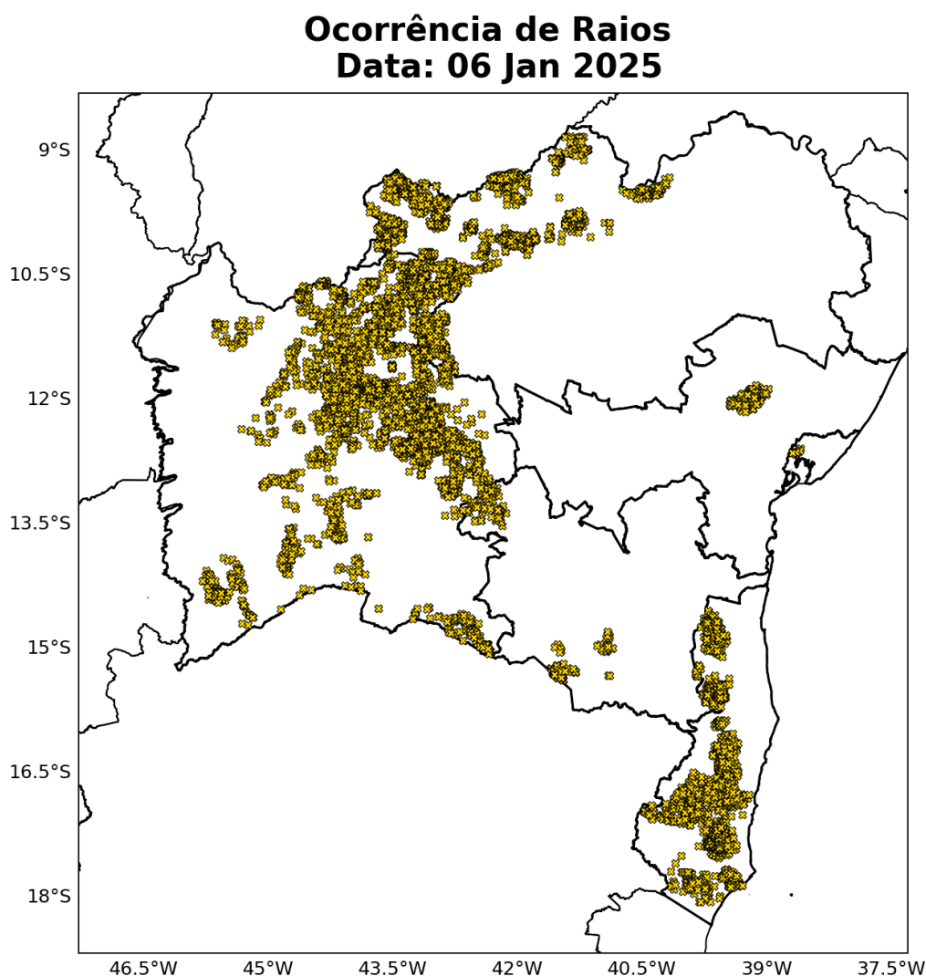
Figura 15: Ocorrência de descargas atmosféricas nuvem-solo detectadas pelo sistema Earth Networks para o dia 06 de janeiro sobre a área de concessão da Neoenergia-COELBA.
