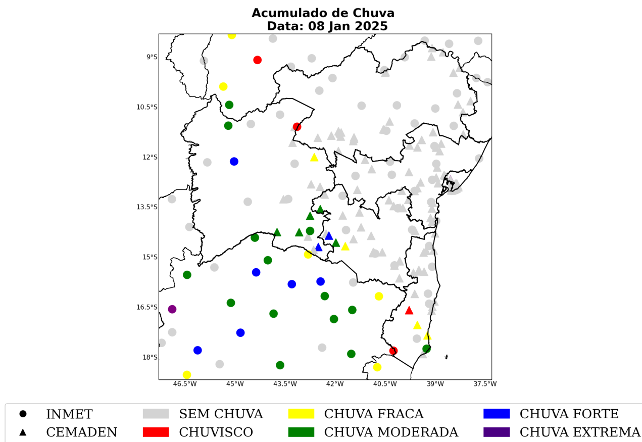
Figura 30: Acumulado diário de precipitação sobre o estado de Bahia para o dia 08 de janeiro, baseado nas estações meteorológicas do INMET e CEMADEN.
