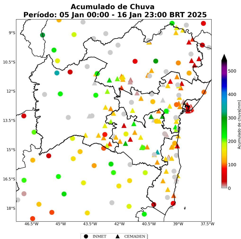
Figura 39: Acumulado de precipitação sobre o estado de Bahia para o período de 05 a 16 de janeiro de 2025, baseado nas estações meteorológicas do INMET e CEMADEN.
