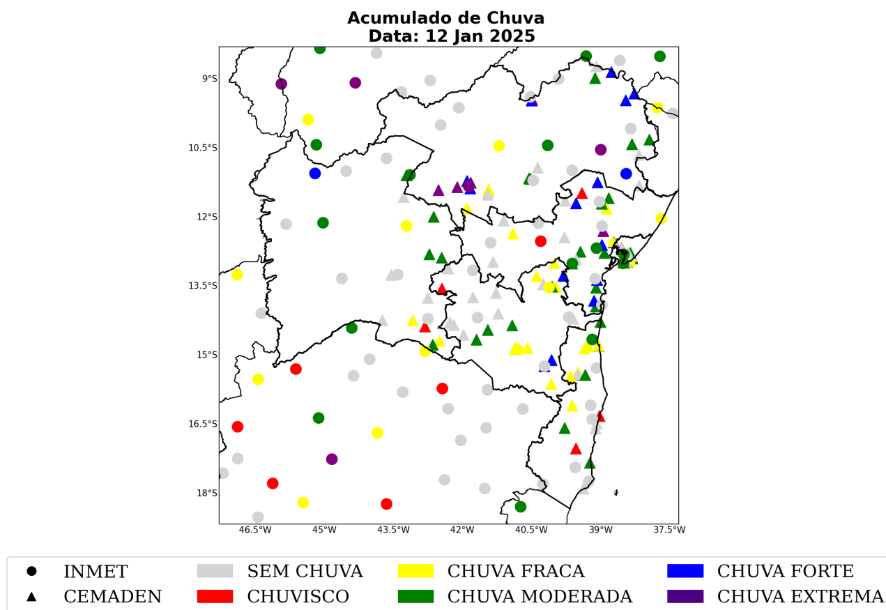
Figura 34: Acumulado diário de precipitação sobre o estado de Bahia para o dia 12 de janeiro, baseado nas estações meteorológicas do INMET e CEMADEN.
