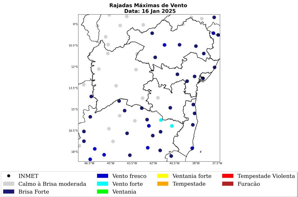
Figura 51: Máxima rajada de vento diária sobre a área de concessão da Neoenergia-COELBA para o dia 16 de janeiro, baseado nas estações meteorológicas do INMET.
