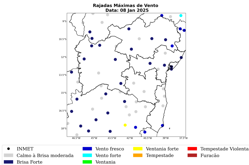
Figura 43: Rajada de vento sobre o estado de Bahia para o dia 08 de janeiro, baseado nas estações meteorológicas do INMET.
