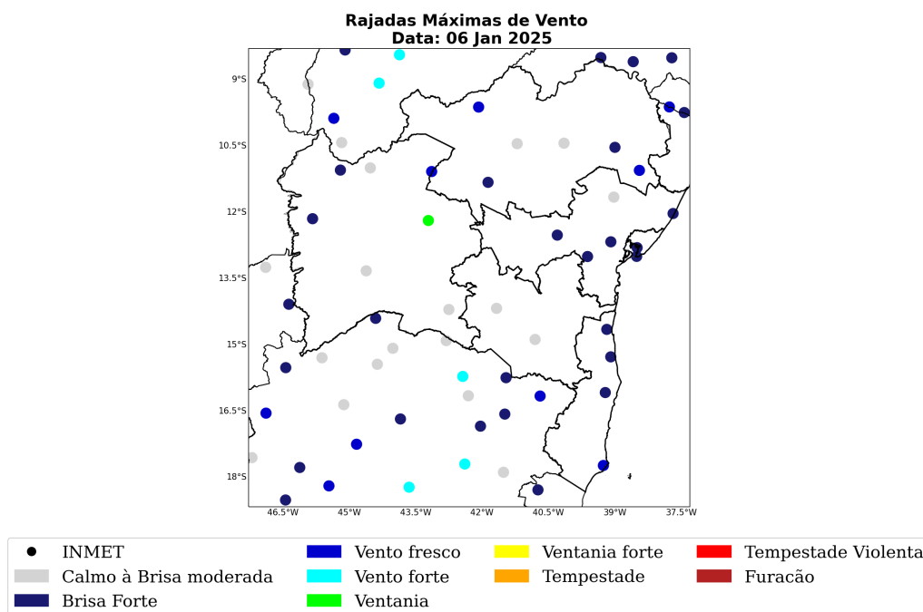
Figura 41: Rajada de vento sobre o estado de Bahia para o dia 06 de janeiro, baseado nas estações meteorológicas do INMET.
