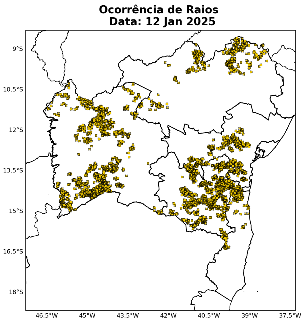
Figura 21: Ocorrência de descargas atmosféricas nuvem-solo detectadas pelo sistema Earth Networks para o dia 12 de janeiro sobre a área de concessão da Neoenergia-COELBA.
