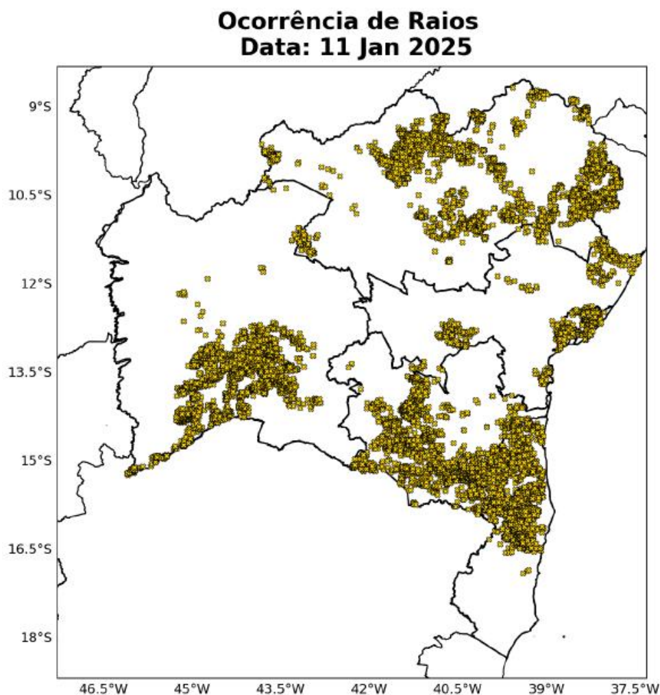
Figura 4 – Mapa de descargas atmosféricas sobre o estado da Bahia no dia 11 de janeiro.
