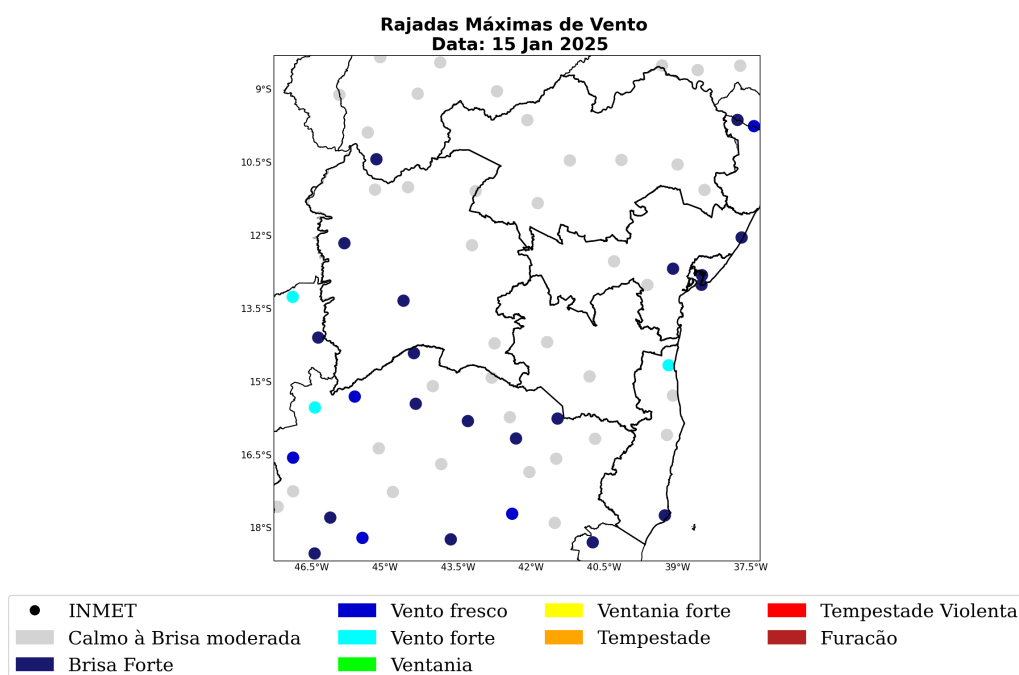
Figura 50: Rajada de vento sobre o estado de Bahia para o dia 15 de janeiro, baseado nas estações meteorológicas do INMET.
