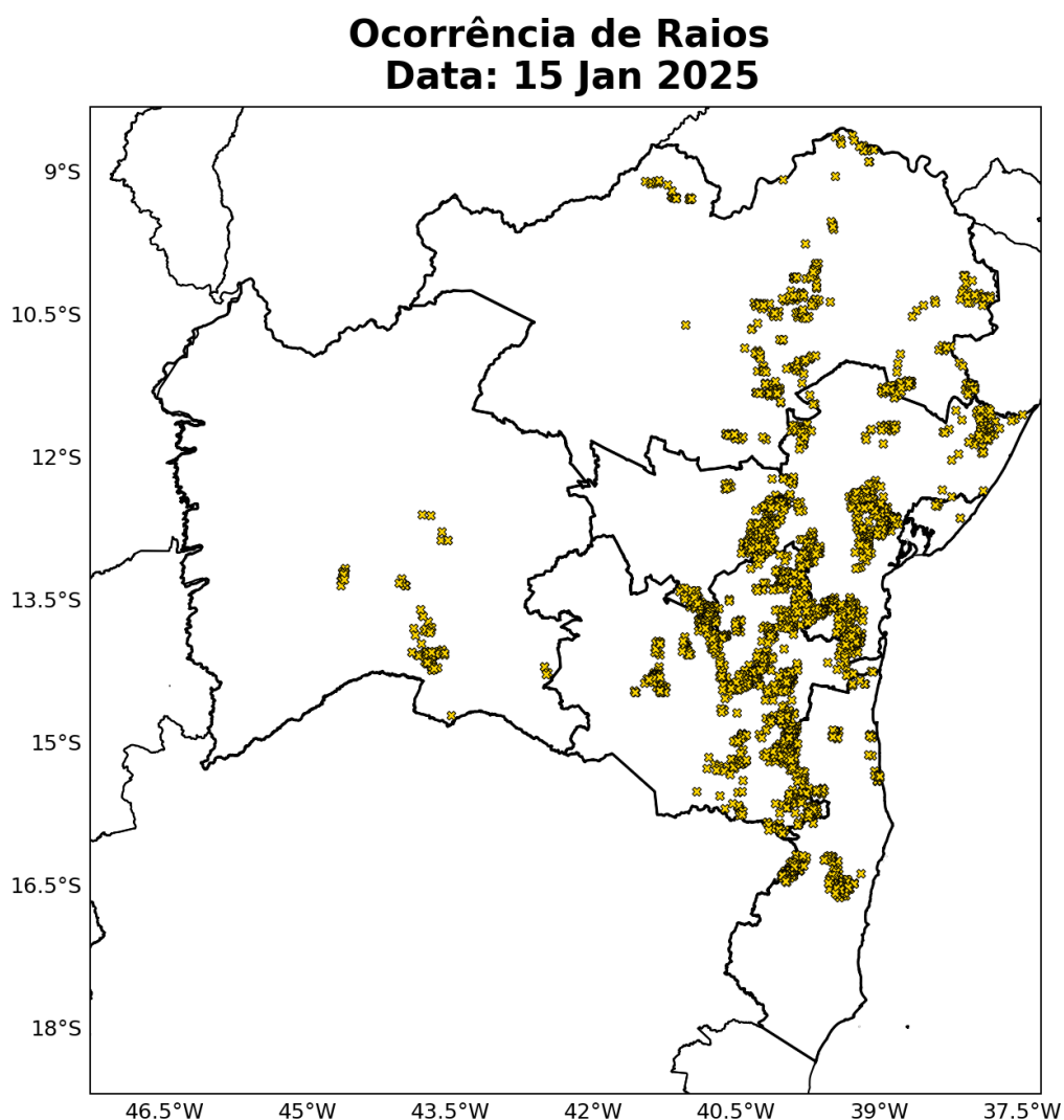
Figura 24: Ocorrência de descargas atmosféricas nuvem-solo detectadas pelo sistema Earth Networks para o dia 15 de janeiro sobre a área de concessão da Neoenergia-COELBA.
