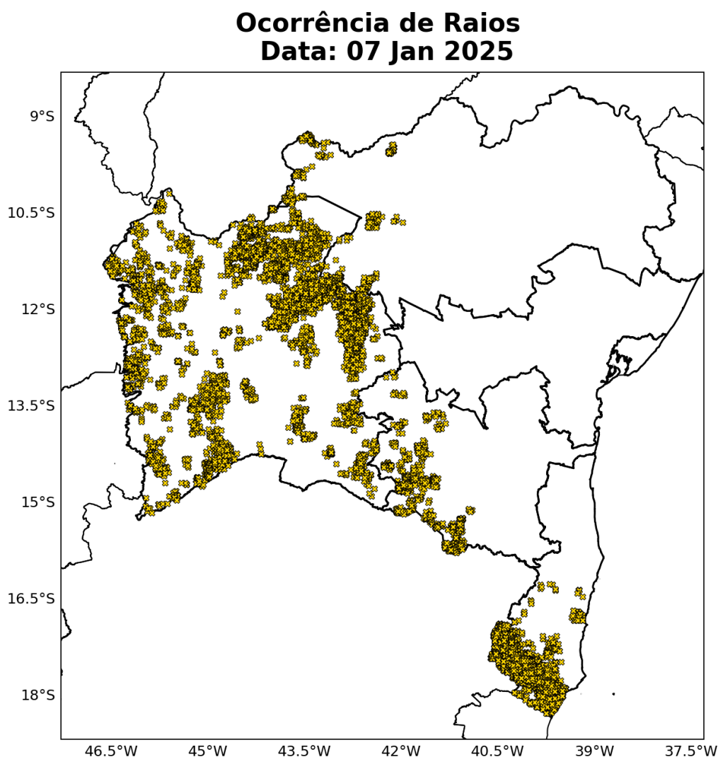
Figura 16: Ocorrência de descargas atmosféricas nuvem-solo detectadas pelo sistema Earth Networks para o dia 07 de janeiro sobre a área de concessão da Neoenergia-COELBA.
