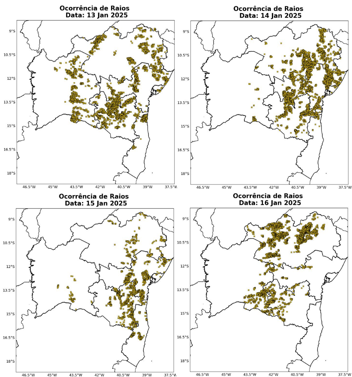
Figura 22 – Mapas de ocorrência de raios nos dias 13, 14, 15 e 16 de janeiro.
