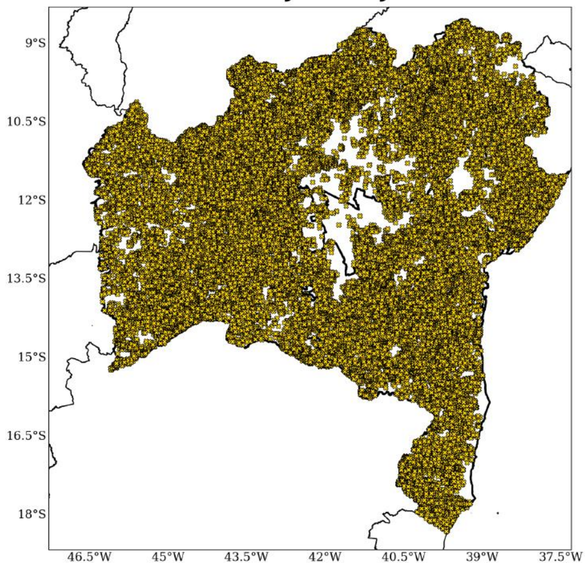
Figura 23 – Mapa de ocorrência de raios acumulado de 05 a 16 de janeiro.
