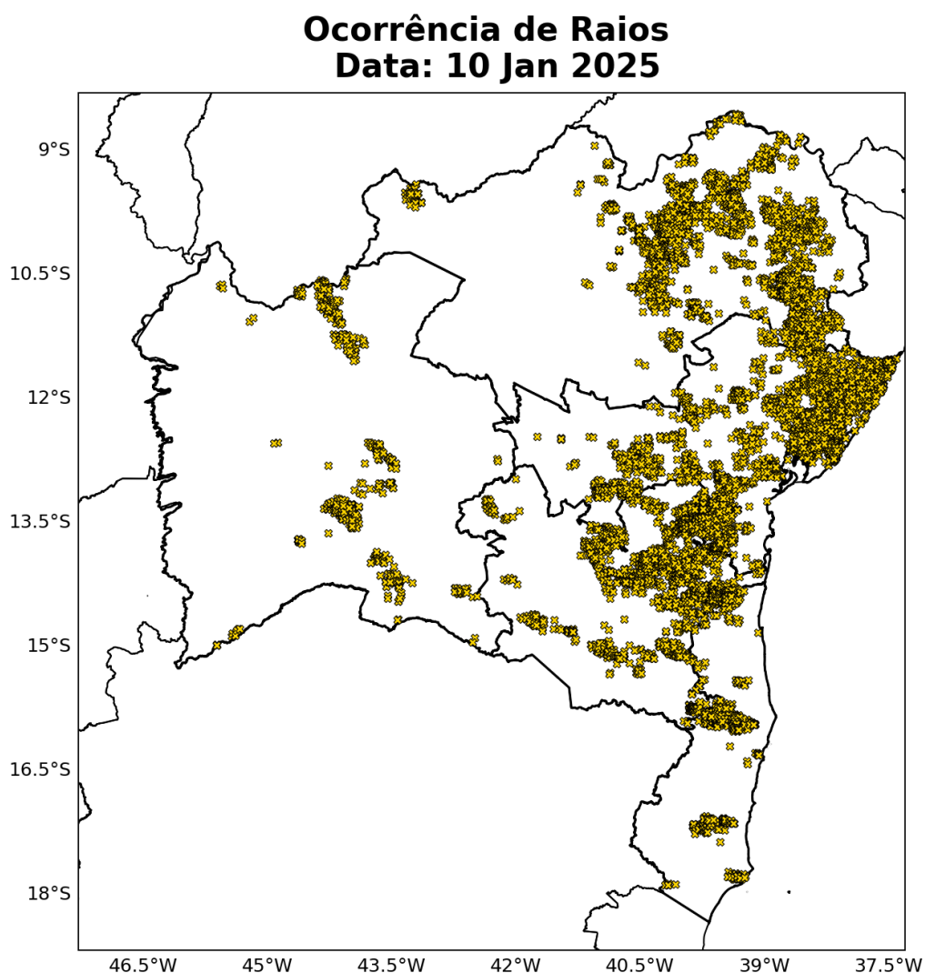
Figura 19: Ocorrência de descargas atmosféricas nuvem-solo detectadas pelo sistema Earth Networks para o dia 10 de janeiro sobre a área de concessão da Neoenergia-COELBA.
