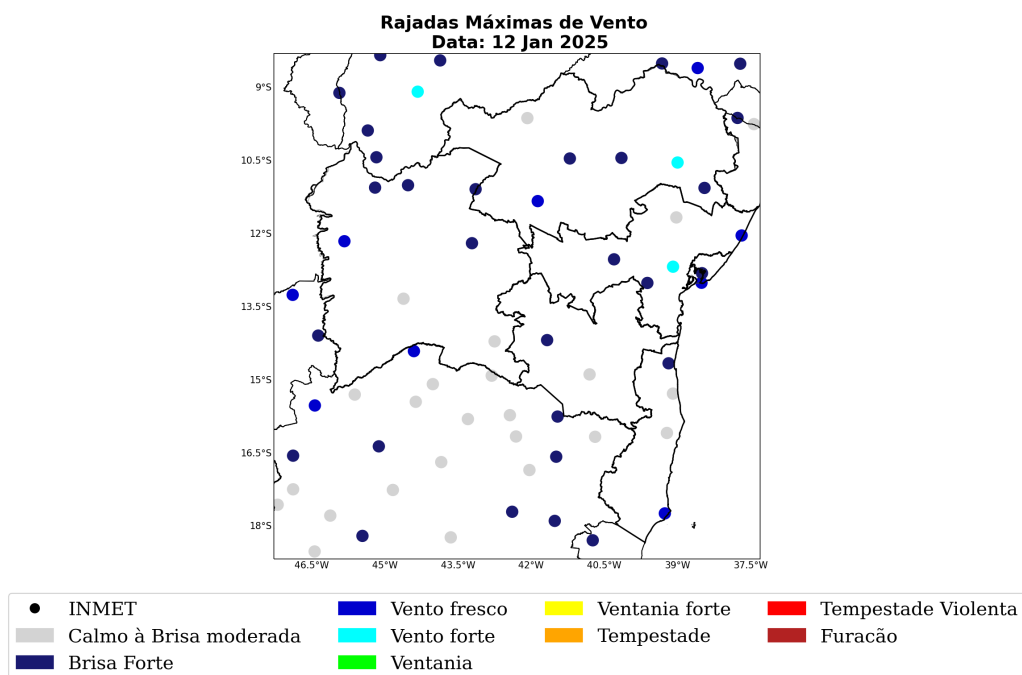
Figura 47: Rajada de vento sobre o estado de Bahia para o dia 12 de janeiro, baseado nas estações meteorológicas do INMET.
