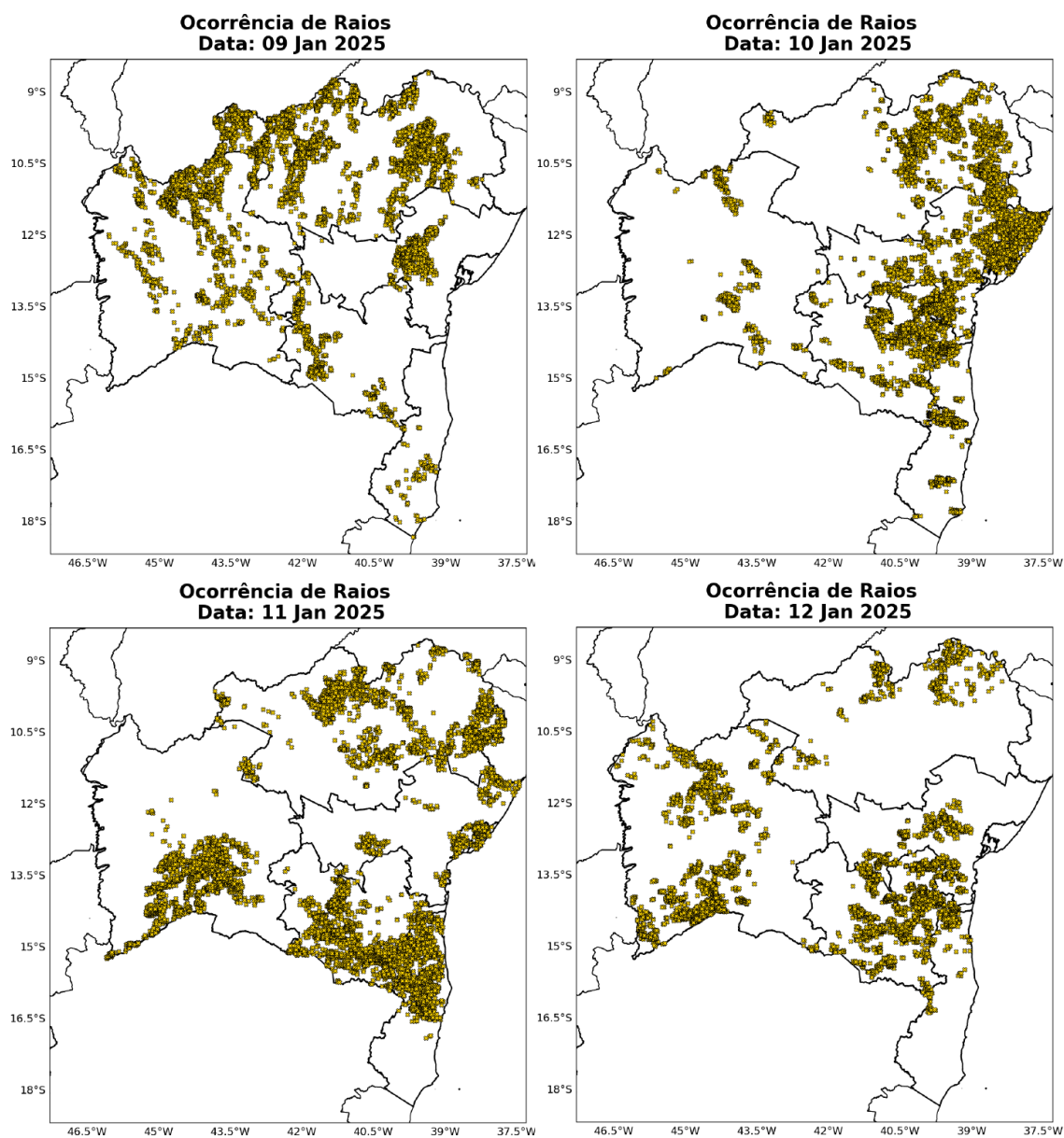
Figura 21 – Mapas de ocorrência de raios nos dias 09, 10, 11 e 12 de janeiro.
