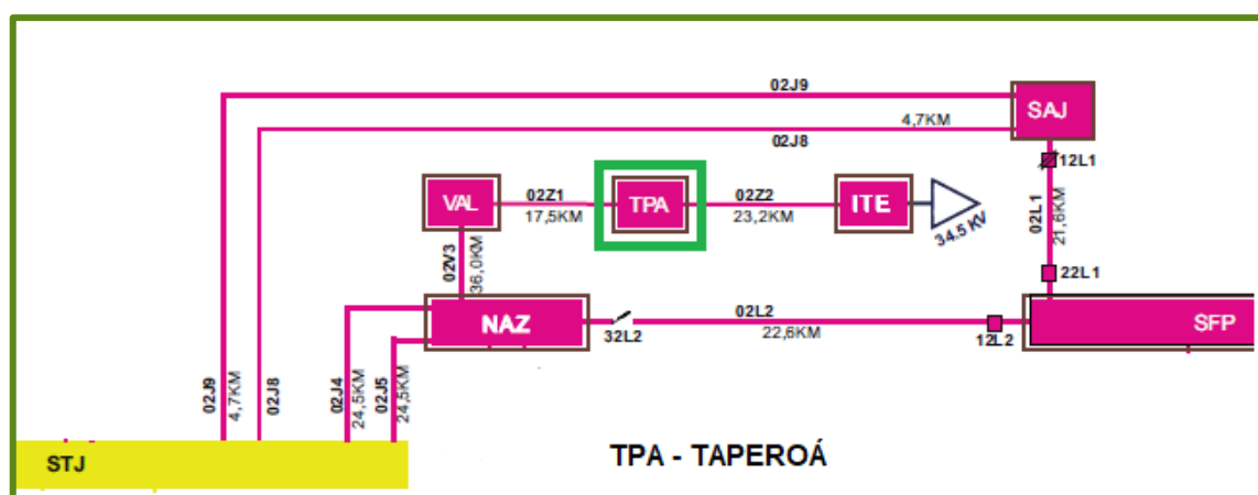
Figura 4 - Diagrama Unifilar Subtransmissão STJ – Santo Antônio de Jesus
