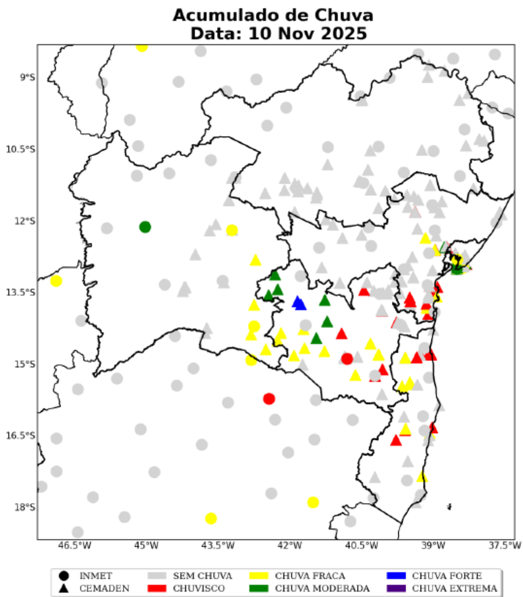
Figura 07 – Mapa de precipitação do dia 10 de novembro de 2025.
