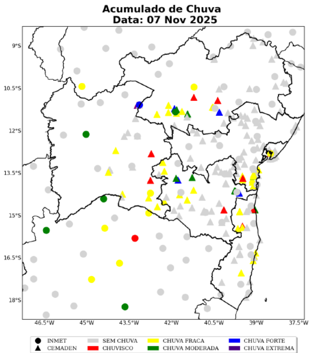
Figura 06 – Mapa de precipitação do dia 07 de novembro de 2025.
