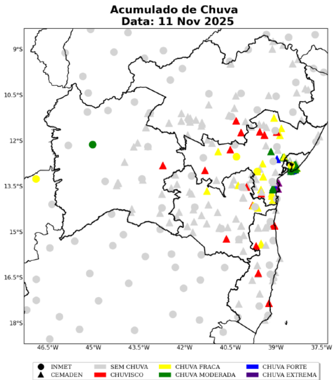
Figura 08 – Mapa de precipitação do dia 11 de novembro de 2025.
