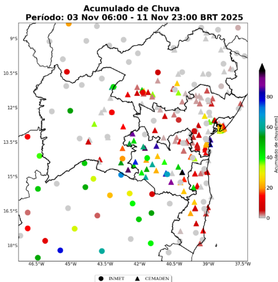
Figura 04– Mapa Acumulado de Chuva na Bahia dos dias 03 a 11 de novembro.
