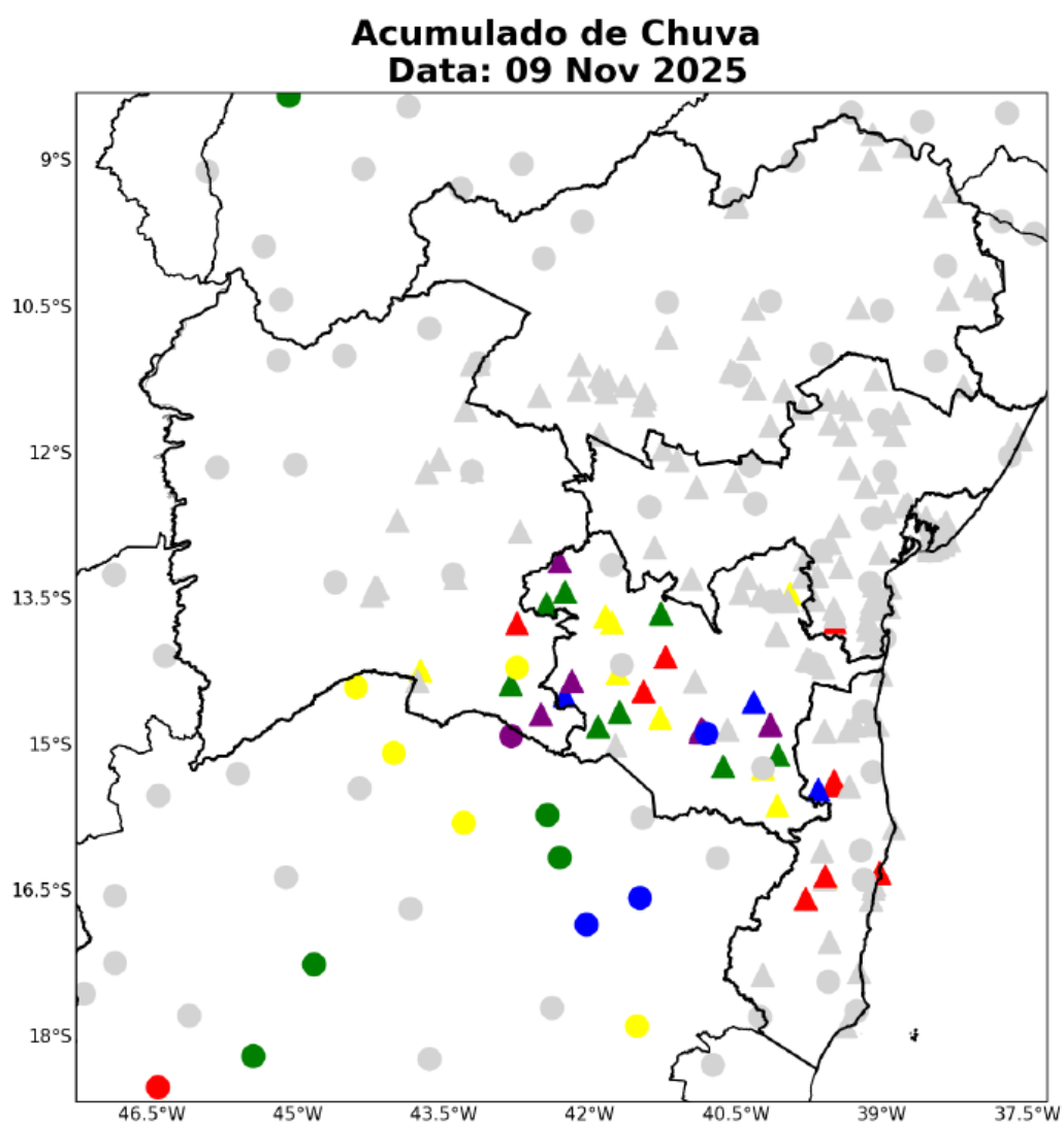
Figura 1 – Mapa do acumulado de chuva sobre o estado da Bahia em 09 de novembro.
