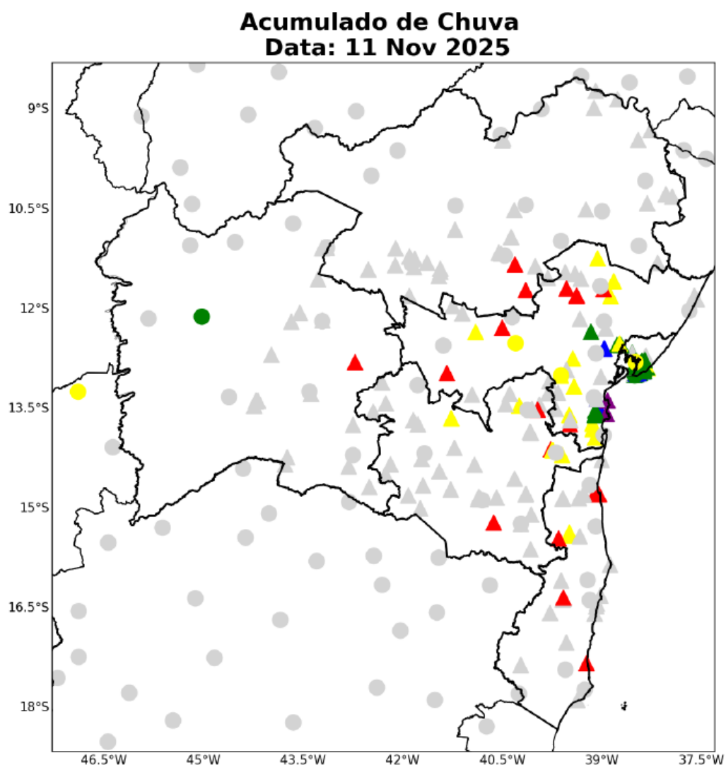
Figura 2 – Mapa do acumulado de chuva sobre o estado da Bahia em 11 de novembro.
