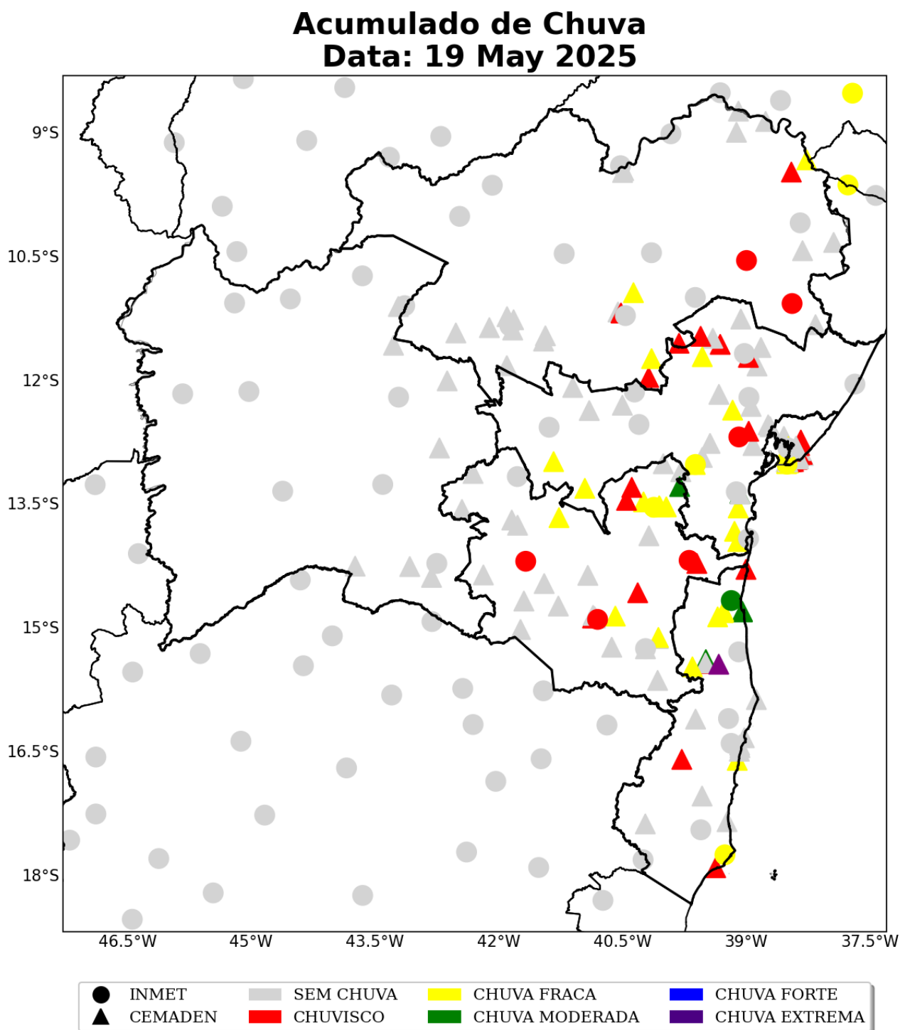
Figura 21: Acumulado diário de precipitação sobre a área de concessão da COELBA para o dia 19 de Maio, baseado nas estações meteorológicas do INMET e CEMADEN.
