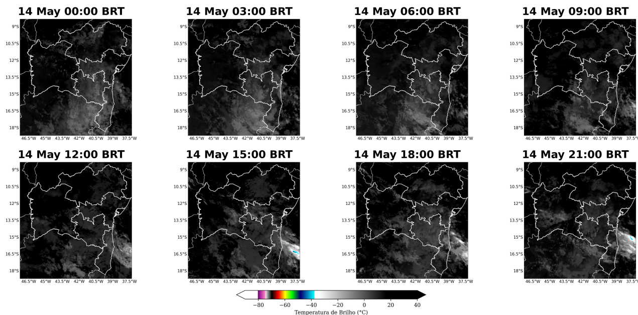
Figura 4: Imagens realçadas do satélite GOES-19 das 00 BRT até 21 BRT (a cada 3 horas) para o dia 14 de Maio.
