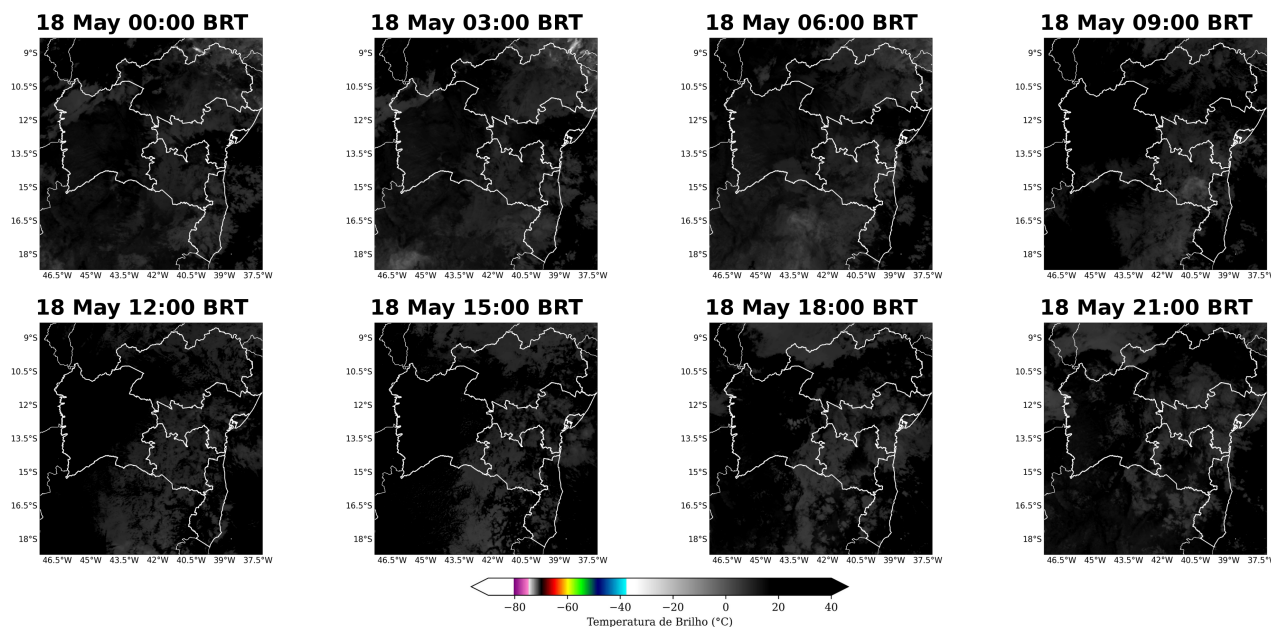
Figura 8: Imagens realçadas do satélite GOES-19 das 00 BRT até 21 BRT (a cada 3 horas) para o dia 18 de Maio.
