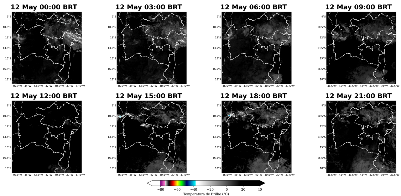
Figura 2: Imagens realçadas do satélite GOES-19 das 00 BRT até 21 BRT (a cada 3 horas) para o dia 12 de Maio.
