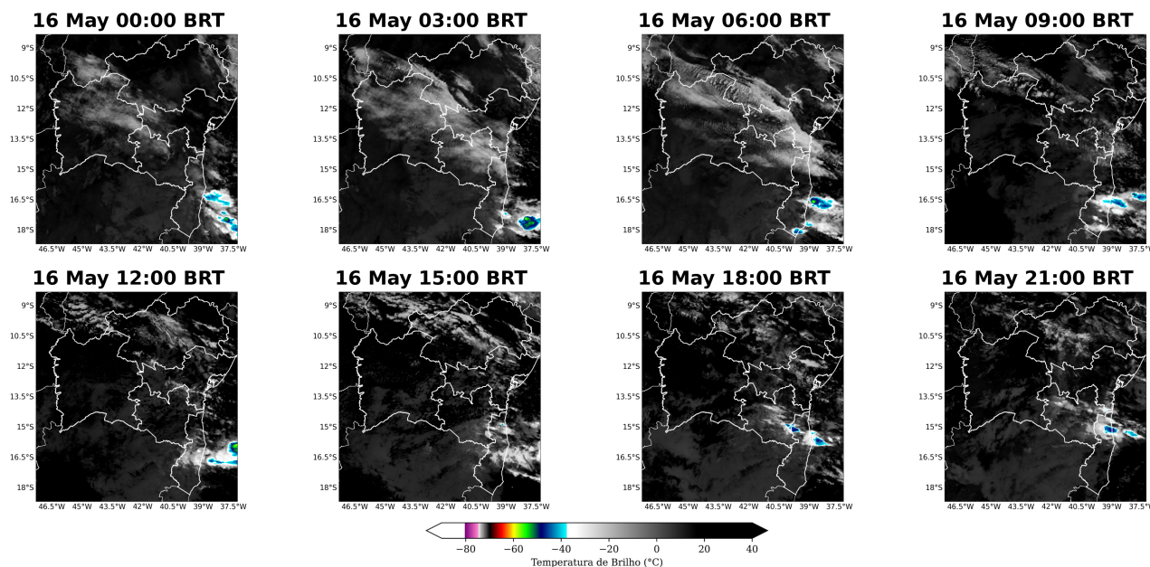
Figura 6: Imagens realçadas do satélite GOES-19 das 00 BRT até 21 BRT (a cada 3 horas) para o dia 16 de Maio.
