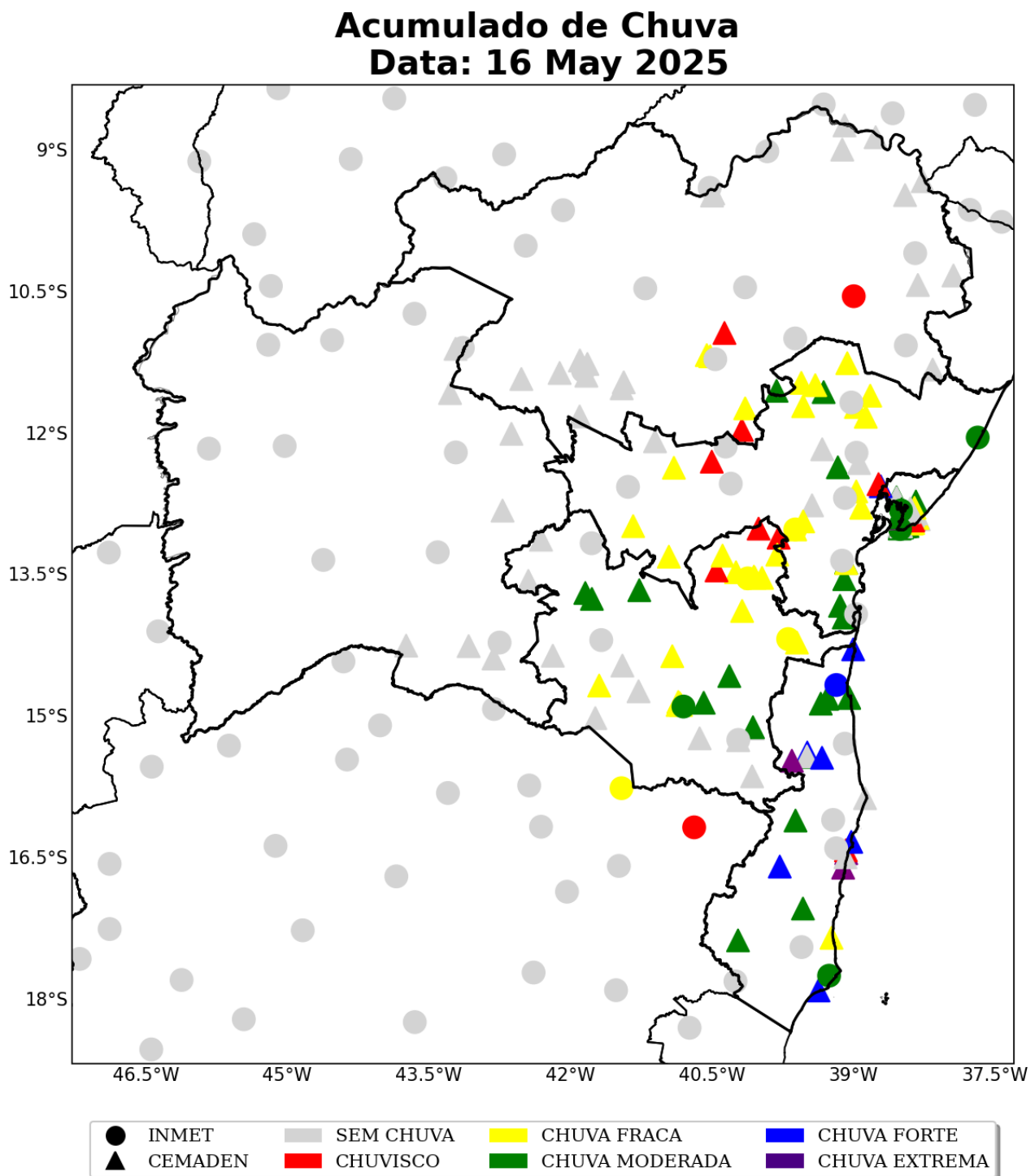
Figura 18: Acumulado diário de precipitação sobre a área de concessão da COELBA para o dia 16 de Maio, baseado nas estações meteorológicas do INMET e CEMADEN.
