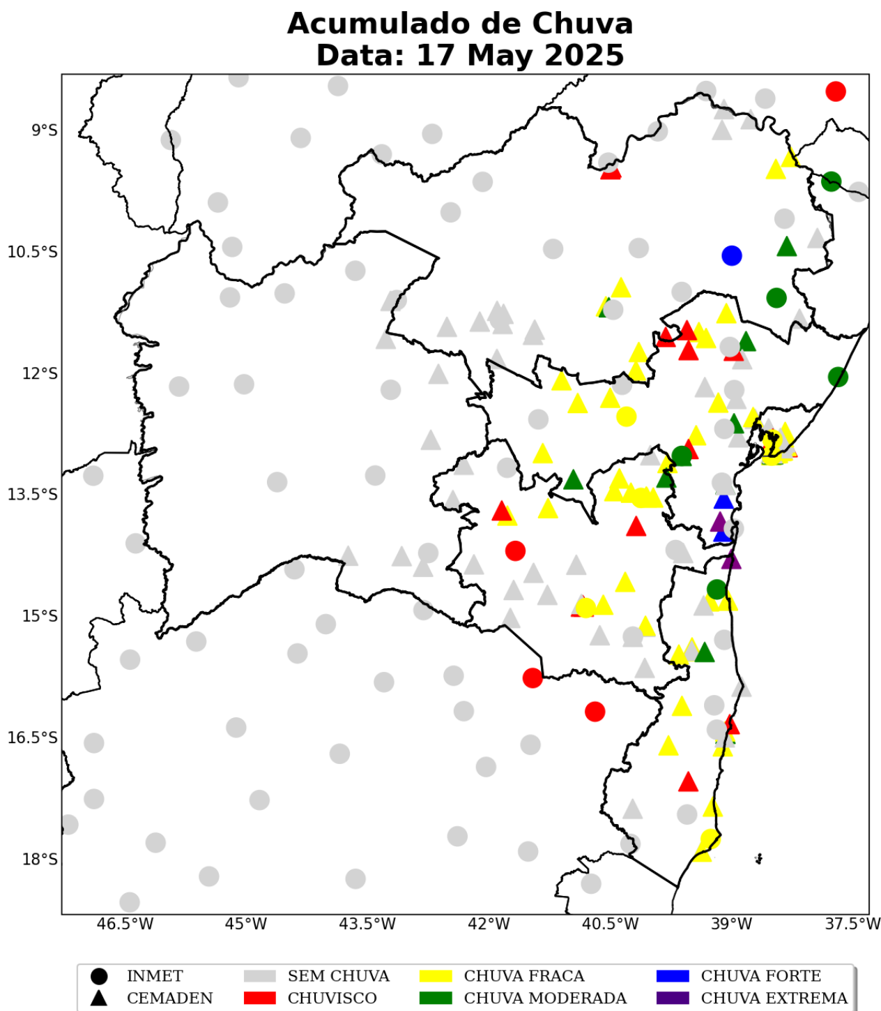
Figura 19: Acumulado diário de precipitação sobre a área de concessão da COELBA para o dia 17 de Maio, baseado nas estações meteorológicas do INMET e CEMADEN.
