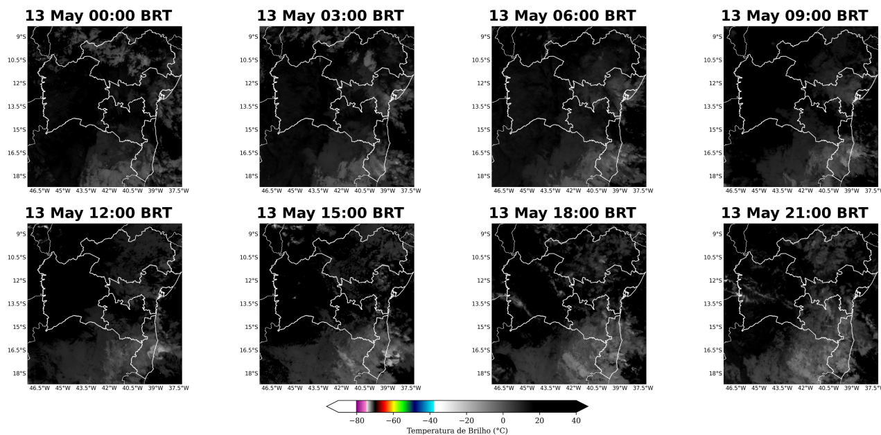
Figura 3: Imagens realçadas do satélite GOES-19 das 00 BRT até 21 BRT (a cada 3 horas) para o dia 13 de Maio.
