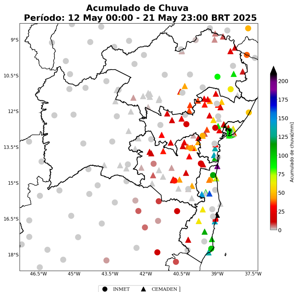
Figura 24: Acumulado de precipitação sobre o estado da Bahia para o período do evento (dias 12 a 21 de Maio de 2025), baseado nas estações meteorológicas do INMET e CEMADEN.
