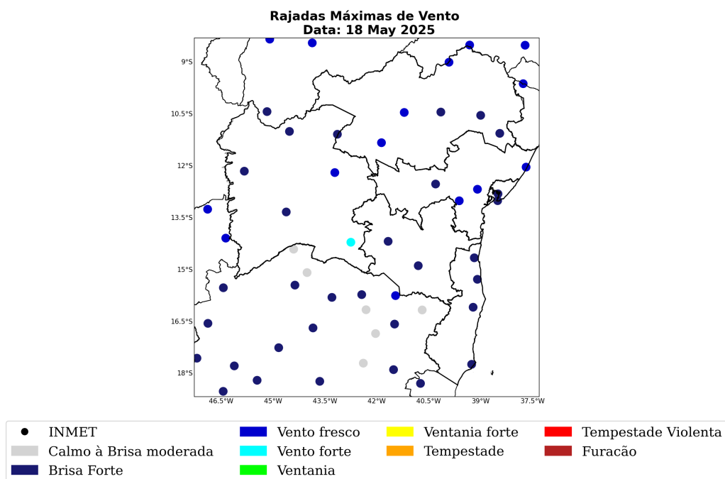
Figura 31: Máxima rajada de vento diária sobre a área de concessão da COELBA para o dia 18 de Maio, baseado nas estações meteorológicas do INMET.
