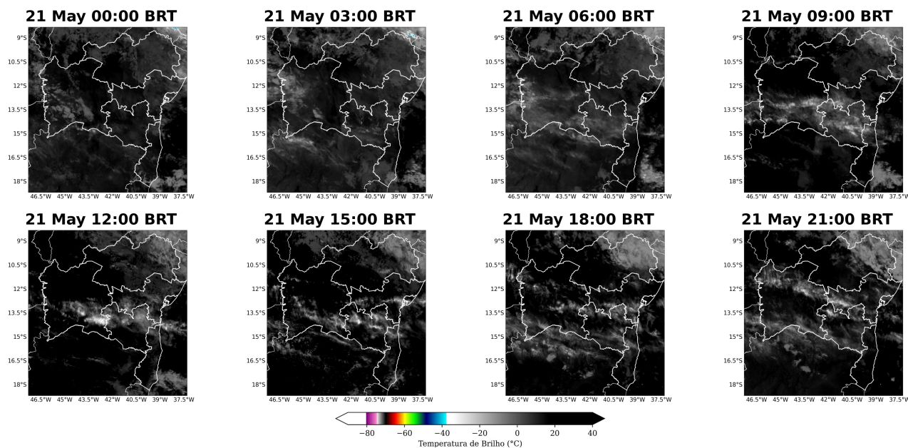
Figura 11: Imagens realçadas do satélite GOES-19 das 00 BRT até 21 BRT (a cada 3 horas) para o dia 21 de Maio.
