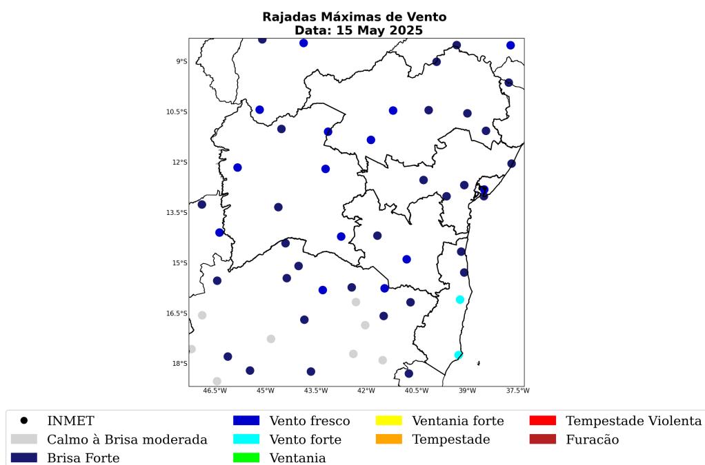
Figura 28: Máxima rajada de vento diária sobre a área de concessão da COELBA para o dia 15 de Maio, baseado nas estações meteorológicas do INMET.
