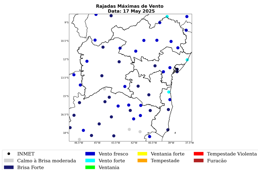
Figura 30: Máxima rajada de vento diária sobre a área de concessão da COELBA para o dia 17 de Maio, baseado nas estações meteorológicas do INMET.
