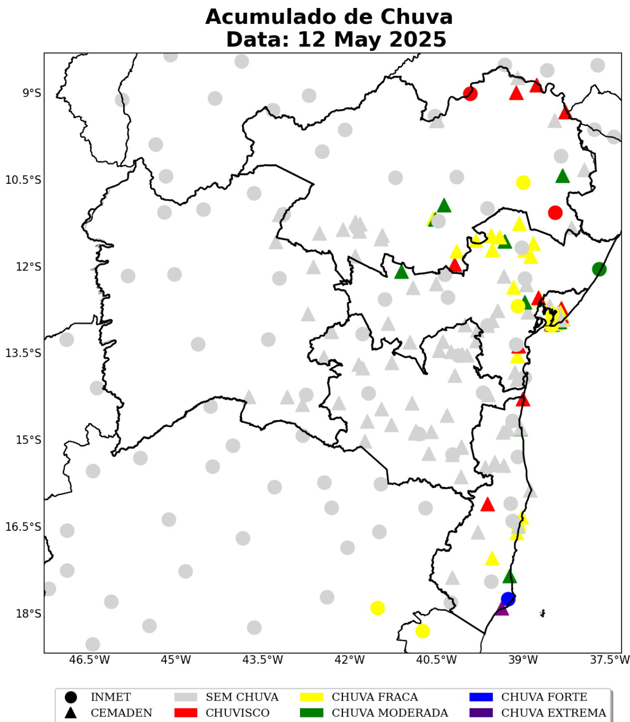
Figura 14: Acumulado diário de precipitação sobre a área de concessão da COELBA para o dia 12 de Maio, baseado nas estações meteorológicas do INMET e CEMADEN.
