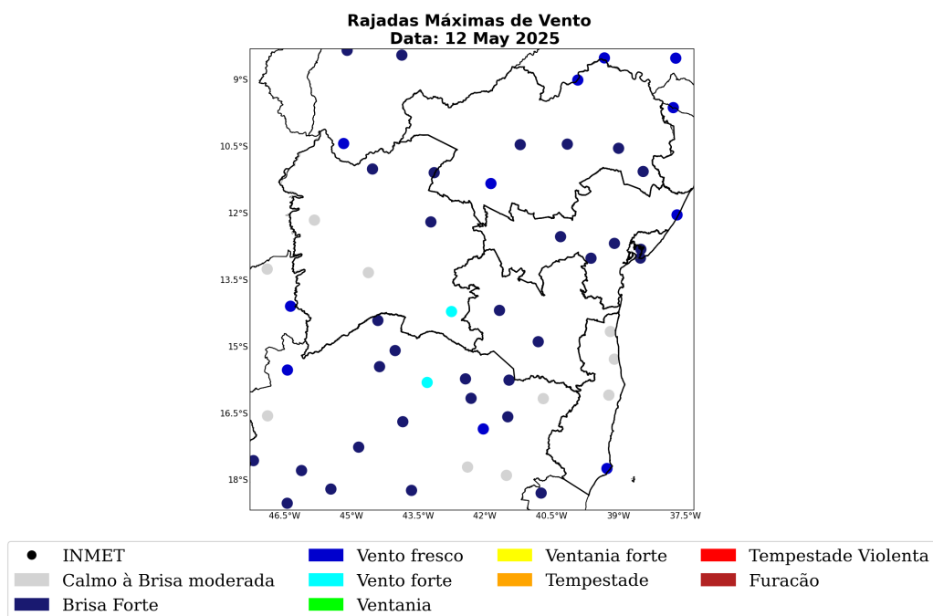
Figura 25: Máxima rajada de vento diária sobre a área de concessão da COELBA para o dia 12 de Maio, baseado nas estações meteorológicas do INMET.
