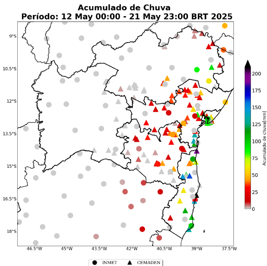
Figura 07 – Mapa Acumulado de Chuva na Bahia do dia 12 a 21 de maio.
