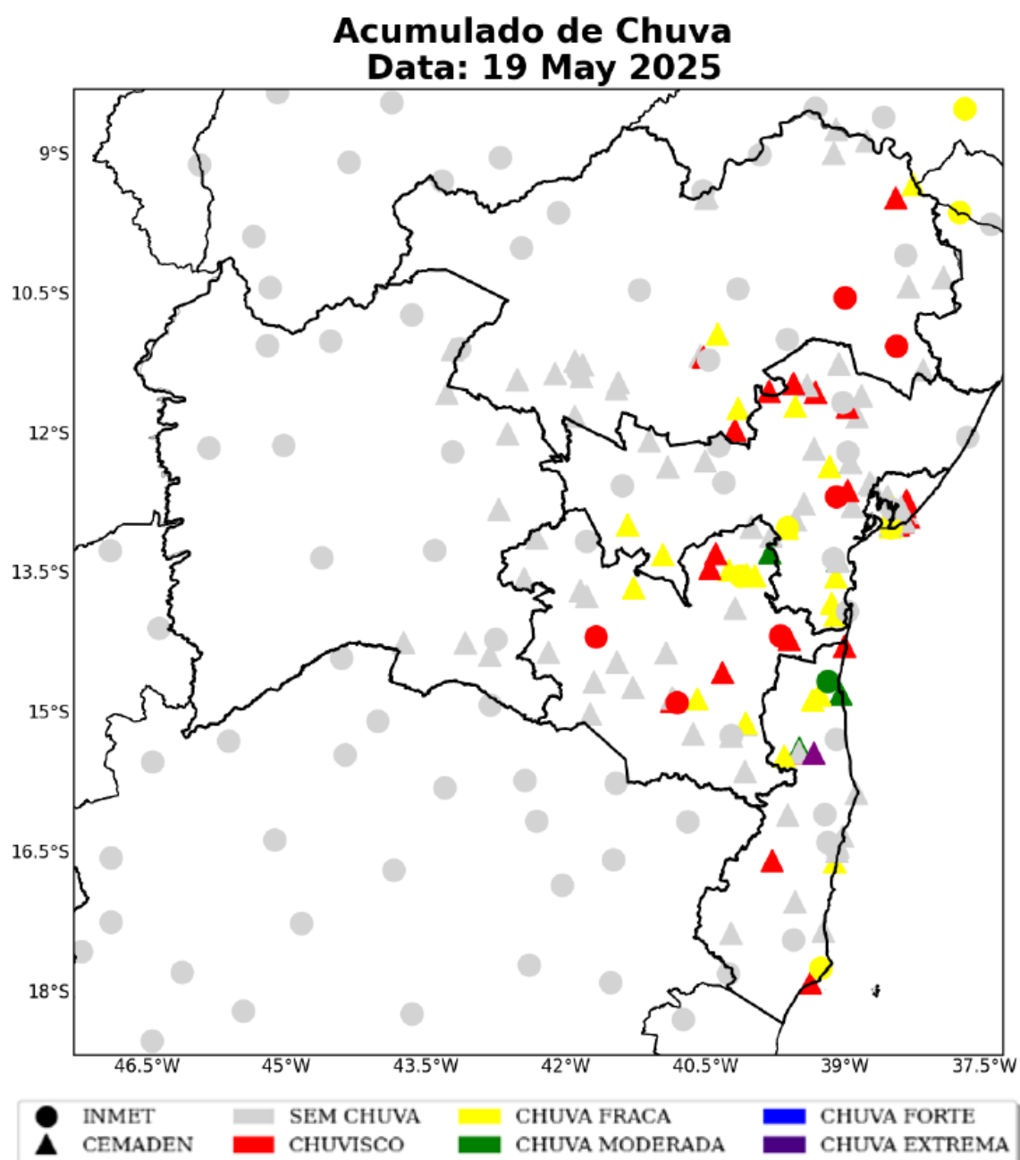
Figura 6 – Mapa de precipitação do dia 19 de maio de 2025.
