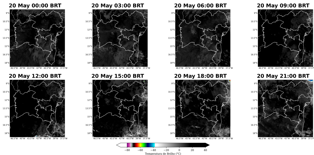
Figura 10: Imagens realçadas do satélite GOES-19 das 00 BRT até 21 BRT (a cada 3 horas) para o dia 20 de Maio.
