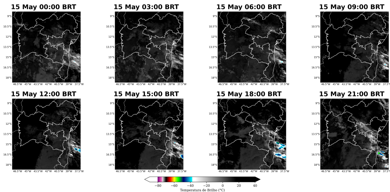
Figura 5: Imagens realçadas do satélite GOES-19 das 00 BRT até 21 BRT (a cada 3 horas) para o dia 15 de Maio.
