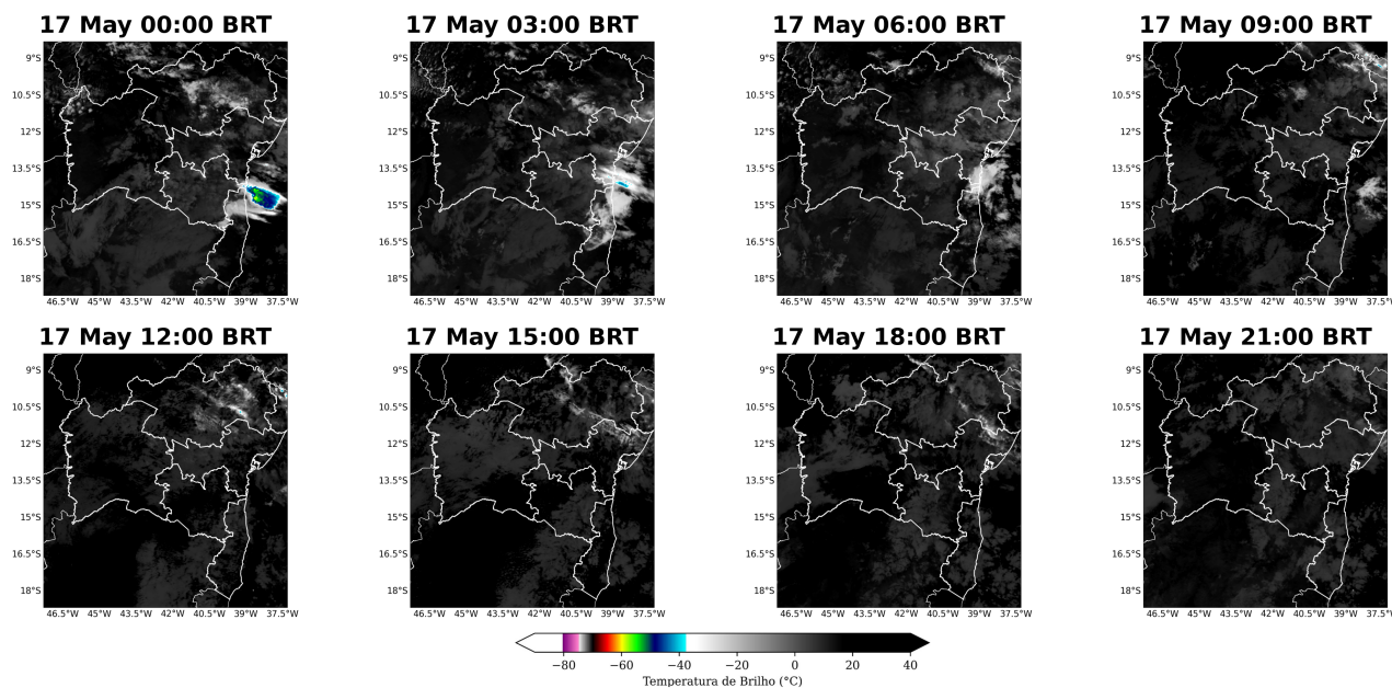
Figura 7: Imagens realçadas do satélite GOES-19 das 00 BRT até 21 BRT (a cada 3 horas) para o dia 17 de Maio.
