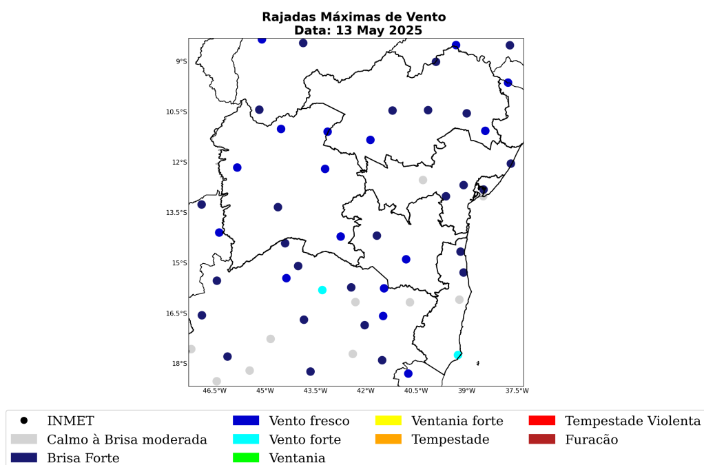
Figura 26: Máxima rajada de vento diária sobre a área de concessão da COELBA para o dia 13 de Maio, baseado nas estações meteorológicas do INMET.
