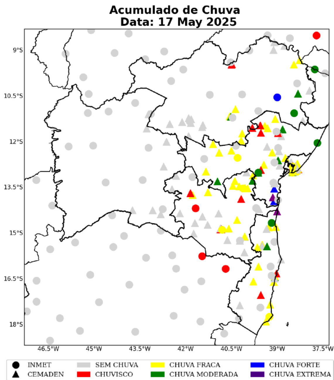
Figura 5 – Mapa de precipitação do dia 17 de maio de 2025.
