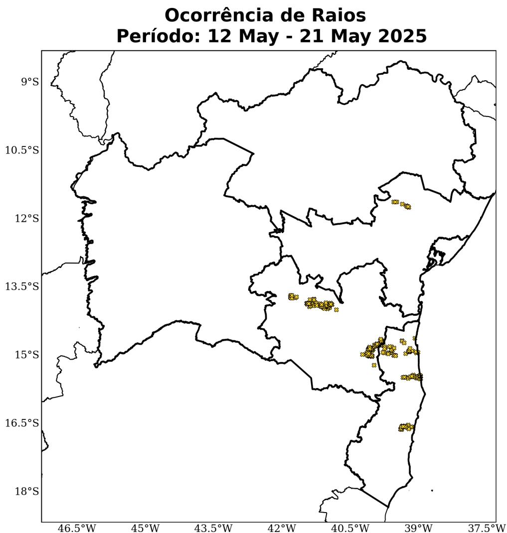
Figura 13: Ocorrências de descargas atmosféricas nuvem-solo detectadas pelo sistema Earth Networks para o período de 12 a 21 de Maio de 2025 sobre a área de concessão da COELBA.
