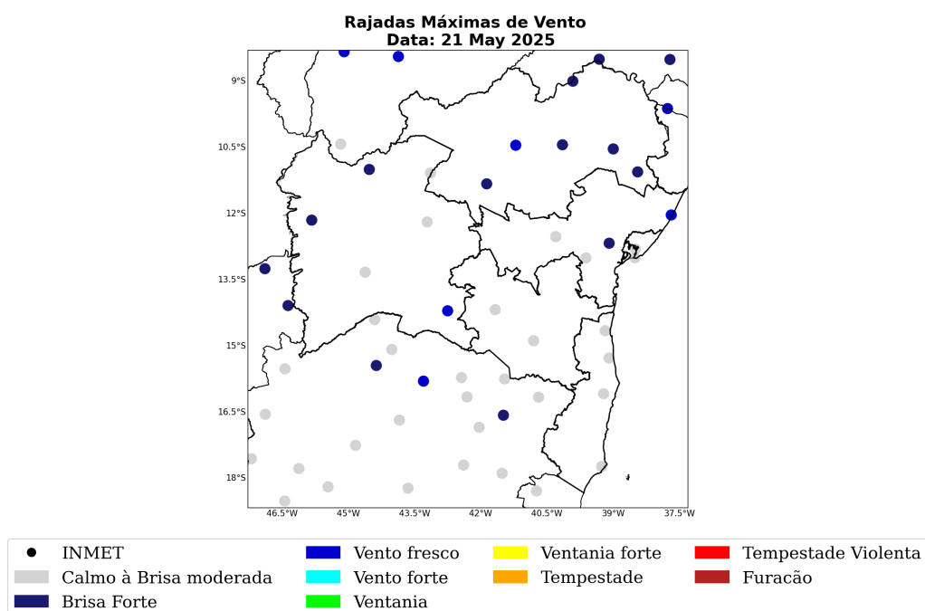
Figura 34: Máxima rajada de vento diária sobre a área de concessão da COELBA para o dia 21 de Maio, baseado nas estações meteorológicas do INMET.
