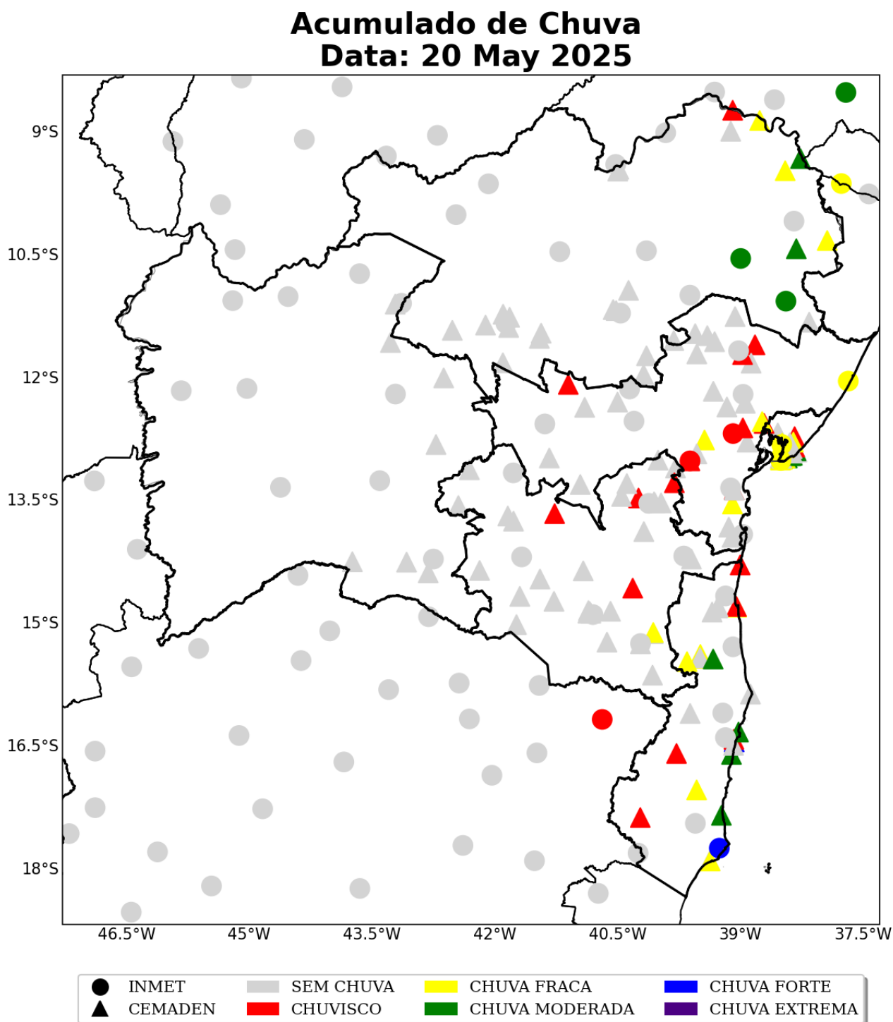
Figura 22: Acumulado diário de precipitação sobre a área de concessão da COELBA para o dia 20 de Maio, baseado nas estações meteorológicas do INMET e CEMADEN.
