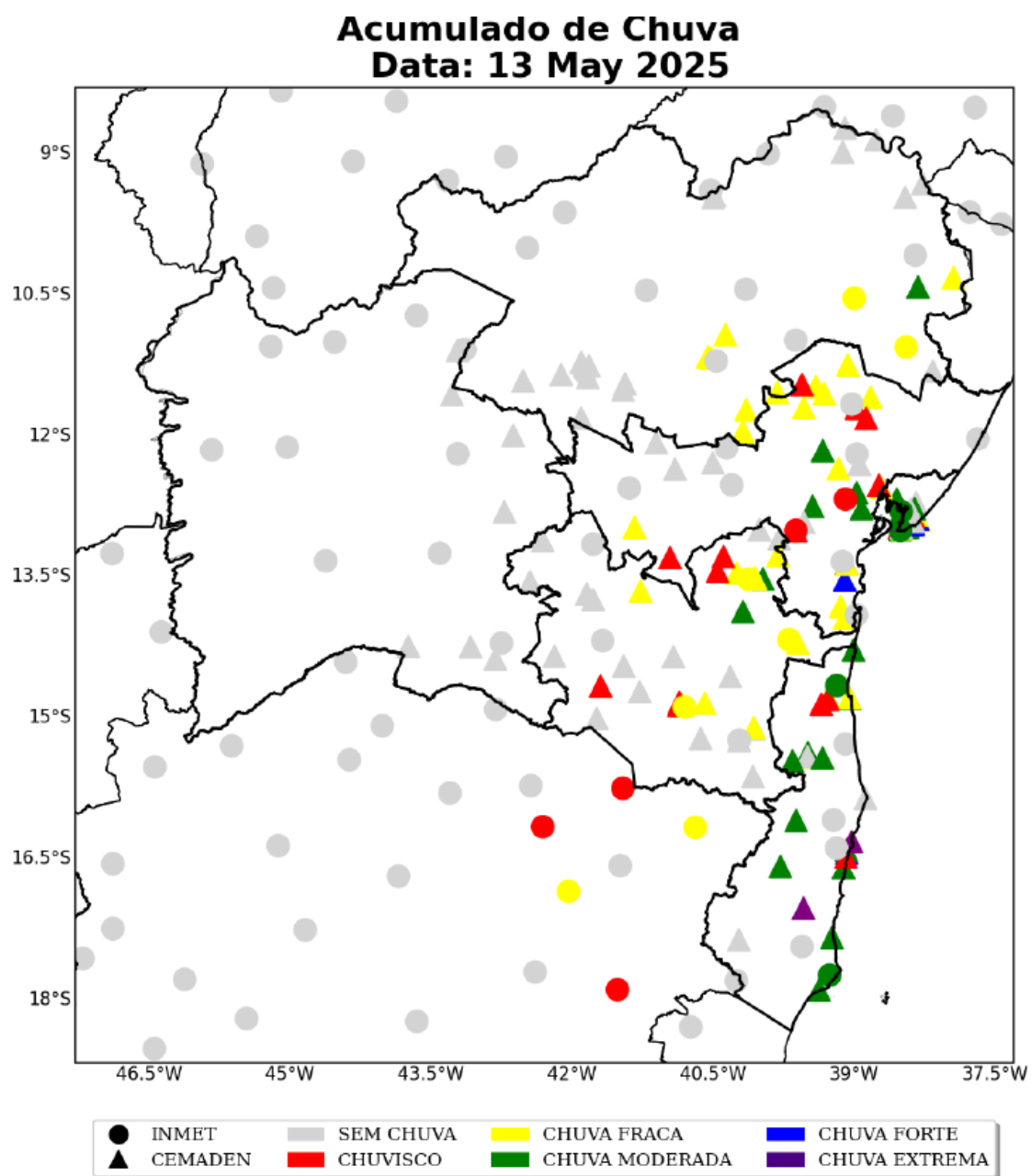
Figura 1 – Mapa do acumulado de chuva sobre o estado da Bahia em 13 de maio.
