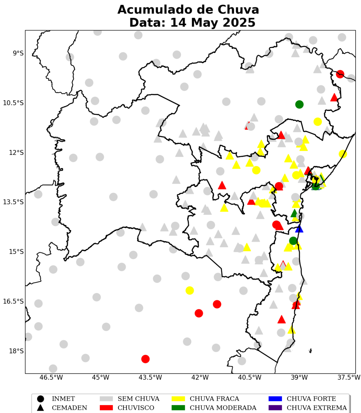
Figura 16: Acumulado diário de precipitação sobre a área de concessão da COELBA para o dia 14 de Maio, baseado nas estações meteorológicas do INMET e CEMADEN.
