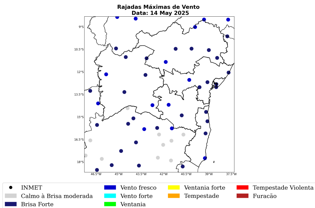
Figura 27: Máxima rajada de vento diária sobre a área de concessão da COELBA para o dia 14 de Maio, baseado nas estações meteorológicas do INMET.
