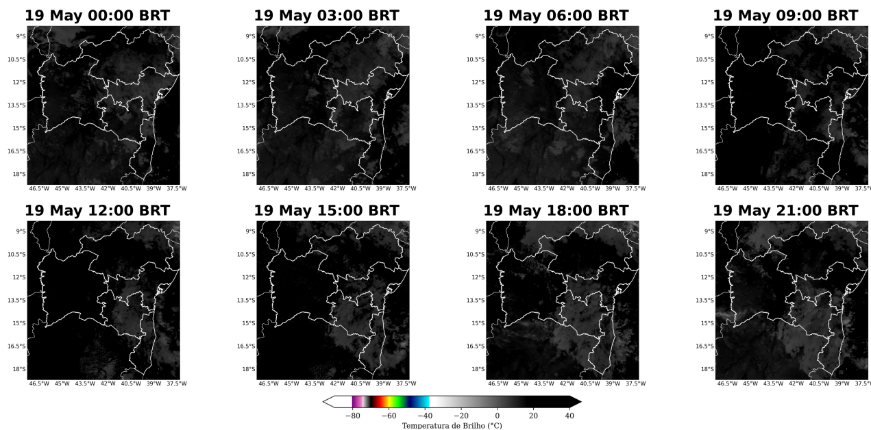
Figura 9: Imagens realçadas do satélite GOES-19 das 00 BRT até 21 BRT (a cada 3 horas) para o dia 19 de Maio.
