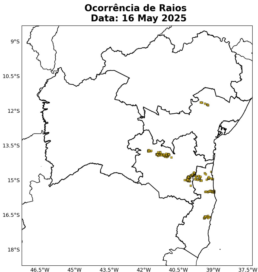
Figura 12: Ocorrências de descargas atmosféricas nuvem-solo detectadas pelo sistema Earth Networks para o dia 16 de Maio sobre a área de concessão da COELBA.
