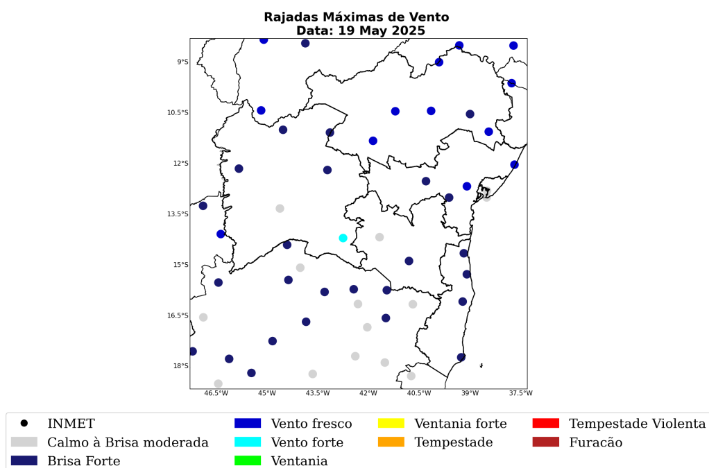
Figura 32: Máxima rajada de vento diária sobre a área de concessão da COELBA para o dia 19 de Maio, baseado nas estações meteorológicas do INMET.
