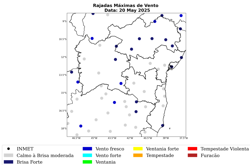
Figura 33: Máxima rajada de vento diária sobre a área de concessão da COELBA para o dia 20 de Maio, baseado nas estações meteorológicas do INMET.
