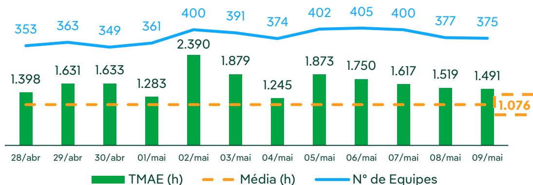
Gráfico 3 – Tempo médio de atendimento emergência e n° de equipes por dia de 28/04 a 09/05 de 2025.
