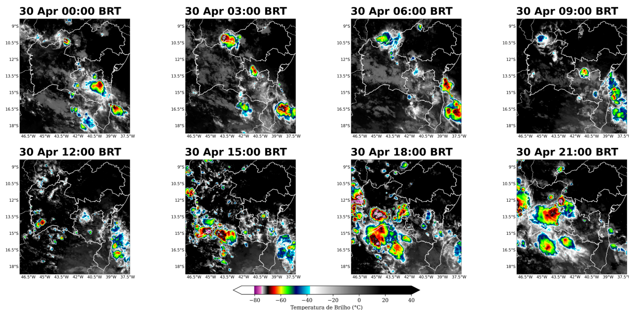
Figura 4: Imagens realçadas do satélite GOES-19 das 00 BRT até 21 BRT (a cada 3 horas) para o dia 30 de Abril.
