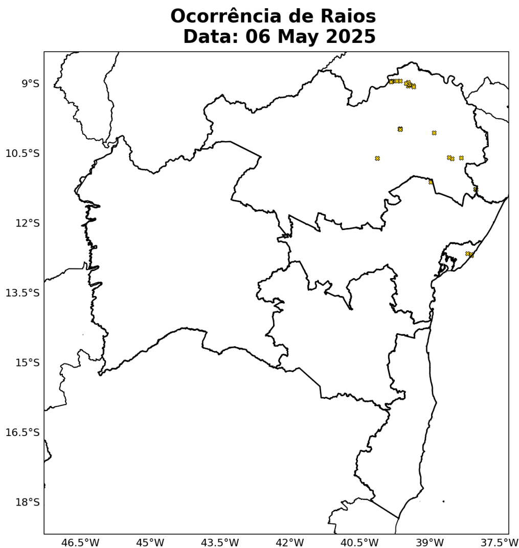
Figura 20: Ocorrências de descargas atmosféricas nuvem-solo detectadas pelo sistema Earth Networks para o dia 06 de Maio sobre a área de concessão da COELBA.
