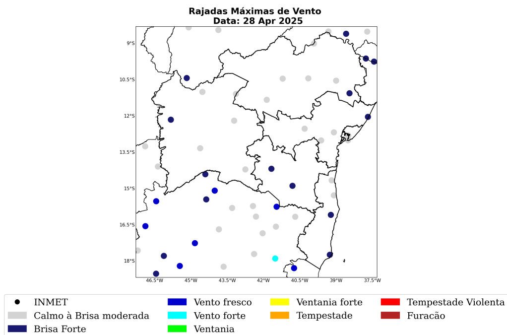
Figura 38: Máxima rajada de vento diária sobre a área de concessão da COELBA para o dia 28 de Abril, baseado nas estações meteorológicas do INMET.
