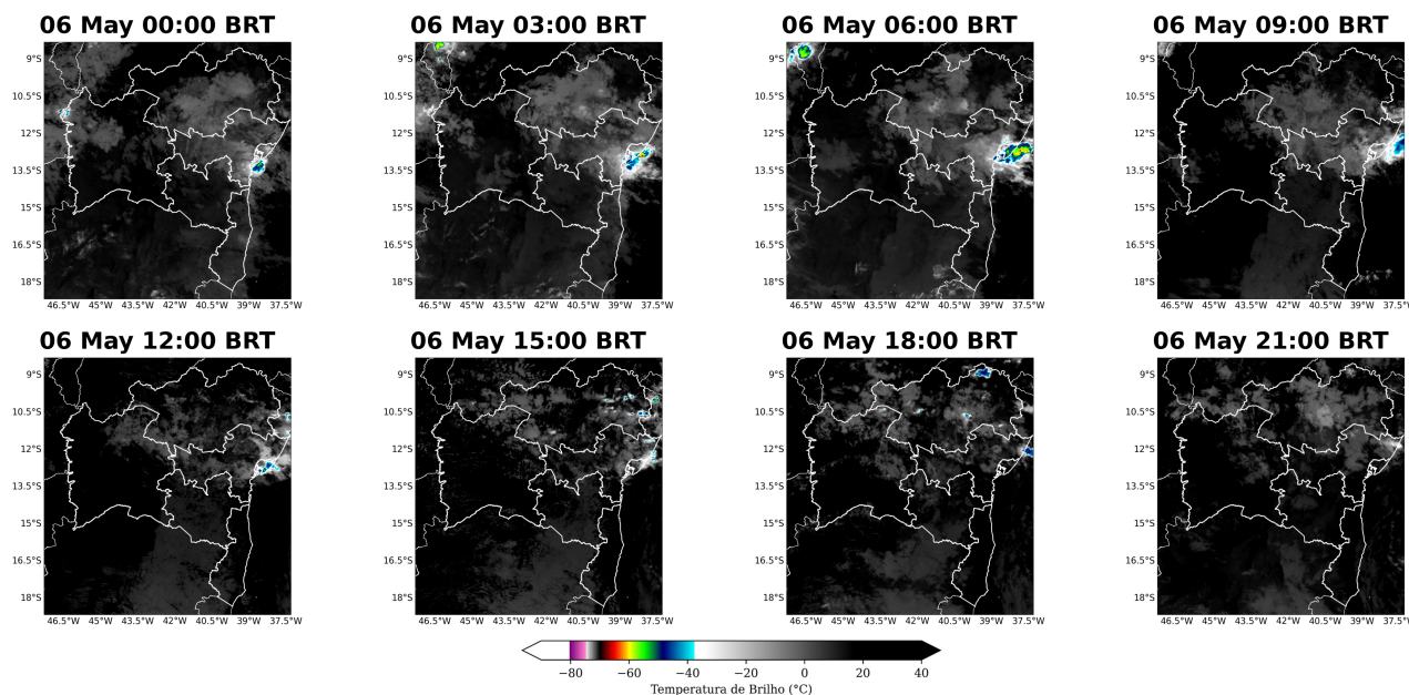
Figura 10: Imagens realçadas do satélite GOES-19 das 00 BRT até 21 BRT (a cada 3 horas) para o dia 06 de Maio.
