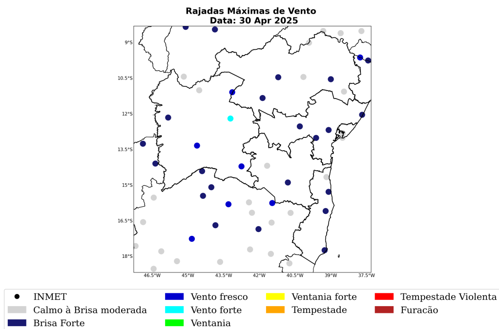
Figura 40: Máxima rajada de vento diária sobre a área de concessão da COELBA para o dia 30 de Abril, baseado nas estações meteorológicas do INMET.
