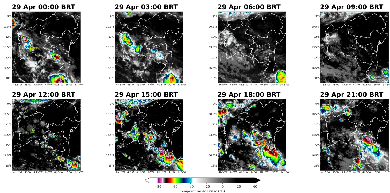
Figura 3: Imagens realçadas do satélite GOES-19 das 00 BRT até 21 BRT (a cada 3 horas) para o dia 29 de Abril.
