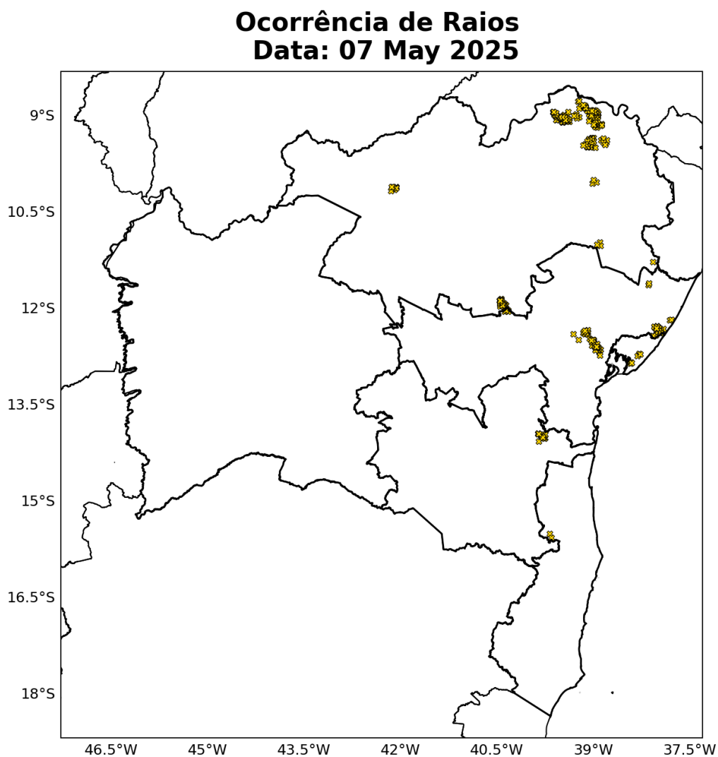
Figura 21: Ocorrências de descargas atmosféricas nuvem-solo detectadas pelo sistema Earth Networks para o dia 07 de Maio sobre a área de concessão da COELBA.
