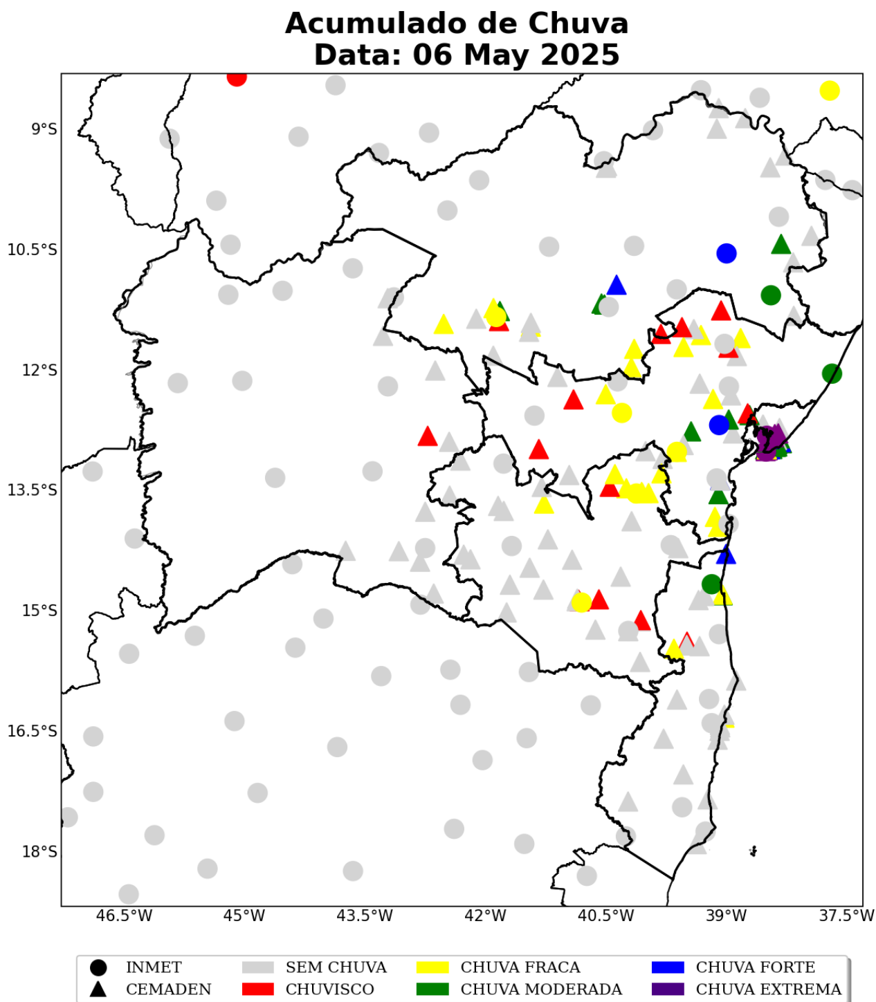
Figura 33: Acumulado diário de precipitação sobre a área de concessão da COELBA para o dia 06 de Maio, baseado nas estações meteorológicas do INMET e CEMADEN.
