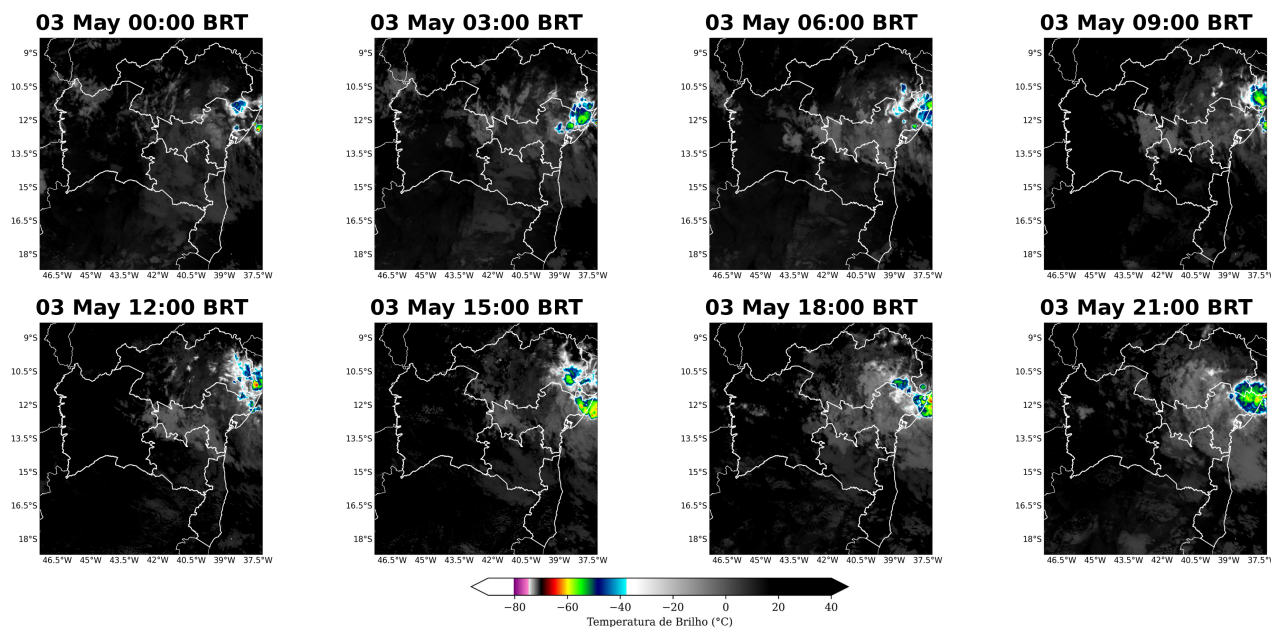
Figura 7: Imagens realçadas do satélite GOES-19 das 00 BRT até 21 BRT (a cada 3 horas) para o dia 03 de Maio.
