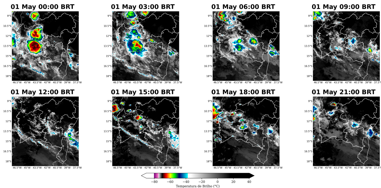
Figura 5: Imagens realçadas do satélite GOES-19 das 00 BRT até 21 BRT (a cada 3 horas) para o dia 01 de Maio.
