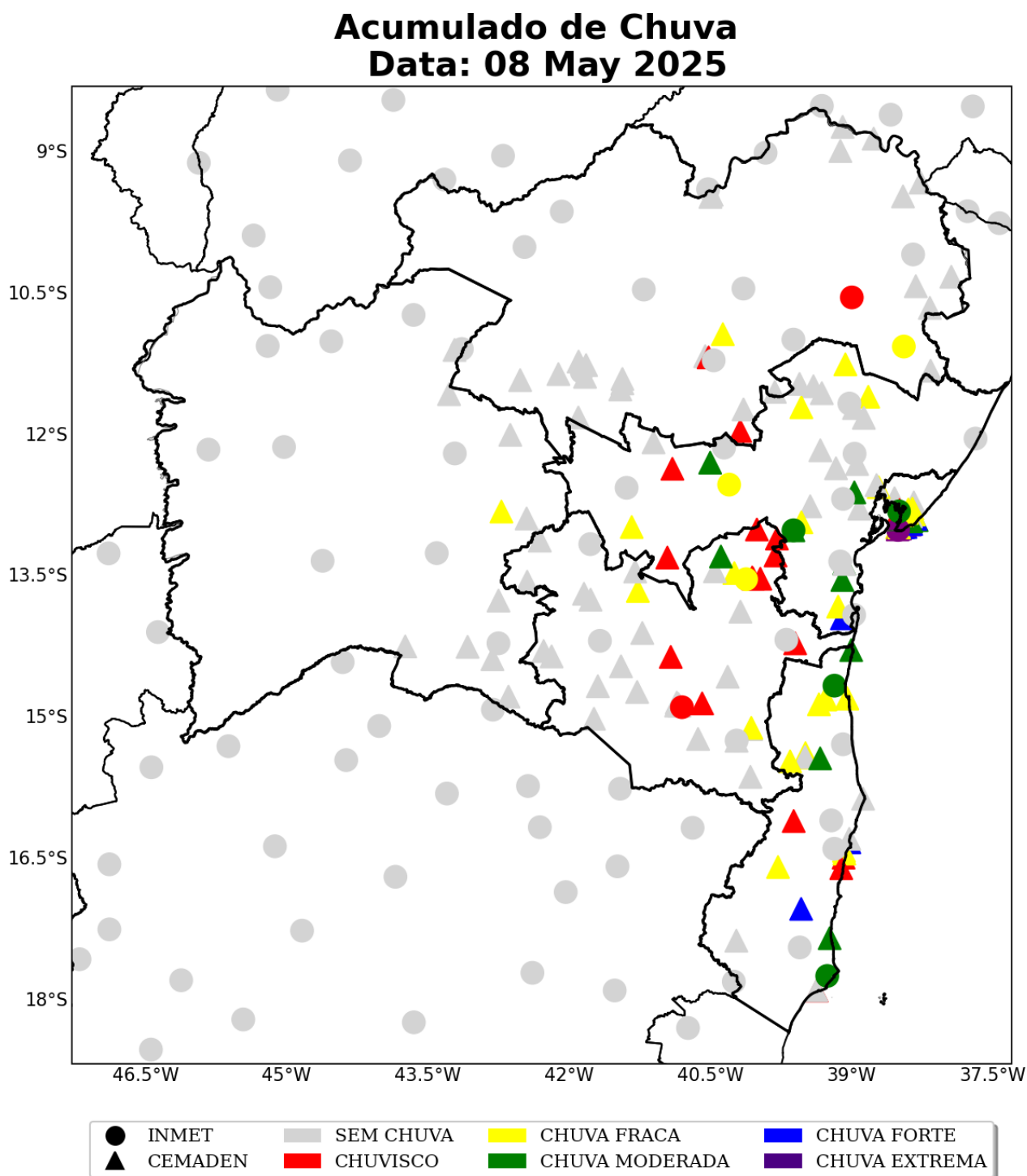
Figura 35: Acumulado diário de precipitação sobre a área de concessão da COELBA para o dia 08 de Maio, baseado nas estações meteorológicas do INMET e CEMADEN.
