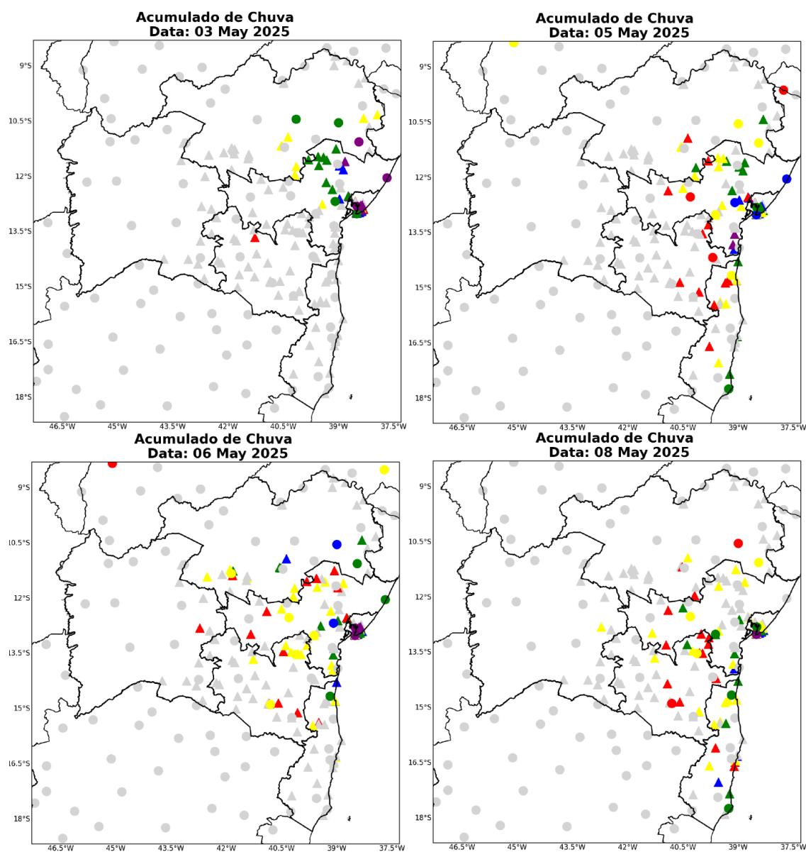
Figura 7 – Mapa de precipitação dos dias 03, 05, 06 e 08 de maio de 2025.
