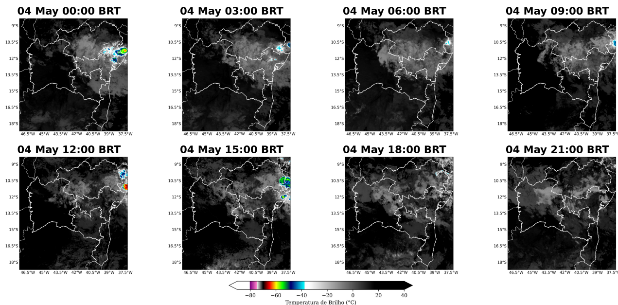
Figura 8: Imagens realçadas do satélite GOES-19 das 00 BRT até 21 BRT (a cada 3 horas) para o dia 04 de Maio.
