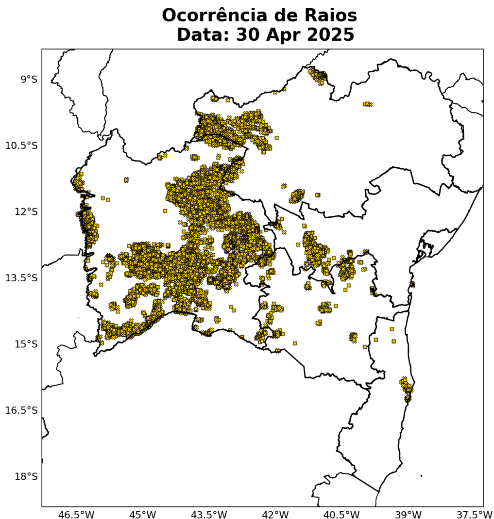
Figura 16: Ocorrências de descargas atmosféricas nuvem-solo detectadas pelo sistema Earth Networks para o dia 30 de Abril sobre a área de concessão da COELBA.
