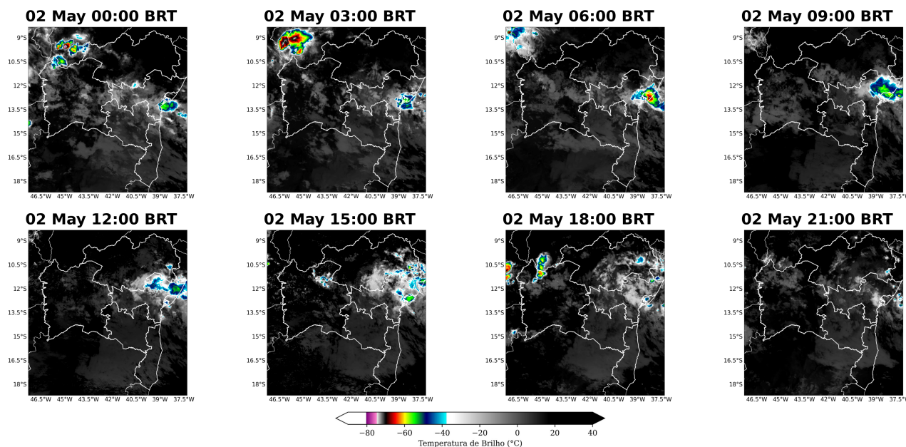
Figura 6: Imagens realçadas do satélite GOES-19 das 00 BRT até 21 BRT (a cada 3 horas) para o dia 02 de Maio.
