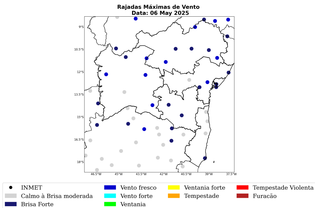
Figura 46: Máxima rajada de vento diária sobre a área de concessão da COELBA para o dia 06 de Maio, baseado nas estações meteorológicas do INMET.
