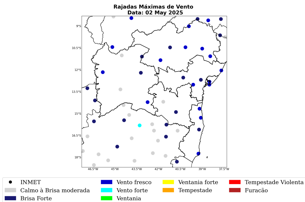
Figura 42: Máxima rajada de vento diária sobre a área de concessão da COELBA para o dia 02 de Maio, baseado nas estações meteorológicas do INMET.
