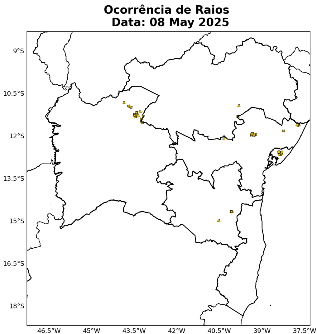
Figura 22: Ocorrências de descargas atmosféricas nuvem-solo detectadas pelo sistema Earth Networks para o dia 08 de Maio sobre a área de concessão da COELBA.
