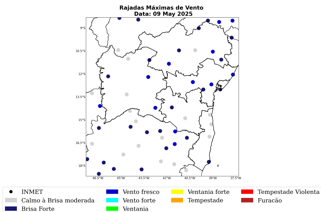
Figura 49: Máxima rajada de vento diária sobre a área de concessão da COELBA para o dia 09 de Maio, baseado nas estações meteorológicas do INMET.
