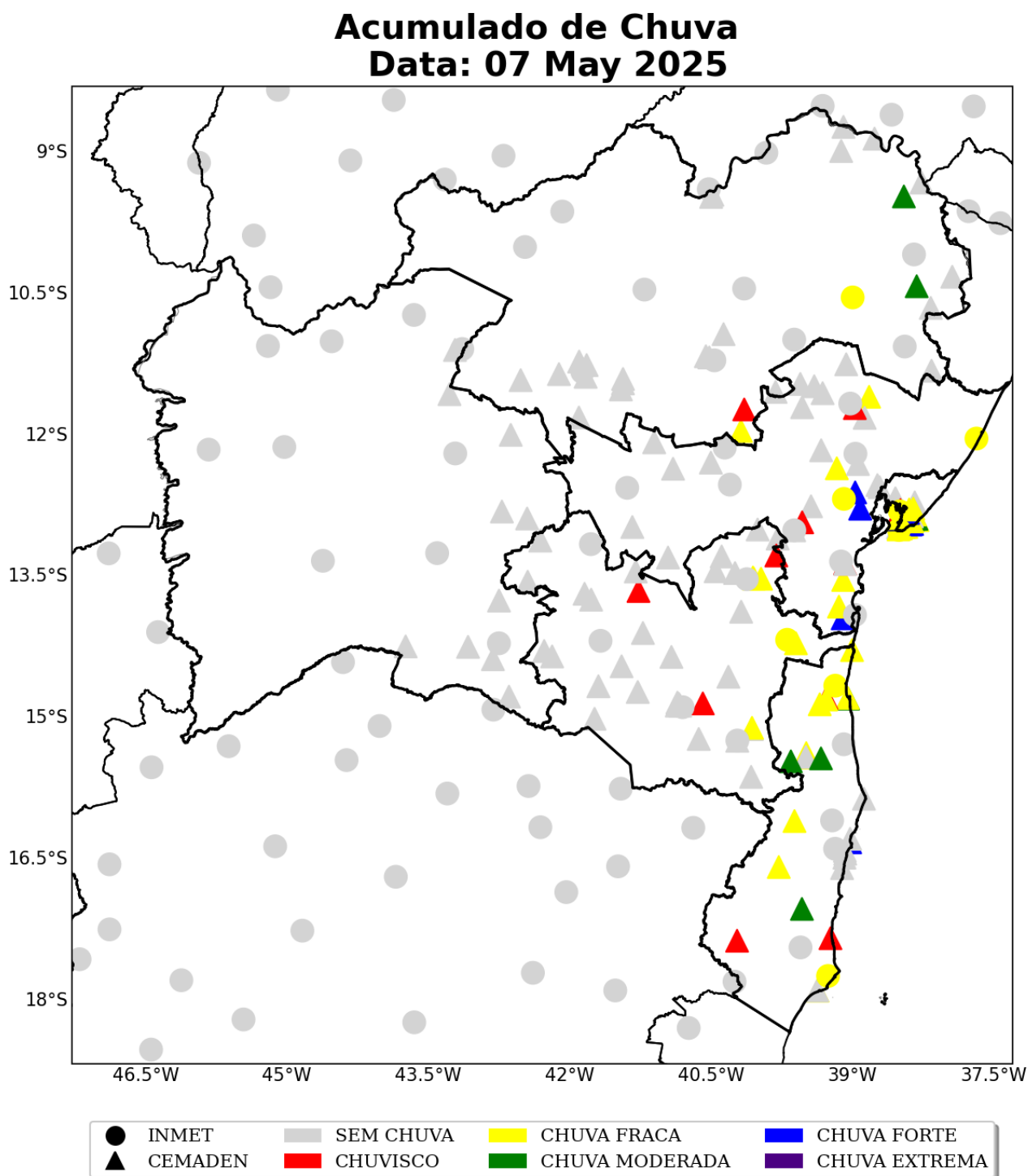
Figura 34: Acumulado diário de precipitação sobre a área de concessão da COELBA para o dia 07 de Maio, baseado nas estações meteorológicas do INMET e CEMADEN.
