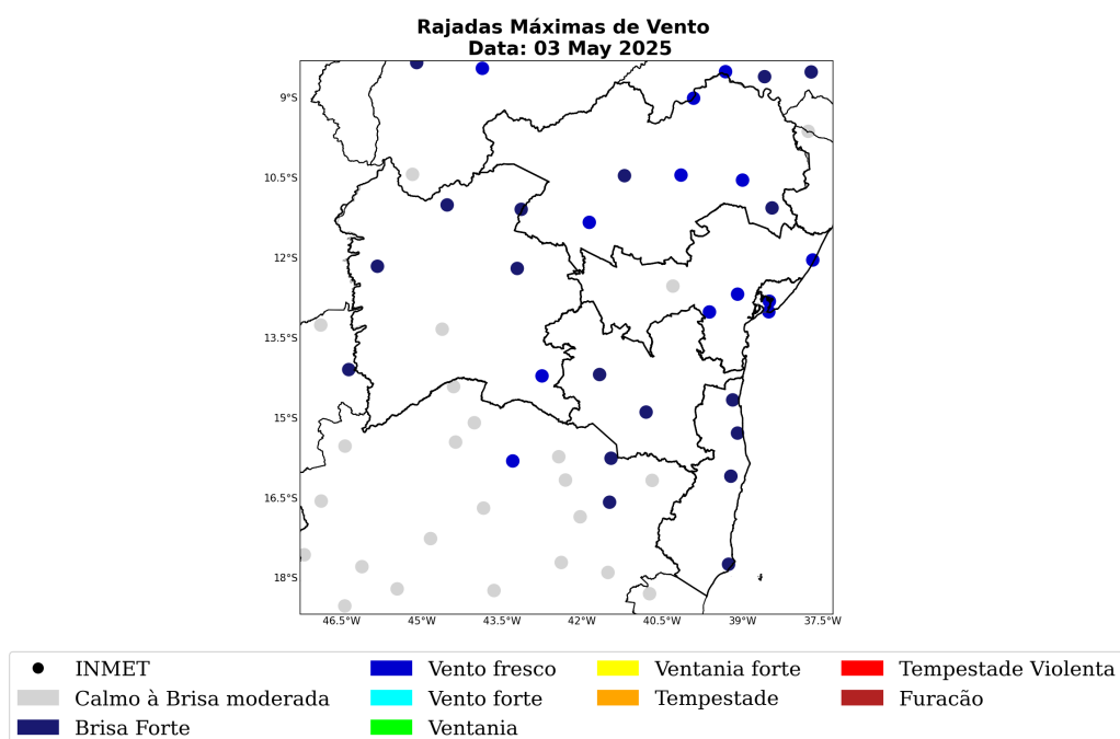
Figura 43: Máxima rajada de vento diária sobre a área de concessão da COELBA para o dia 03 de Maio, baseado nas estações meteorológicas do INMET.
