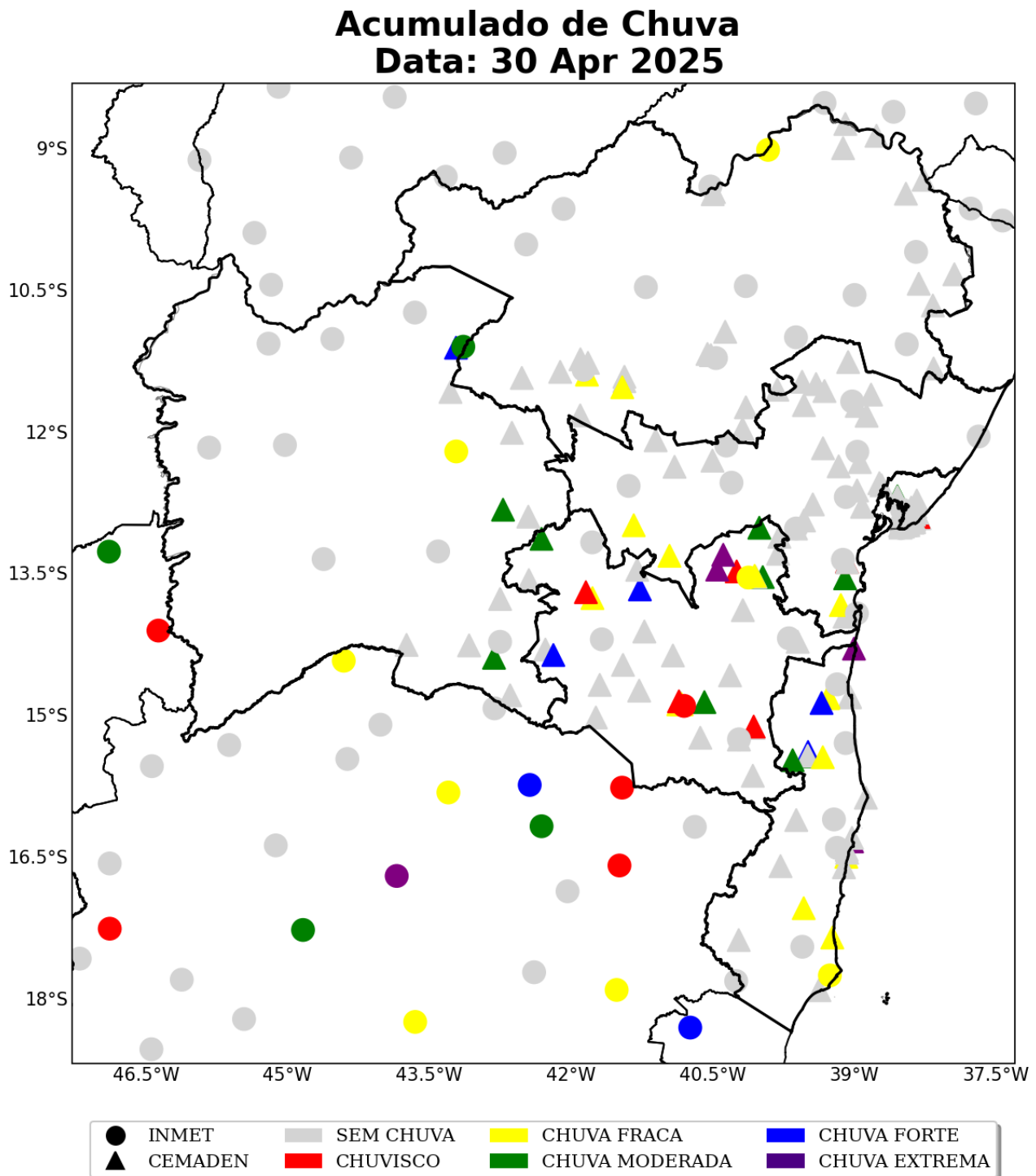
Figura 27: Acumulado diário de precipitação sobre a área de concessão da COELBA para o dia 30 de Abril, baseado nas estações meteorológicas do INMET e CEMADEN.
