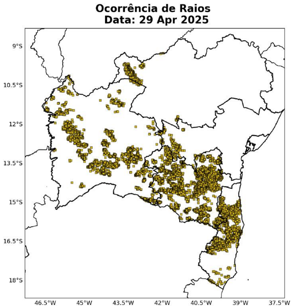
Figura 3 – Mapa de descargas atmosféricas sobre o estado da Bahia no dia 29 de abril.
