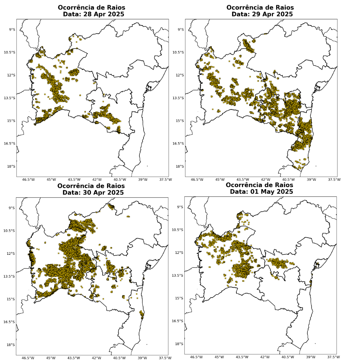
Figura 13 – Mapas de ocorrências de descargas atmosféricas do dia 28 de abril a 01 de maio de 2025
