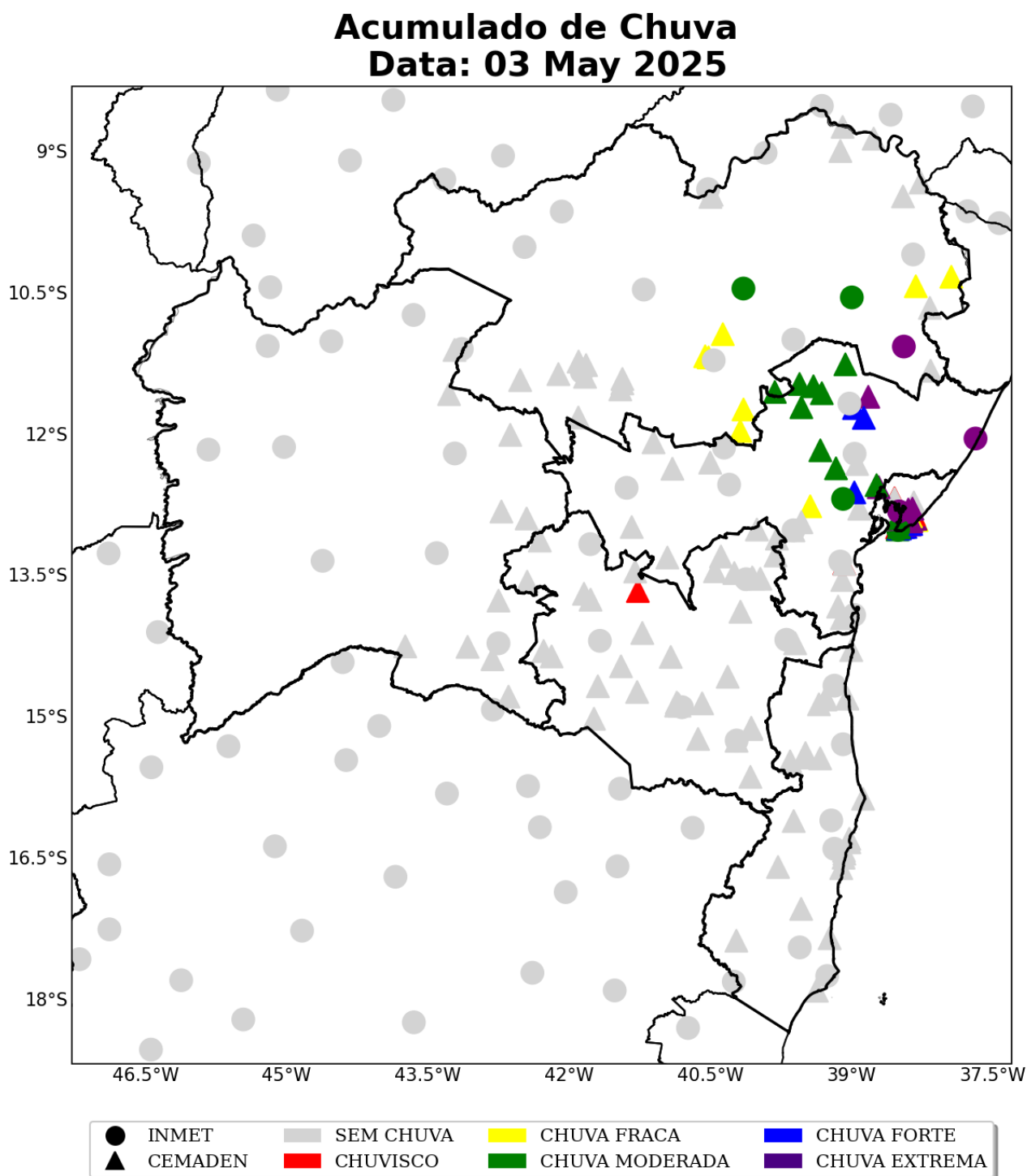
Figura 30: Acumulado diário de precipitação sobre a área de concessão da COELBA para o dia 03 de Maio, baseado nas estações meteorológicas do INMET e CEMADEN.
