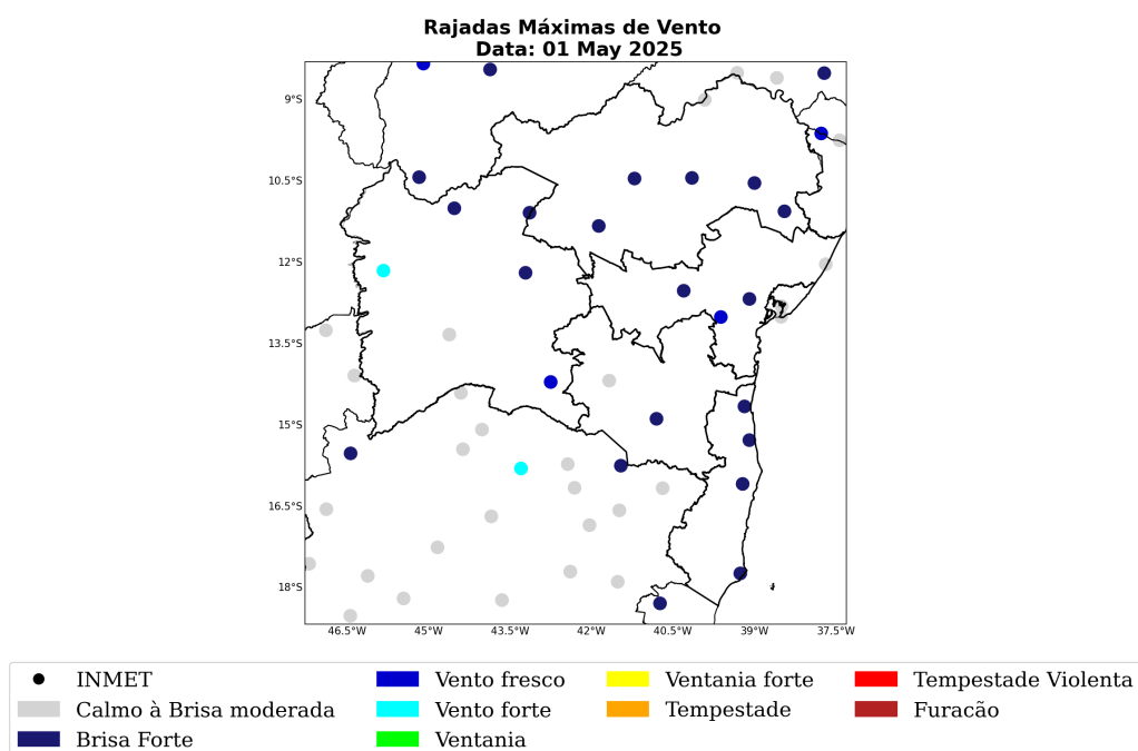
Figura 41: Máxima rajada de vento diária sobre a área de concessão da COELBA para o dia 01 de Maio, baseado nas estações meteorológicas do INMET.
