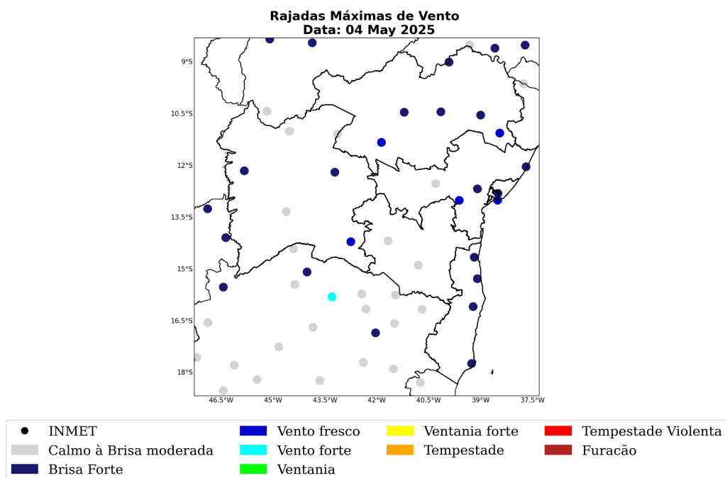
Figura 44: Máxima rajada de vento diária sobre a área de concessão da COELBA para o dia 04 de Maio, baseado nas estações meteorológicas do INMET.
