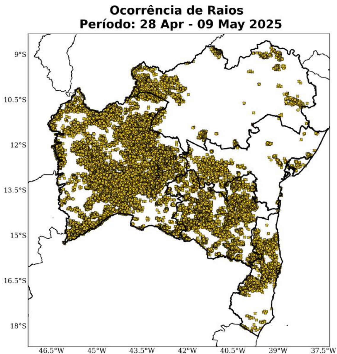
Figura 14 – Mapa de ocorrência de raios acumulado de 28 de abril a 09 de maio de 2025
