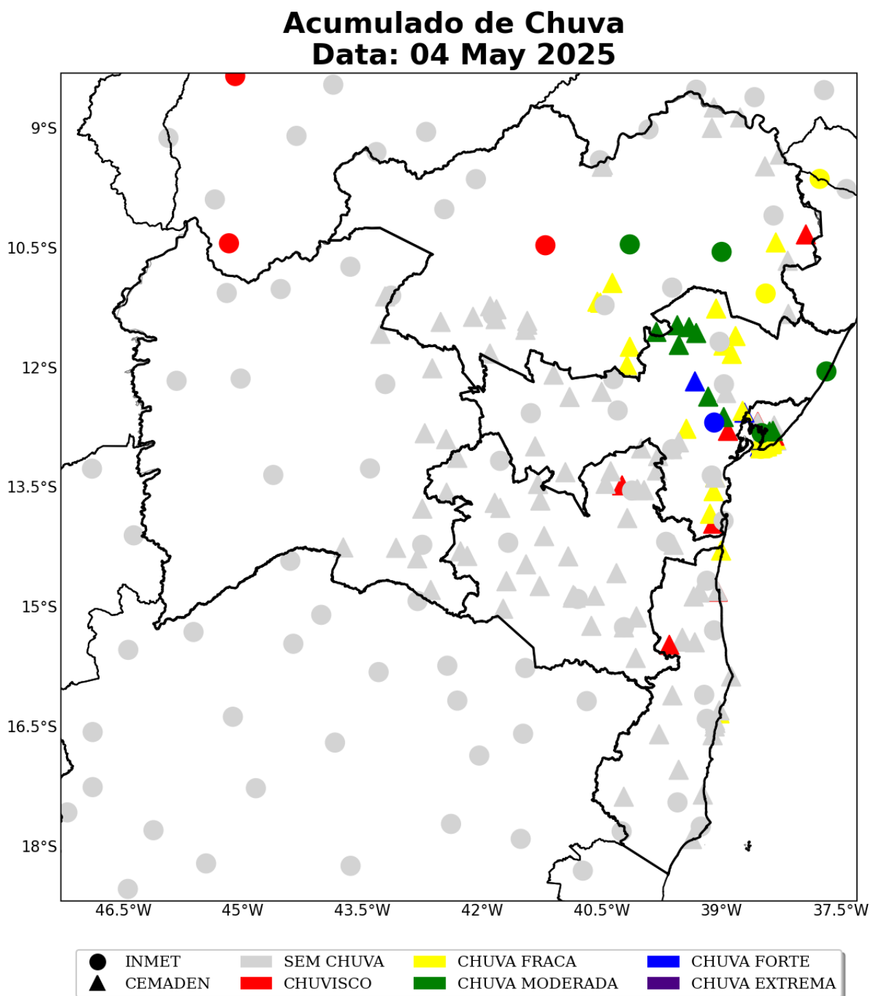
Figura 31: Acumulado diário de precipitação sobre a área de concessão da COELBA para o dia 04 de Maio, baseado nas estações meteorológicas do INMET e CEMADEN.
