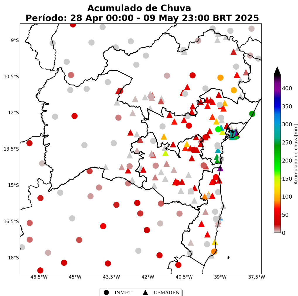
Figura 37: Acumulado de precipitação sobre o estado da Bahia para o período do evento (dias 28 a 09 de Abril de 2025), baseado nas estações meteorológicas do INMET e CEMADEN.
