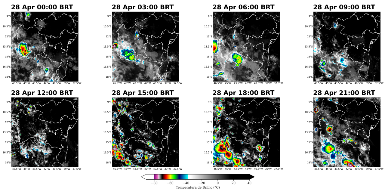
Figura 2: Imagens realçadas do satélite GOES-19 das 00 BRT até 21 BRT (a cada 3 horas) para o dia 28 de Abril.
