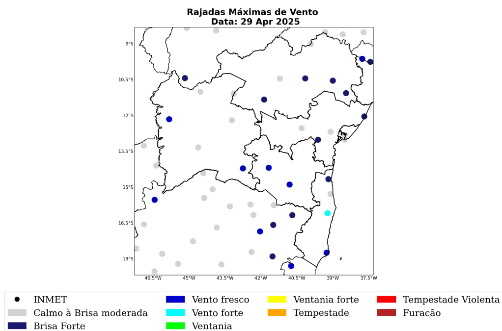
Figura 39: Máxima rajada de vento diária sobre a área de concessão da COELBA para o dia 29 de Abril, baseado nas estações meteorológicas do INMET.
