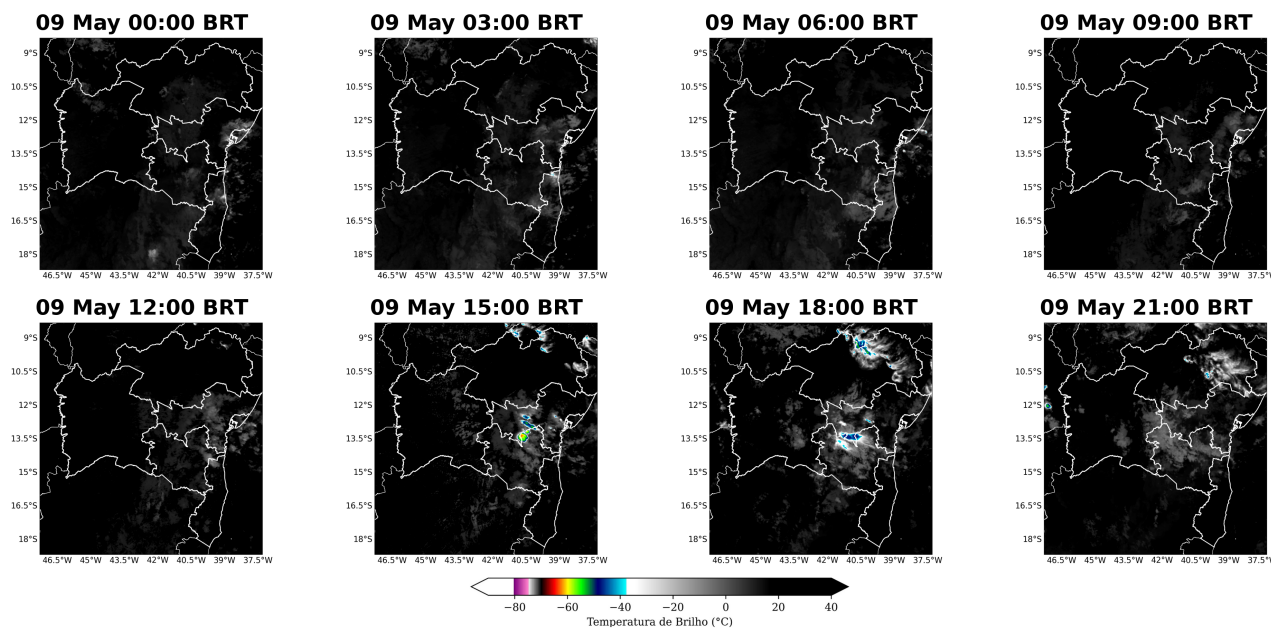
Figura 13: Imagens realçadas do satélite GOES-19 das 00 BRT até 21 BRT (a cada 3 horas) para o dia 09 de Maio.
