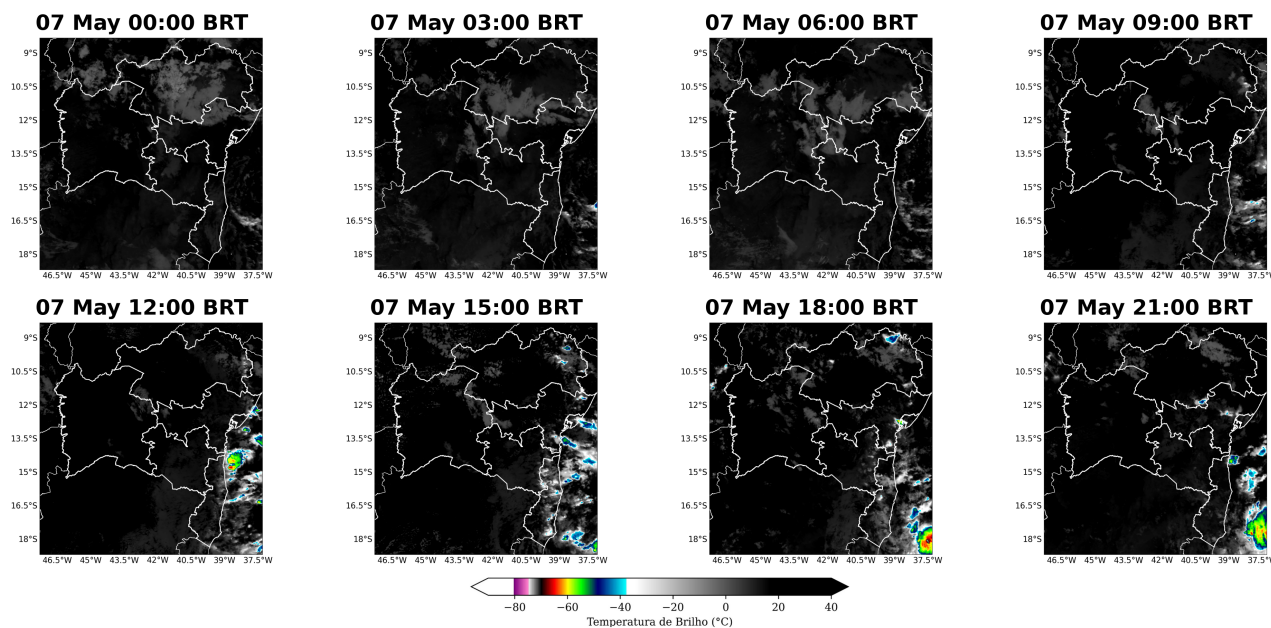
Figura 11: Imagens realçadas do satélite GOES-19 das 00 BRT até 21 BRT (a cada 3 horas) para o dia 07 de Maio.
