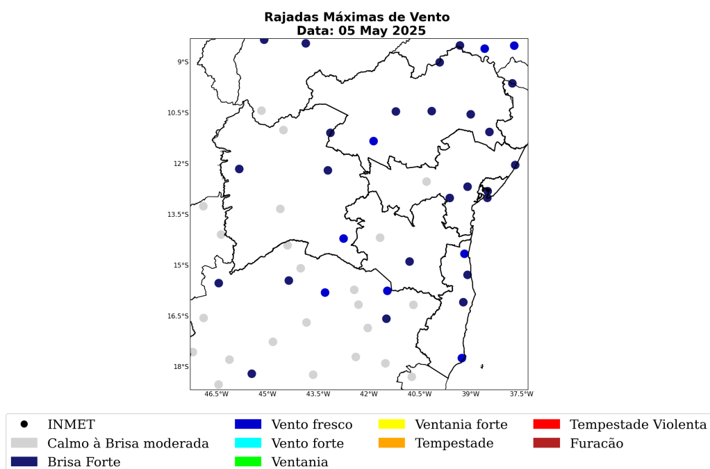
Figura 45: Máxima rajada de vento diária sobre a área de concessão da COELBA para o dia 05 de Maio, baseado nas estações meteorológicas do INMET.
