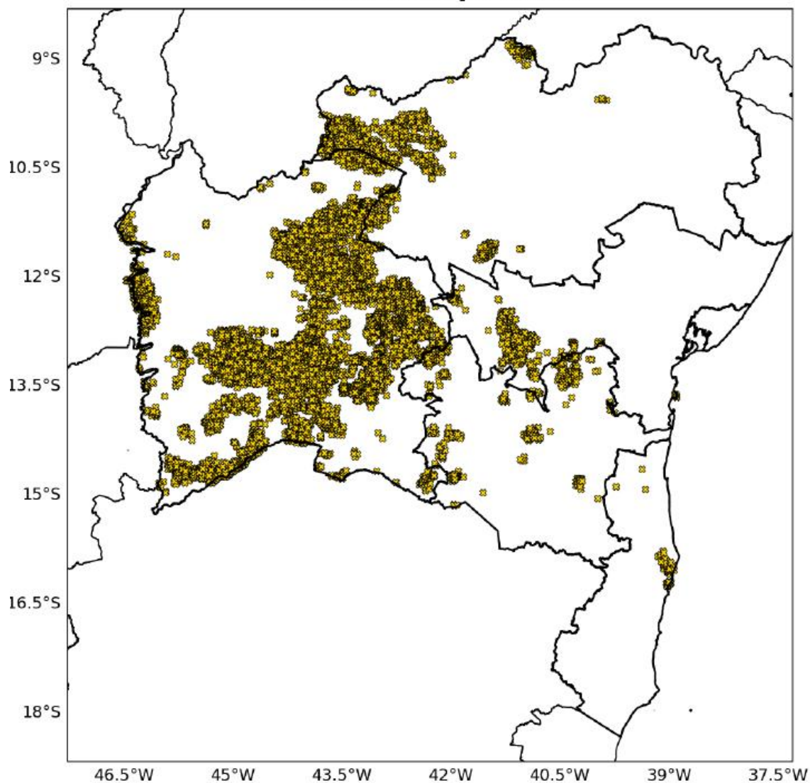
Figura 4 – Mapa de descargas atmosféricas sobre o estado da Bahia no dia 30 de abril.
