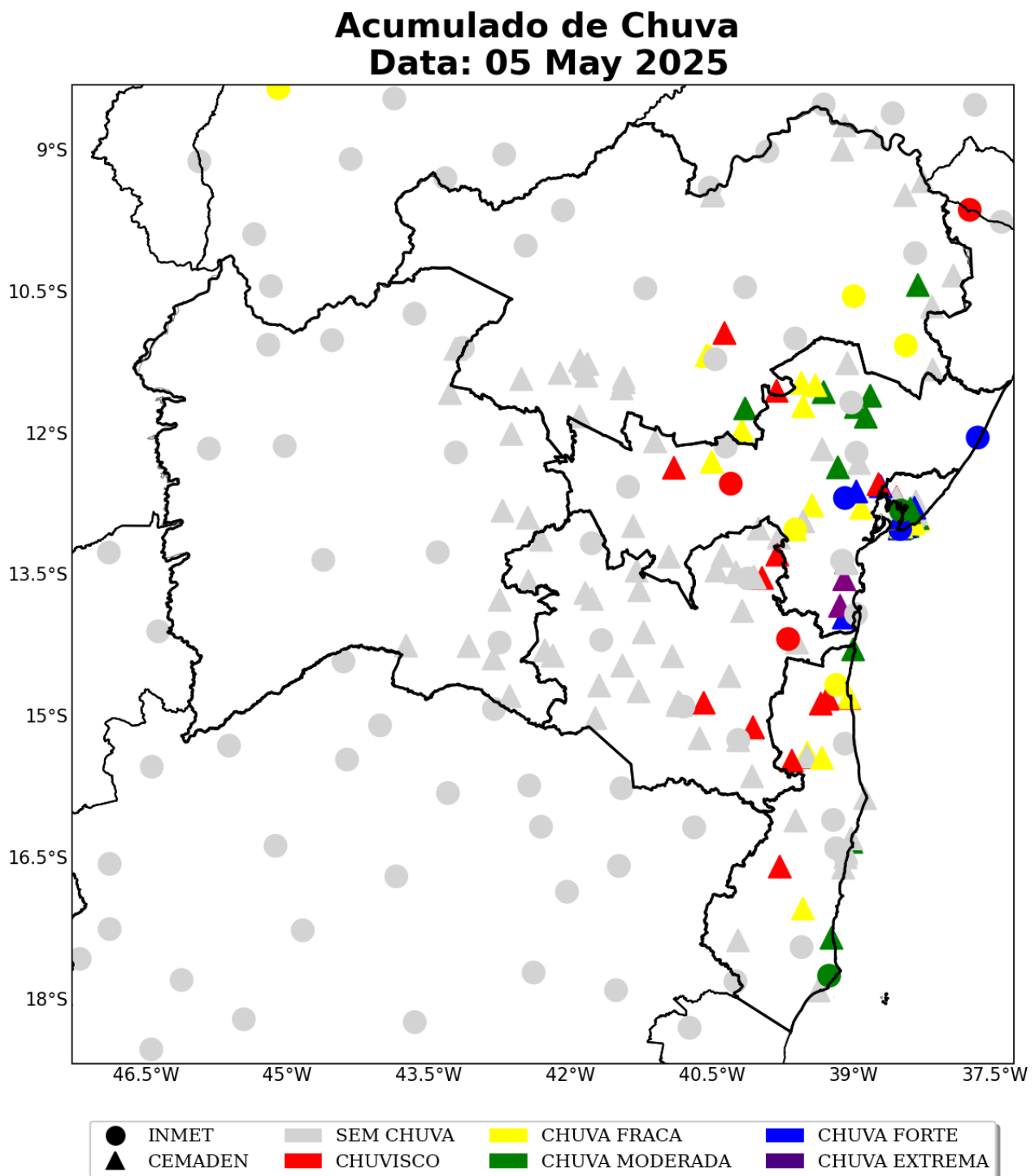
Figura 32: Acumulado diário de precipitação sobre a área de concessão da COELBA para o dia 05 de Maio, baseado nas estações meteorológicas do INMET e CEMADEN.
