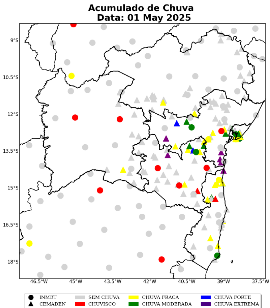
Figura 1 – Mapa do acumulado de chuva sobre o estado da Bahia em 1 de maio.
