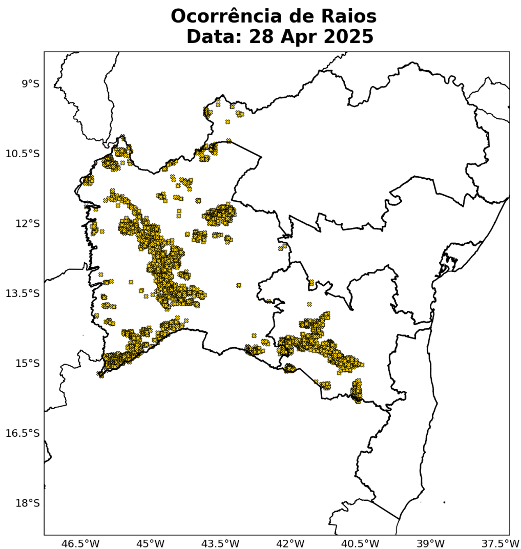
Figura 14: Ocorrências de descargas atmosféricas nuvem-solo detectadas pelo sistema Earth Networks para o dia 28 de Abril sobre a área de concessão da COELBA.
