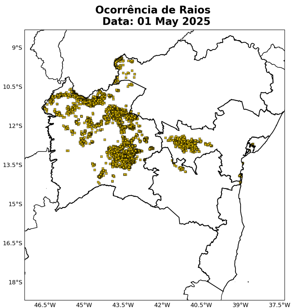
Figura 17: Ocorrências de descargas atmosféricas nuvem-solo detectadas pelo sistema Earth Networks para o dia 01 de Maio sobre a área de concessão da COELBA.
