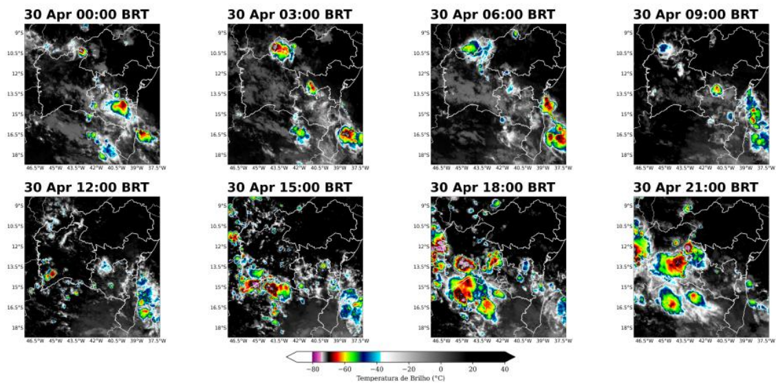
Figura 11 – Imagens realçadas do satélite GOES-16 das 00h00, 03h00, 06h00, 09h00, 12h00, 15h00, 18h00, e 21h00 do dia 30 de abril de 2025. Fonte: Climatempo
