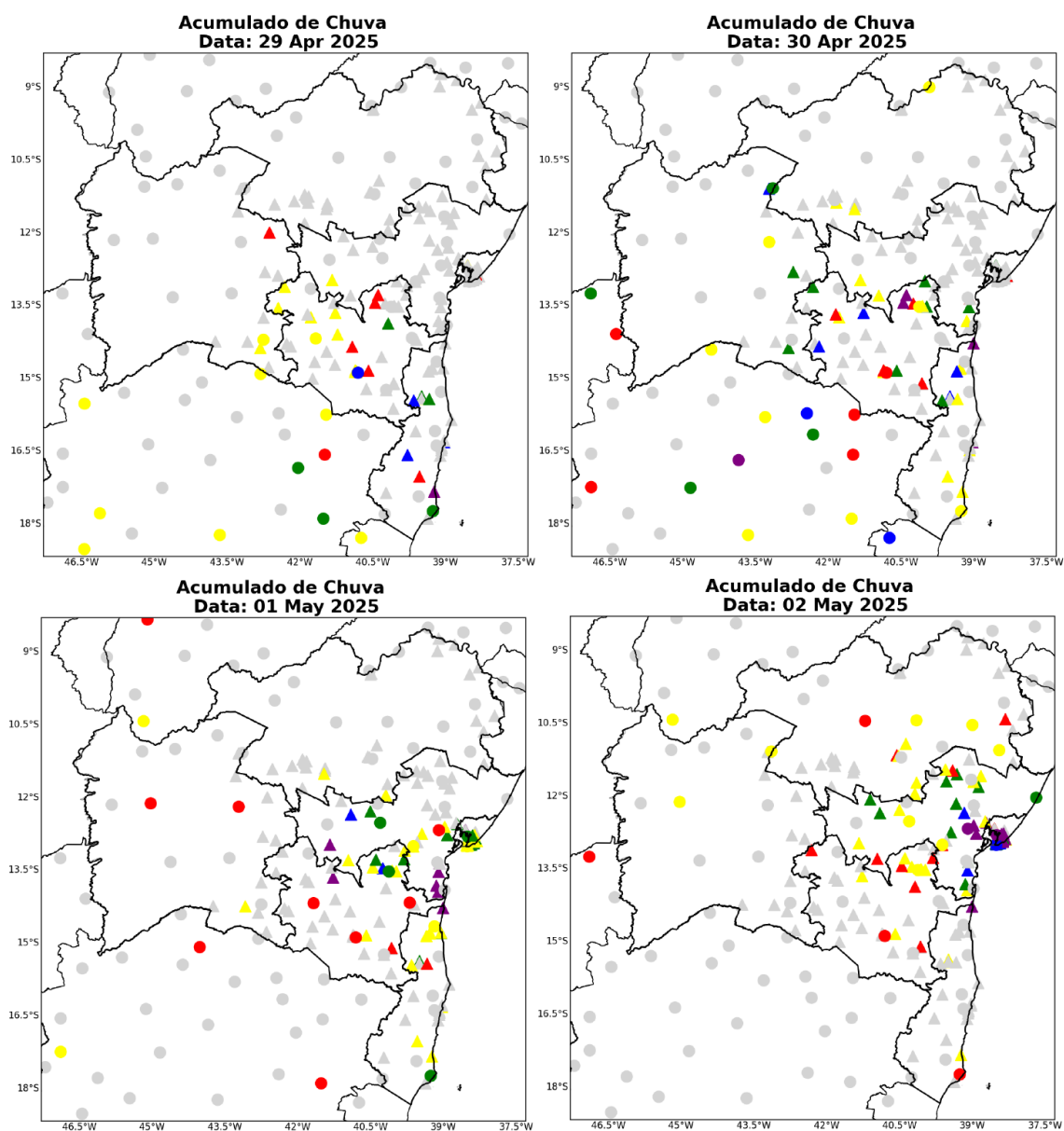
Figura 6 – Mapa de precipitação do dia 29 de abril a 02 de maio de 2025.
