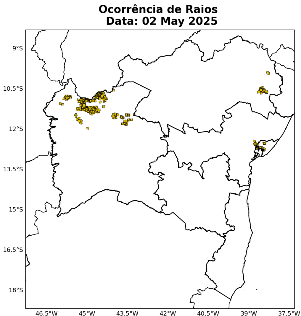
Figura 18: Ocorrências de descargas atmosféricas nuvem-solo detectadas pelo sistema Earth Networks para o dia 02 de Maio sobre a área de concessão da COELBA.
