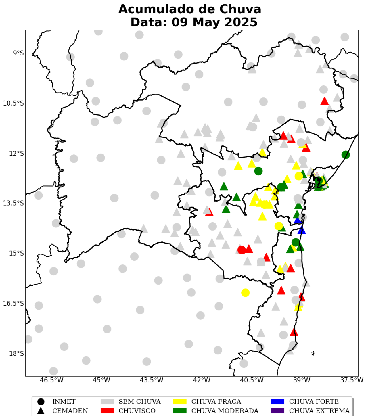
Figura 36: Acumulado diário de precipitação sobre a área de concessão da COELBA para o dia 09 de Maio, baseado nas estações meteorológicas do INMET e CEMADEN.
