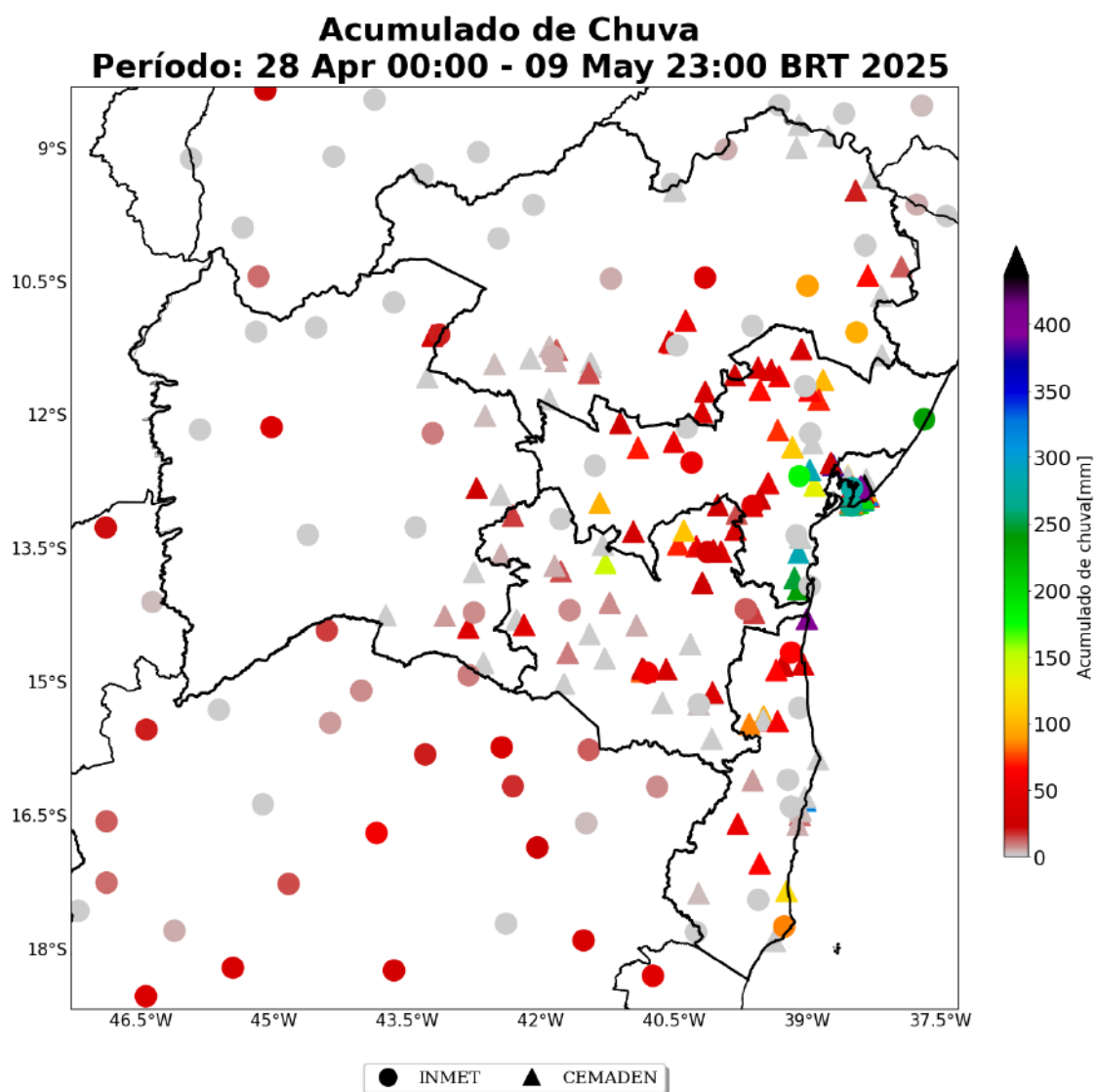
Figura 08 – Mapa Acumulado de Chuva na Bahia do dia 28 de abril a 09 de maio.
