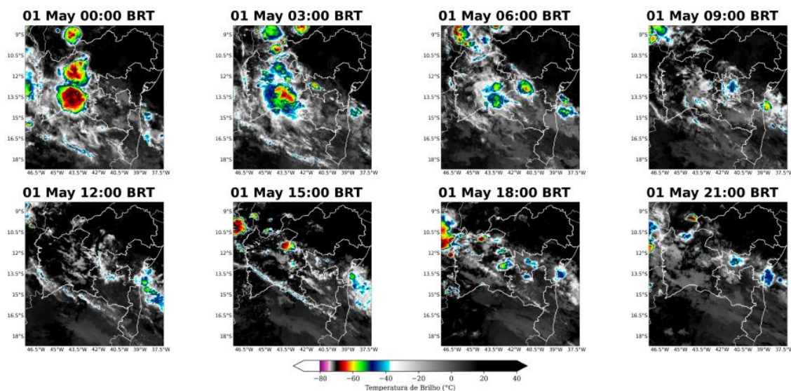
Figura 12 – Imagens realçadas do satélite GOES-16 das 00h00, 03h00, 06h00, 09h00, 12h00, 15h00, 18h00, e 21h00 do dia 01 de maio de 2025. Fonte: Climatempo
