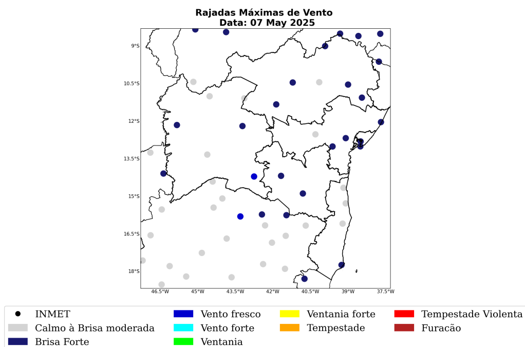
Figura 47: Máxima rajada de vento diária sobre a área de concessão da COELBA para o dia 07 de Maio, baseado nas estações meteorológicas do INMET.
