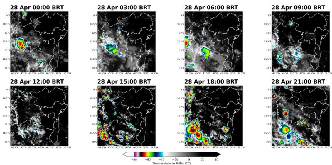
Figura 09 – Imagens realçadas do satélite GOES-16 das 00h00, 03h00, 06h00, 09h00, 12h00, 15h00, 18h00, e 21h00 do dia 28 de abril de 2025. Fonte: Climatempo
