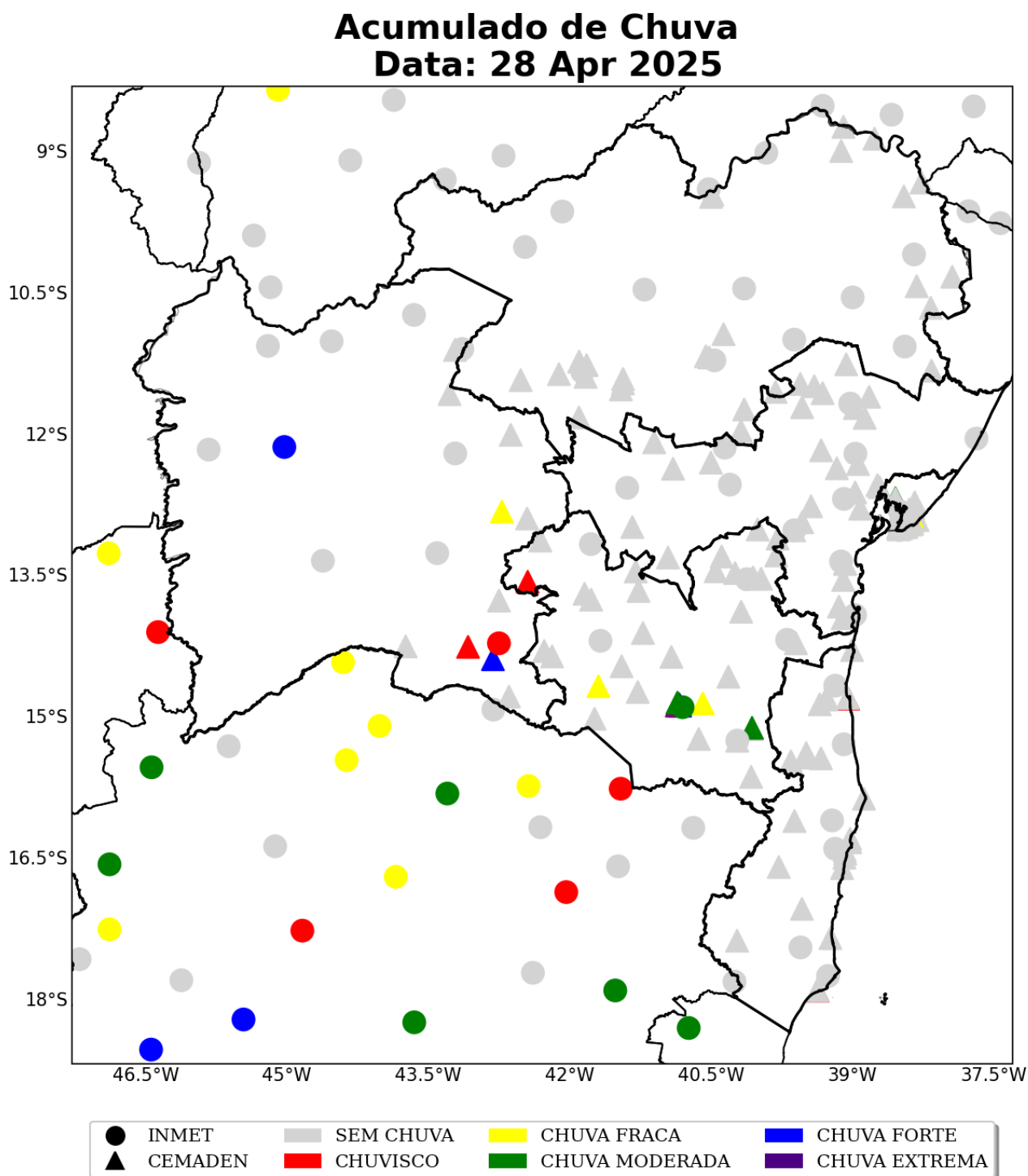
Figura 25: Acumulado diário de precipitação sobre a área de concessão da COELBA para o dia 28 de Abril, baseado nas estações meteorológicas do INMET e CEMADEN.
