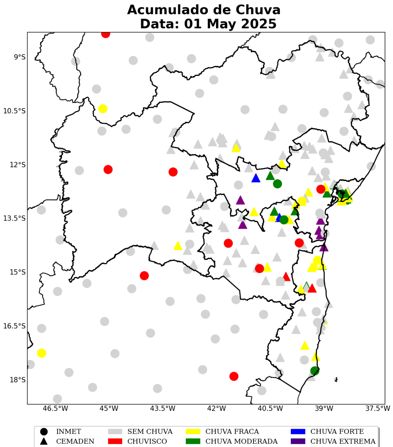
Figura 28: Acumulado diário de precipitação sobre a área de concessão da COELBA para o dia 01 de Maio, baseado nas estações meteorológicas do INMET e CEMADEN.
