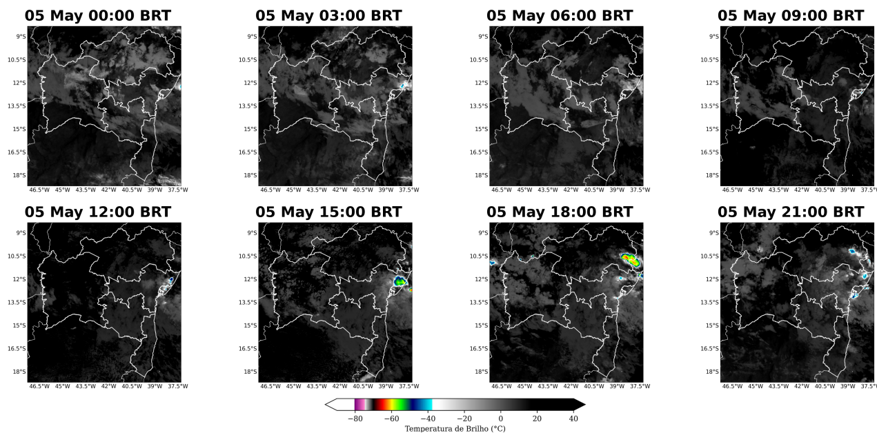
Figura 9: Imagens realçadas do satélite GOES-19 das 00 BRT até 21 BRT (a cada 3 horas) para o dia 05 de Maio.
