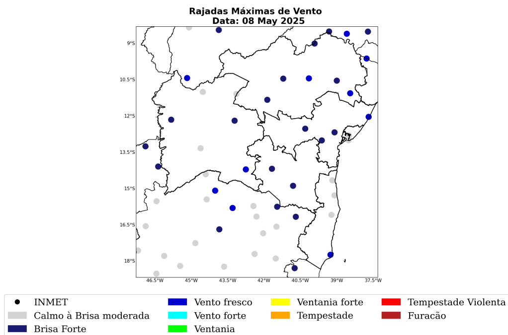
Figura 48: Máxima rajada de vento diária sobre a área de concessão da COELBA para o dia 08 de Maio, baseado nas estações meteorológicas do INMET.
