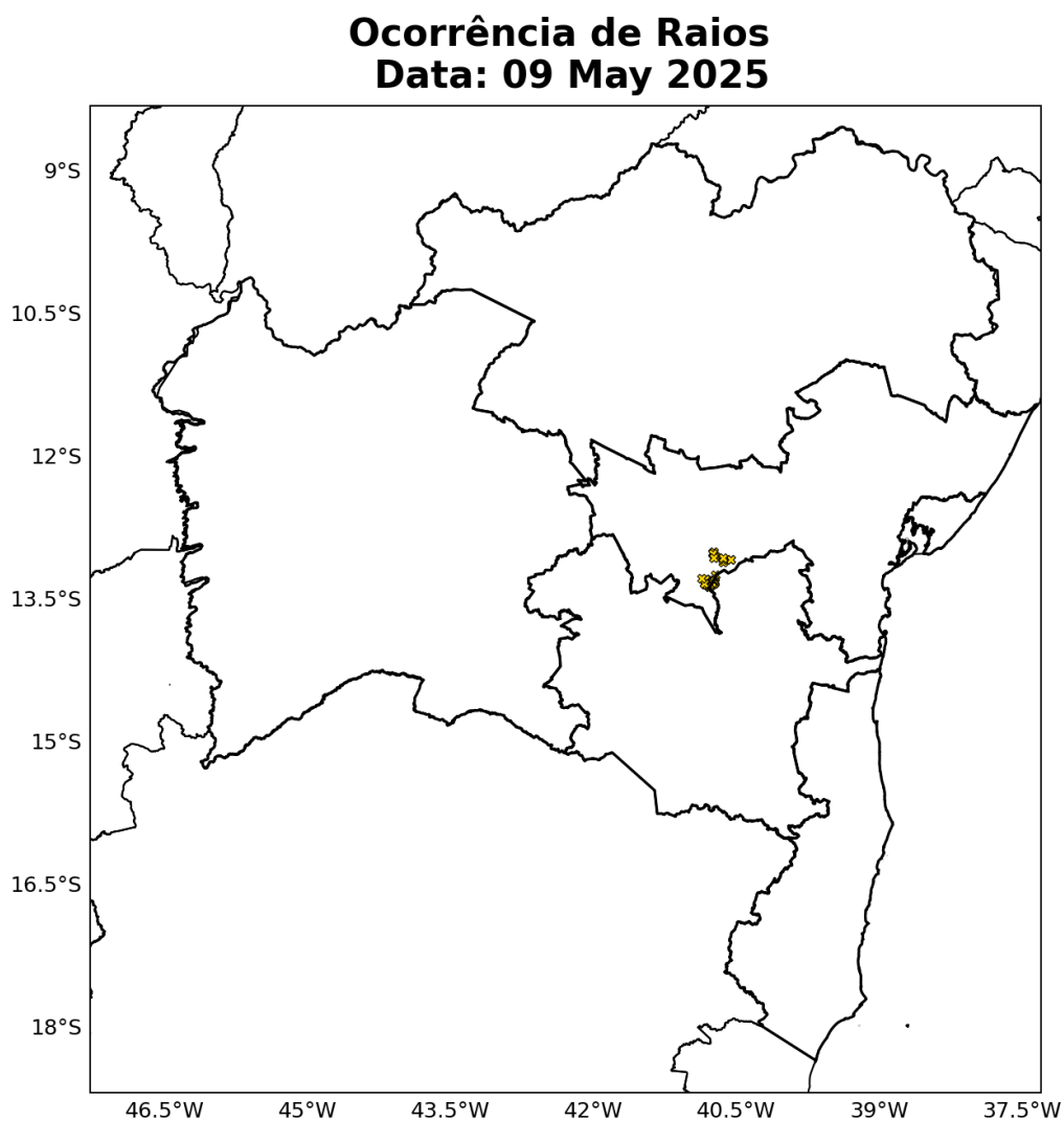
Figura 23: Ocorrências de descargas atmosféricas nuvem-solo detectadas pelo sistema Earth Networks para o dia 09 de Maio sobre a área de concessão da COELBA.
