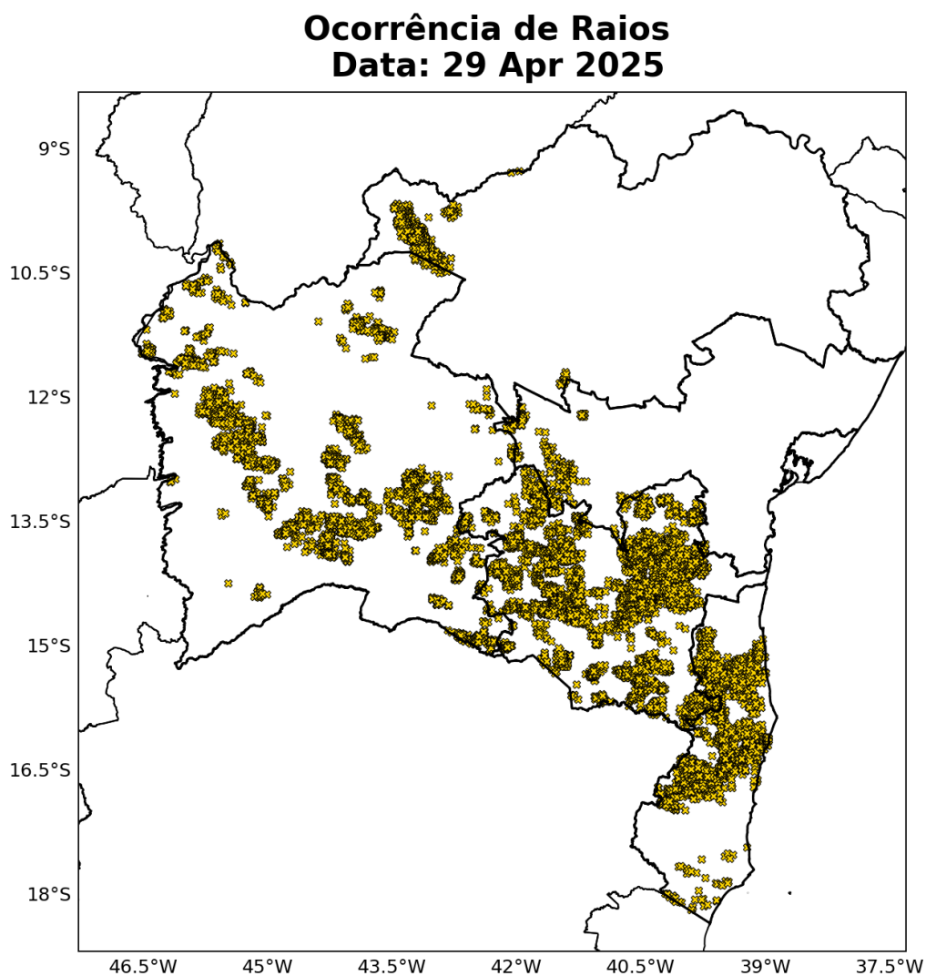
Figura 15: Ocorrências de descargas atmosféricas nuvem-solo detectadas pelo sistema Earth Networks para o dia 29 de Abril sobre a área de concessão da COELBA.
