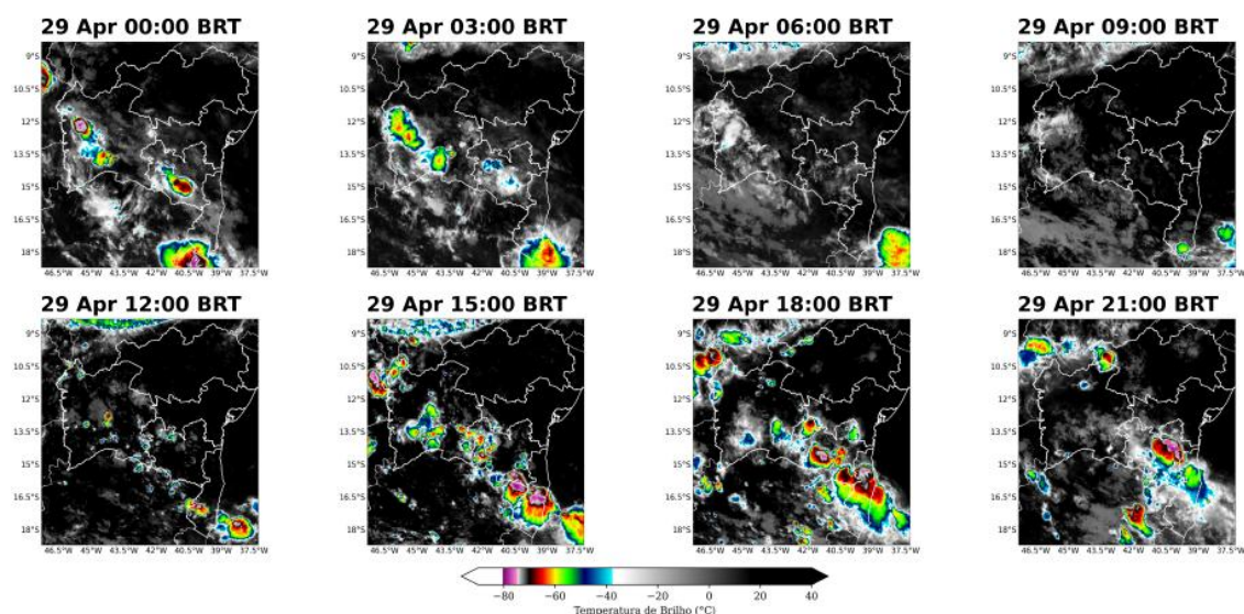
Figura 10 – Imagens realçadas do satélite GOES-16 das 00h00, 03h00, 06h00, 09h00, 12h00, 15h00, 18h00, e 21h00 do dia 29 de abril de 2025. Fonte: Climatempo
