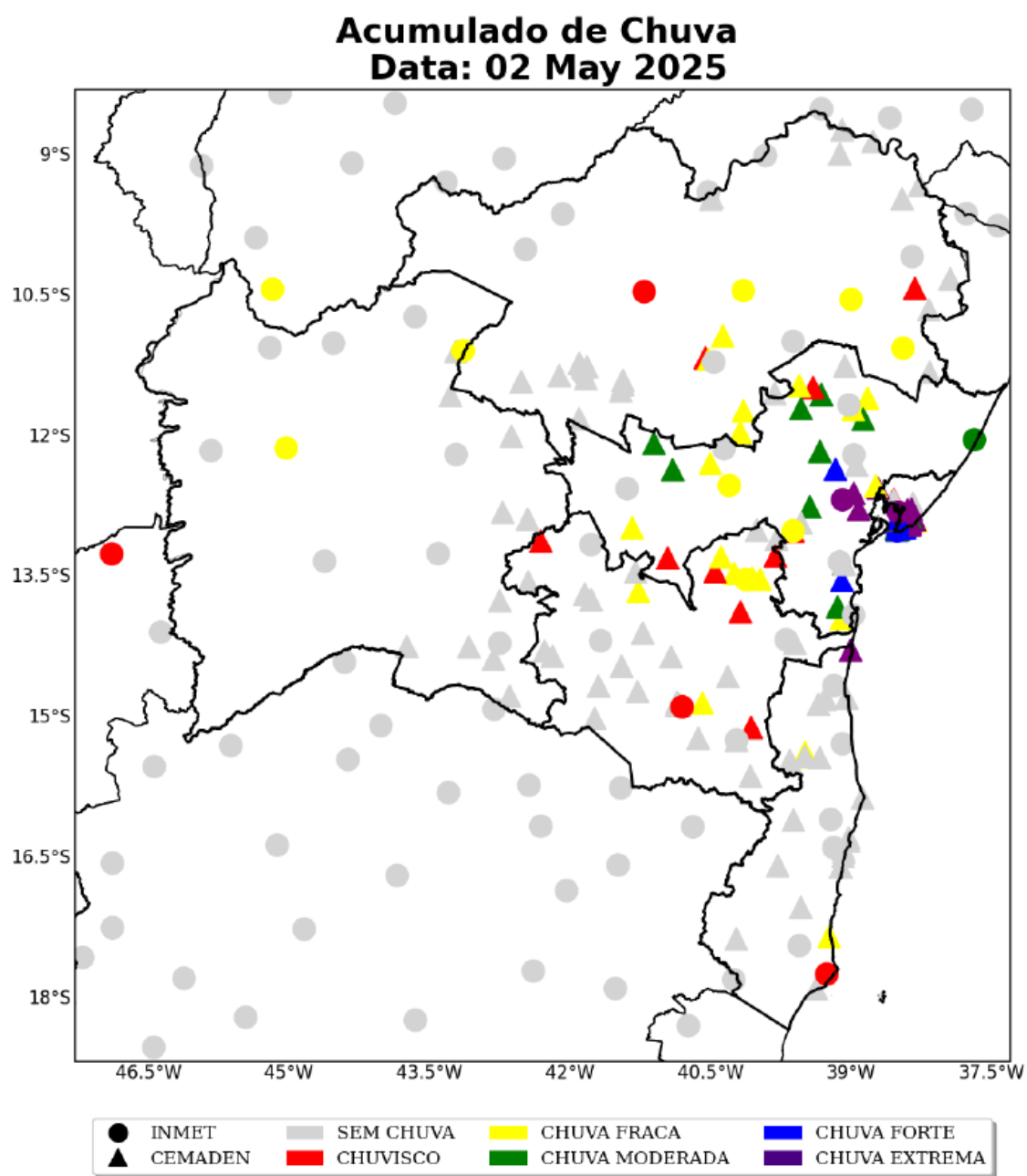
Figura 2 – Mapa do acumulado de chuva sobre o estado da Bahia em 2 de maio.
