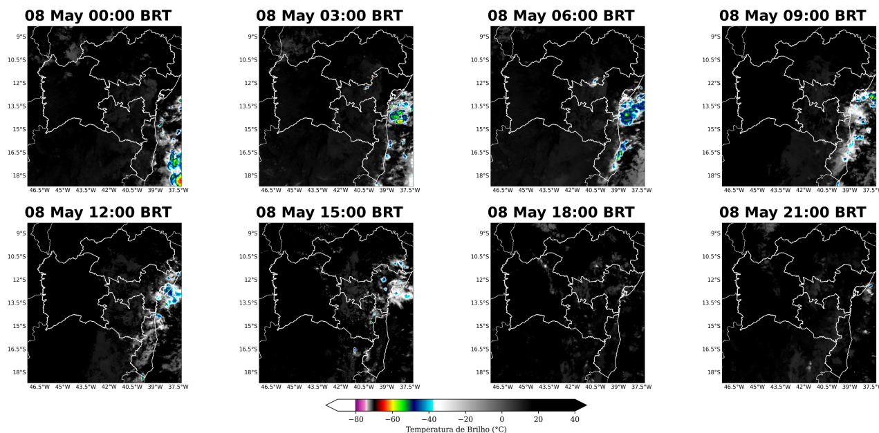
Figura 12: Imagens realçadas do satélite GOES-19 das 00 BRT até 21 BRT (a cada 3 horas) para o dia 08 de Maio.
