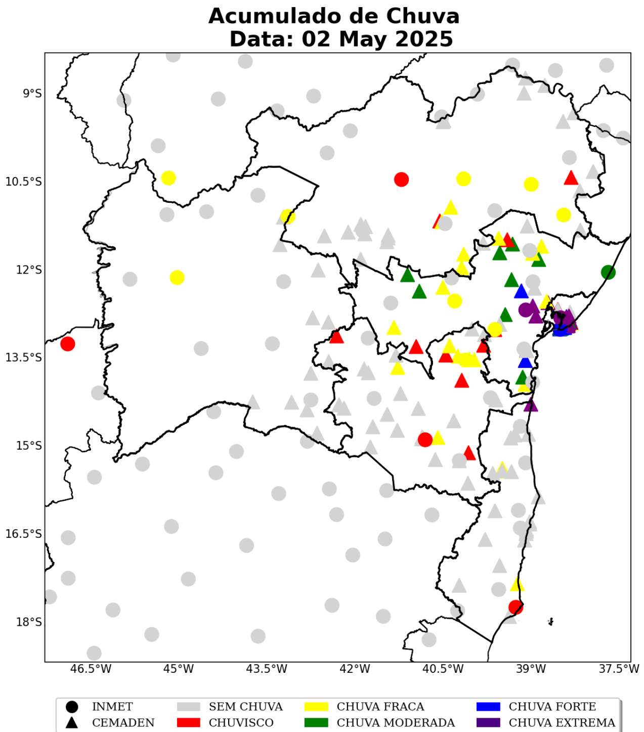
Figura 29: Acumulado diário de precipitação sobre a área de concessão da COELBA para o dia 02 de Maio, baseado nas estações meteorológicas do INMET e CEMADEN.
