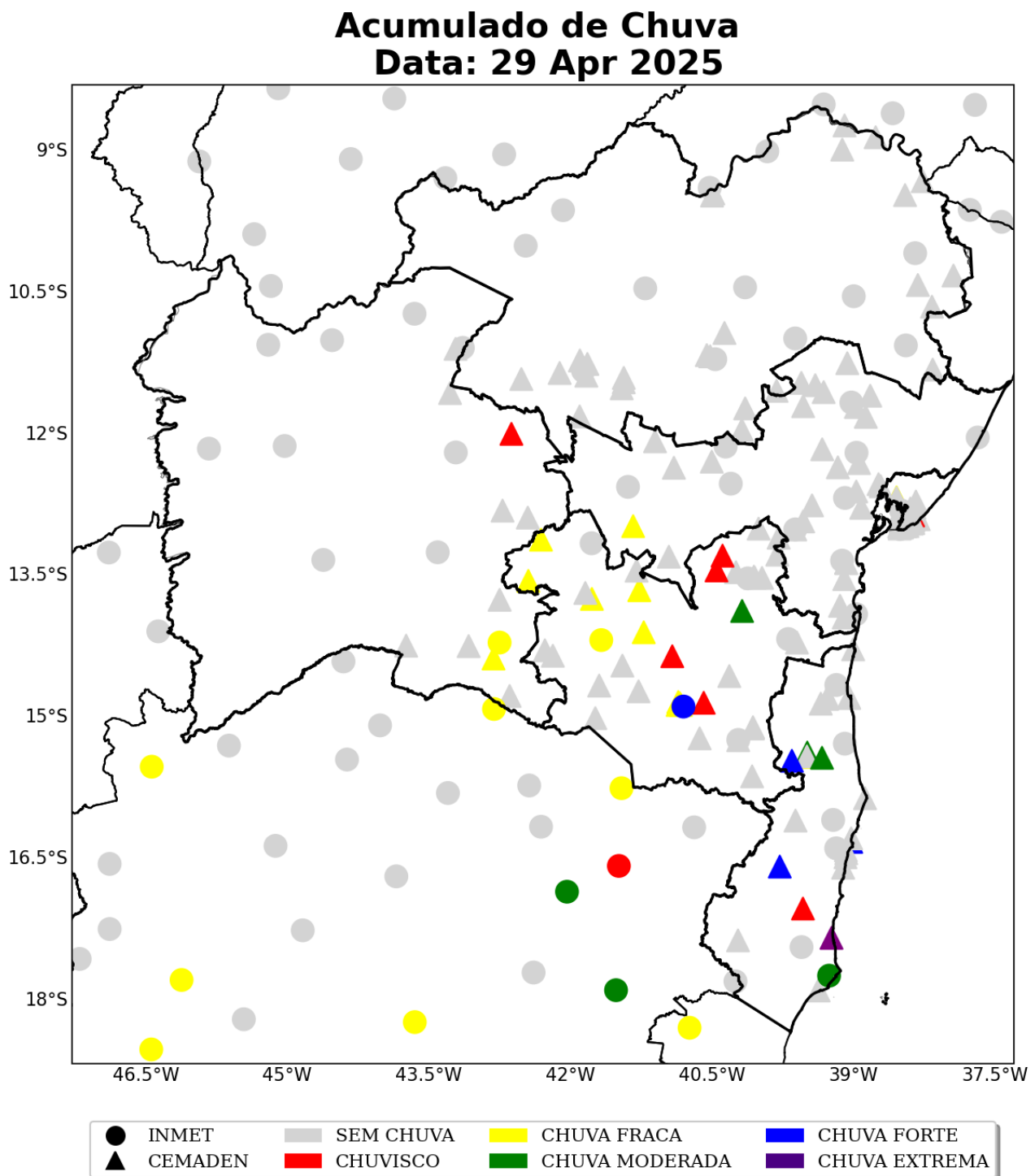
Figura 26: Acumulado diário de precipitação sobre a área de concessão da COELBA para o dia 29 de Abril, baseado nas estações meteorológicas do INMET e CEMADEN.
