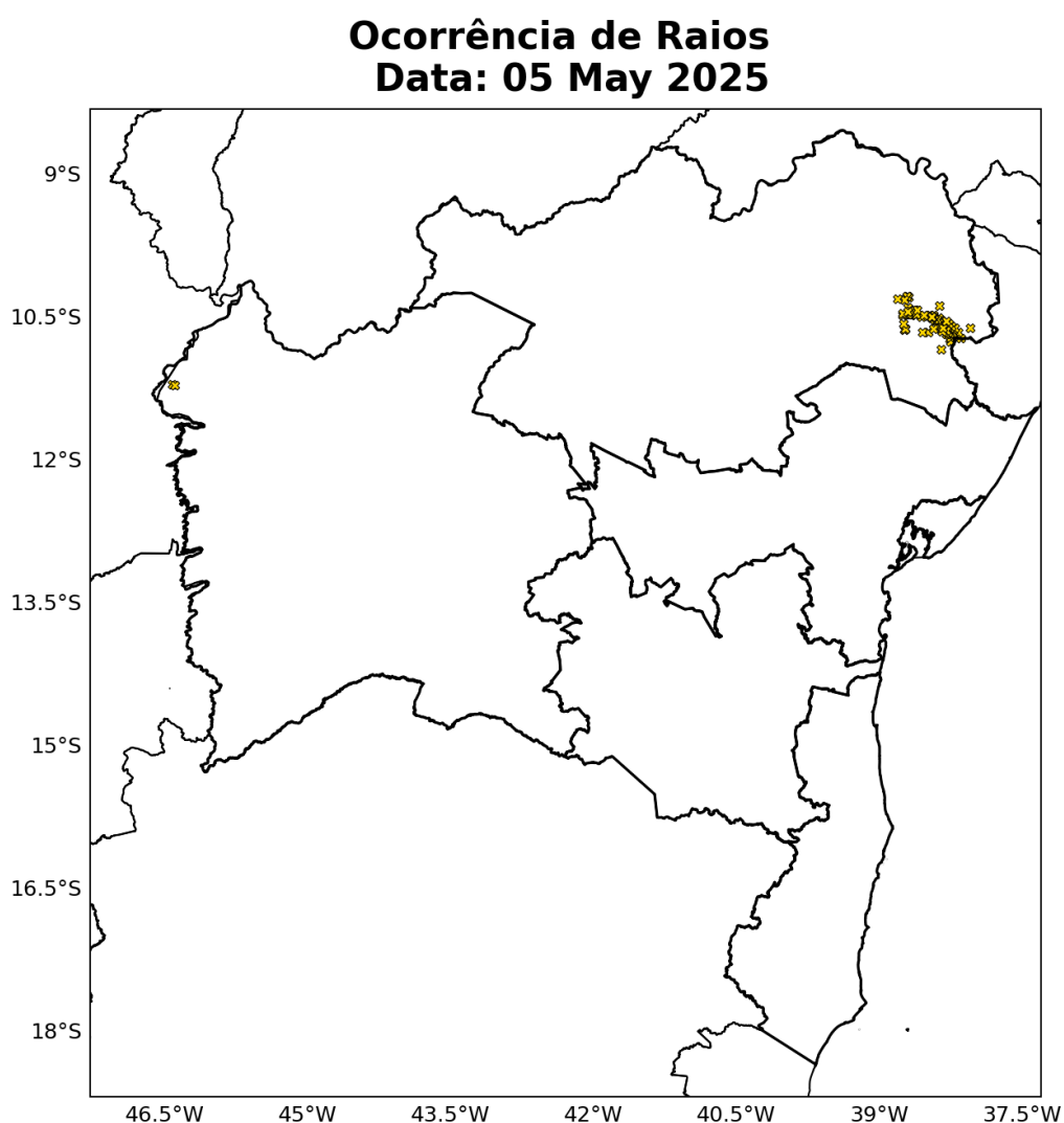
Figura 19: Ocorrências de descargas atmosféricas nuvem-solo detectadas pelo sistema Earth Networks para o dia 05 de Maio sobre a área de concessão da COELBA.
