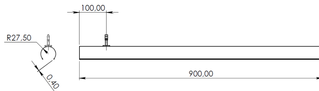
Imagem ilustrativa do eletrodo para cobertura flexível Ø55mm
