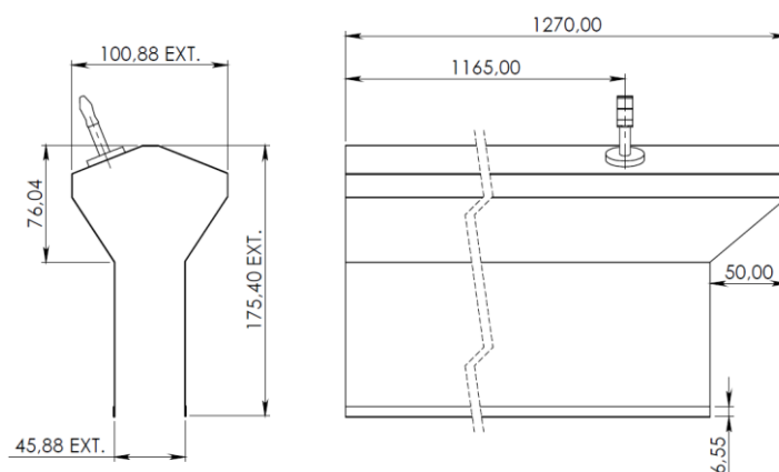
Imagem ilustrativa do eletrodo para cobertura rígida de classe 4
