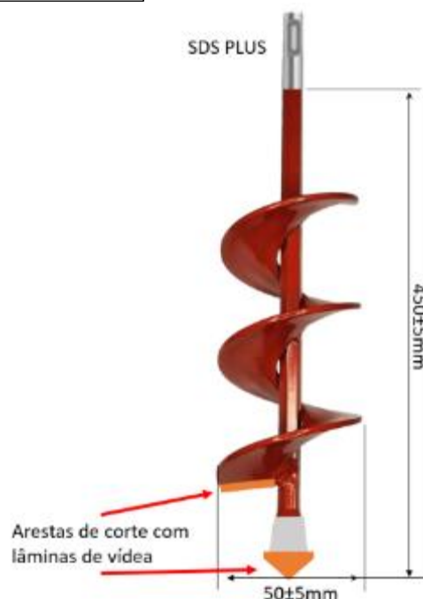
Item 2: Broca SDS Plus 450x50x8
