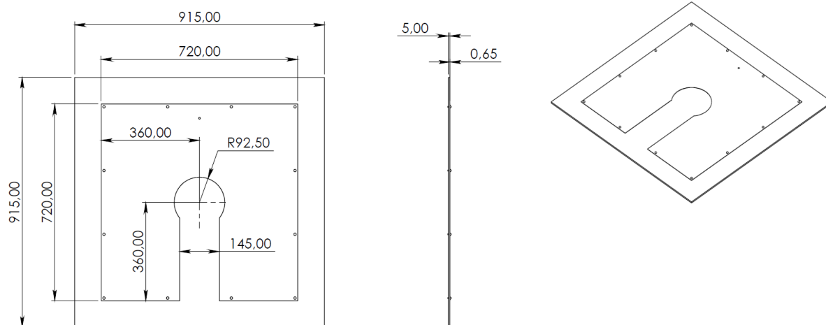
Item 27 – Eletrodo para lençol semi partido classe 4
