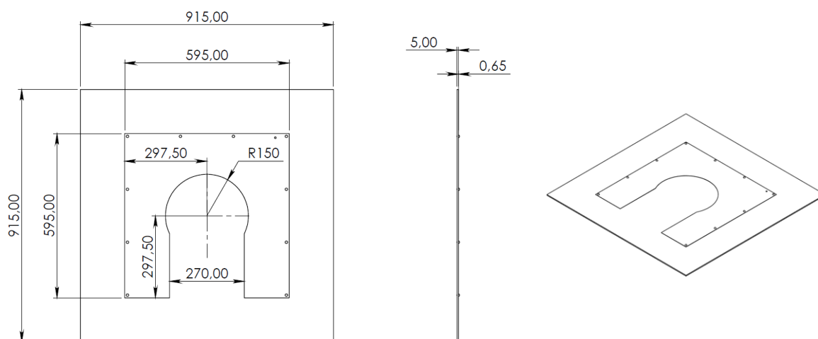
Item 27 – Eletrodo para lençol semi partido classe 4
