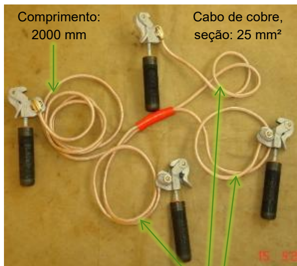
Grampo de aterramento
