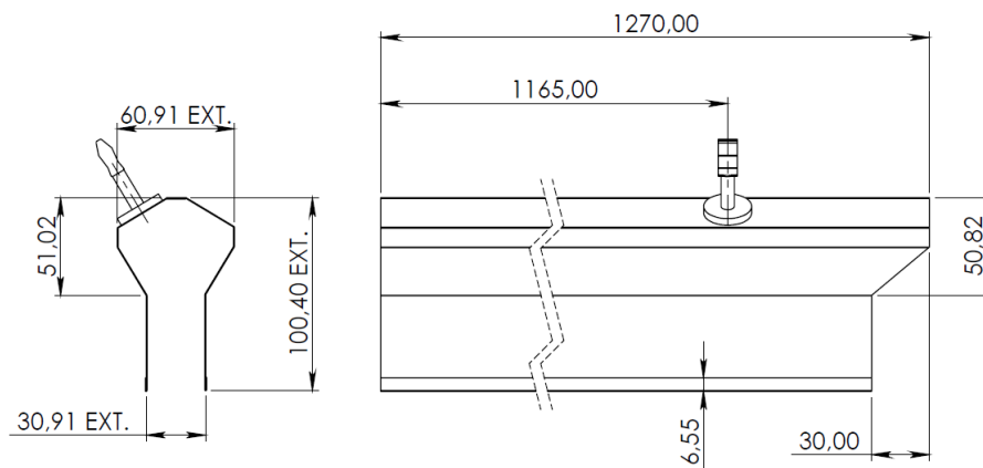
Imagem ilustrativa do eletrodo para cobertura rígida de classe 2
