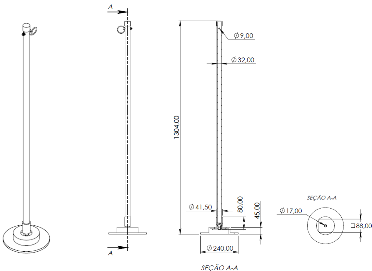
Imagem ilustrativa do braço de apoio – Item 2
