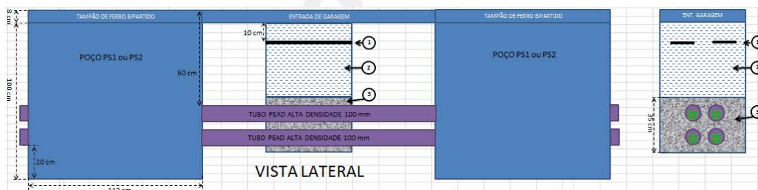
Eletroduto de polietileno de alta densidade (PEAD) em entrada de garagem
