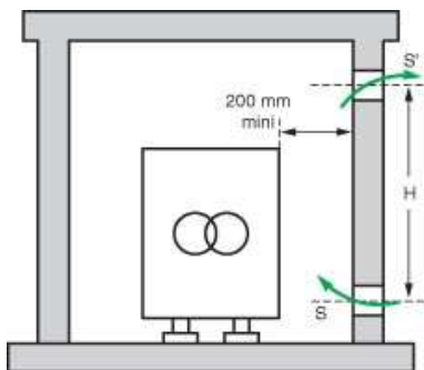
Figura 5 – Troca de Calor pelo Modo de Convecção Livre
