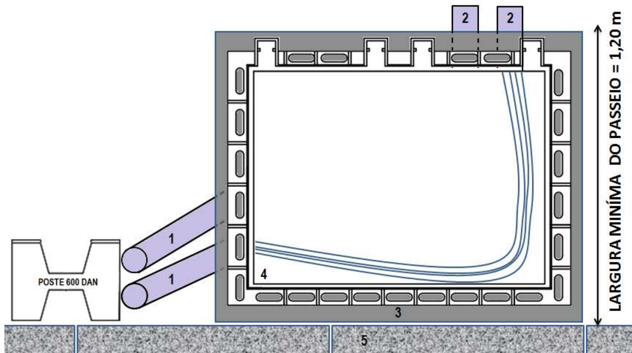
Desenho 26 - Representação Descida do Poste com Poço PSI para Rede de BT
