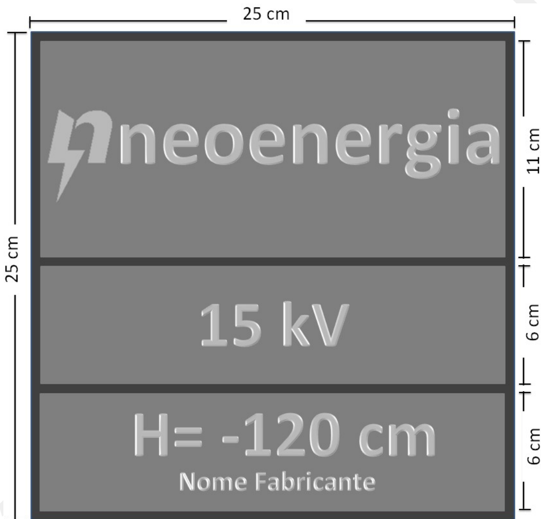
Desenho 55 – Placa para Sinalização de Rede de Distribuição Subterrânea
