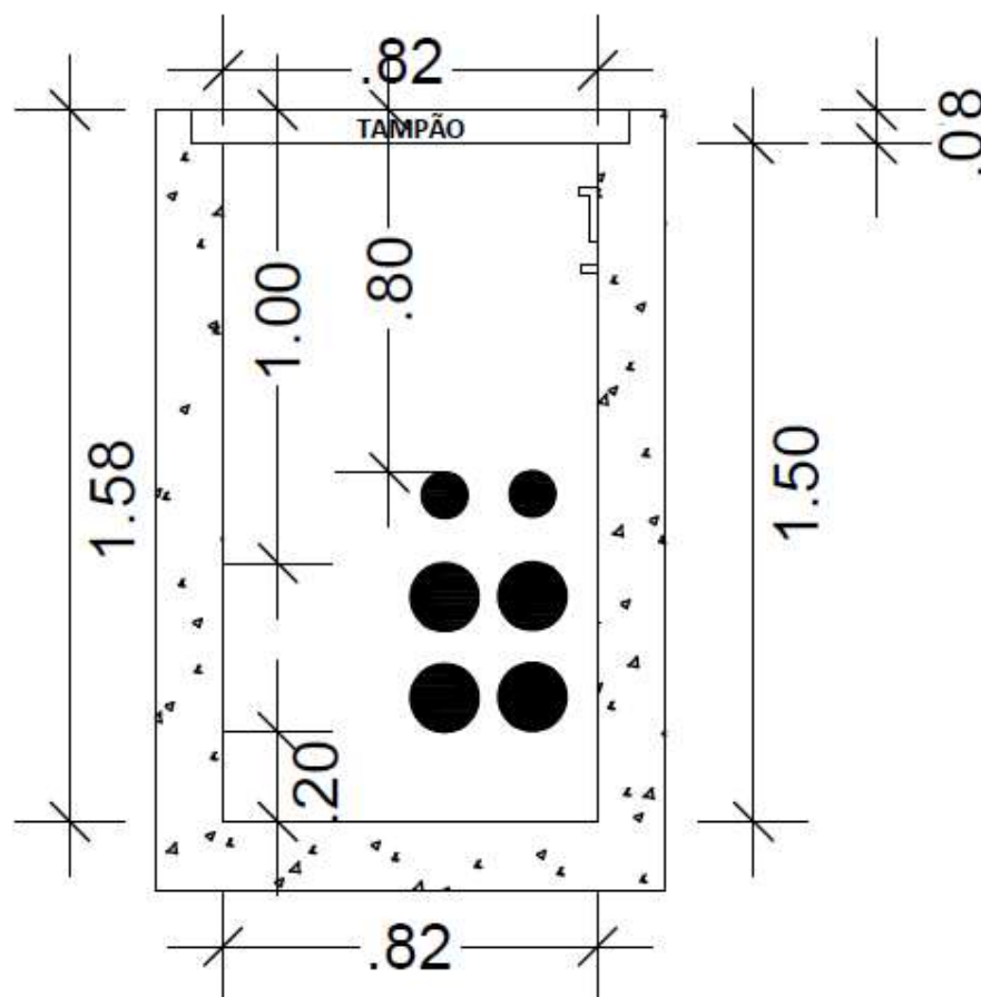
Desenho 18 - Poço Primário (PP) - 15 kV - 3/6
