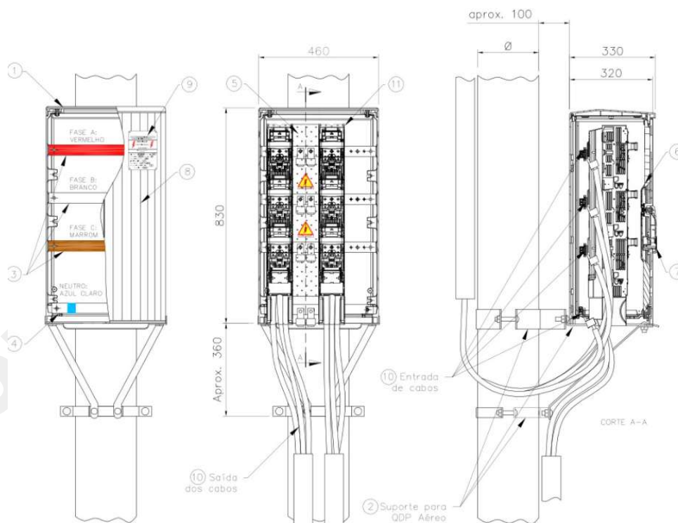
Quadro para dois circuitos (I202012)
