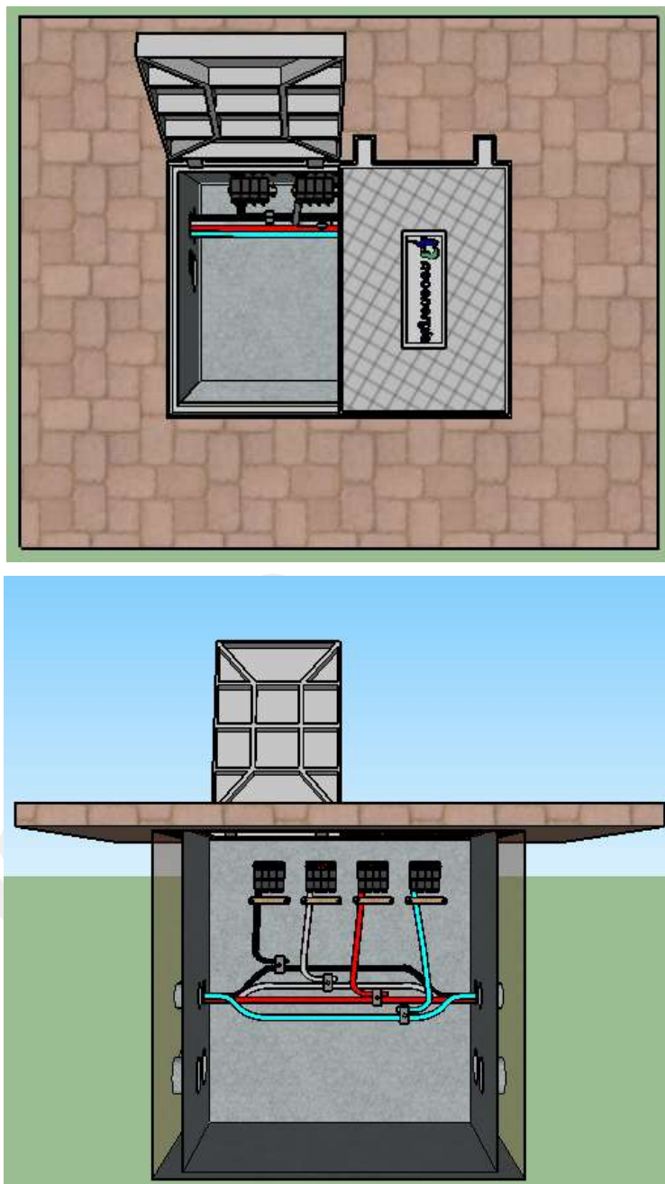
Desenho 18 - Poço Primário (PP) - 15 kV - 4/6
