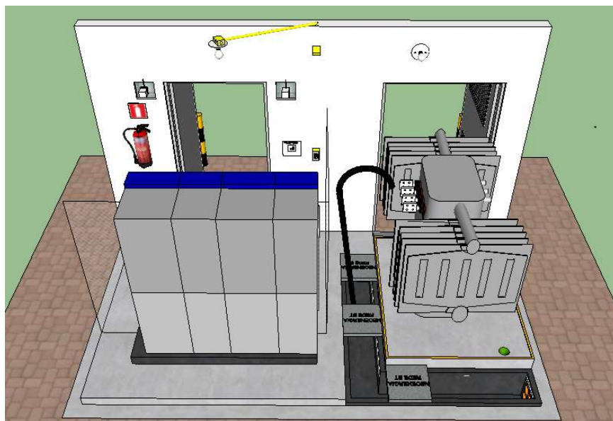
Desenho 8 - CTE para 1 Transformador de até 225 kVA - 7/9 (CTE-R-225/CTE-225-RE+P/ CTE-225-RE+2P/ CTE-225-RE+3P)
