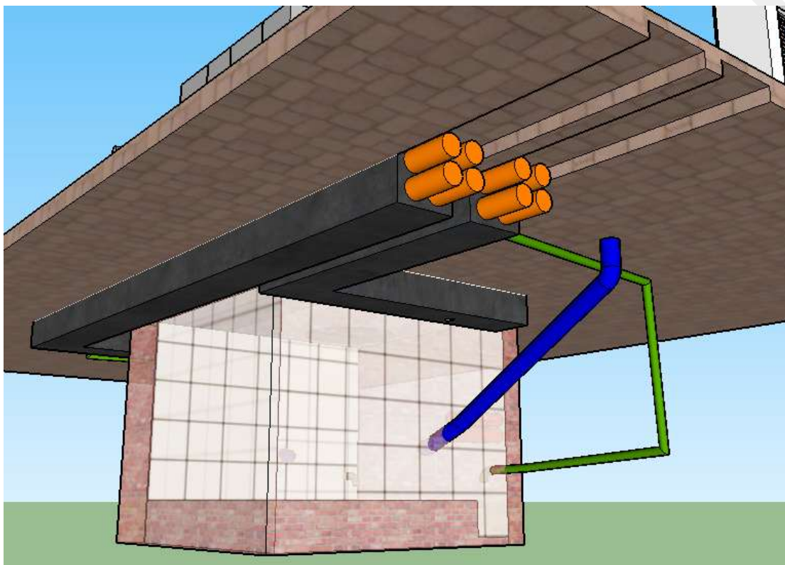
Desenho 10 - CTE para 2 Transformadores de até 225 kVA - 8/8 (CTE-R-450-RE+2P/ CTE-R-450-RE+3P/CTE-A-2L+P)
