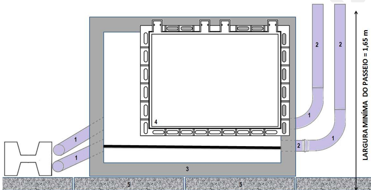
Desenho 30 - Representação da descida do poste com poço PE para rede de MT 50/120 mm 2
