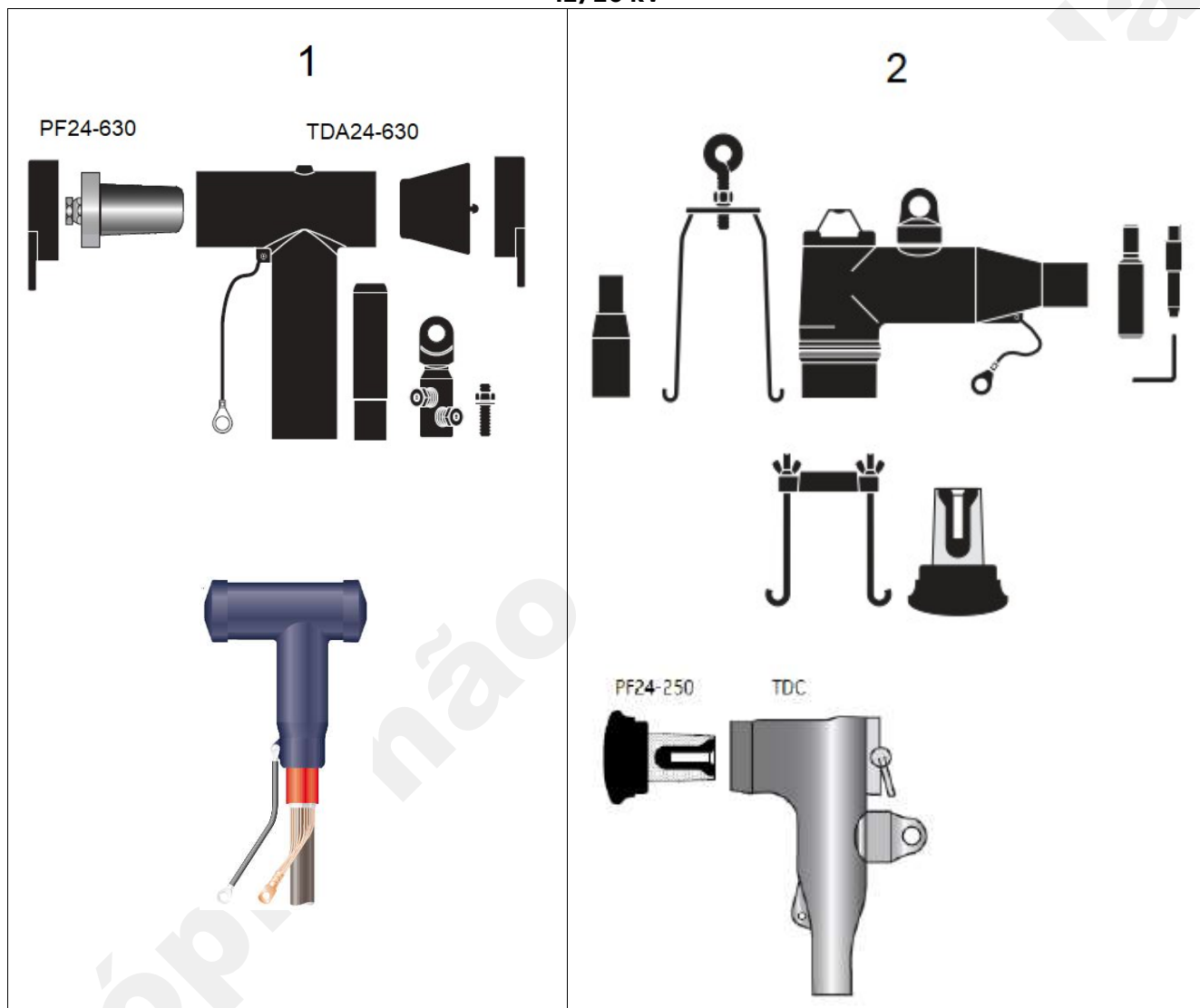
Desenho 35 - Representação da Conexão do 4 cabo Para o Sistema Radial com Cabo 50 mm 2 12/20 kV
