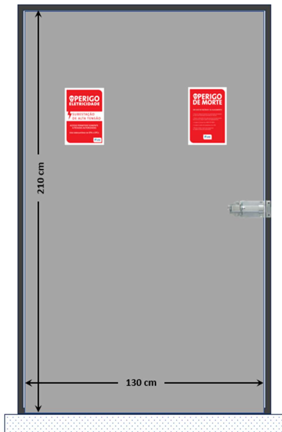
Porta acesso para pessoas: CT 15/34,5 kV
