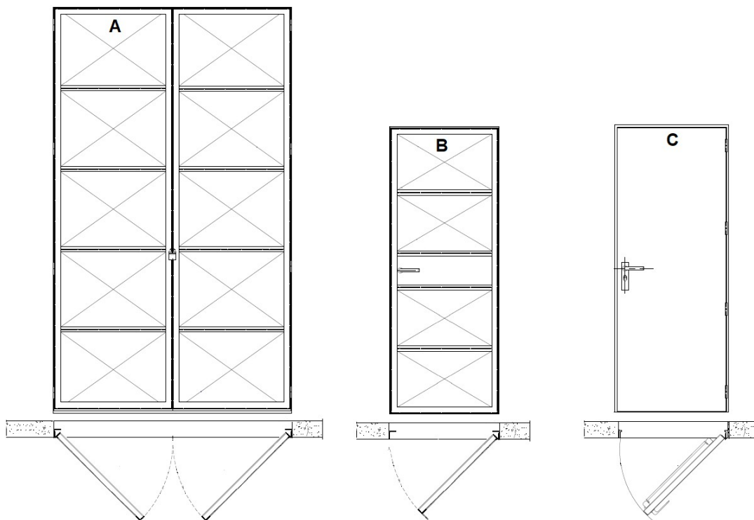
Desenho 69 – Portas das Câmaras sem área de ventilação
