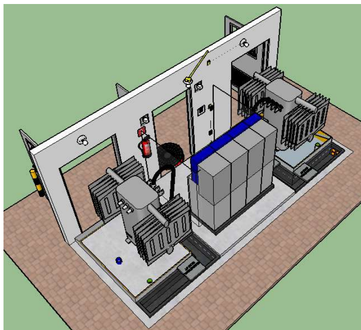
Desenho 9 - CTE para 2 Transformadores de até 225 kVA - 8/10 (CTE-R-450-RE+2P/ CTE-R-450-RE+3P/CTE-A-2L+P)
