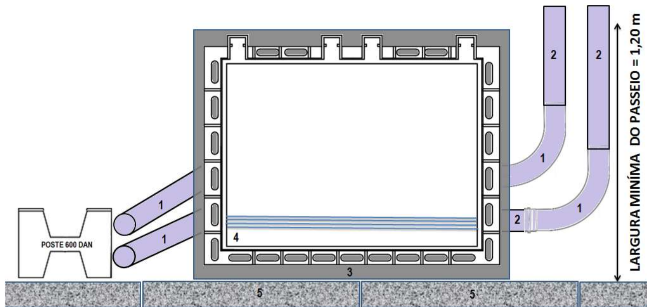
Desenho 27 - Representação Descida do Poste com Poço PS1 para Rede de BT
