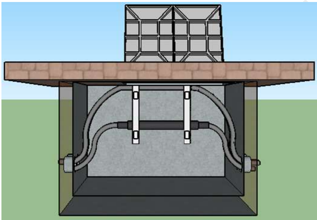
Desenho 31 - Representação da Folga dos Cabos no Poço PE
