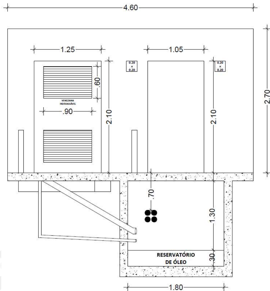
Desenho 8 - CTE para 1 Transformador de até 225 kVA - 2/9 (CTE-R-225/CTE-225-RE+P/ CTE-225-RE+2P/ CTE-225-RE+3P)
