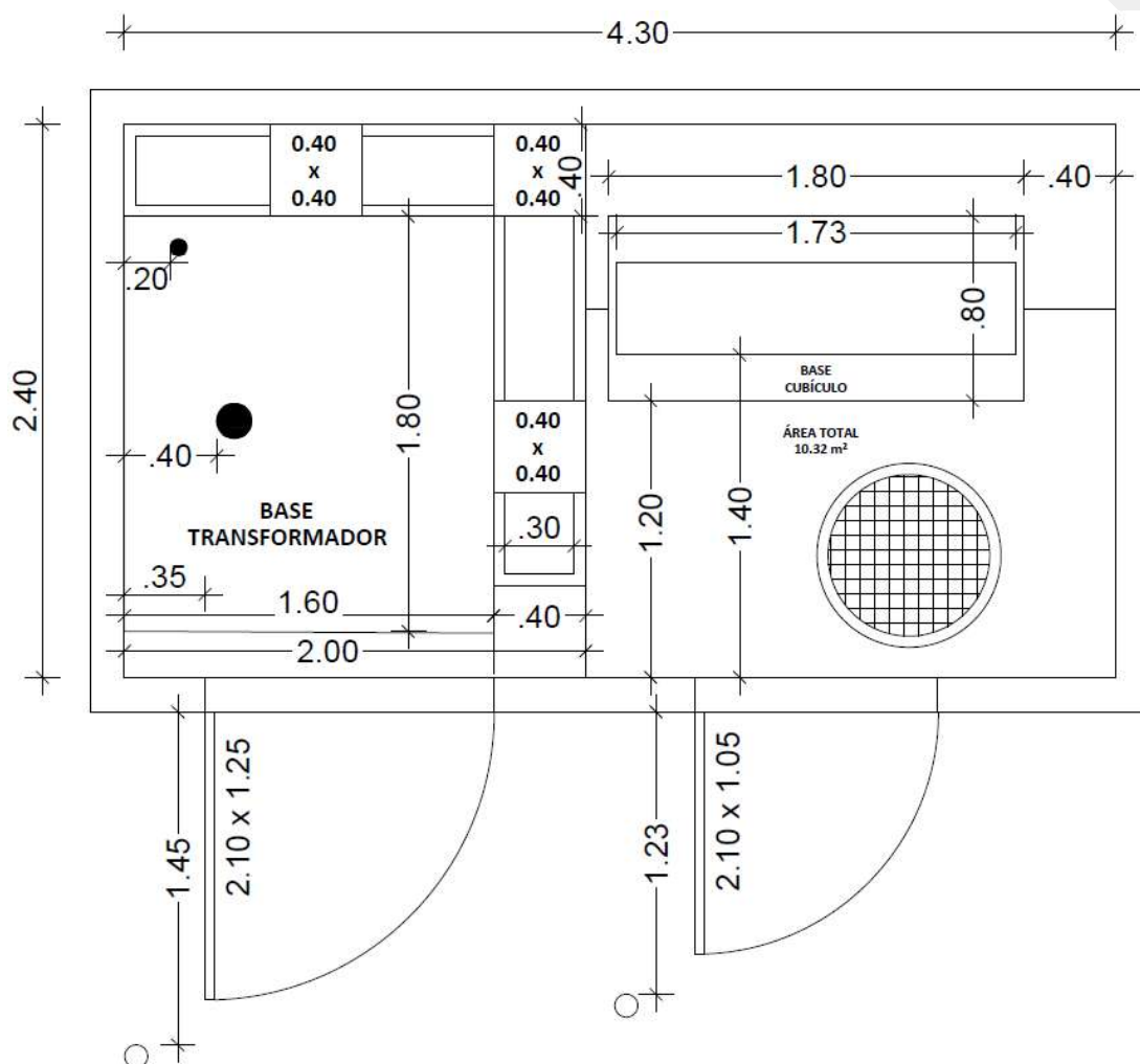
Desenho 8 - CTE para 1 Transformador de até 225 kVA - 1/9 (CTE-R-225/CTE-225-RE+P/ CTE-225-RE+2P/ CTE-225-RE+3P)
