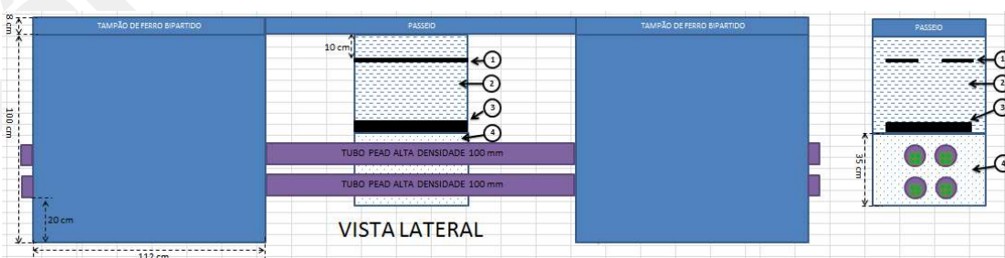
Eletroduto de polietileno de alta densidade (PEAD) em passeio
