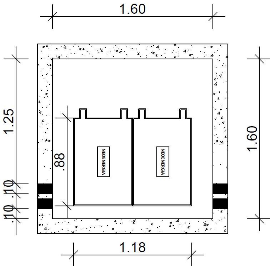
Desenho 17 - Poço Secundário (PS3) - 1/3
