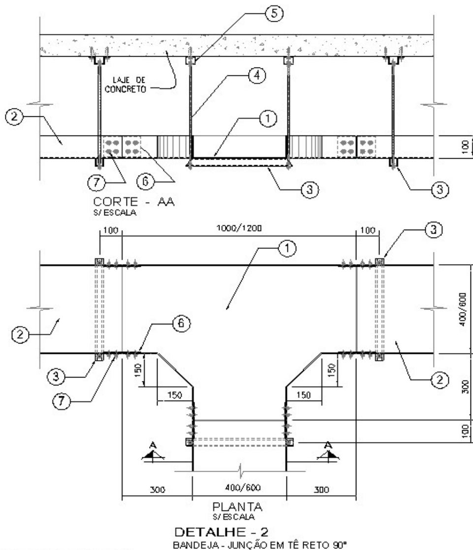
Desenho 51 – Trecho de Bandeja com Junção em T
