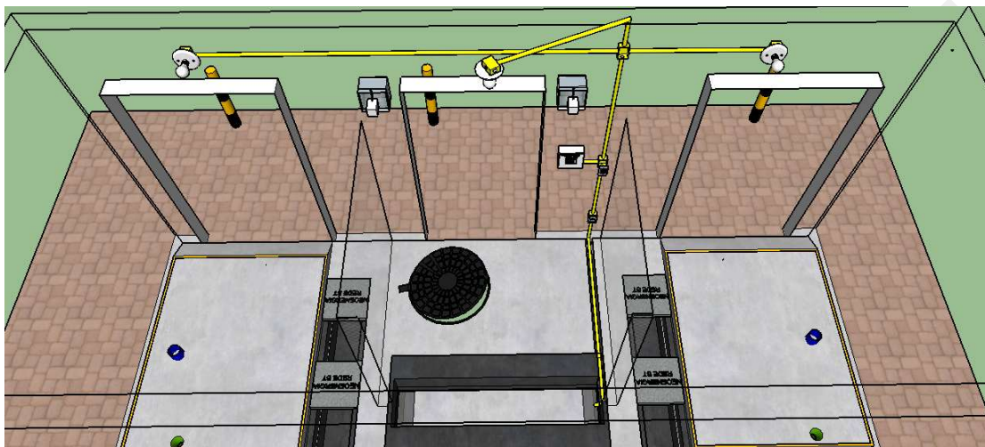
Desenho 20 - Disposição Pontos de Iluminação e Tomada - 1/3
