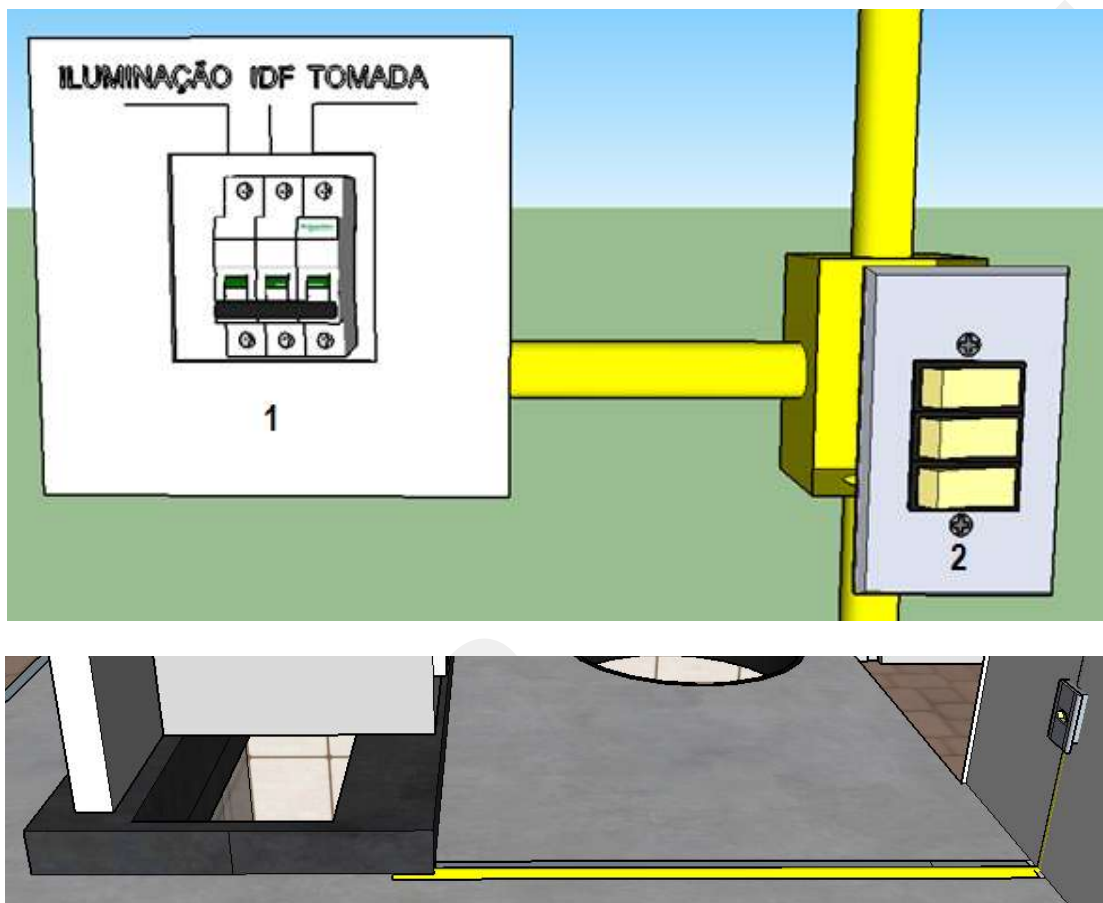
Desenho 20 - Disposição Pontos de Iluminação e Tomada - 2/3
