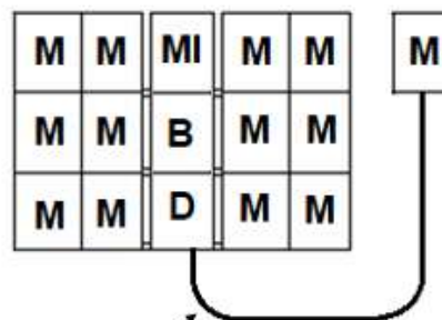
6 - CENTRO DE MEDIÇÃO RESIDENCIAL COM CAIXA INDIVIDUAL PARA MEDIÇÃO DO SERVIÇO
