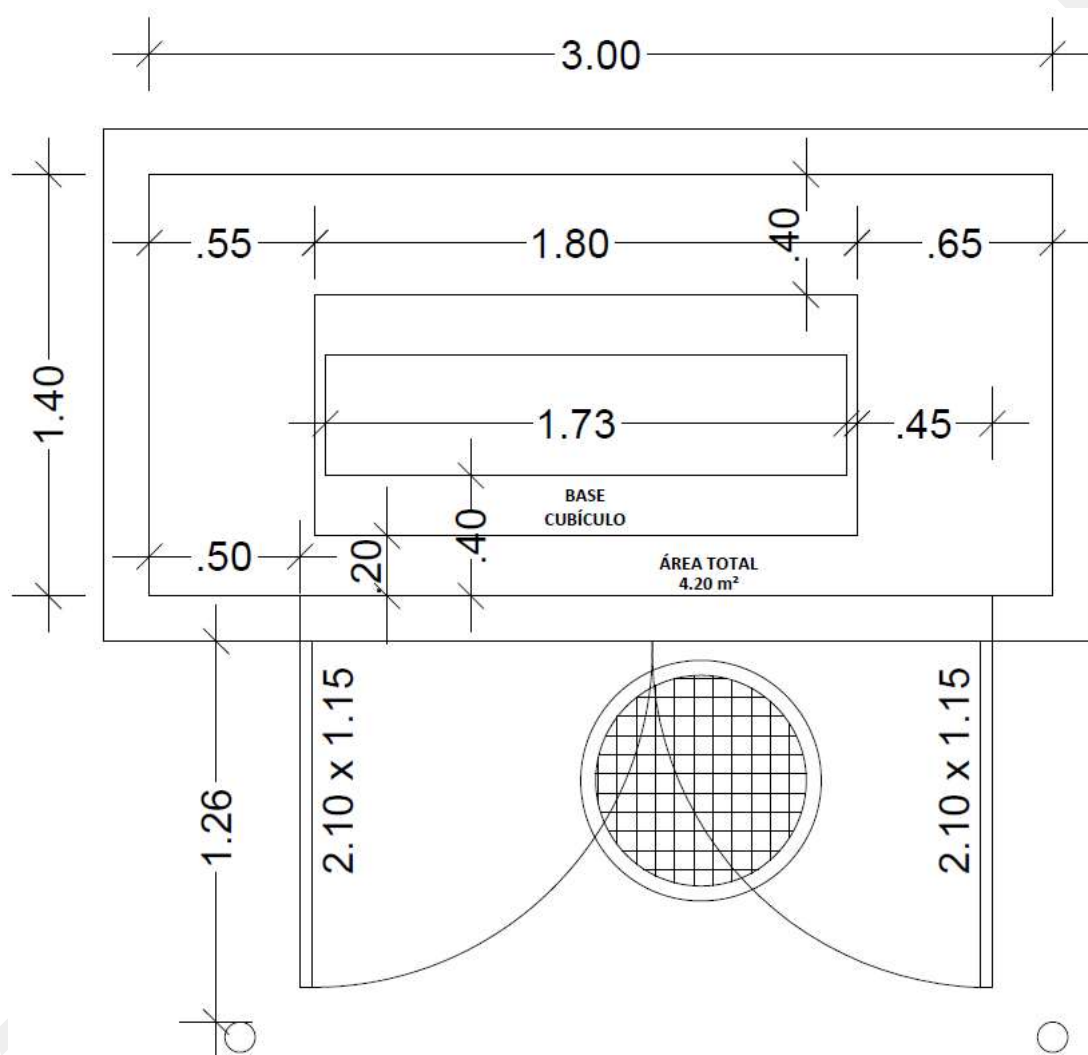
Desenho 14 - Câmara de Manobra - 1/7 (CM-R-RE+2P/ CM-R-RE+3P/CM-A-3L/ CM-A-4L)
