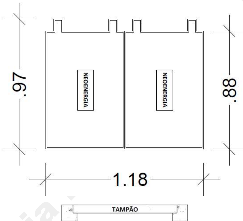
Desenho 18 - Poço Primário (PP) - 15 kV - 1/6
