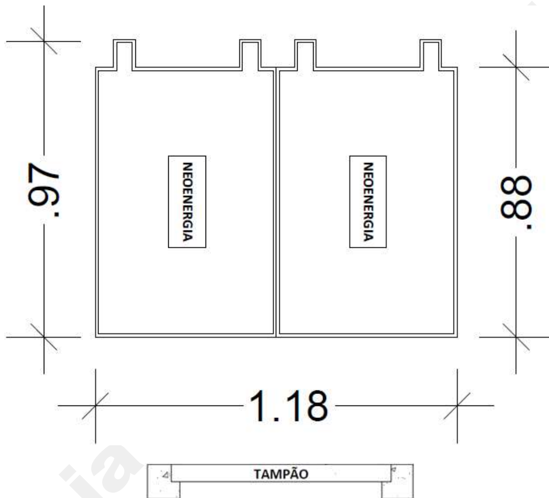
Desenho 15 - Poço Secundário (PS1) - 1/7
