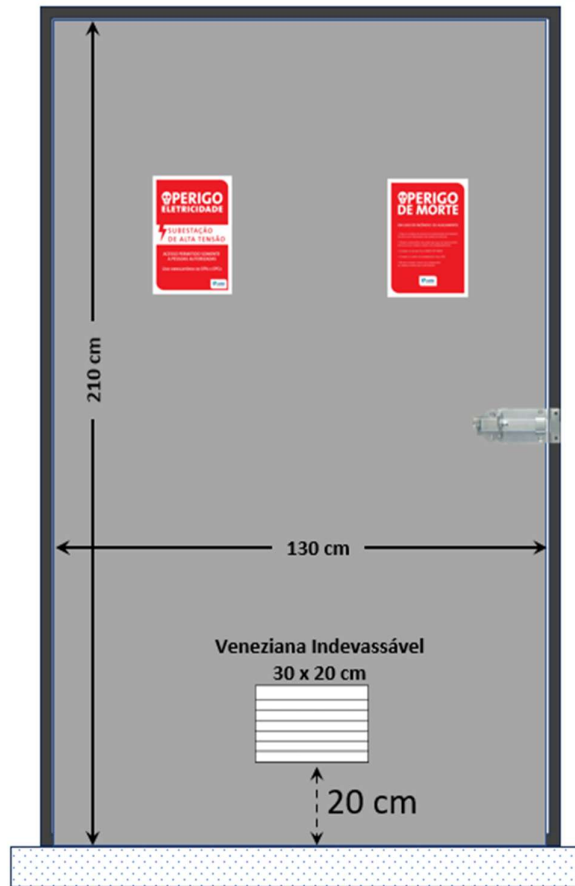
Porta acesso para pessoas: CM 15/34,5 kV
