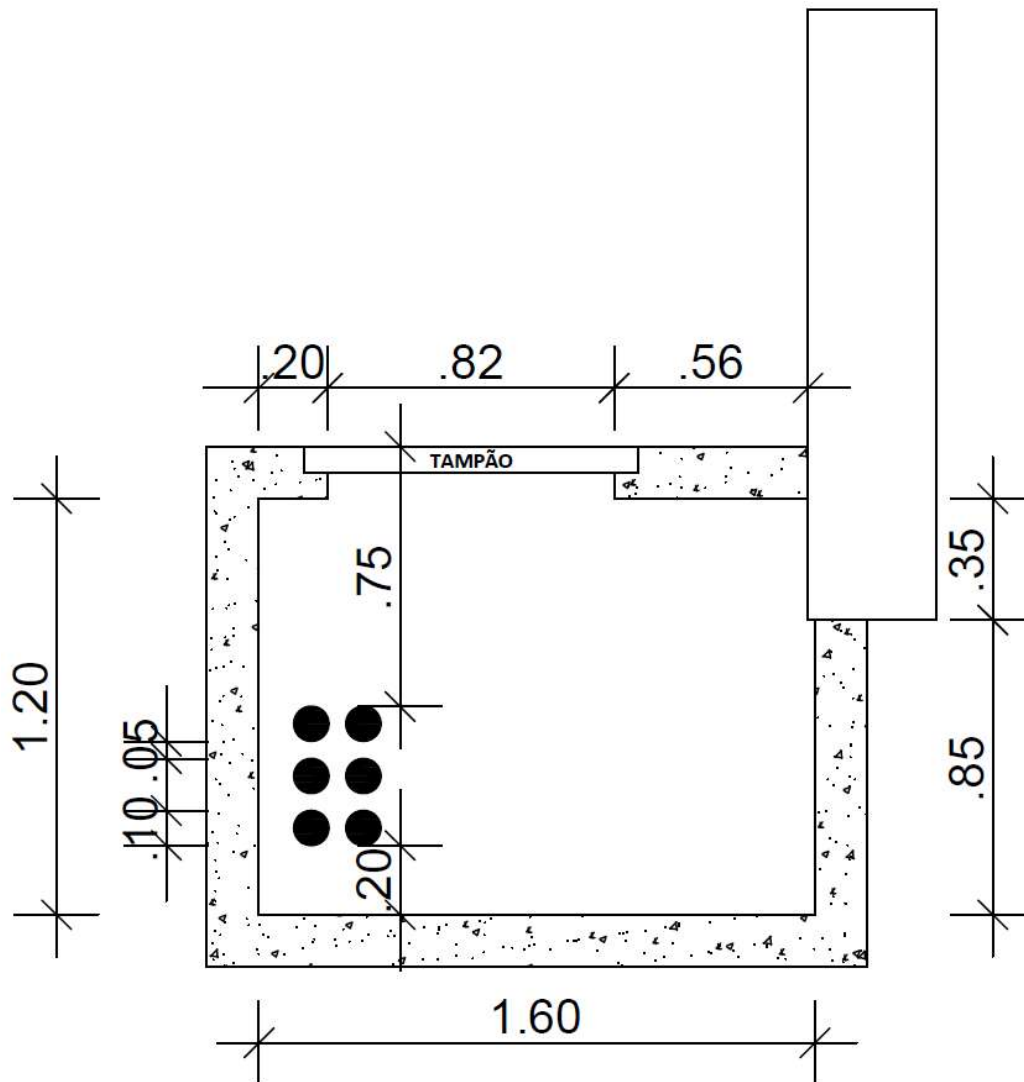
Desenho 17 - Poço Secundário (PS3) - 2/3
