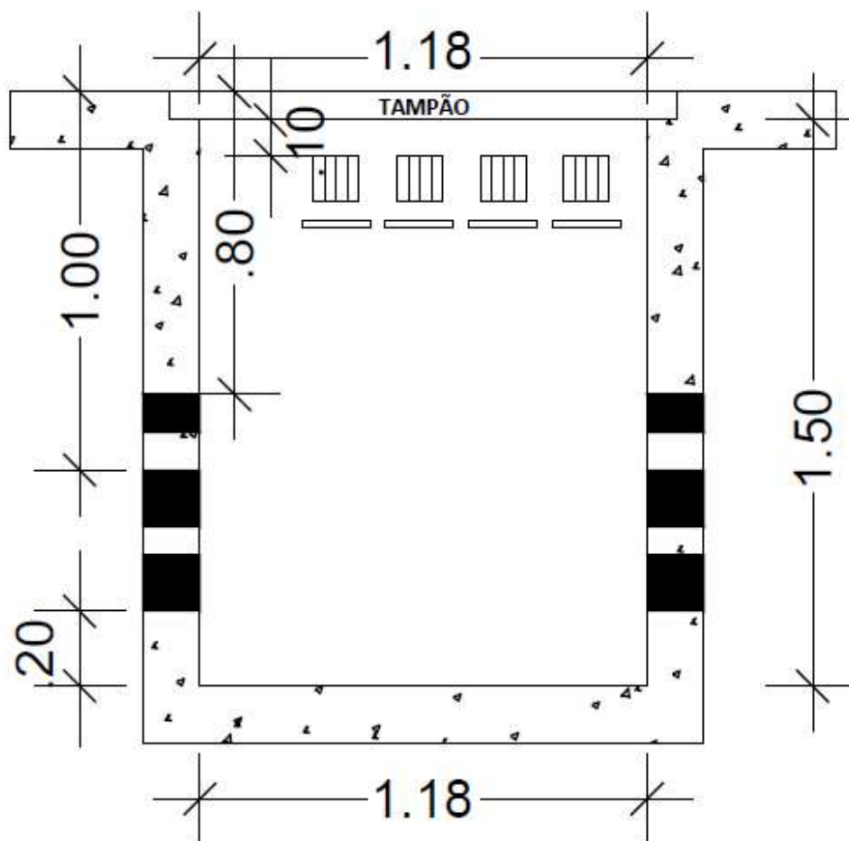
Desenho 18 - Poço Primário (PP) - 15 kV - 2/6
