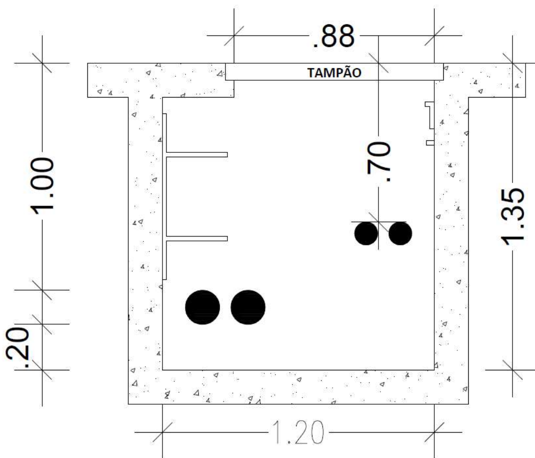
Desenho 19 - Poço Primário (PE) - 15 kV - 3/7
