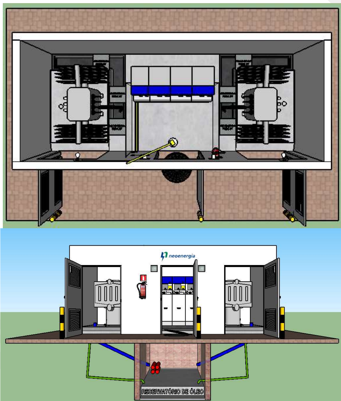
Desenho 11 - CTE para 2 Transformadores de até 225 kVA - 4/8 (CTE-R-450-RE+2P/ CTE-R-450-RE+3P/CTE-A-2L+P)
