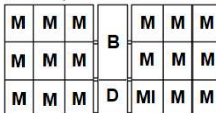
5 - CENTRO DE MEDIÇÃO PARA 20 MEDIDORES RESIDENCIAIS
