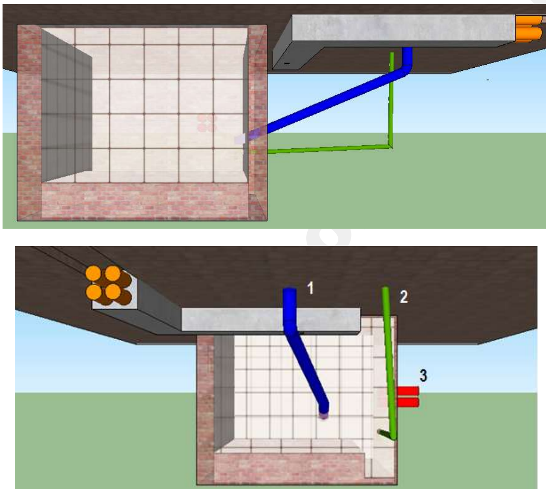
Desenho 8 - CTE para 1 Transformador de até 225 kVA - 9/9 (CTE-R-225/CTE-225-RE+P/ CTE-225-RE+2P/ CTE-225-RE+3P)
