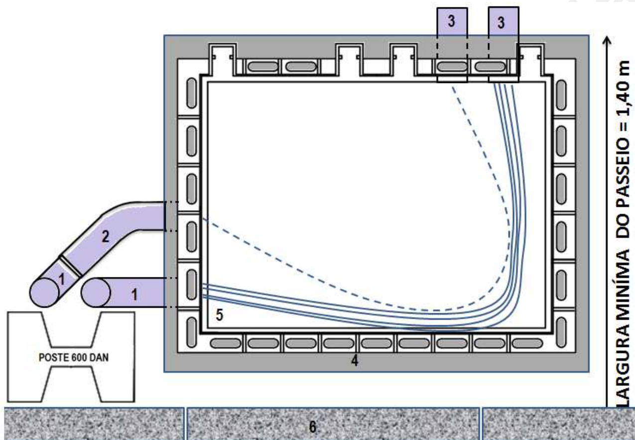
Desenho 25 - Representação Descida do Poste com Poço PS1 para Rede de BT
