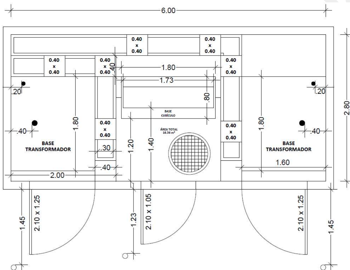
Desenho 10 - CTE para 2 Transformadores de até 225 kVA - 1/8 (CTE-R-450-RE+2P/ CTE-R-450-RE+3P/CTE-A-2L+P)
