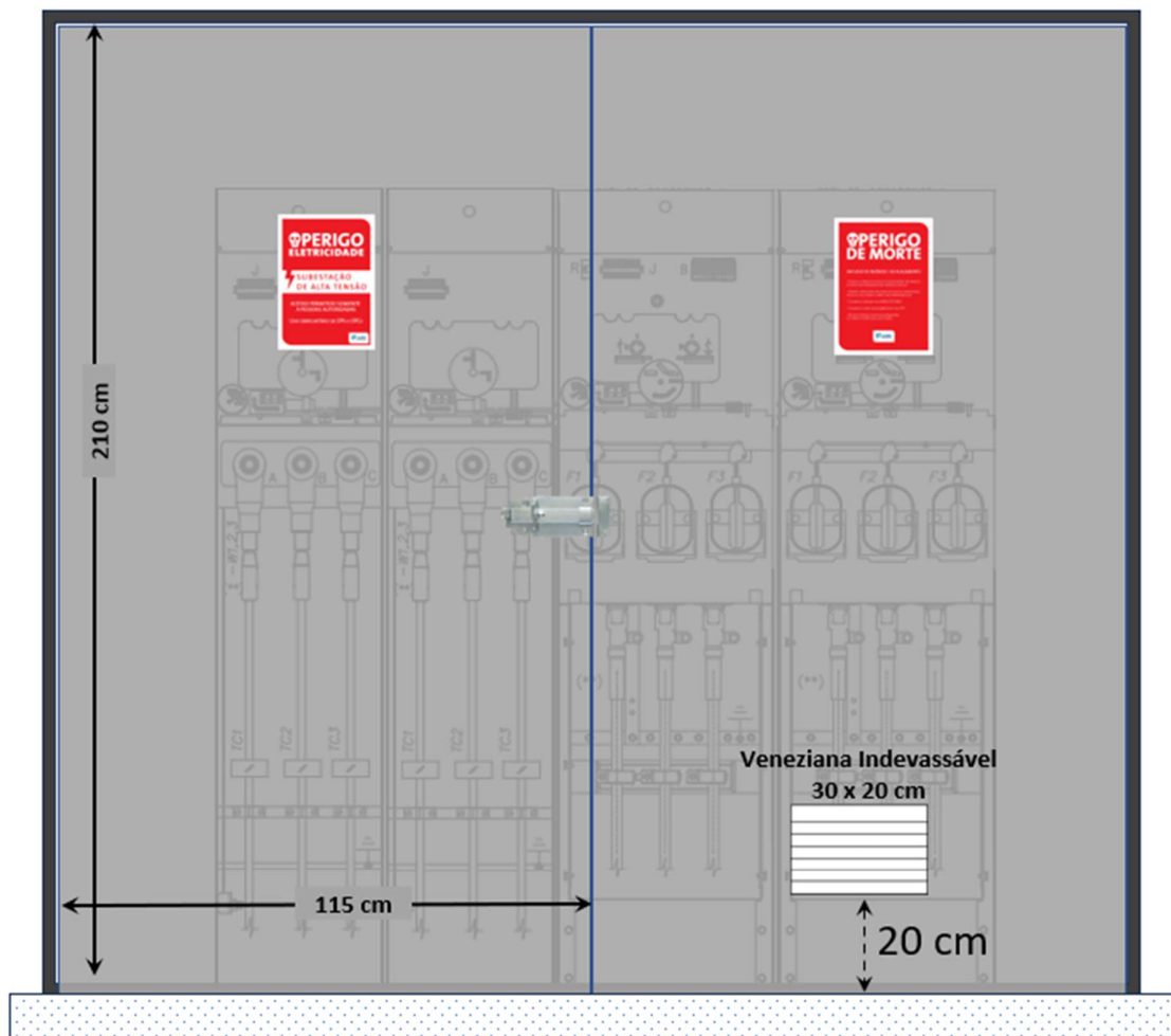
Porta acesso para câmara de manobra com operação externa 15/34,5 kV
